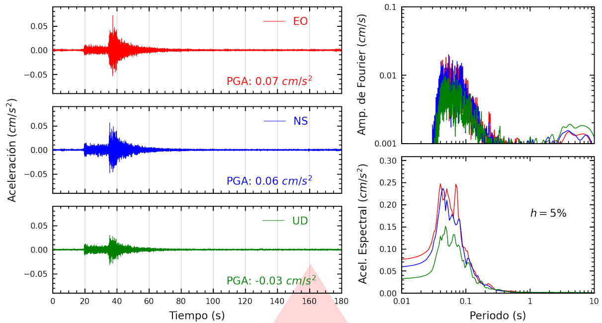
Figura A.1: Registros tiempo-historia, espectros de Fourier y de respuesta en las direcciones EO, NS y vertical de la estación UNSA2. Sismo de Moquegua, Mariscal Nieto - Moquegua del 2026-07-09, 07:27:18 (Hora local)
