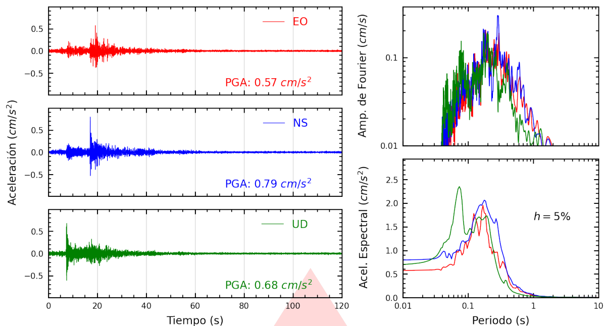
Figura A.1: Registros tiempo-historia, espectros de Fourier y de respuesta en las direcciones EO, NS y vertical de la estación UNICA. Sismo de Ica, Ica - Ica del 2026-07-13, 21:55:03 (Hora local)
