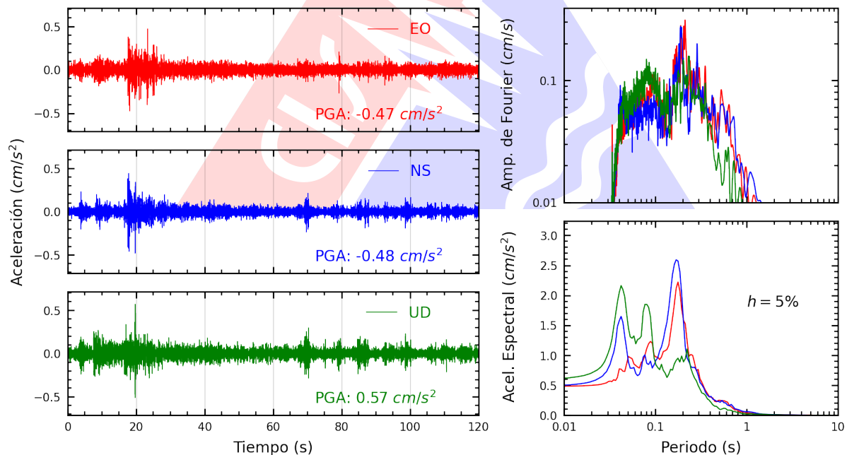
Figura A.2: Registros tiempo-historia, espectros de Fourier y de respuesta en las direcciones EO, NS y vertical de la estación SCICA. Sismo de Ica, Ica - Ica del 2026-07-13, 21:55:03 (Hora local)
