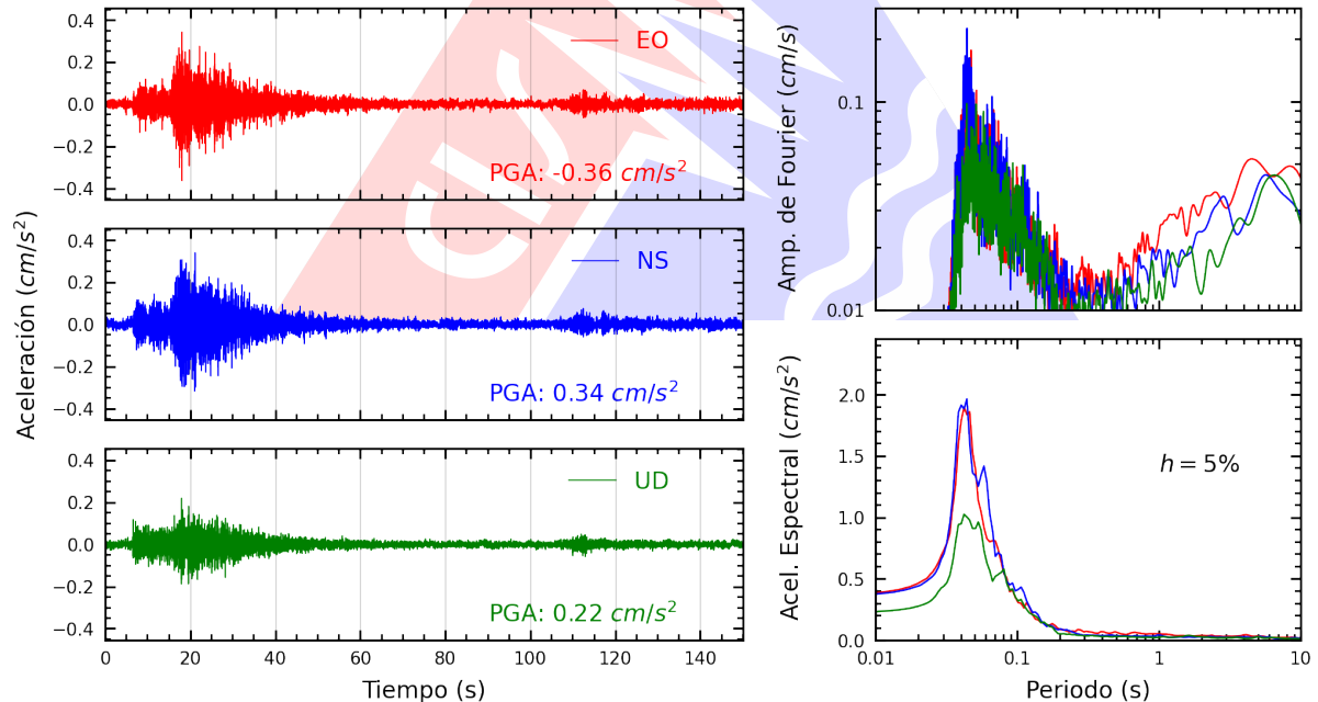
Figura A.2: Registros tiempo-historia, espectros de Fourier y de respuesta en las direcciones EO, NS y vertical de la estación UNAB. Sismo de Huacho, Huaura - Lima del 2026-07-14, 21:11:33 (Hora local)
