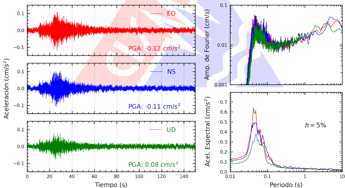
Figura A.6: Registros tiempo-historia, espectros de Fourier y de respuesta en las direcciones EO, NS y vertical de la estación UCSS. Sismo de Huacho, Huaura - Lima del 2026-07-14, 21:11:33 (Hora local)
