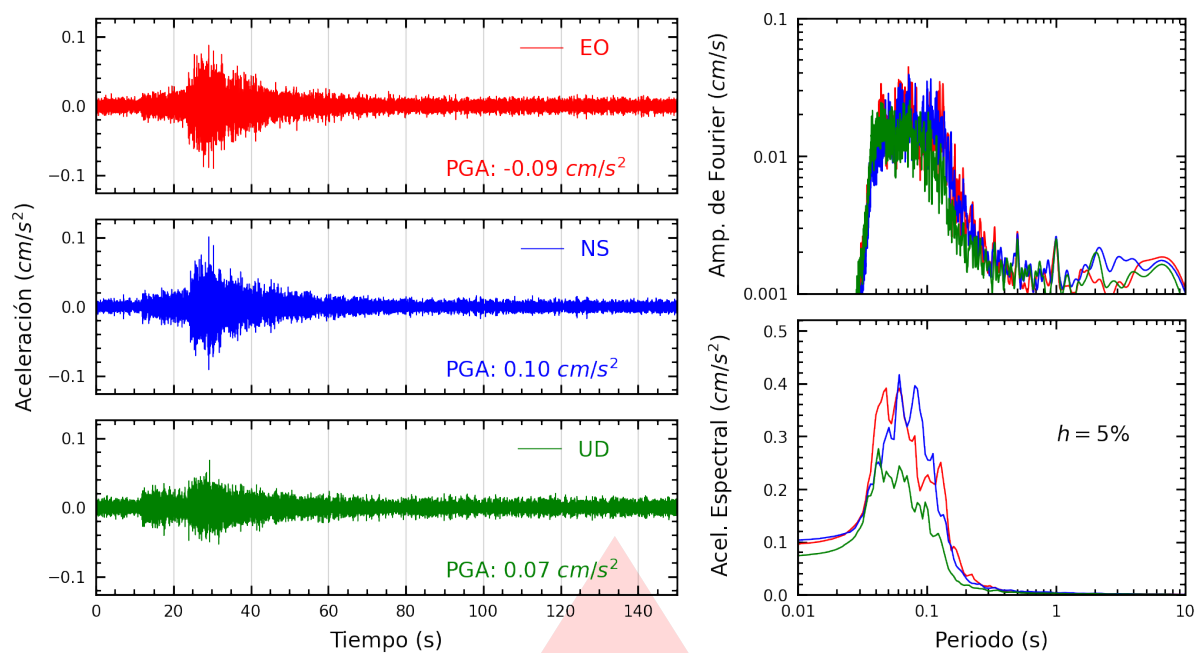
Figura A.7: Registros tiempo-historia, espectros de Fourier y de respuesta en las direcciones EO, NS y vertical de la estación ATARJ. Sismo de Huacho, Huaura - Lima del 2026-07-14, 21:11:33 (Hora local)
