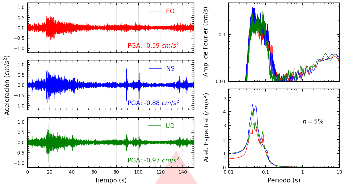
Figura A.1: Registros tiempo-historia, espectros de Fourier y de respuesta en las direcciones EO, NS y vertical de la estación SROSA. Sismo de Huacho, Huaura - Lima del 2026-07-14, 21:11:33 (Hora local)
