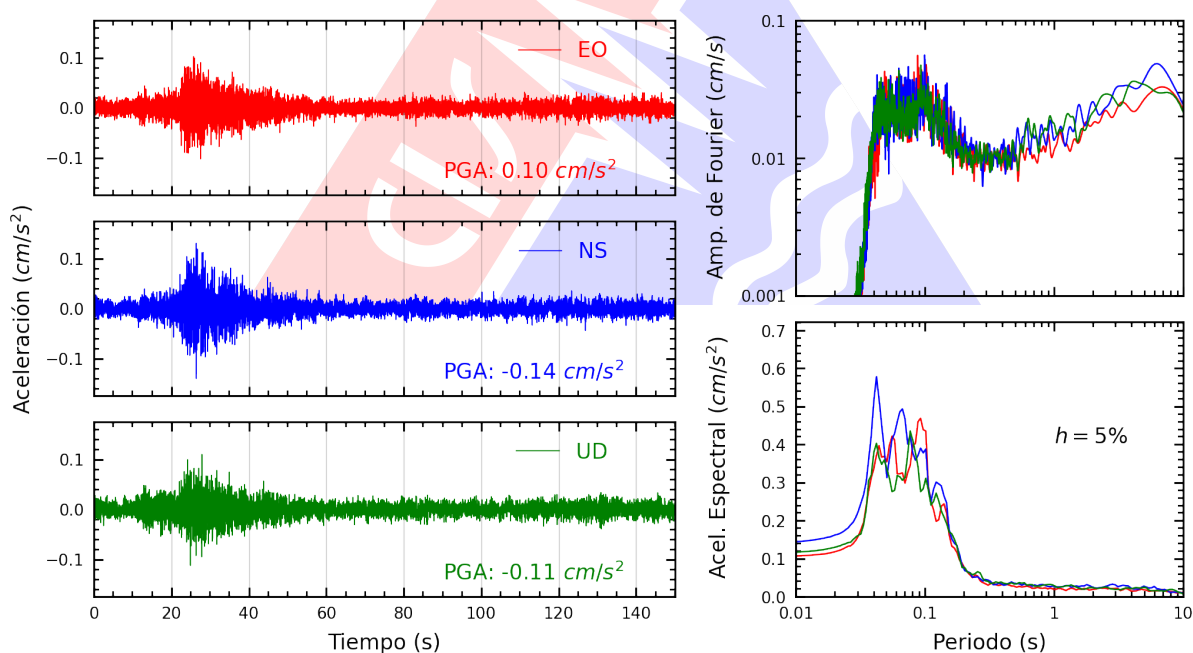
Figura A.4: Registros tiempo-historia, espectros de Fourier y de respuesta en las direcciones EO, NS y vertical de la estación JALVA. Sismo de Huacho, Huaura - Lima del 2026-07-14, 21:11:33 (Hora local)
