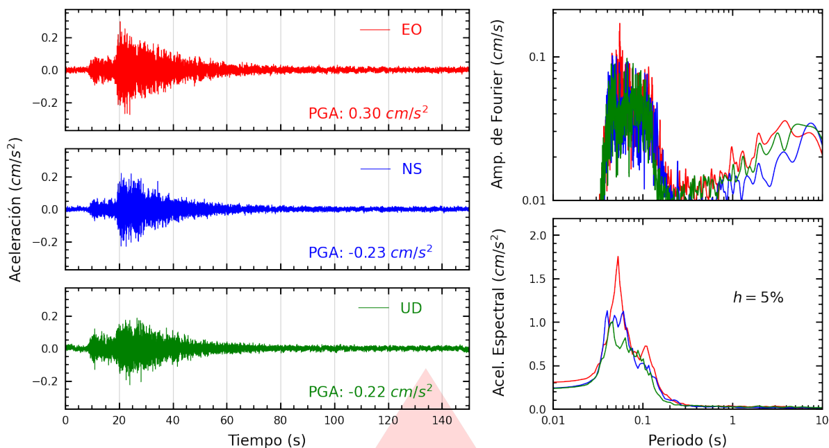
Figura A.3: Registros tiempo-historia, espectros de Fourier y de respuesta en las direcciones EO, NS y vertical de la estación AMORE. Sismo de Huacho, Huaura - Lima del 2026-07-14, 21:11:33 (Hora local)
