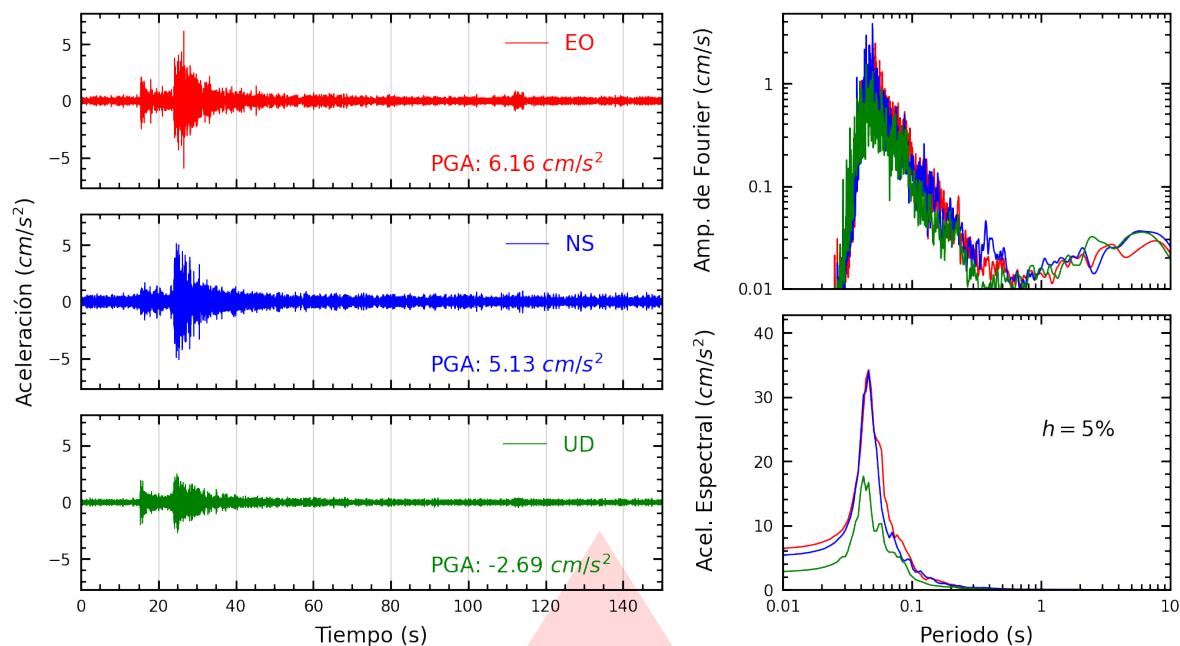
Figura A.1: Registros tiempo-historia, espectros de Fourier y de respuesta en las direcciones EO, NS y vertical de la estación USP. Sismo de Chimbote, Santa - Áncash del 2026-07-14, 21:28:42 (Hora local)
