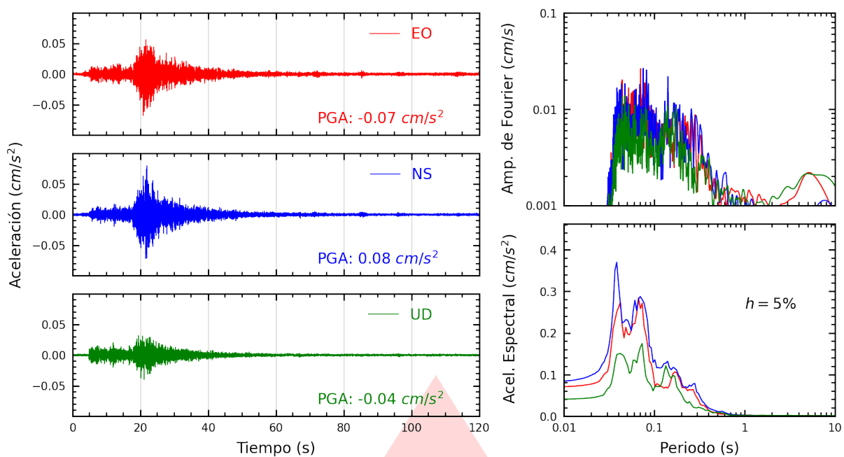
Figura A.1: Registros tiempo-historia, espectros de Fourier y de respuesta en las direcciones EO, NS y vertical de la estación UNSA2. Sismo de Aplao, Castilla - Arequipa del 2026-07-16, 07:27:36 (Hora local)
