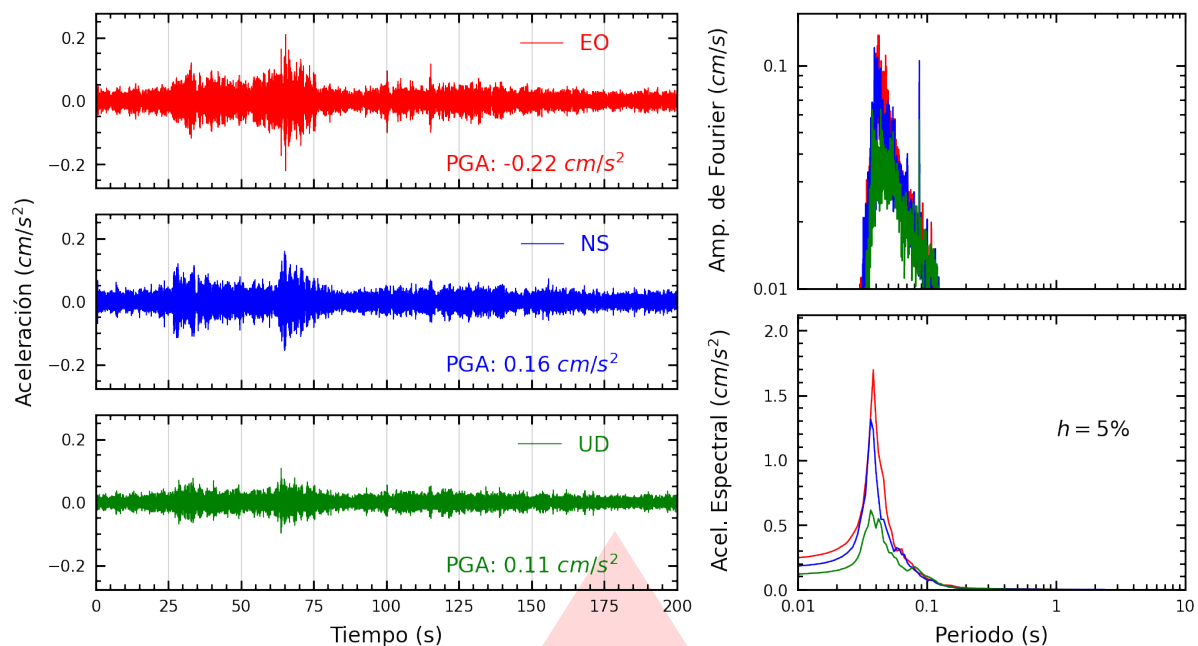
Figura A.1: Registros tiempo-historia, espectros de Fourier y de respuesta en las direcciones EO, NS y vertical de la estación BORJA. Sismo de Marcona, Nasca - Ica del 2026-07-16, 11:38:09 (Hora local)
