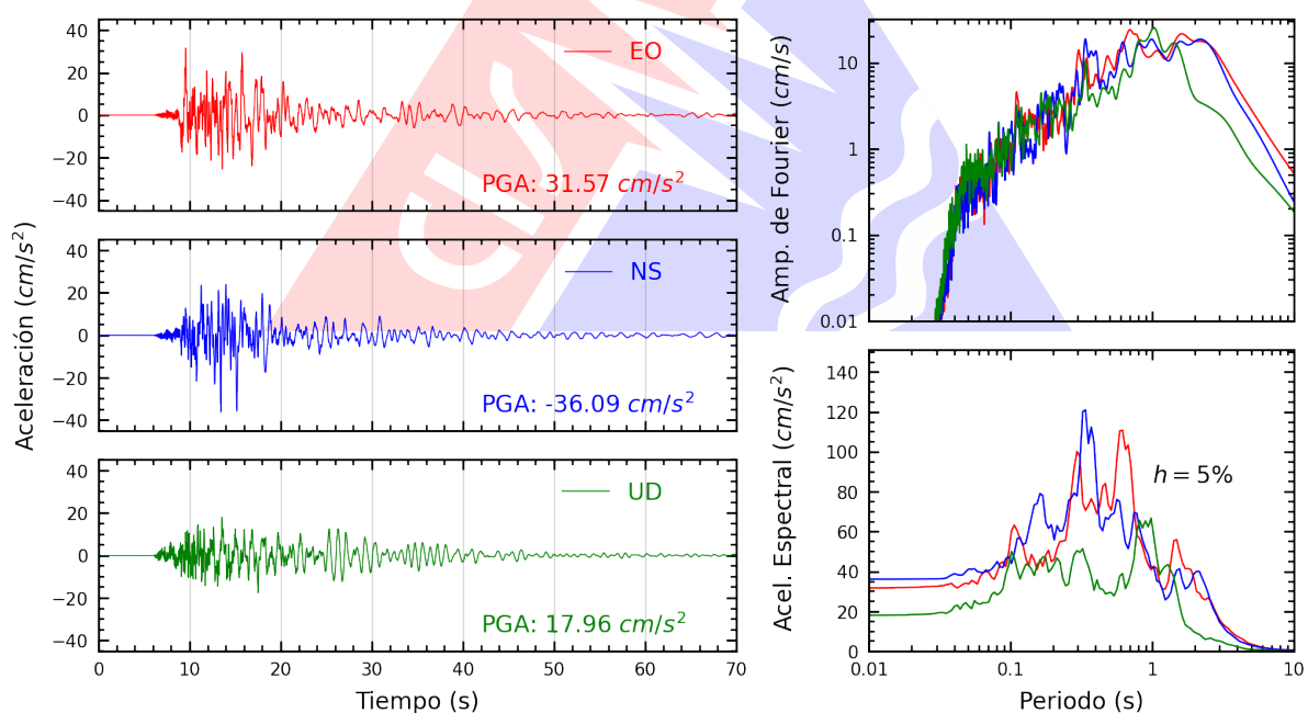
Figura A.2: Registros tiempo-historia, espectros de Fourier y de respuesta en las direcciones EO, NS y vertical de la estación UNCP. Sismo de Chupaca, Chupaca - Junín del 2026-07-18, 21:24:34 (Hora local)
