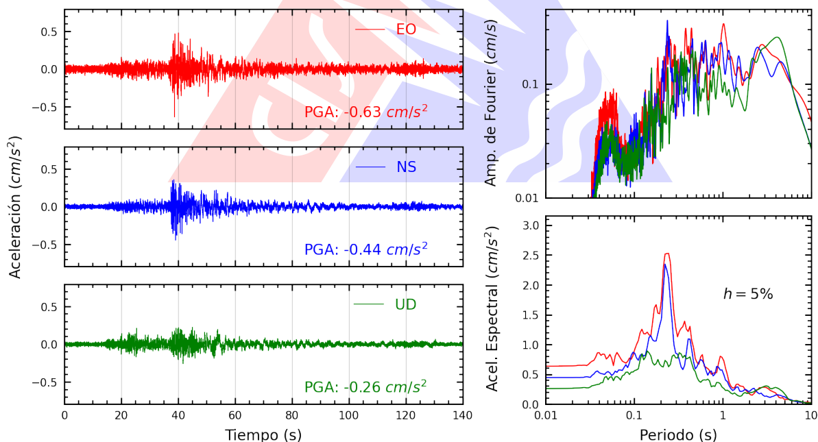
Figura A.26: Registros tiempo-historia, espectros de Fourier y de respuesta en las direcciones EO, NS y vertical de la estación INICT. Sismo de Chupaca, Chupaca - Junín del 2026-07-18, 21:24:34 (Hora local)
