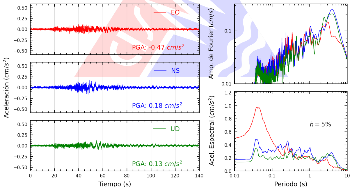
Figura A.30: Registros tiempo-historia, espectros de Fourier y de respuesta en las direcciones EO, NS y vertical de la estación SJLCE. Sismo de Chupaca, Chupaca - Junín del 2026-07-18, 21:24:34 (Hora local)
