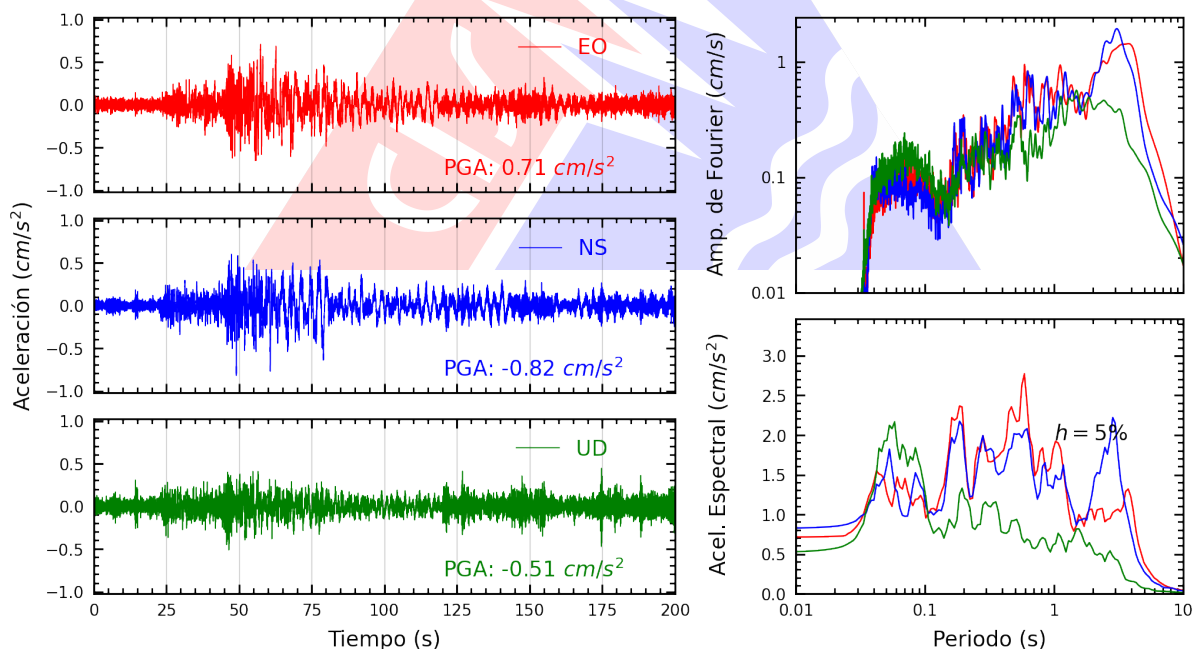
Figura A.18: Registros tiempo-historia, espectros de Fourier y de respuesta en las direcciones EO, NS y vertical de la estación SCICA. Sismo de Chupaca, Chupaca - Junín del 2026-07-18, 21:24:34 (Hora local)
