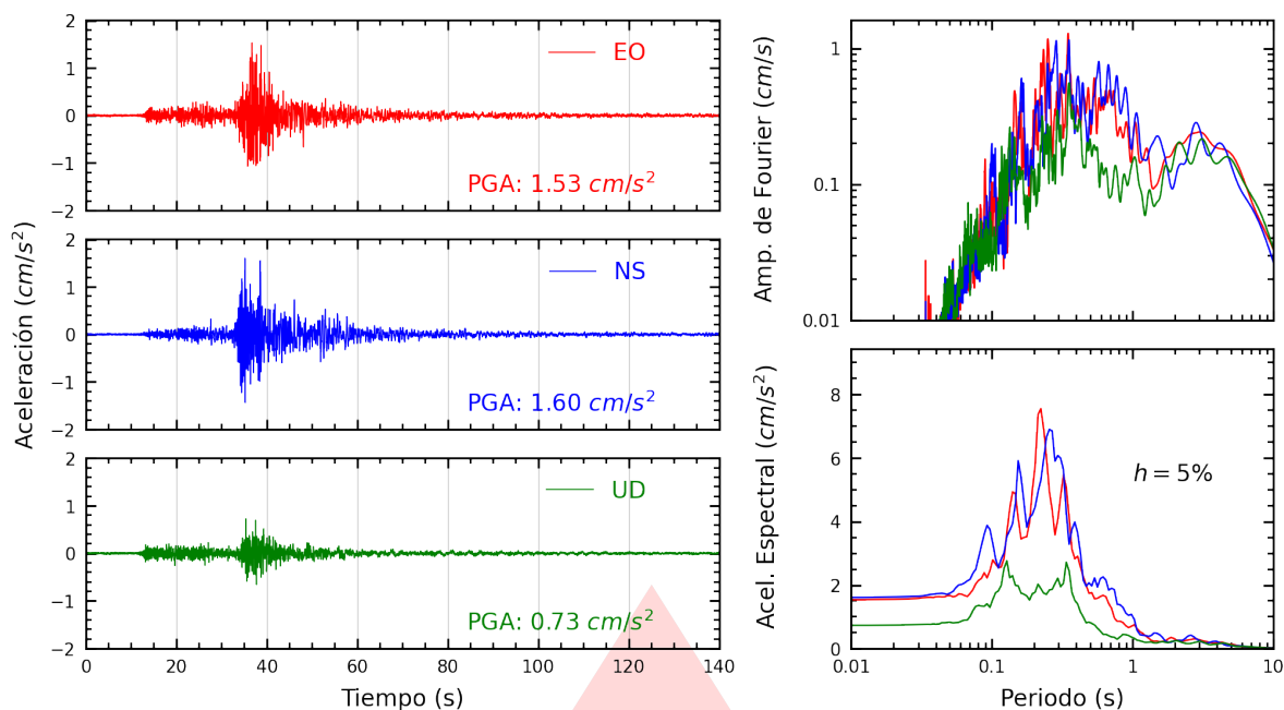
Figura A.7: Registros tiempo-historia, espectros de Fourier y de respuesta en las direcciones EO, NS y vertical de la estación USILP. Sismo de Chupaca, Chupaca - Junín del 2026-07-18, 21:24:34 (Hora local)
