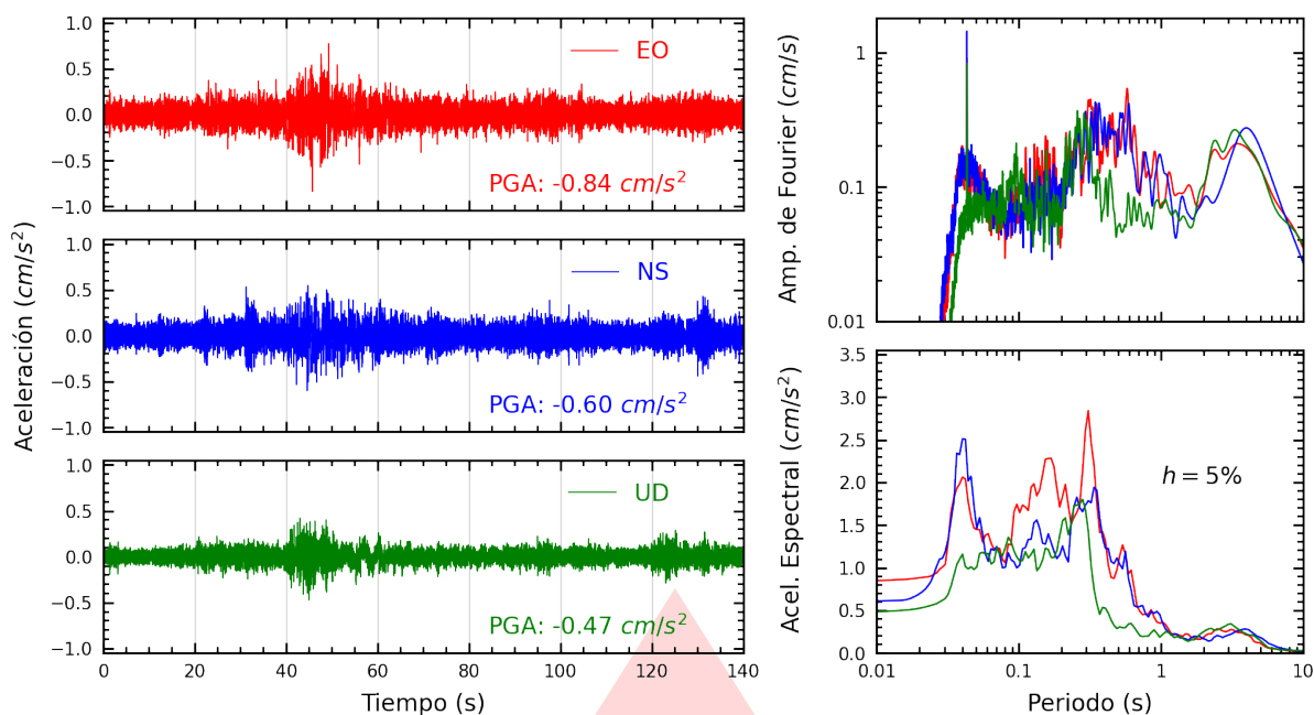
Figura A.17: Registros tiempo-historia, espectros de Fourier y de respuesta en las direcciones EO, NS y vertical de la estación OLIVO. Sismo de Chupaca, Chupaca - Junín del 2026-07-18, 21:24:34 (Hora local)
