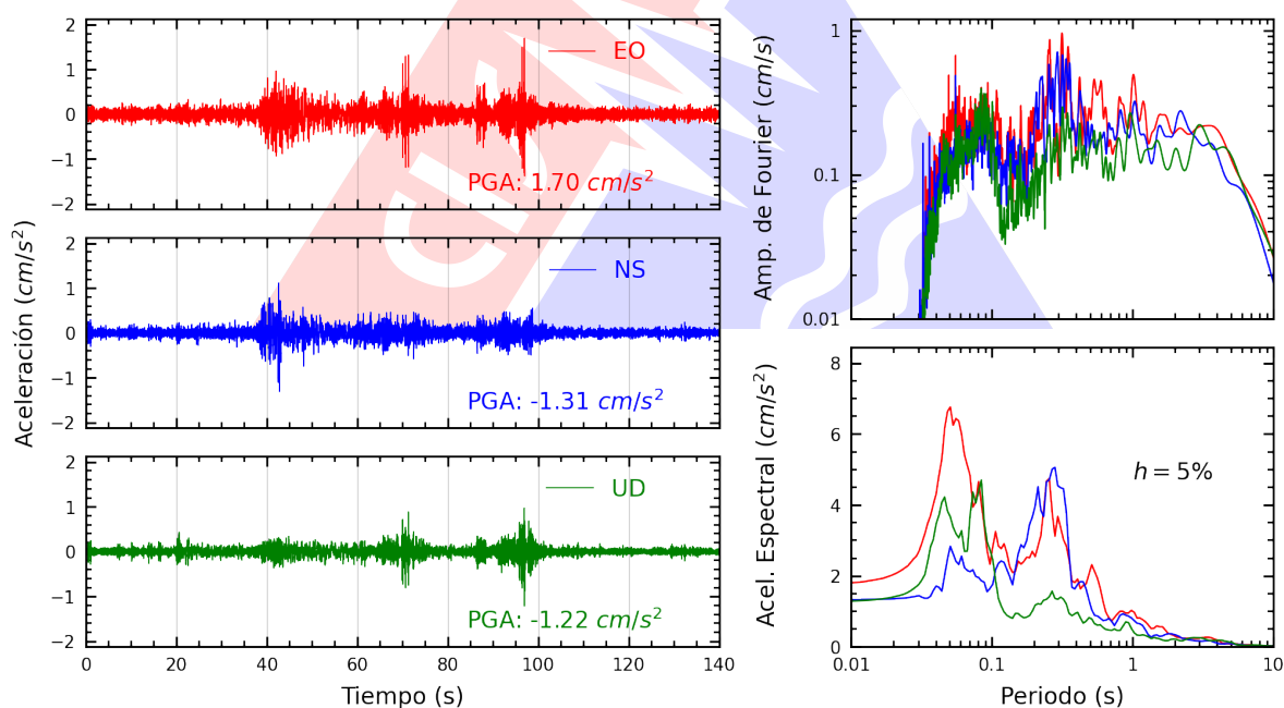
Figura A.6: Registros tiempo-historia, espectros de Fourier y de respuesta en las direcciones EO, NS y vertical de la estación SOBAR. Sismo de Chupaca, Chupaca - Junín del 2026-07-18, 21:24:34 (Hora local)
