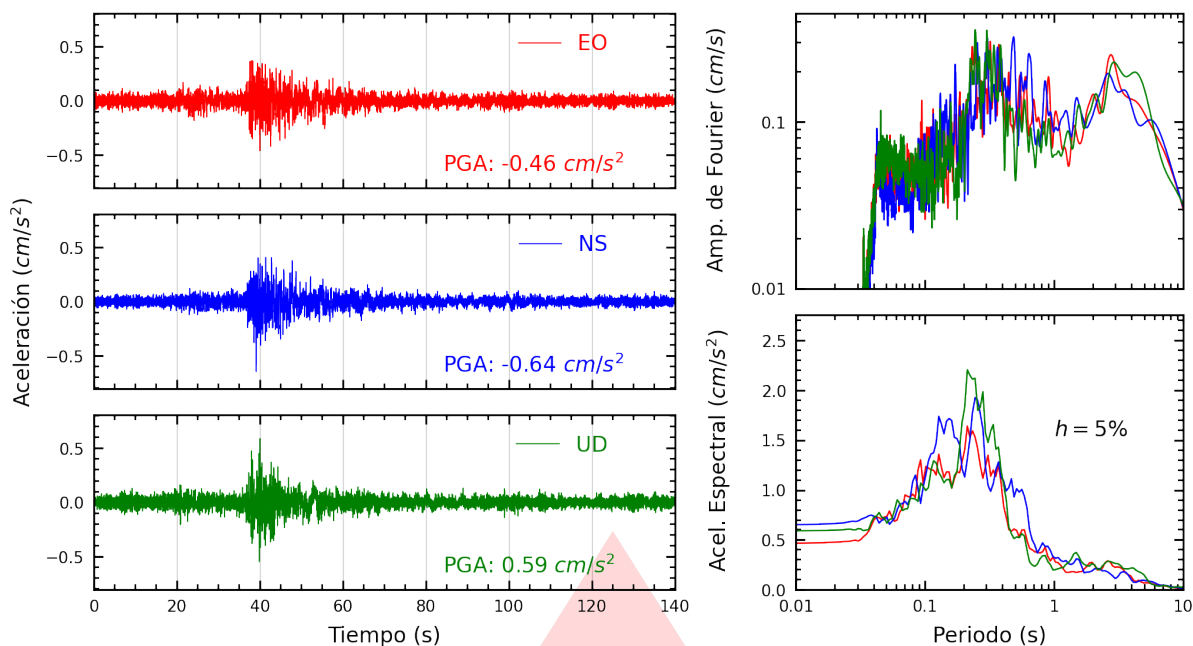
Figura A.25: Registros tiempo-historia, espectros de Fourier y de respuesta en las direcciones EO, NS y vertical de la estación URPE. Sismo de Chupaca, Chupaca - Junín del 2026-07-18, 21:24:34 (Hora local)
