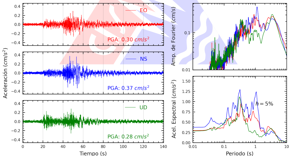
Figura A.38: Registros tiempo-historia, espectros de Fourier y de respuesta en las direcciones EO, NS y vertical de la estación BONDY. Sismo de Chupaca, Chupaca - Junín del 2026-07-18, 21:24:34 (Hora local)
