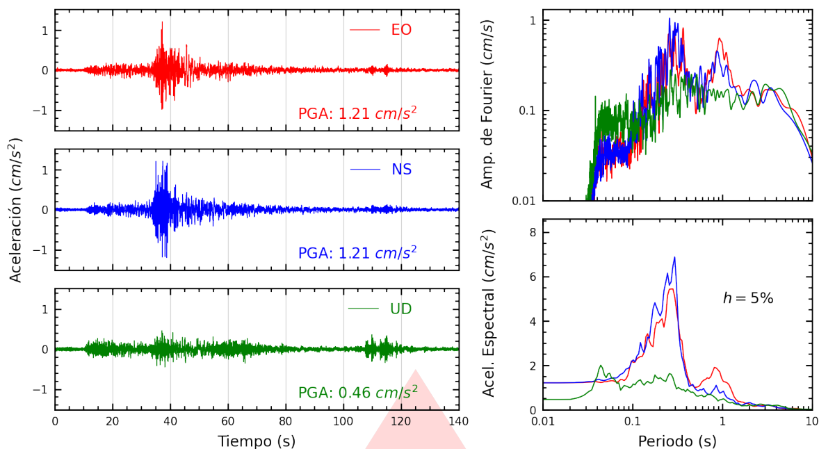
Figura A.13: Registros tiempo-historia, espectros de Fourier y de respuesta en las direcciones EO, NS y vertical de la estación SOCHO. Sismo de Chupaca, Chupaca - Junín del 2026-07-18, 21:24:34 (Hora local)
