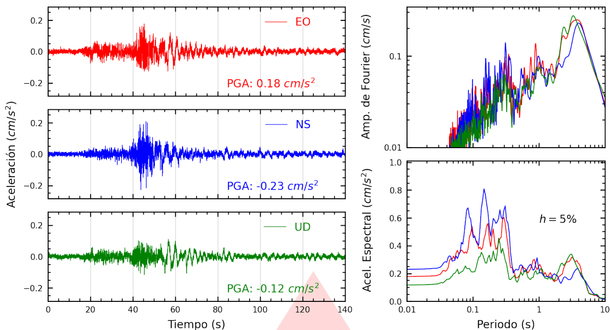
Figura A.43: Registros tiempo-historia, espectros de Fourier y de respuesta en las direcciones EO, NS y vertical de la estación UCSS. Sismo de Chupaca, Chupaca - Junín del 2026-07-18, 21:24:34 (Hora local)
