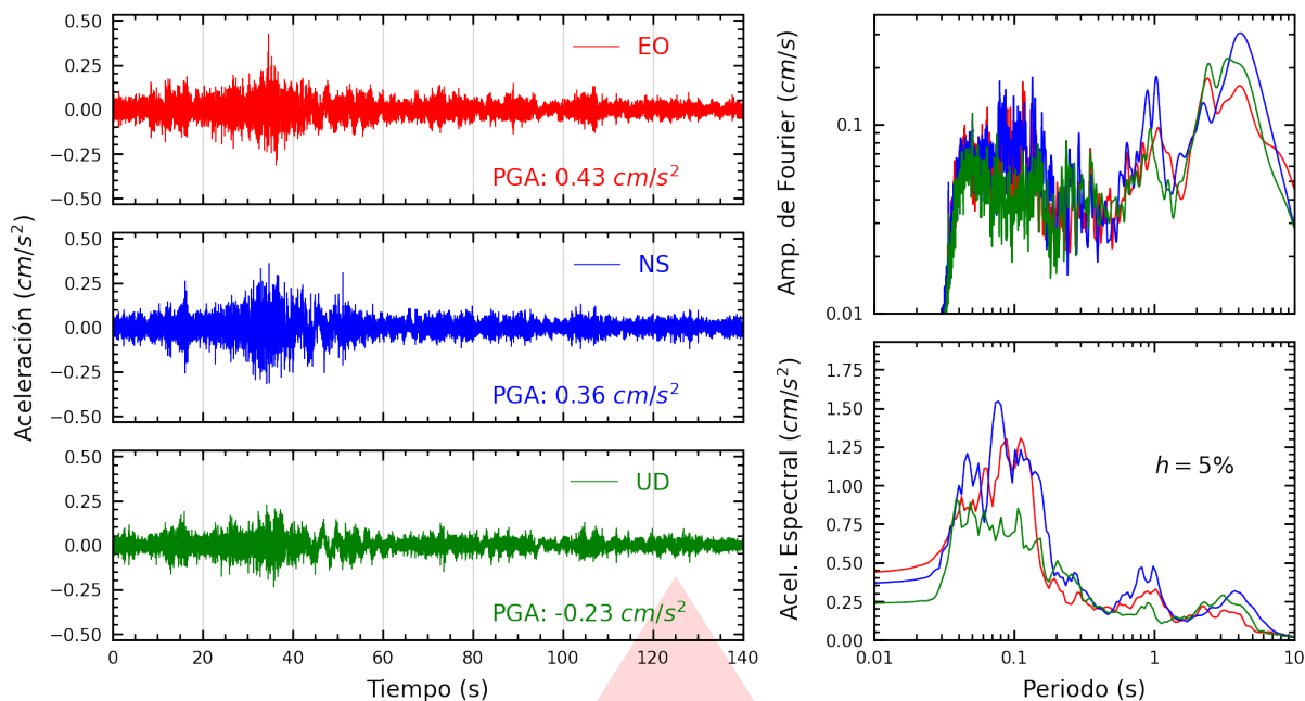
Figura A.33: Registros tiempo-historia, espectros de Fourier y de respuesta en las direcciones EO, NS y vertical de la estación JOSEO. Sismo de Chupaca, Chupaca - Junín del 2026-07-18, 21:24:34 (Hora local)
