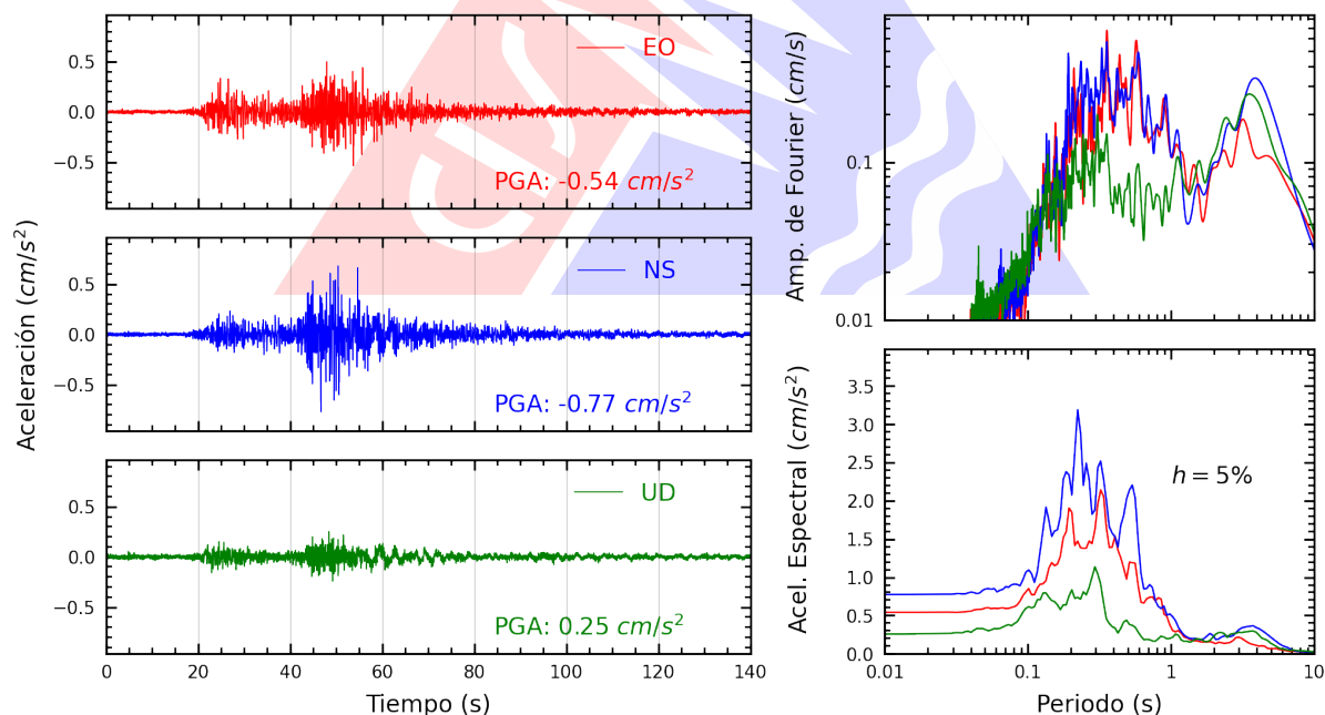
Figura A.20: Registros tiempo-historia, espectros de Fourier y de respuesta en las direcciones EO, NS y vertical de la estación VHAYA. Sismo de Chupaca, Chupaca - Junín del 2026-07-18, 21:24:34 (Hora local)
