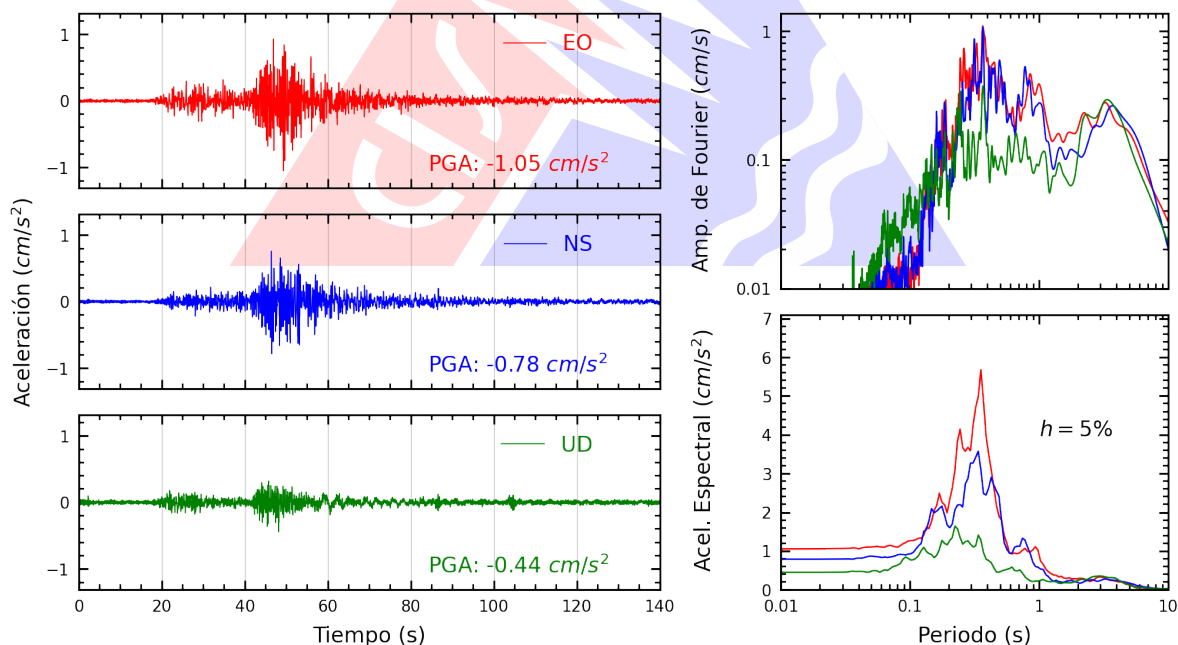
Figura A.14: Registros tiempo-historia, espectros de Fourier y de respuesta en las direcciones EO, NS y vertical de la estación ACAPU. Sismo de Chupaca, Chupaca - Junín del 2026-07-18, 21:24:34 (Hora local)
