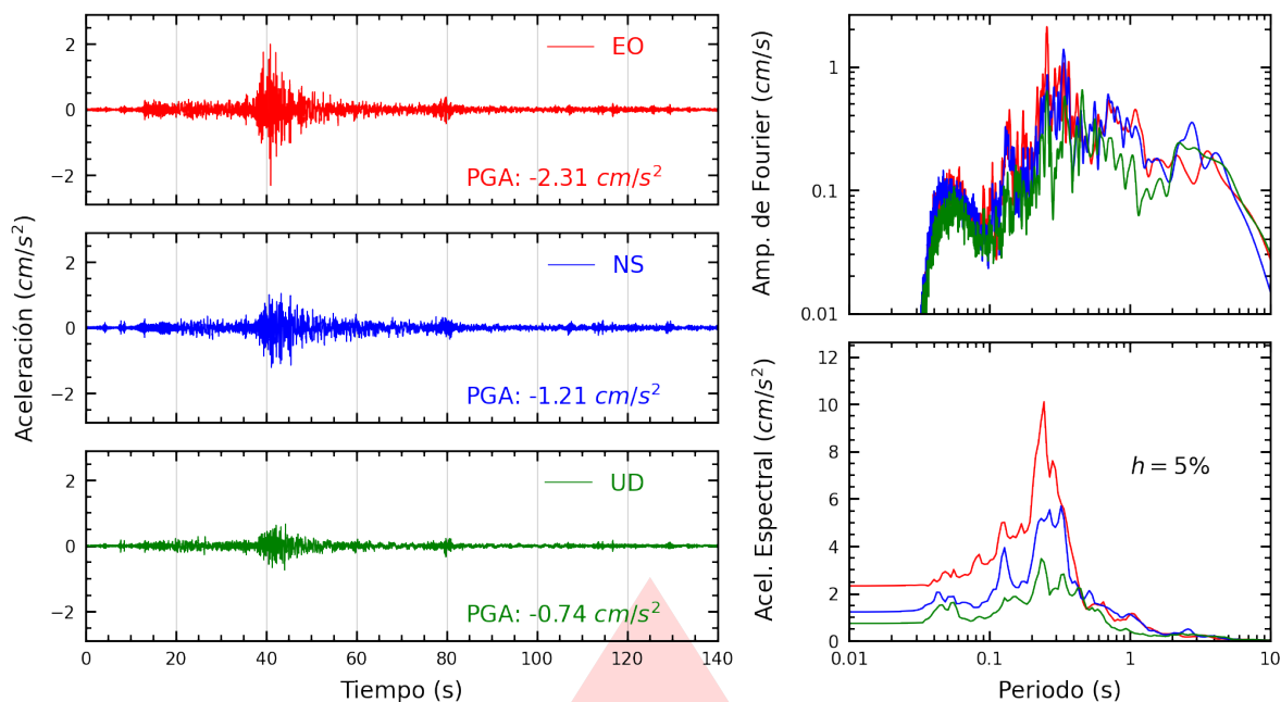
Figura A.3: Registros tiempo-historia, espectros de Fourier y de respuesta en las direcciones EO, NS y vertical de la estación BRISA. Sismo de Chupaca, Chupaca - Junín del 2026-07-18, 21:24:34 (Hora local)
