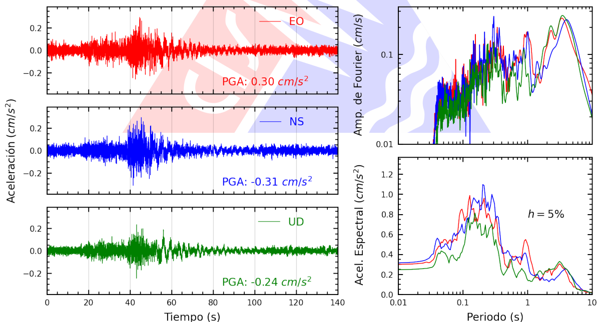
Figura A.42: Registros tiempo-historia, espectros de Fourier y de respuesta en las direcciones EO, NS y vertical de la estación FICPE. Sismo de Chupaca, Chupaca - Junín del 2026-07-18, 21:24:34 (Hora local)
