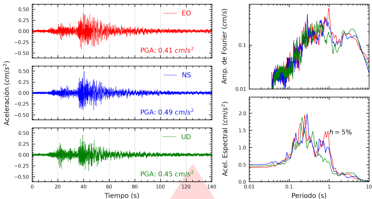
Figura A.29: Registros tiempo-historia, espectros de Fourier y de respuesta en las direcciones EO, NS y vertical de la estación IMCA. Sismo de Chupaca, Chupaca - Junín del 2026-07-18, 21:24:34 (Hora local)
