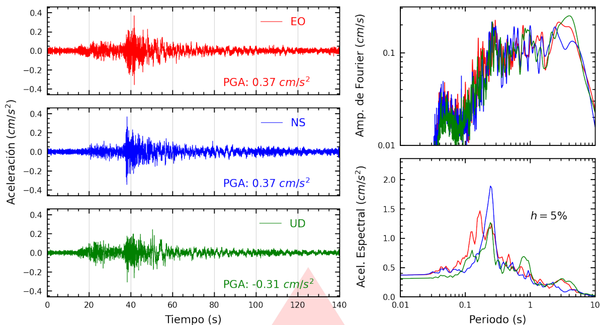
Figura A.39: Registros tiempo-historia, espectros de Fourier y de respuesta en las direcciones EO, NS y vertical de la estación BORJA. Sismo de Chupaca, Chupaca - Junín del 2026-07-18, 21:24:34 (Hora local)
