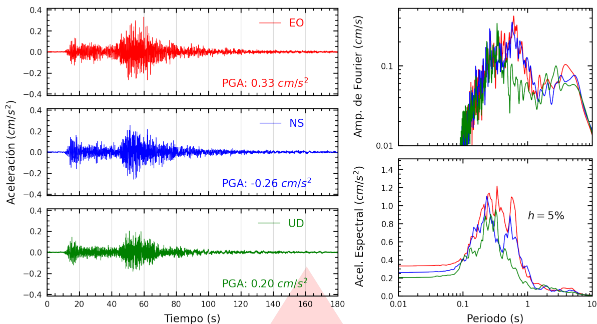
Figura A.41: Registros tiempo-historia, espectros de Fourier y de respuesta en las direcciones EO, NS y vertical de la estación CARAL. Sismo de Chupaca, Chupaca - Junín del 2026-07-18, 21:24:34 (Hora local)
