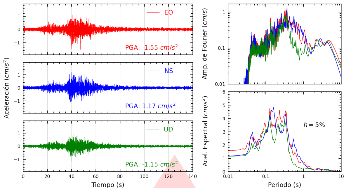
Figura A.9: Registros tiempo-historia, espectros de Fourier y de respuesta en las direcciones EO, NS y vertical de la estación UNTEL. Sismo de Chupaca, Chupaca - Junín del 2026-07-18, 21:24:34 (Hora local)
