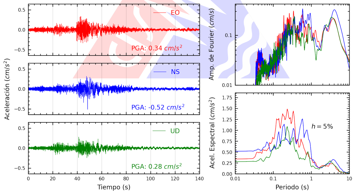
Figura A.28: Registros tiempo-historia, espectros de Fourier y de respuesta en las direcciones EO, NS y vertical de la estación COMAS. Sismo de Chupaca, Chupaca - Junín del 2026-07-18, 21:24:34 (Hora local)
