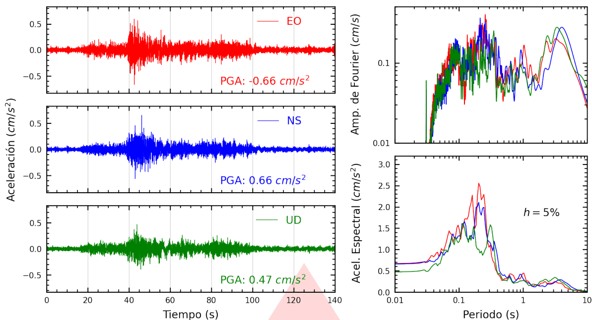
Figura A.23: Registros tiempo-historia, espectros de Fourier y de respuesta en las direcciones EO, NS y vertical de la estación INDEP. Sismo de Chupaca, Chupaca - Junín del 2026-07-18, 21:24:34 (Hora local)
