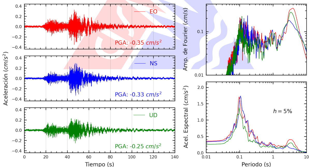
Figura A.40: Registros tiempo-historia, espectros de Fourier y de respuesta en las direcciones EO, NS y vertical de la estación AMORE. Sismo de Chupaca, Chupaca - Junín del 2026-07-18, 21:24:34 (Hora local)
