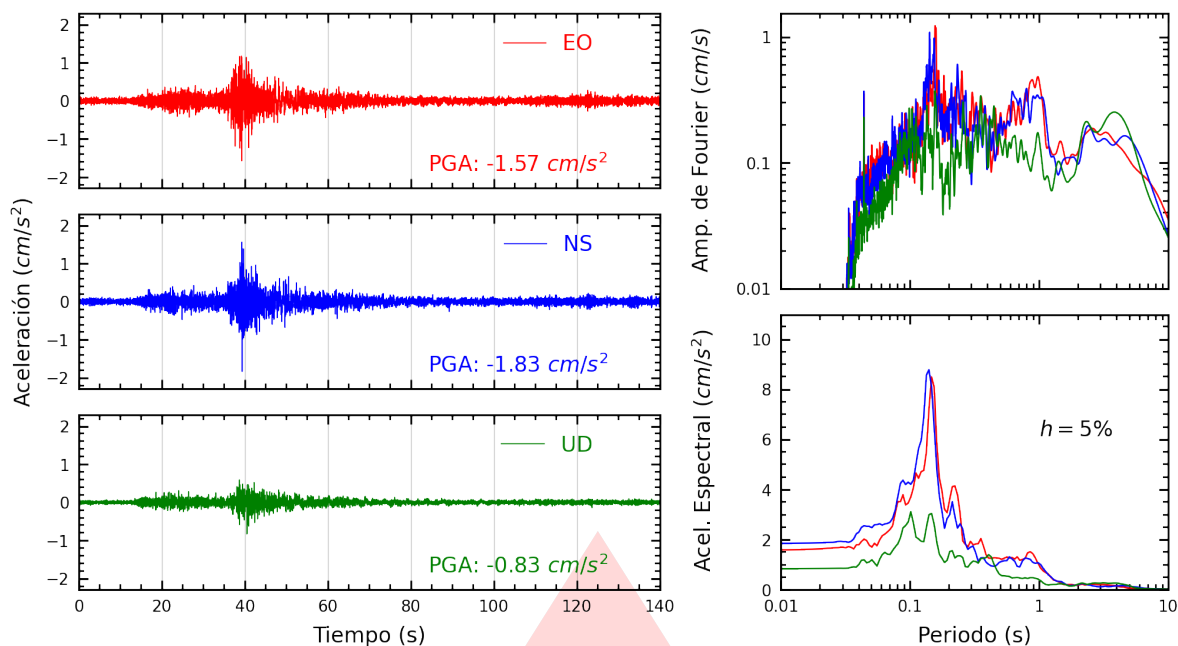
Figura A.5: Registros tiempo-historia, espectros de Fourier y de respuesta en las direcciones EO, NS y vertical de la estación USILM. Sismo de Chupaca, Chupaca - Junín del 2026-07-18, 21:24:34 (Hora local)
