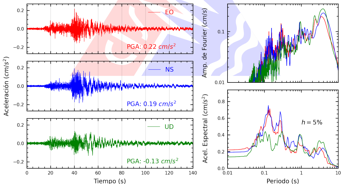
Figura A.44: Registros tiempo-historia, espectros de Fourier y de respuesta en las direcciones EO, NS y vertical de la estación ATARJ. Sismo de Chupaca, Chupaca - Junín del 2026-07-18, 21:24:34 (Hora local)
