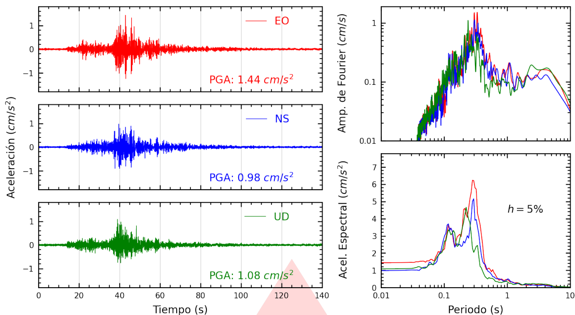
Figura A.11: Registros tiempo-historia, espectros de Fourier y de respuesta en las direcciones EO, NS y vertical de la estación SOVES. Sismo de Chupaca, Chupaca - Junín del 2026-07-18, 21:24:34 (Hora local)
