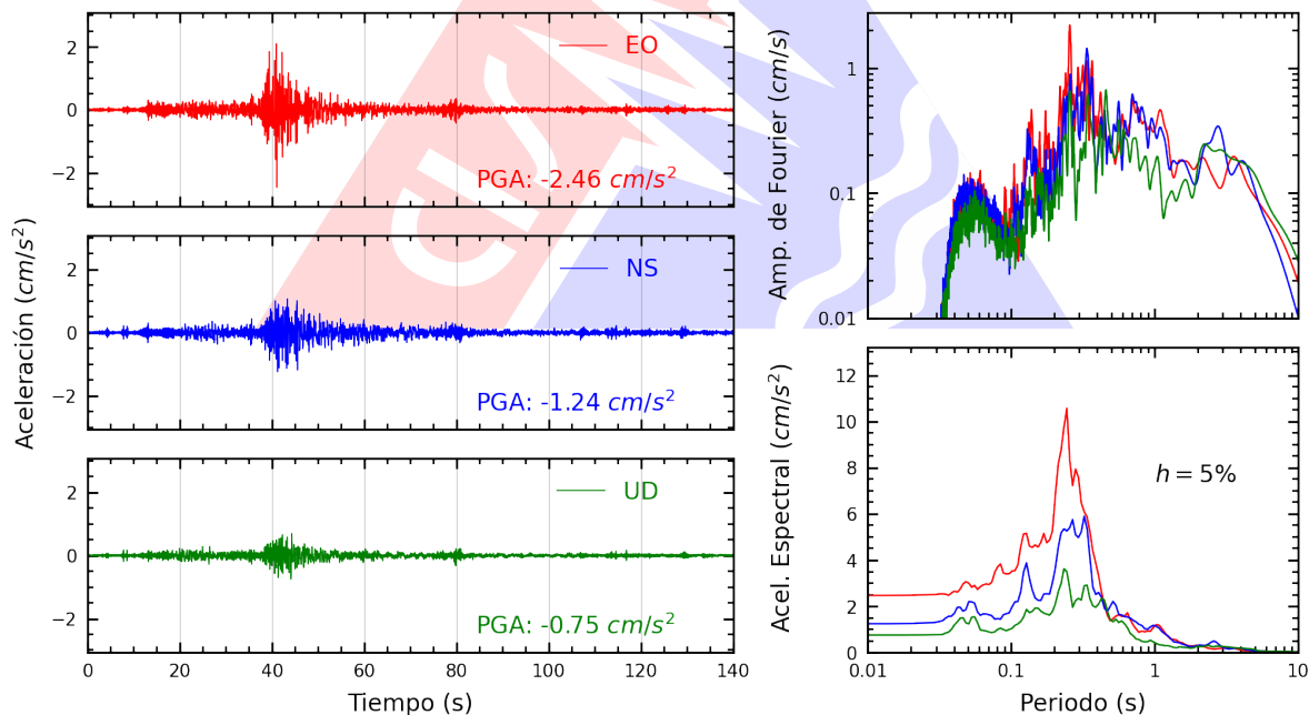
Figura A.2: Registros tiempo-historia, espectros de Fourier y de respuesta en las direcciones EO, NS y vertical de la estación BRIS2. Sismo de Chupaca, Chupaca - Junín del 2026-07-18, 21:24:34 (Hora local)
