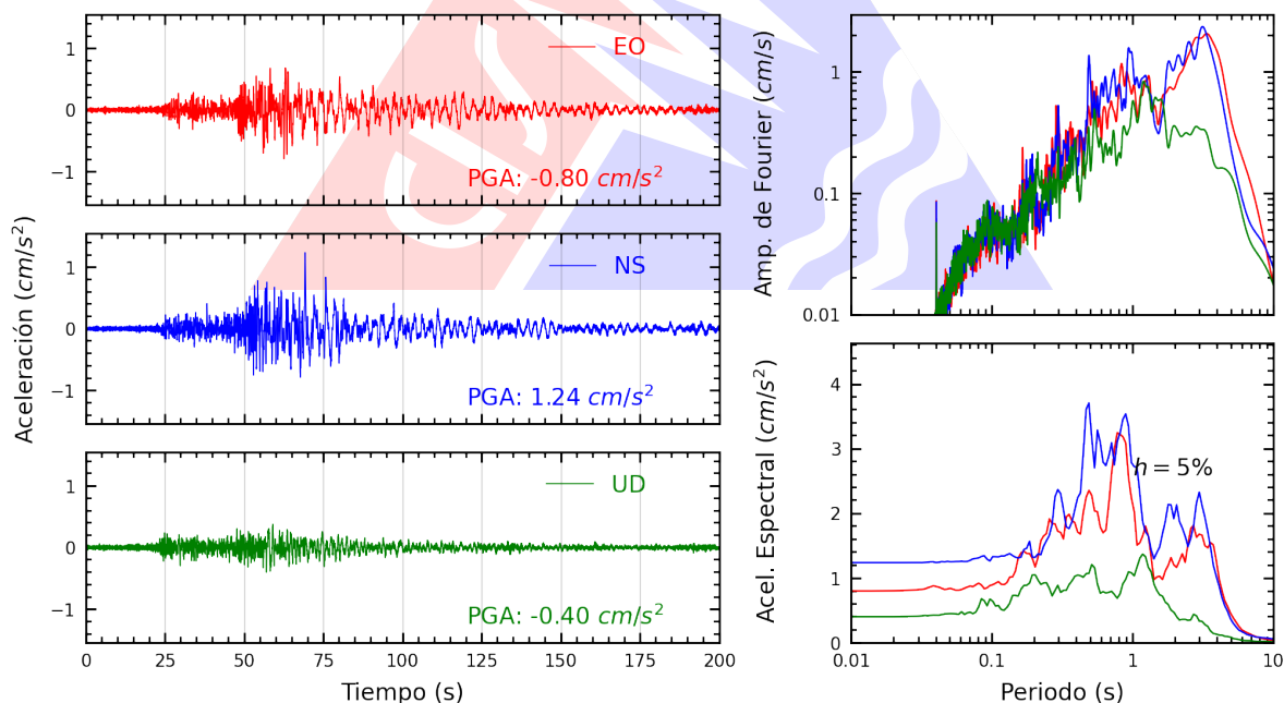
Figura A.12: Registros tiempo-historia, espectros de Fourier y de respuesta en las direcciones EO, NS y vertical de la estación UNICA. Sismo de Chupaca, Chupaca - Junín del 2026-07-18, 21:24:34 (Hora local)
