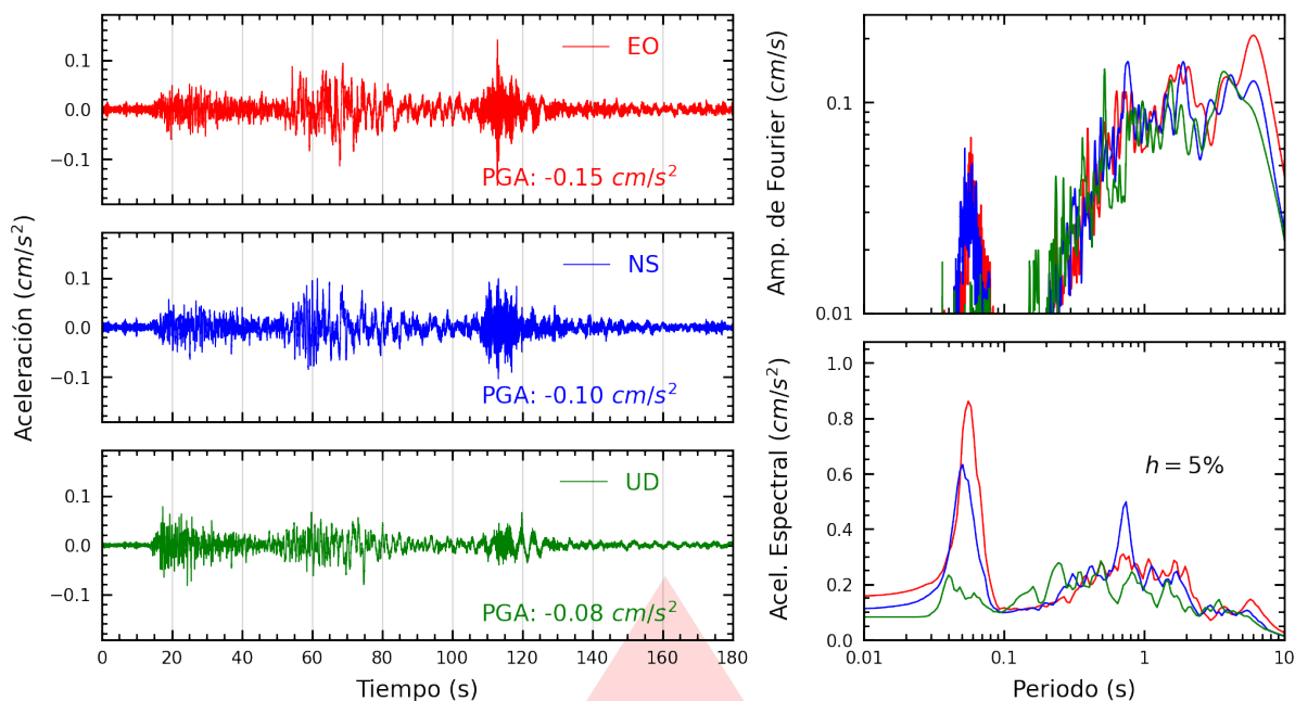
Figura A.45: Registros tiempo-historia, espectros de Fourier y de respuesta en las direcciones EO, NS y vertical de la estación UNMBA. Sismo de Chupaca, Chupaca - Junín del 2026-07-18, 21:24:34 (Hora local)
