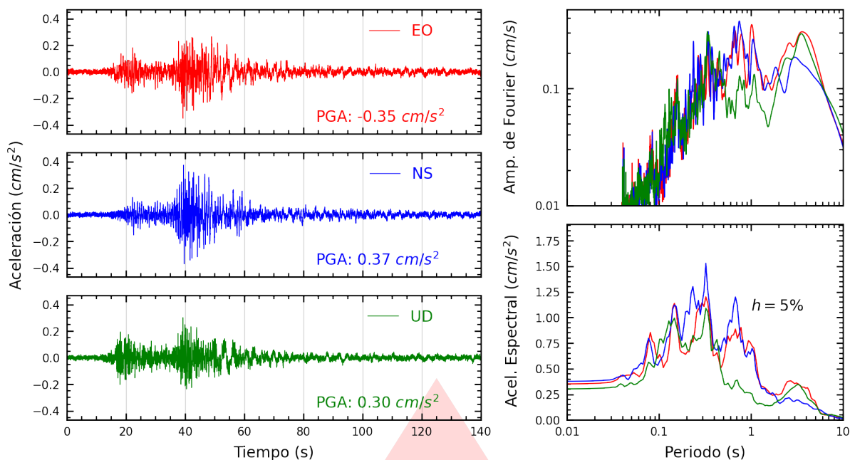
Figura A.37: Registros tiempo-historia, espectros de Fourier y de respuesta en las direcciones EO, NS y vertical de la estación UNMSM. Sismo de Chupaca, Chupaca - Junín del 2026-07-18, 21:24:34 (Hora local)
