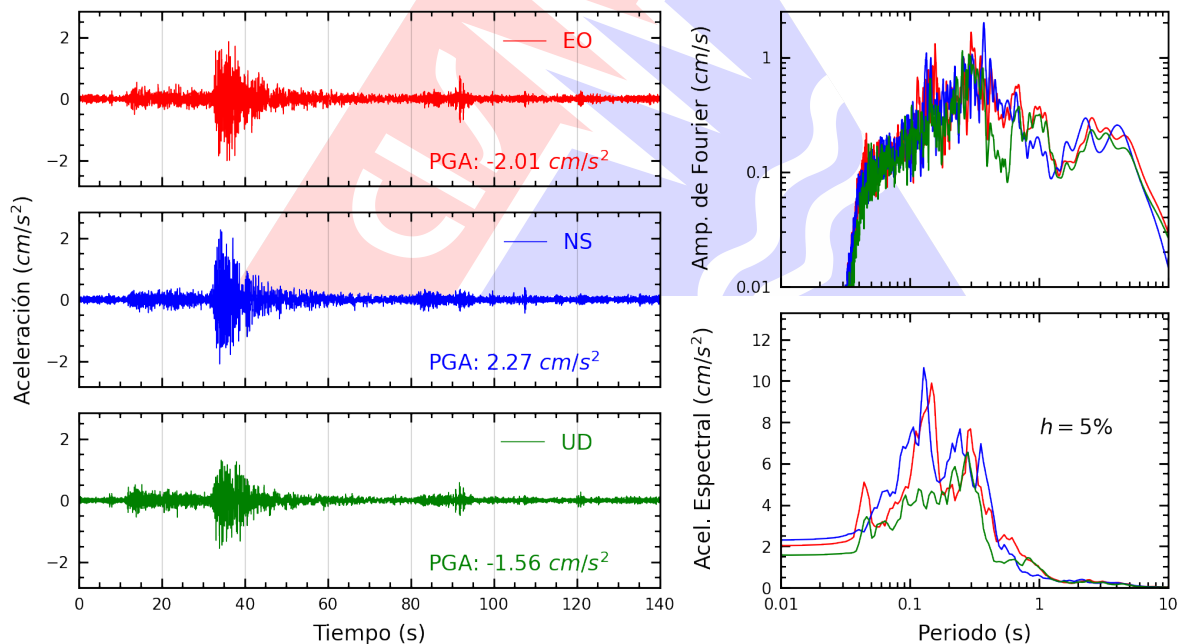
Figura A.4: Registros tiempo-historia, espectros de Fourier y de respuesta en las direcciones EO, NS y vertical de la estación PHERM. Sismo de Chupaca, Chupaca - Junín del 2026-07-18, 21:24:34 (Hora local)
