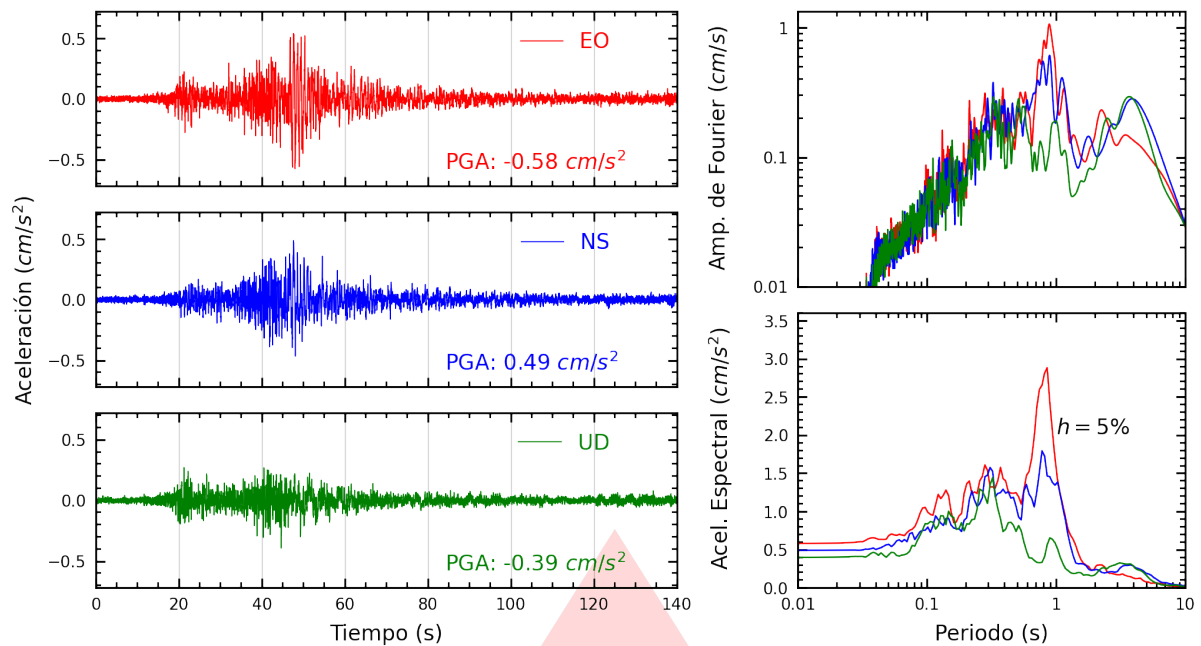
Figura A.27: Registros tiempo-historia, espectros de Fourier y de respuesta en las direcciones EO, NS y vertical de la estación UCVAT. Sismo de Chupaca, Chupaca - Junín del 2026-07-18, 21:24:34 (Hora local)
