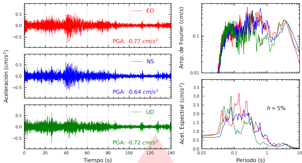
Figura A.19: Registros tiempo-historia, espectros de Fourier y de respuesta en las direcciones EO, NS y vertical de la estación SJLSV. Sismo de Chupaca, Chupaca - Junín del 2026-07-18, 21:24:34 (Hora local)
