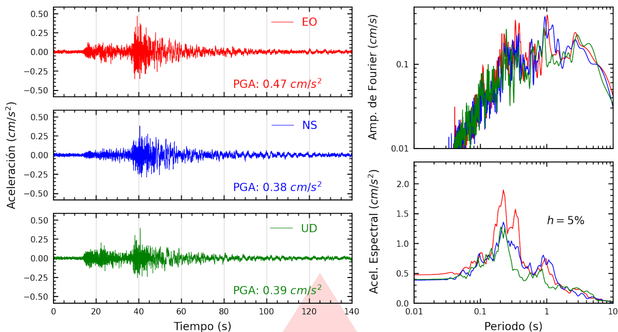
Figura A.31: Registros tiempo-historia, espectros de Fourier y de respuesta en las direcciones EO, NS y vertical de la estación SERVI. Sismo de Chupaca, Chupaca - Junín del 2026-07-18, 21:24:34 (Hora local)
