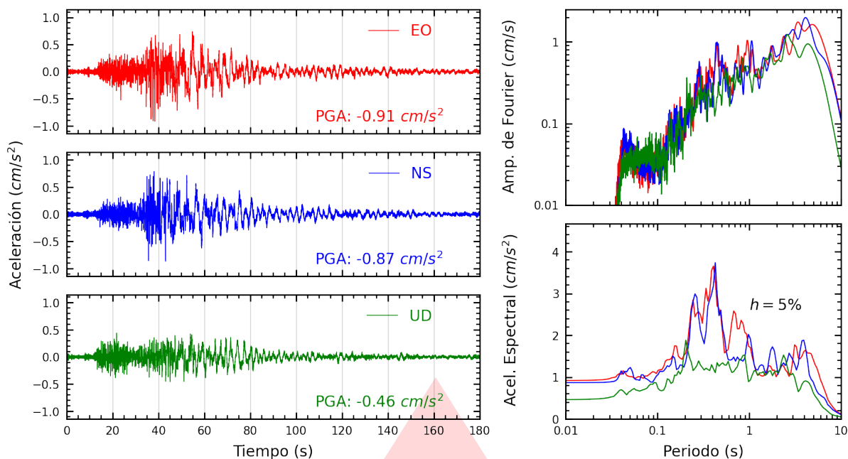
Figura A.15: Registros tiempo-historia, espectros de Fourier y de respuesta en las direcciones EO, NS y vertical de la estación SCAYA. Sismo de Chupaca, Chupaca - Junín del 2026-07-18, 21:24:34 (Hora local)
