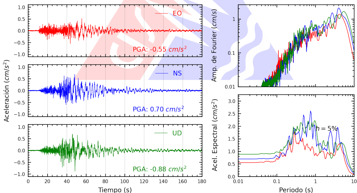
Figura A.16: Registros tiempo-historia, espectros de Fourier y de respuesta en las direcciones EO, NS y vertical de la estación UNSCH. Sismo de Chupaca, Chupaca - Junín del 2026-07-18, 21:24:34 (Hora local)
