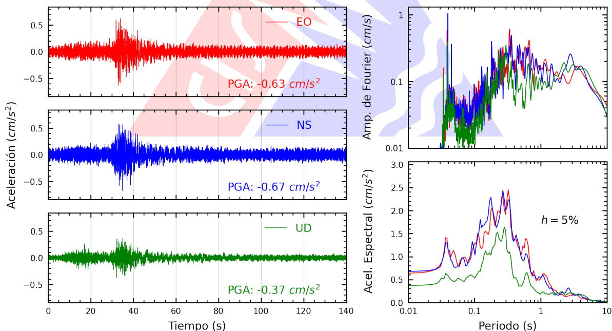
Figura A.22: Registros tiempo-historia, espectros de Fourier y de respuesta en las direcciones EO, NS y vertical de la estación UPCVI. Sismo de Chupaca, Chupaca - Junín del 2026-07-18, 21:24:34 (Hora local)
