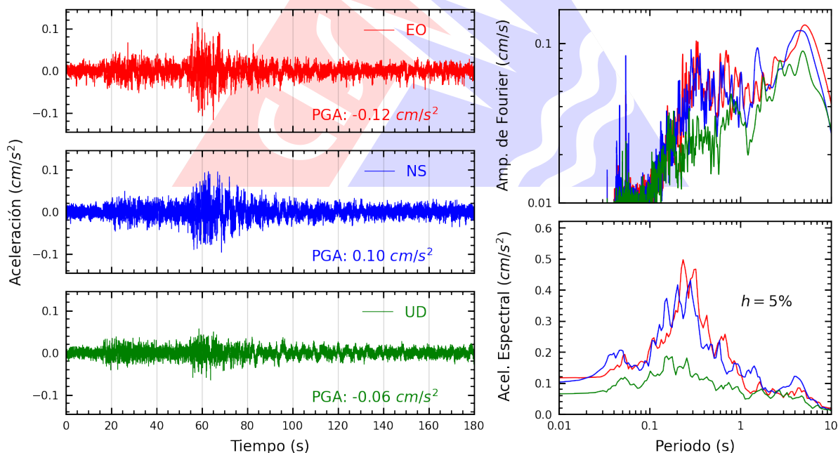
Figura A.46: Registros tiempo-historia, espectros de Fourier y de respuesta en las direcciones EO, NS y vertical de la estación UNAB. Sismo de Chupaca, Chupaca - Junín del 2026-07-18, 21:24:34 (Hora local)
