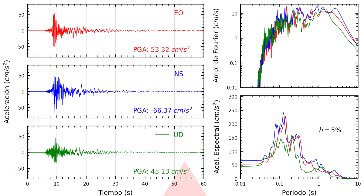
Figura A.1: Registros tiempo-historia, espectros de Fourier y de respuesta en las direcciones EO, NS y vertical de la estación SCHYO. Sismo de Chupaca, Chupaca - Junín del 2026-07-18, 21:24:34 (Hora local)
