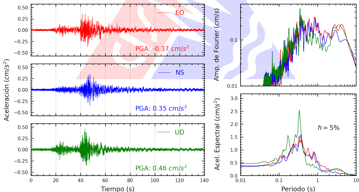
Figura A.32: Registros tiempo-historia, espectros de Fourier y de respuesta en las direcciones EO, NS y vertical de la estación UNFV. Sismo de Chupaca, Chupaca - Junín del 2026-07-18, 21:24:34 (Hora local)
