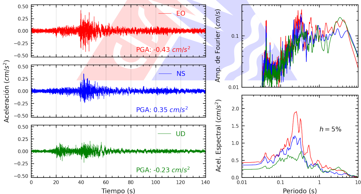
Figura A.34: Registros tiempo-historia, espectros de Fourier y de respuesta en las direcciones EO, NS y vertical de la estación CEPRE. Sismo de Chupaca, Chupaca - Junín del 2026-07-18, 21:24:34 (Hora local)
