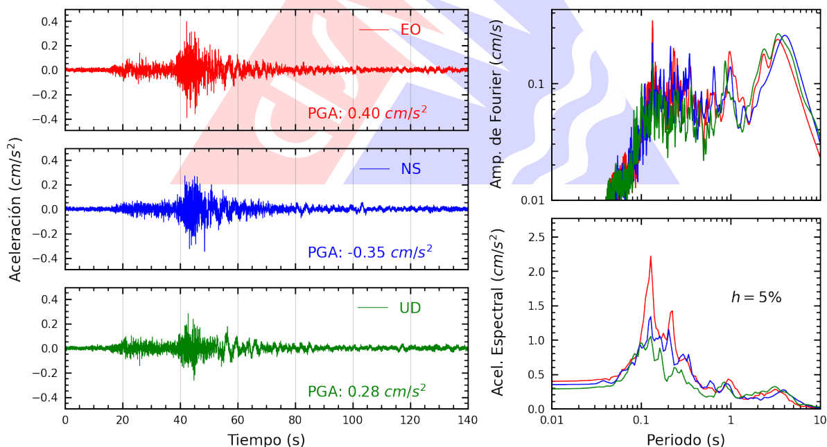
Figura A.36: Registros tiempo-historia, espectros de Fourier y de respuesta en las direcciones EO, NS y vertical de la estación JALVA. Sismo de Chupaca, Chupaca - Junín del 2026-07-18, 21:24:34 (Hora local)
