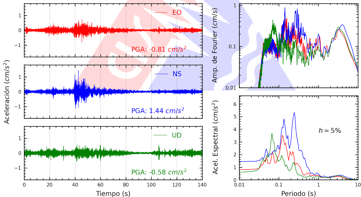
Figura A.10: Registros tiempo-historia, espectros de Fourier y de respuesta en las direcciones EO, NS y vertical de la estación CARAB. Sismo de Chupaca, Chupaca - Junín del 2026-07-18, 21:24:34 (Hora local)
