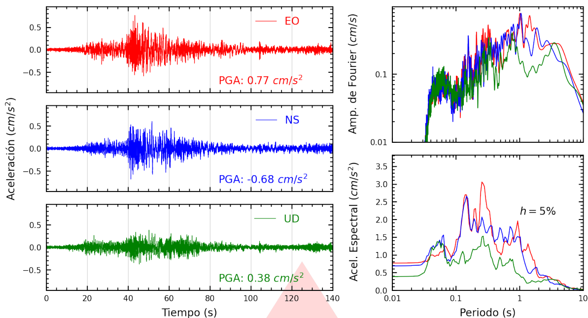
Figura A.21: Registros tiempo-historia, espectros de Fourier y de respuesta en las direcciones EO, NS y vertical de la estación PRADO. Sismo de Chupaca, Chupaca - Junín del 2026-07-18, 21:24:34 (Hora local)
