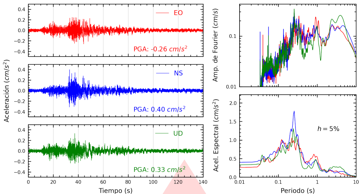
Figura A.35: Registros tiempo-historia, espectros de Fourier y de respuesta en las direcciones EO, NS y vertical de la estación USMP. Sismo de Chupaca, Chupaca - Junín del 2026-07-18, 21:24:34 (Hora local)
