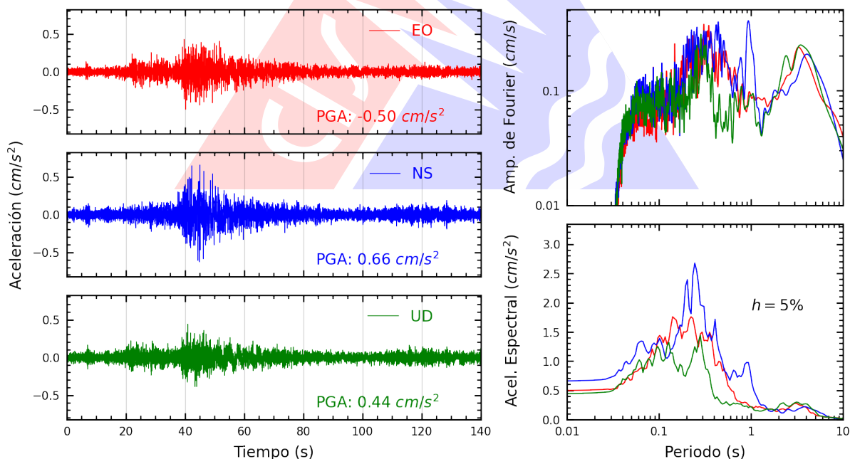
Figura A.24: Registros tiempo-historia, espectros de Fourier y de respuesta en las direcciones EO, NS y vertical de la estación SJLSC. Sismo de Chupaca, Chupaca - Junín del 2026-07-18, 21:24:34 (Hora local)
