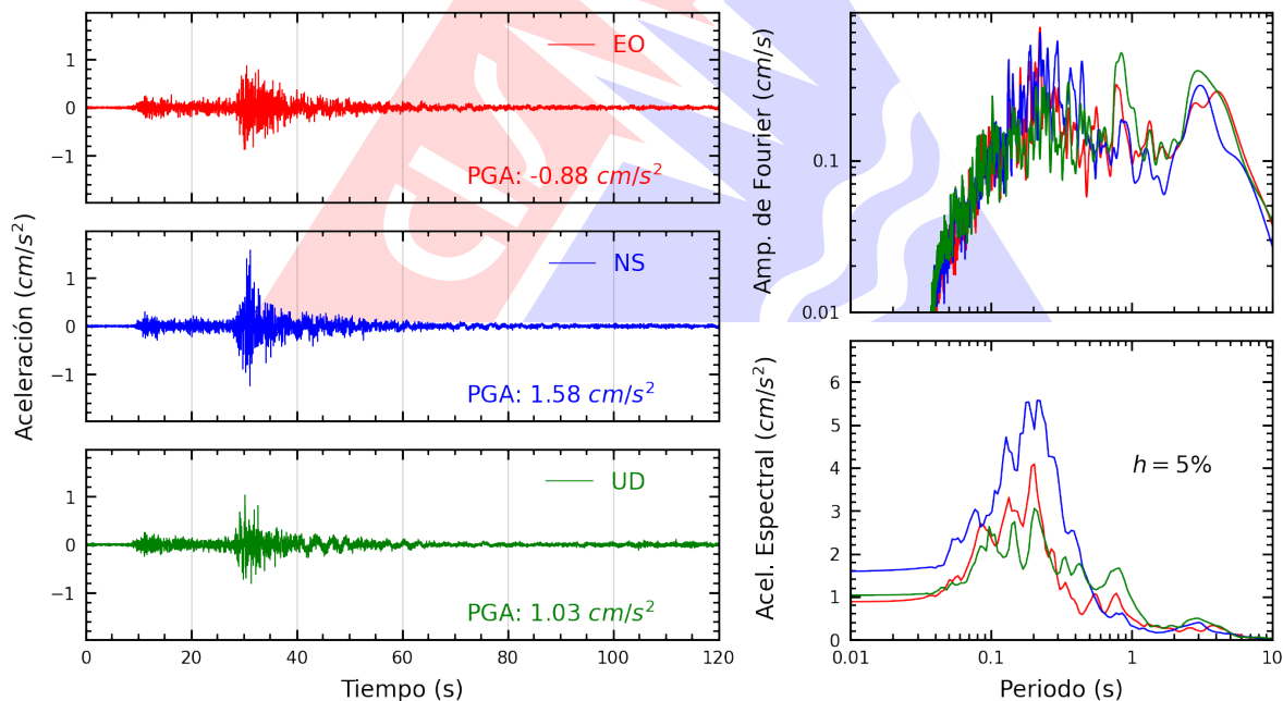
Figura A.8: Registros tiempo-historia, espectros de Fourier y de respuesta en las direcciones EO, NS y vertical de la estación ASIA. Sismo de Chupaca, Chupaca - Junín del 2026-07-18, 21:24:34 (Hora local)
