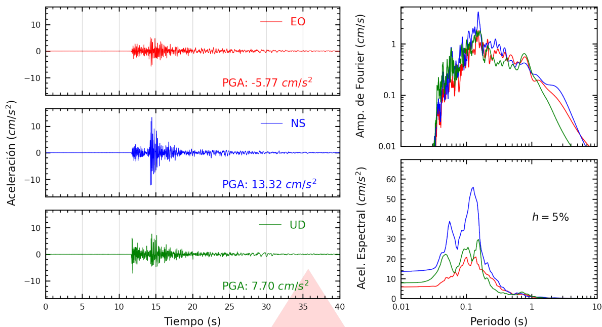
Figura A.1: Registros tiempo-historia, espectros de Fourier y de respuesta en las direcciones EO, NS y vertical de la estación SCHYO. Sismo de Chupaca, Chupaca - Junín del 2026-07-18, 21:41:37 (Hora local)
