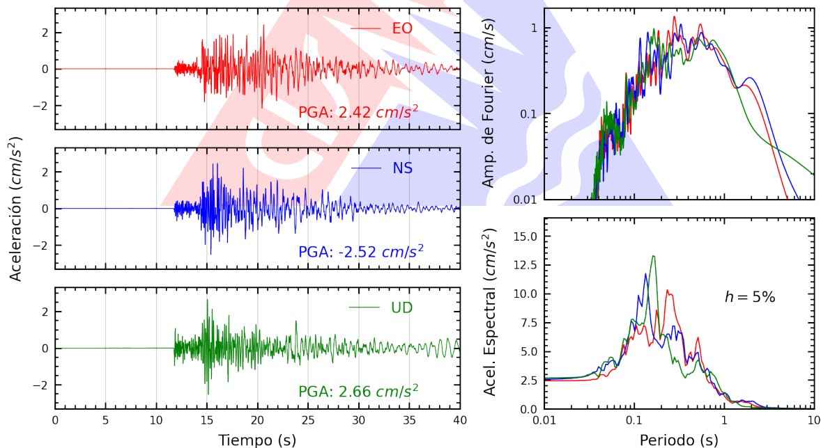
Figura A.2: Registros tiempo-historia, espectros de Fourier y de respuesta en las direcciones EO, NS y vertical de la estación UNCP. Sismo de Chupaca, Chupaca - Junín del 2026-07-18, 21:41:37 (Hora local)
