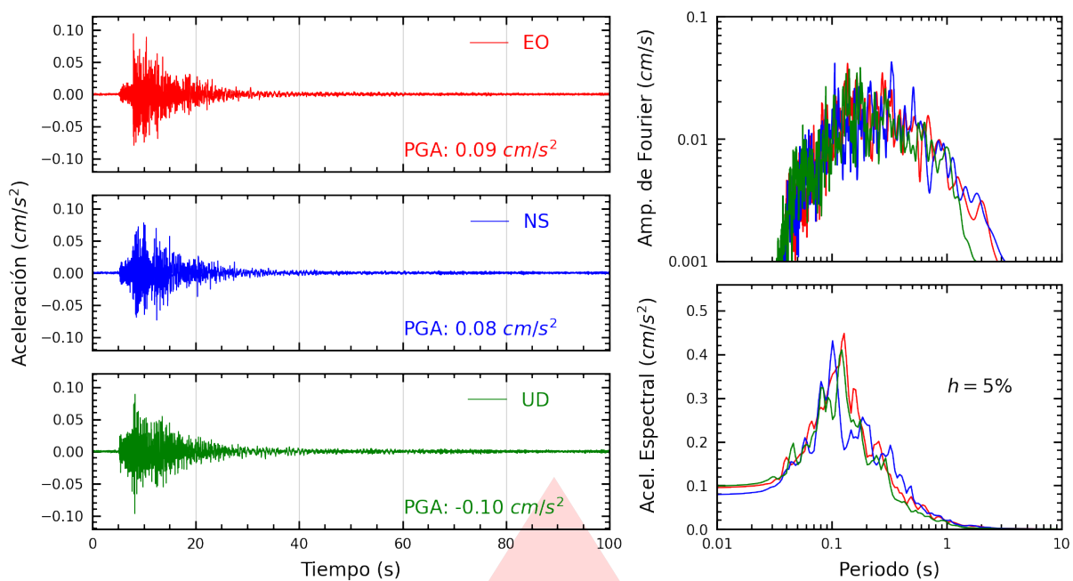
Figura A.1: Registros tiempo-historia, espectros de Fourier y de respuesta en las direcciones EO, NS y vertical de la estación UNCP. Sismo de Chupaca, Chupaca - Junín del 2026-07-20, 04:39:52 (Hora local)
