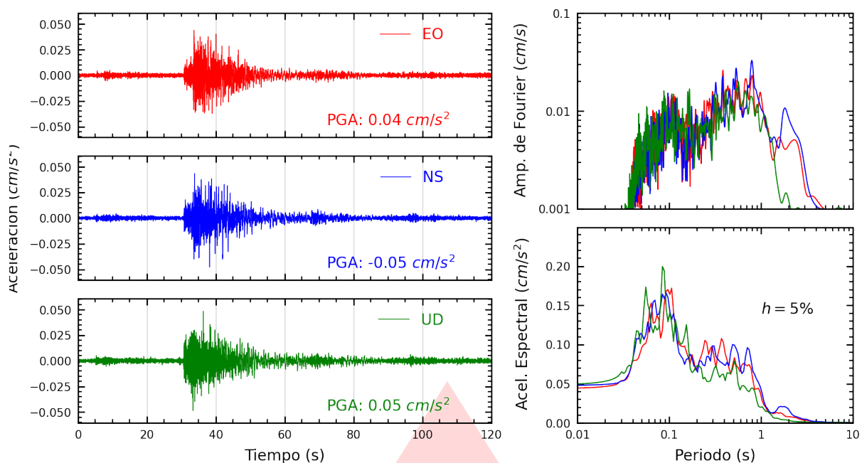
Figura A.1: Registros tiempo-historia, espectros de Fourier y de respuesta en las direcciones EO, NS y vertical de la estación UNCP. Sismo de Chupaca, Chupaca - Junín del 2026-07-20, 21:45:27 (Hora local)
