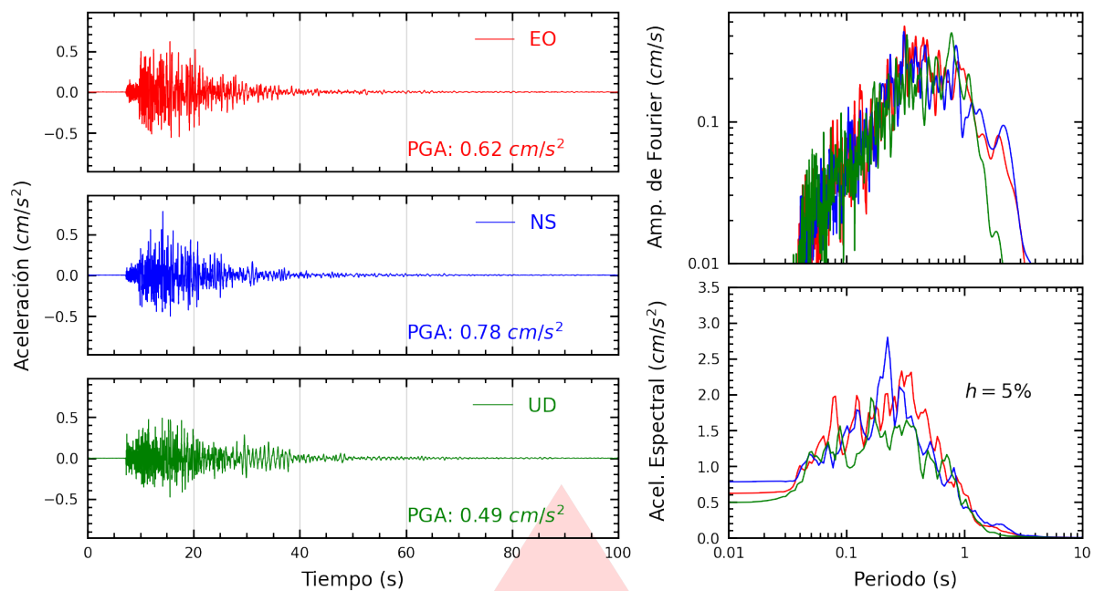
Figura A.1: Registros tiempo-historia, espectros de Fourier y de respuesta en las direcciones EO, NS y vertical de la estación UNCP. Sismo de Chupaca, Chupaca - Junín del 2026-07-21, 02:24:54 (Hora local)
