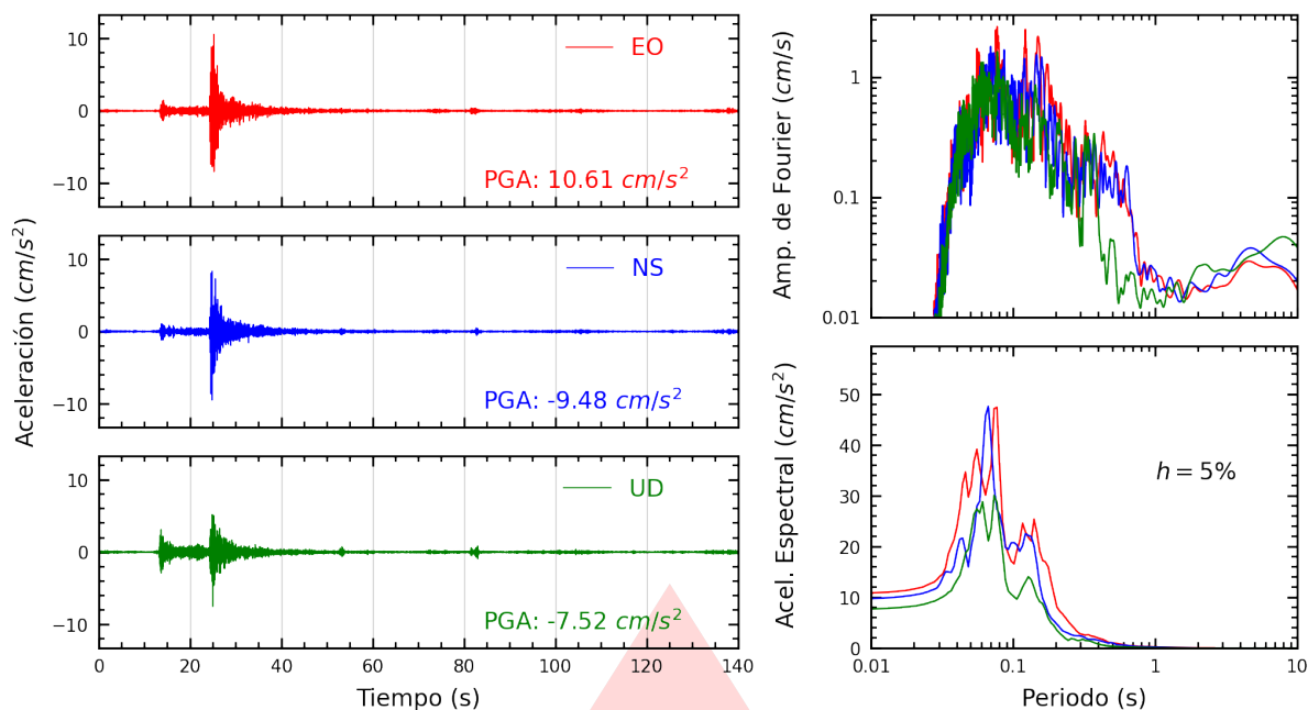
Figura A.7: Registros tiempo-historia, espectros de Fourier y de respuesta en las direcciones EO, NS y vertical de la estación SJLSV. Sismo de Ricardo Palma, Huarochirí - Lima del 2026-07-22, 07:25:57 (Hora local)
