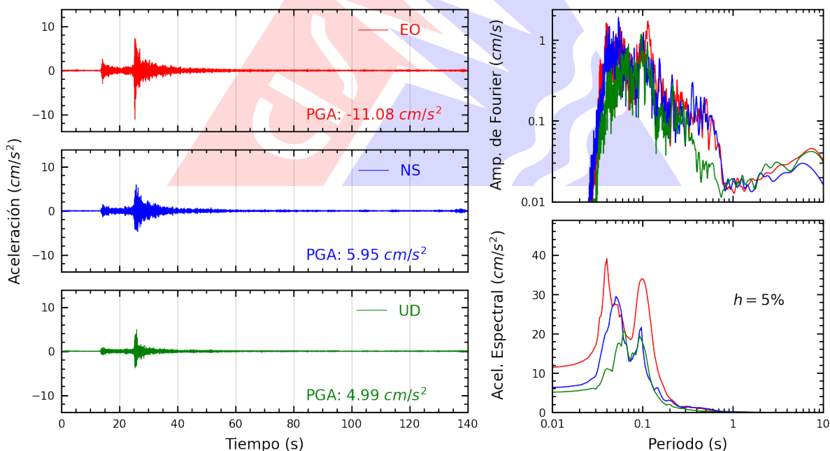
Figura A.6: Registros tiempo-historia, espectros de Fourier y de respuesta en las direcciones EO, NS y vertical de la estación OLIVO. Sismo de Ricardo Palma, Huarochirí - Lima del 2026-07-22, 07:25:57 (Hora local)
