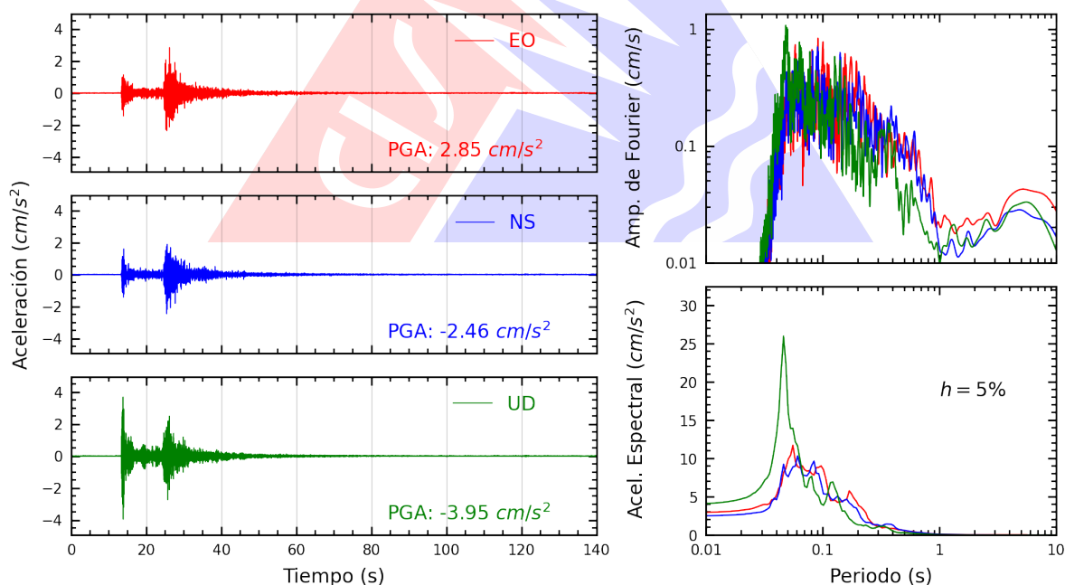
Figura A.22: Registros tiempo-historia, espectros de Fourier y de respuesta en las direcciones EO, NS y vertical de la estación USILP. Sismo de Ricardo Palma, Huarochirí - Lima del 2026-07-22, 07:25:57 (Hora local)
