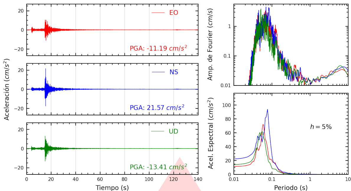
Figura A.1: Registros tiempo-historia, espectros de Fourier y de respuesta en las direcciones EO, NS y vertical de la estación JOSEO. Sismo de Ricardo Palma, Huarochirí - Lima del 2026-07-22, 07:25:57 (Hora local)
