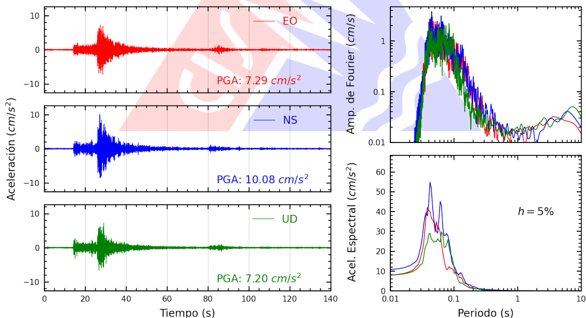
Figura A.8: Registros tiempo-historia, espectros de Fourier y de respuesta en las direcciones EO, NS y vertical de la estación SROSA. Sismo de Ricardo Palma, Huarochirí - Lima del 2026-07-22, 07:25:57 (Hora local)
