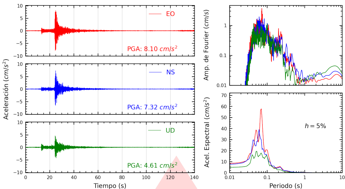
Figura A.11: Registros tiempo-historia, espectros de Fourier y de respuesta en las direcciones EO, NS y vertical de la estación INDEP. Sismo de Ricardo Palma, Huarochirí - Lima del 2026-07-22, 07:25:57 (Hora local)
