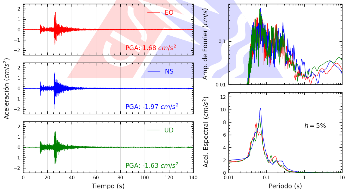
Figura A.30: Registros tiempo-historia, espectros de Fourier y de respuesta en las direcciones EO, NS y vertical de la estación UNFV. Sismo de Ricardo Palma, Huarochirí - Lima del 2026-07-22, 07:25:57 (Hora local)
