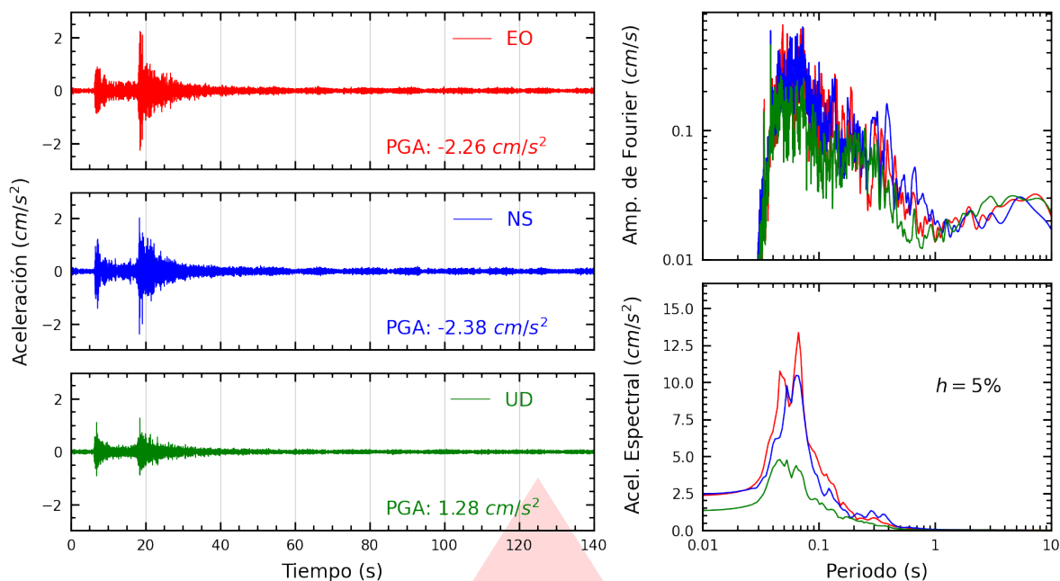
Figura A.29: Registros tiempo-historia, espectros de Fourier y de respuesta en las direcciones EO, NS y vertical de la estación UPCVI. Sismo de Ricardo Palma, Huarochirí - Lima del 2026-07-22, 07:25:57 (Hora local)
