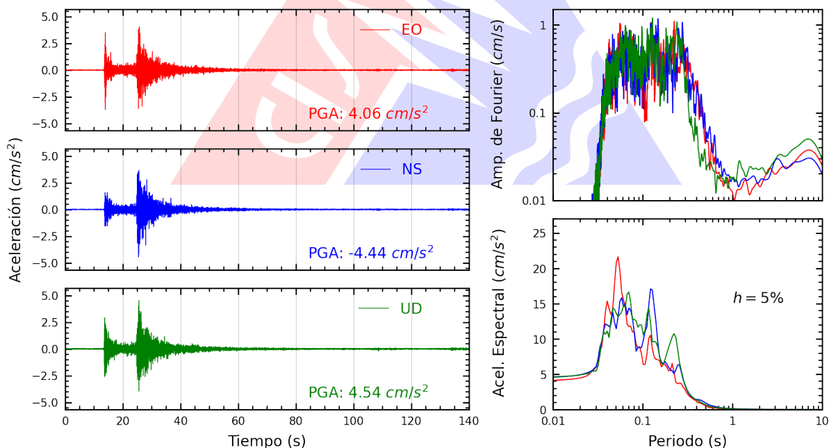
Figura A.20: Registros tiempo-historia, espectros de Fourier y de respuesta en las direcciones EO, NS y vertical de la estación SOVES. Sismo de Ricardo Palma, Huarochirí - Lima del 2026-07-22, 07:25:57 (Hora local)
