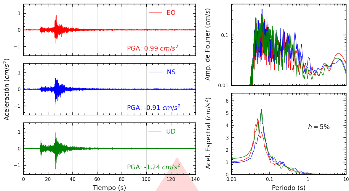
Figura A.33: Registros tiempo-historia, espectros de Fourier y de respuesta en las direcciones EO, NS y vertical de la estación BONDY. Sismo de Ricardo Palma, Huarochirí - Lima del 2026-07-22, 07:25:57 (Hora local)
