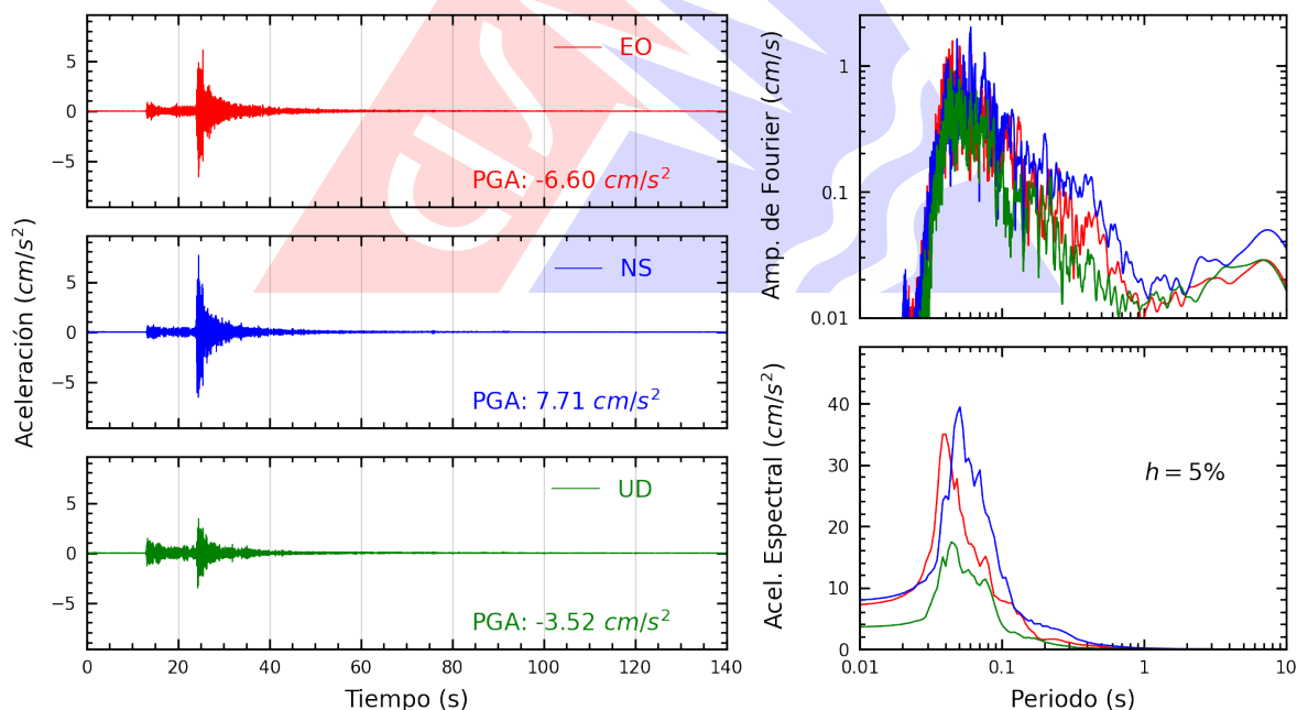
Figura A.12: Registros tiempo-historia, espectros de Fourier y de respuesta en las direcciones EO, NS y vertical de la estación SJLCE. Sismo de Ricardo Palma, Huarochirí - Lima del 2026-07-22, 07:25:57 (Hora local)
