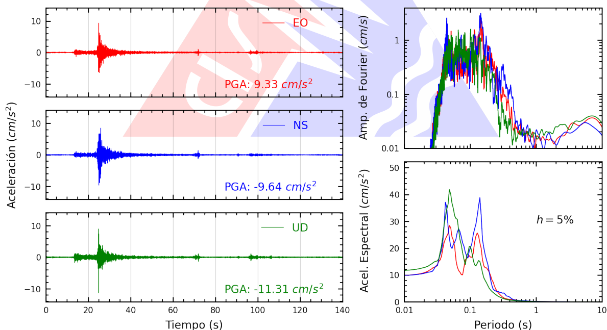
Figura A.4: Registros tiempo-historia, espectros de Fourier y de respuesta en las direcciones EO, NS y vertical de la estación CARAB. Sismo de Ricardo Palma, Huarochirí - Lima del 2026-07-22, 07:25:57 (Hora local)
