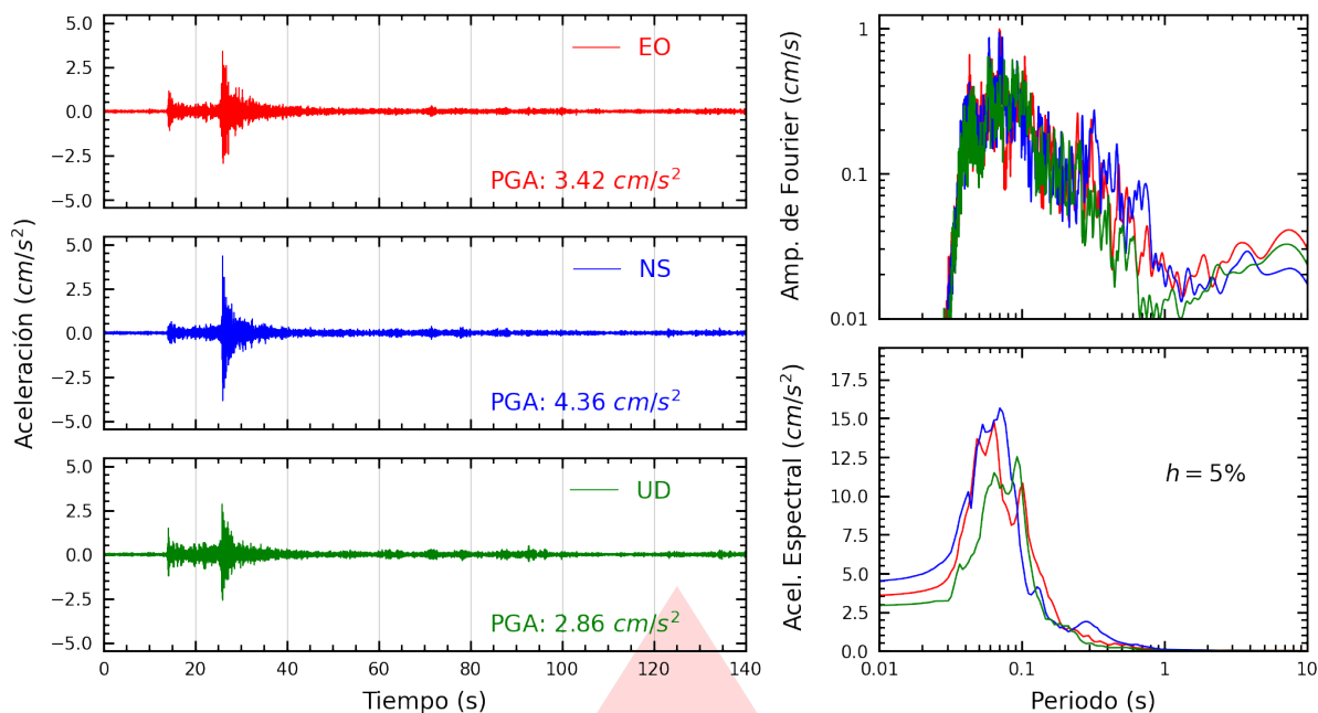
Figura A.21: Registros tiempo-historia, espectros de Fourier y de respuesta en las direcciones EO, NS y vertical de la estación MADRE. Sismo de Ricardo Palma, Huarochirí - Lima del 2026-07-22, 07:25:57 (Hora local)
