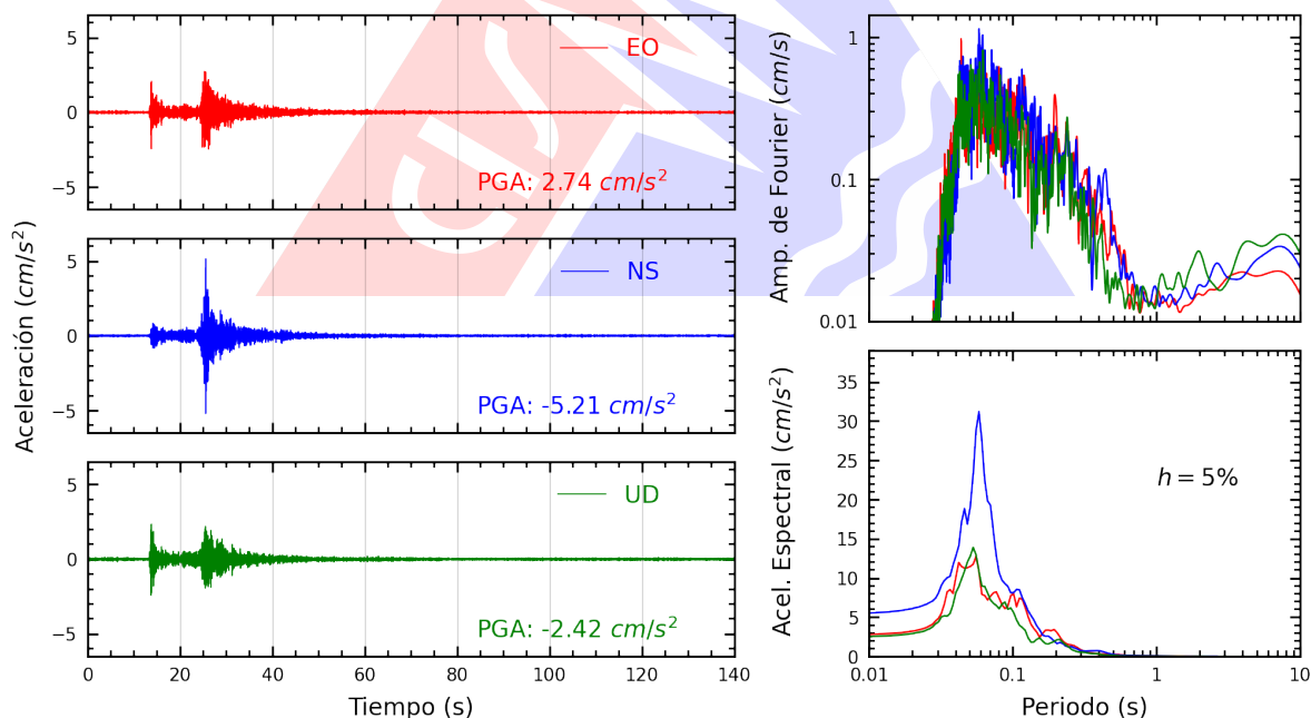
Figura A.18: Registros tiempo-historia, espectros de Fourier y de respuesta en las direcciones EO, NS y vertical de la estación URPE. Sismo de Ricardo Palma, Huarochirí - Lima del 2026-07-22, 07:25:57 (Hora local)
