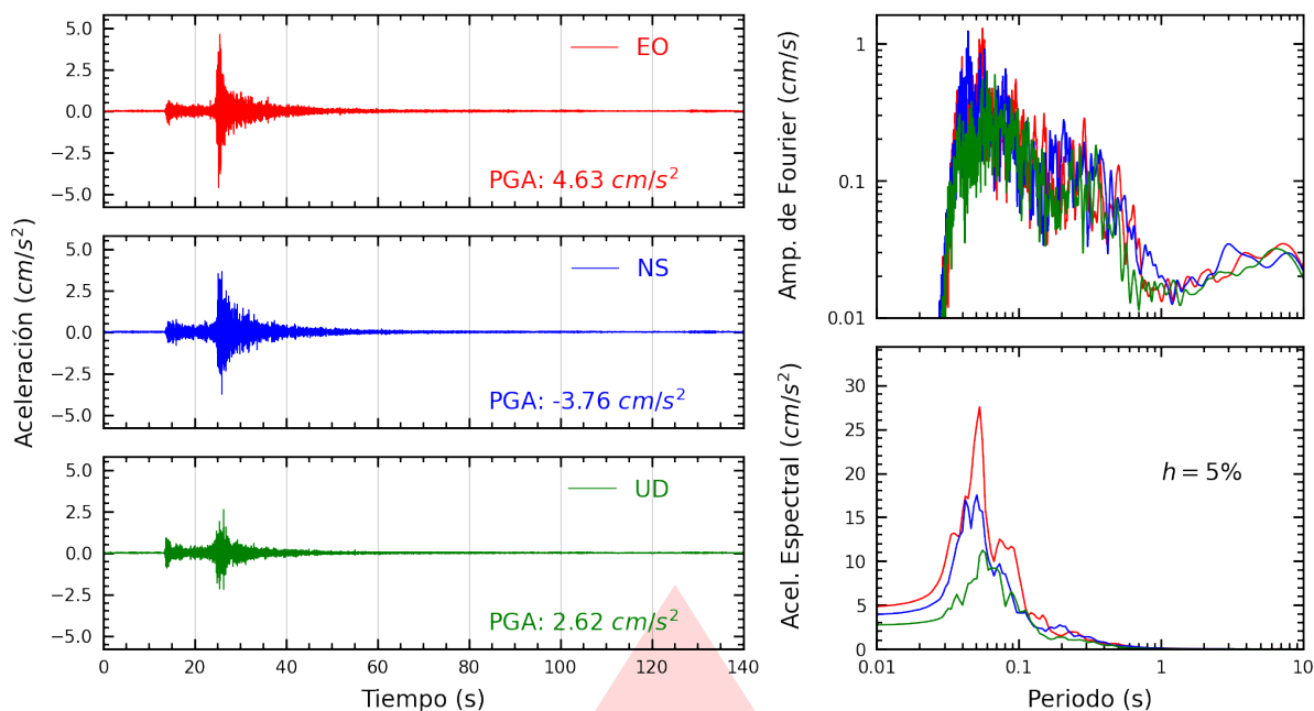
Figura A.19: Registros tiempo-historia, espectros de Fourier y de respuesta en las direcciones EO, NS y vertical de la estación COMAS. Sismo de Ricardo Palma, Huarochirí - Lima del 2026-07-22, 07:25:57 (Hora local)
