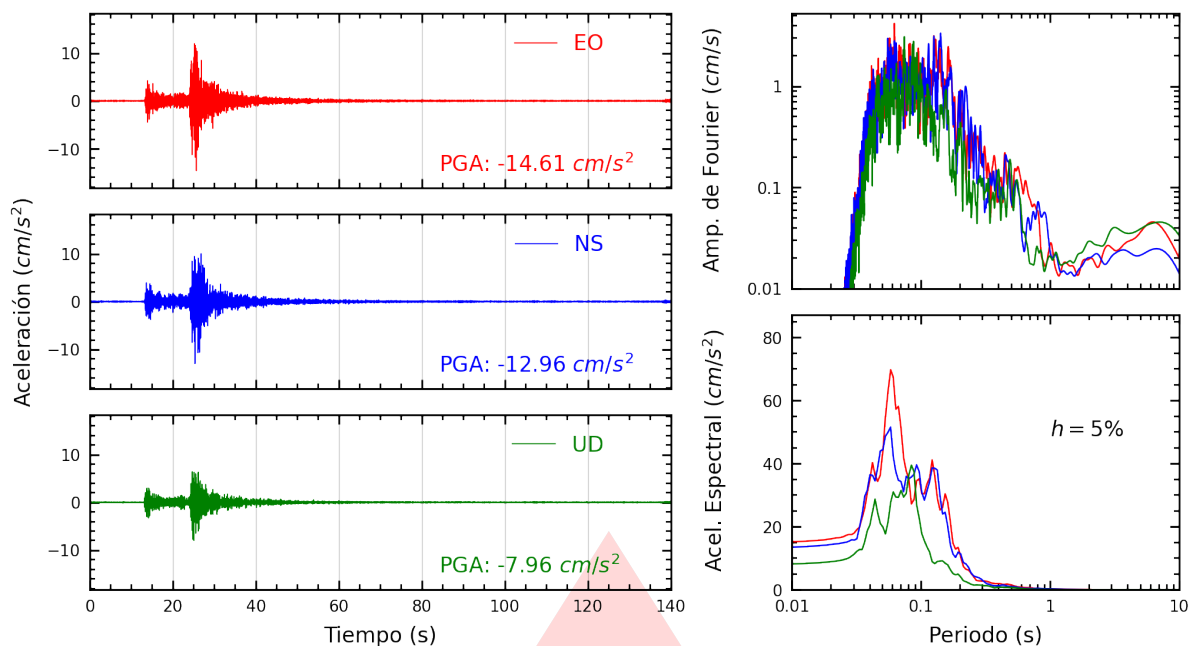
Figura A.3: Registros tiempo-historia, espectros de Fourier y de respuesta en las direcciones EO, NS y vertical de la estación USILM. Sismo de Ricardo Palma, Huarochirí - Lima del 2026-07-22, 07:25:57 (Hora local)
