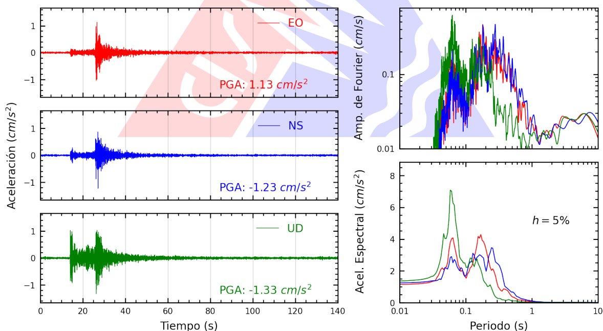
Figura A.32: Registros tiempo-historia, espectros de Fourier y de respuesta en las direcciones EO, NS y vertical de la estación ACAPU. Sismo de Ricardo Palma, Huarochirí - Lima del 2026-07-22, 07:25:57 (Hora local)
