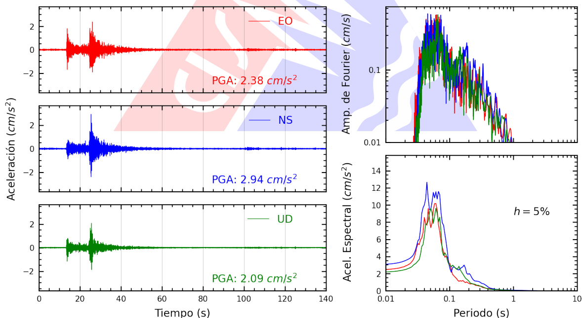
Figura A.28: Registros tiempo-historia, espectros de Fourier y de respuesta en las direcciones EO, NS y vertical de la estación BORJA. Sismo de Ricardo Palma, Huarochirí - Lima del 2026-07-22, 07:25:57 (Hora local)
