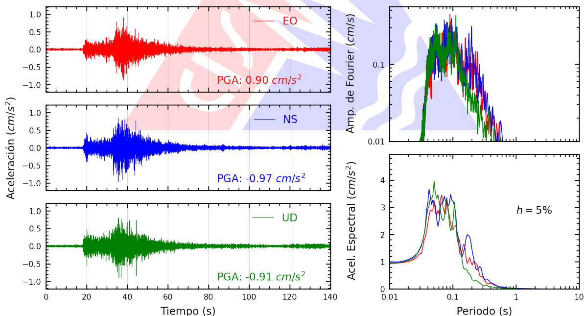
Figura A.34: Registros tiempo-historia, espectros de Fourier y de respuesta en las direcciones EO, NS y vertical de la estación ASIA. Sismo de Ricardo Palma, Huarochirí - Lima del 2026-07-22, 07:25:57 (Hora local)
