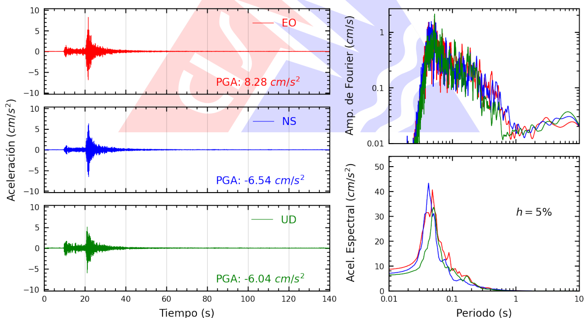
Figura A.10: Registros tiempo-historia, espectros de Fourier y de respuesta en las direcciones EO, NS y vertical de la estación USMP. Sismo de Ricardo Palma, Huarochirí - Lima del 2026-07-22, 07:25:57 (Hora local)
