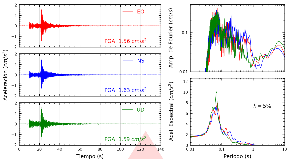
Figura A.31: Registros tiempo-historia, espectros de Fourier y de respuesta en las direcciones EO, NS y vertical de la estación UNMSM. Sismo de Ricardo Palma, Huarochirí - Lima del 2026-07-22, 07:25:57 (Hora local)
