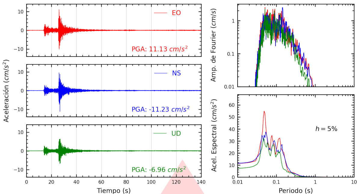
Figura A.5: Registros tiempo-historia, espectros de Fourier y de respuesta en las direcciones EO, NS y vertical de la estación PHERM. Sismo de Ricardo Palma, Huarochirí - Lima del 2026-07-22, 07:25:57 (Hora local)
