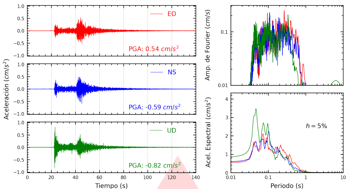
Figura A.35: Registros tiempo-historia, espectros de Fourier y de respuesta en las direcciones EO, NS y vertical de la estación CARAL. Sismo de Ricardo Palma, Huarochirí - Lima del 2026-07-22, 07:25:57 (Hora local)
