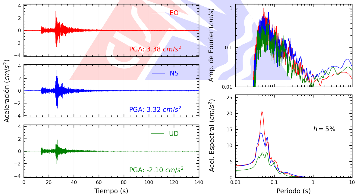
Figura A.24: Registros tiempo-historia, espectros de Fourier y de respuesta en las direcciones EO, NS y vertical de la estación CEPRE. Sismo de Ricardo Palma, Huarochirí - Lima del 2026-07-22, 07:25:57 (Hora local)
