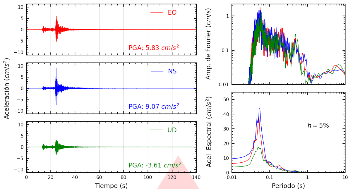
Figura A.9: Registros tiempo-historia, espectros de Fourier y de respuesta en las direcciones EO, NS y vertical de la estación IMCA. Sismo de Ricardo Palma, Huarochirí - Lima del 2026-07-22, 07:25:57 (Hora local)
