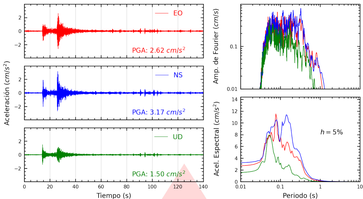
Figura A.25: Registros tiempo-historia, espectros de Fourier y de respuesta en las direcciones EO, NS y vertical de la estación BRISA. Sismo de Ricardo Palma, Huarochirí - Lima del 2026-07-22, 07:25:57 (Hora local)
