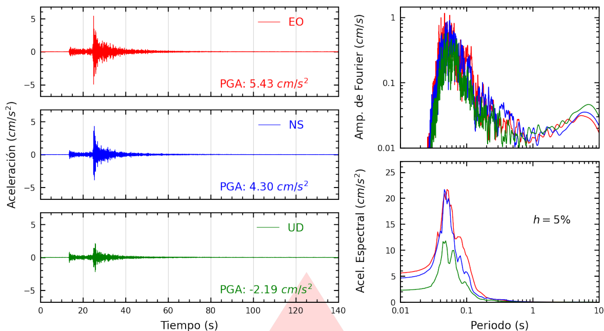
Figura A.17: Registros tiempo-historia, espectros de Fourier y de respuesta en las direcciones EO, NS y vertical de la estación UCSS. Sismo de Ricardo Palma, Huarochirí - Lima del 2026-07-22, 07:25:57 (Hora local)
