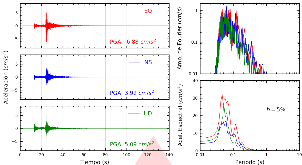
Figura A.15: Registros tiempo-historia, espectros de Fourier y de respuesta en las direcciones EO, NS y vertical de la estación ATARJ. Sismo de Ricardo Palma, Huarochirí - Lima del 2026-07-22, 07:25:57 (Hora local)
