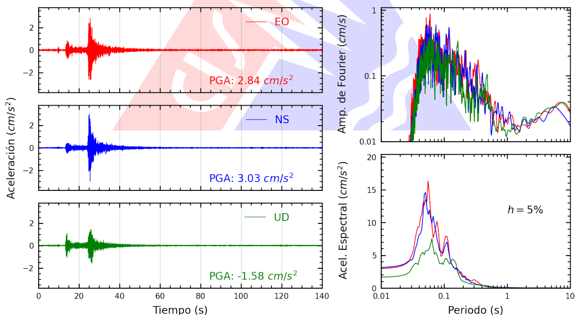
Figura A.26: Registros tiempo-historia, espectros de Fourier y de respuesta en las direcciones EO, NS y vertical de la estación INICT. Sismo de Ricardo Palma, Huarochirí - Lima del 2026-07-22, 07:25:57 (Hora local)
