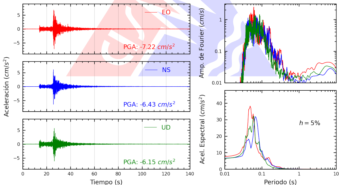
Figura A.14: Registros tiempo-historia, espectros de Fourier y de respuesta en las direcciones EO, NS y vertical de la estación AMORE. Sismo de Ricardo Palma, Huarochirí - Lima del 2026-07-22, 07:25:57 (Hora local)
