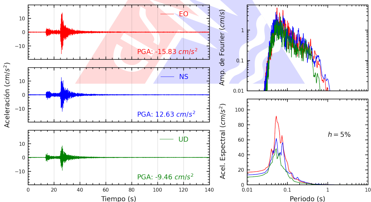
Figura A.2: Registros tiempo-historia, espectros de Fourier y de respuesta en las direcciones EO, NS y vertical de la estación UNTEL. Sismo de Ricardo Palma, Huarochirí - Lima del 2026-07-22, 07:25:57 (Hora local)
