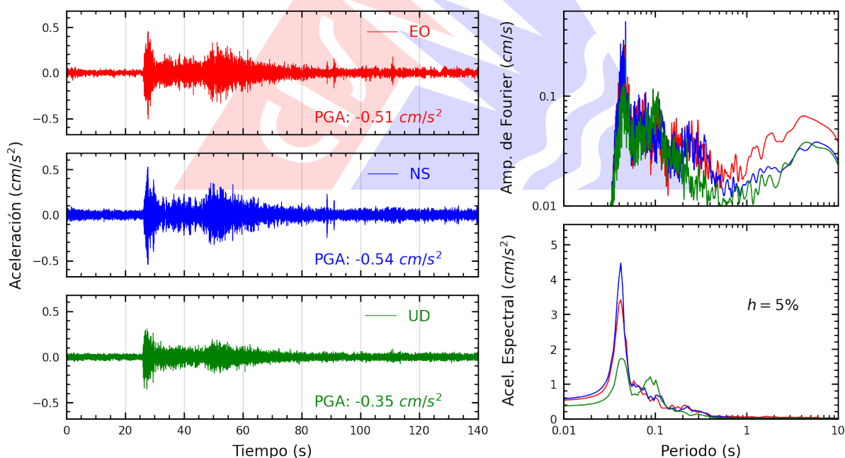
Figura A.36: Registros tiempo-historia, espectros de Fourier y de respuesta en las direcciones EO, NS y vertical de la estación UNAB. Sismo de Ricardo Palma, Huarochirí - Lima del 2026-07-22, 07:25:57 (Hora local)
