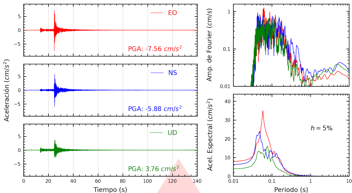
Figura A.13: Registros tiempo-historia, espectros de Fourier y de respuesta en las direcciones EO, NS y vertical de la estación JALVA. Sismo de Ricardo Palma, Huarochirí - Lima del 2026-07-22, 07:25:57 (Hora local)
