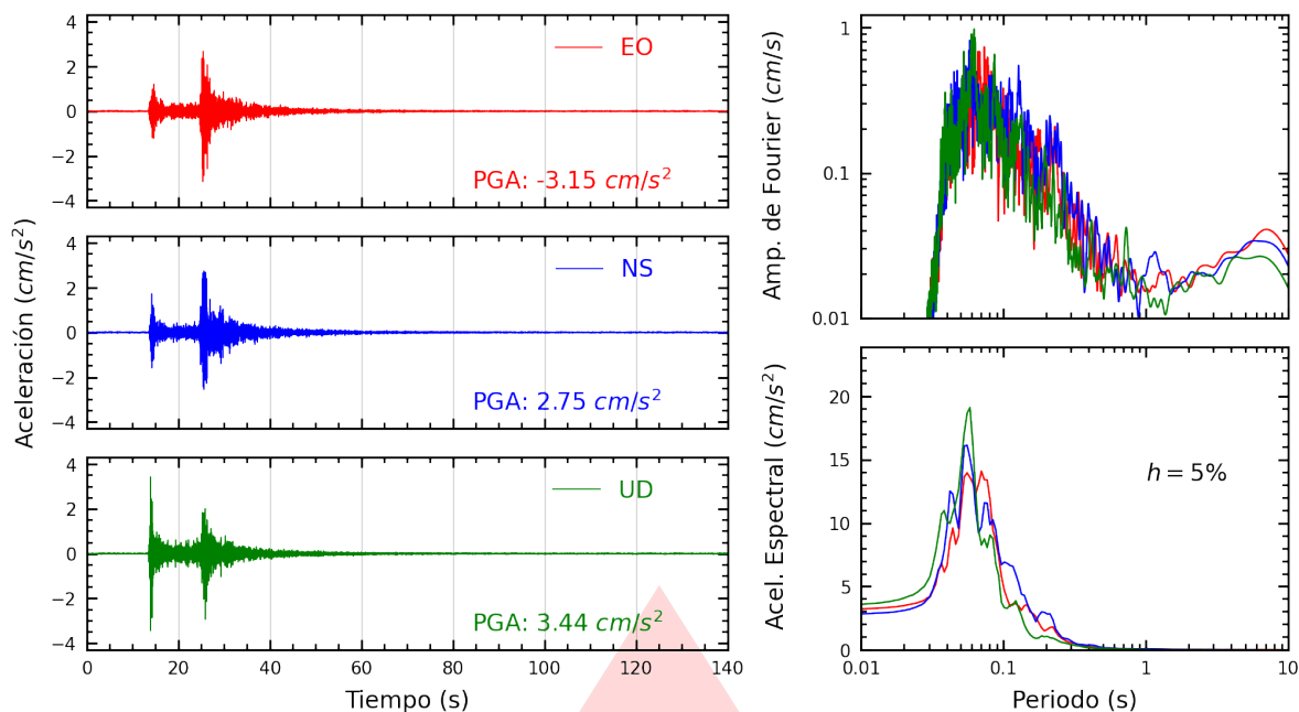
Figura A.23: Registros tiempo-historia, espectros de Fourier y de respuesta en las direcciones EO, NS y vertical de la estación SERVI. Sismo de Ricardo Palma, Huarochirí - Lima del 2026-07-22, 07:25:57 (Hora local)
