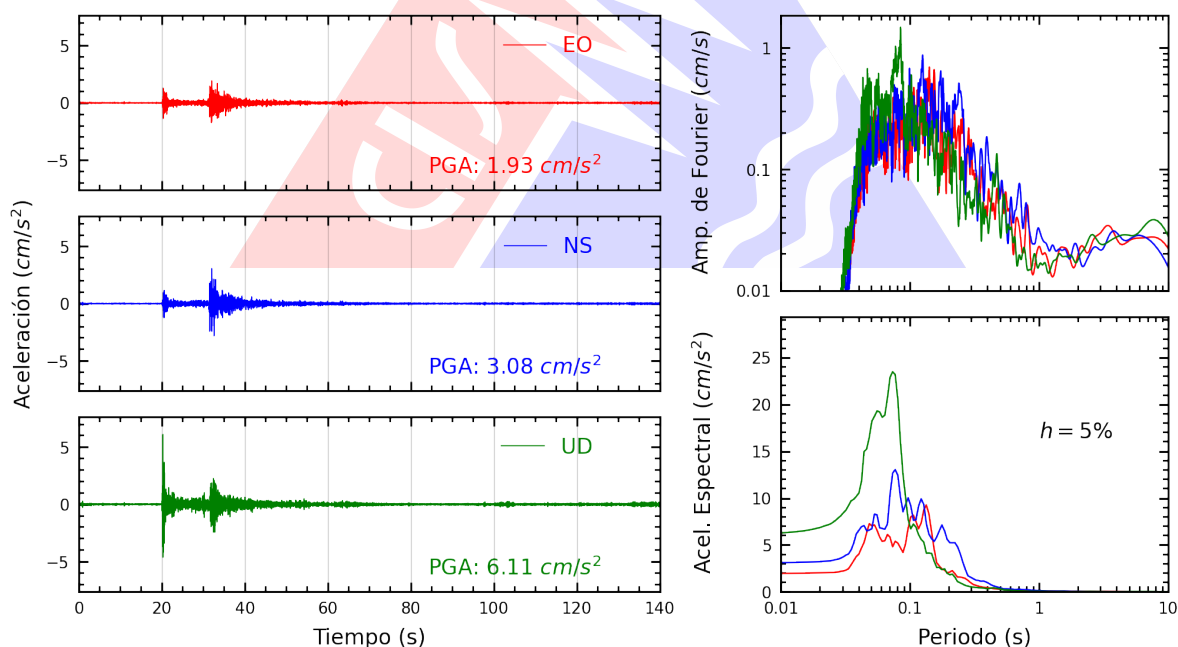
Figura A.16: Registros tiempo-historia, espectros de Fourier y de respuesta en las direcciones EO, NS y vertical de la estación SOCHO. Sismo de Ricardo Palma, Huarochirí - Lima del 2026-07-22, 07:25:57 (Hora local)
