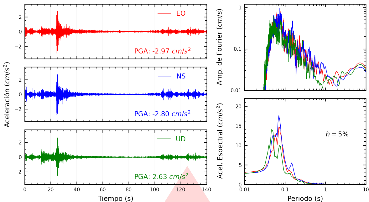
Figura A.27: Registros tiempo-historia, espectros de Fourier y de respuesta en las direcciones EO, NS y vertical de la estación UPCSM. Sismo de Ricardo Palma, Huarochirí - Lima del 2026-07-22, 07:25:57 (Hora local)
