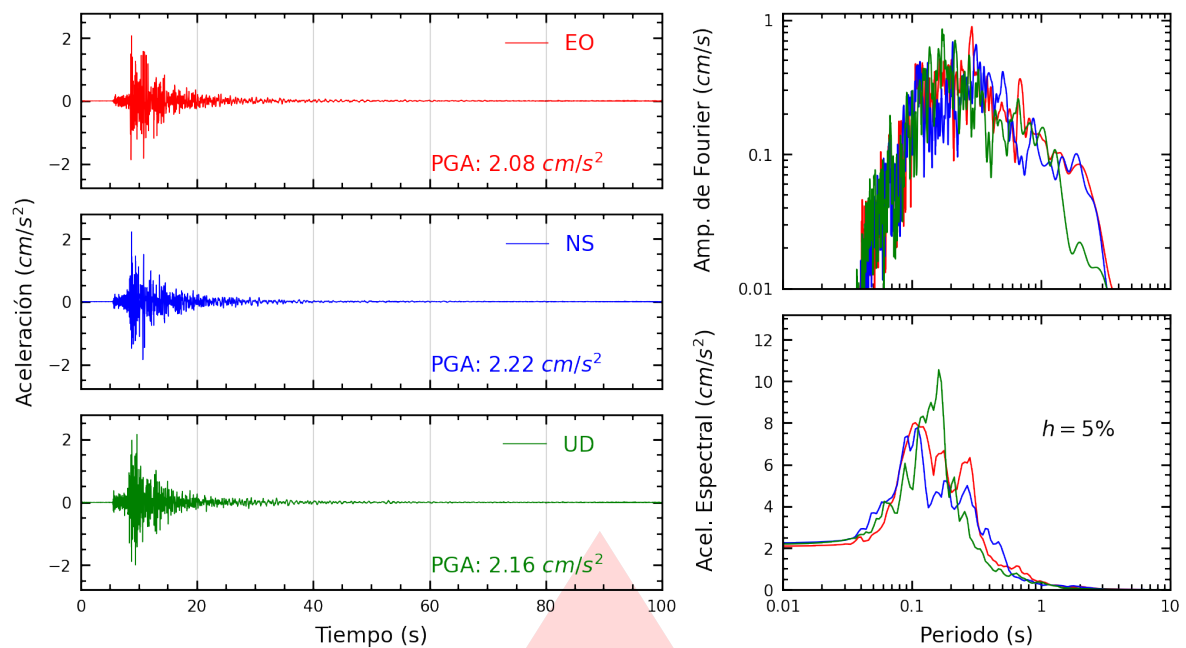
Figura A.1: Registros tiempo-historia, espectros de Fourier y de respuesta en las direcciones EO, NS y vertical de la estación UNCP. Sismo de Chupaca, Chupaca - Junín del 2026-07-22, 11:15:21 (Hora local)
