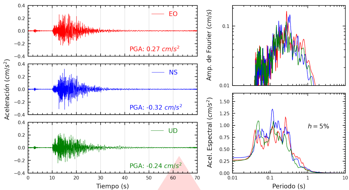
Figura A.1: Registros tiempo-historia, espectros de Fourier y de respuesta en las direcciones EO, NS y vertical de la estación UNCP. Sismo de Chupaca, Chupaca - Junín del 2026-07-22, 17:55:37 (Hora local)
