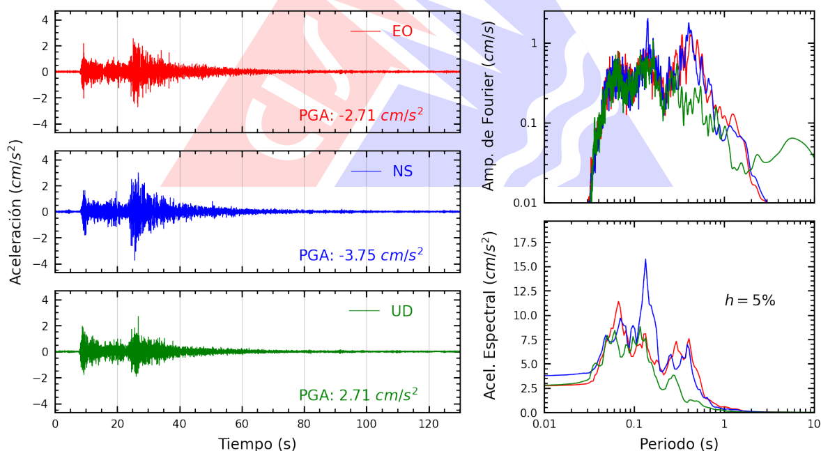
Figura A.2: Registros tiempo-historia, espectros de Fourier y de respuesta en las direcciones EO, NS y vertical de la estación SCARQ. Sismo de Camaná, Camaná - Arequipa del 2026-07-22, 21:38:25 (Hora local)
