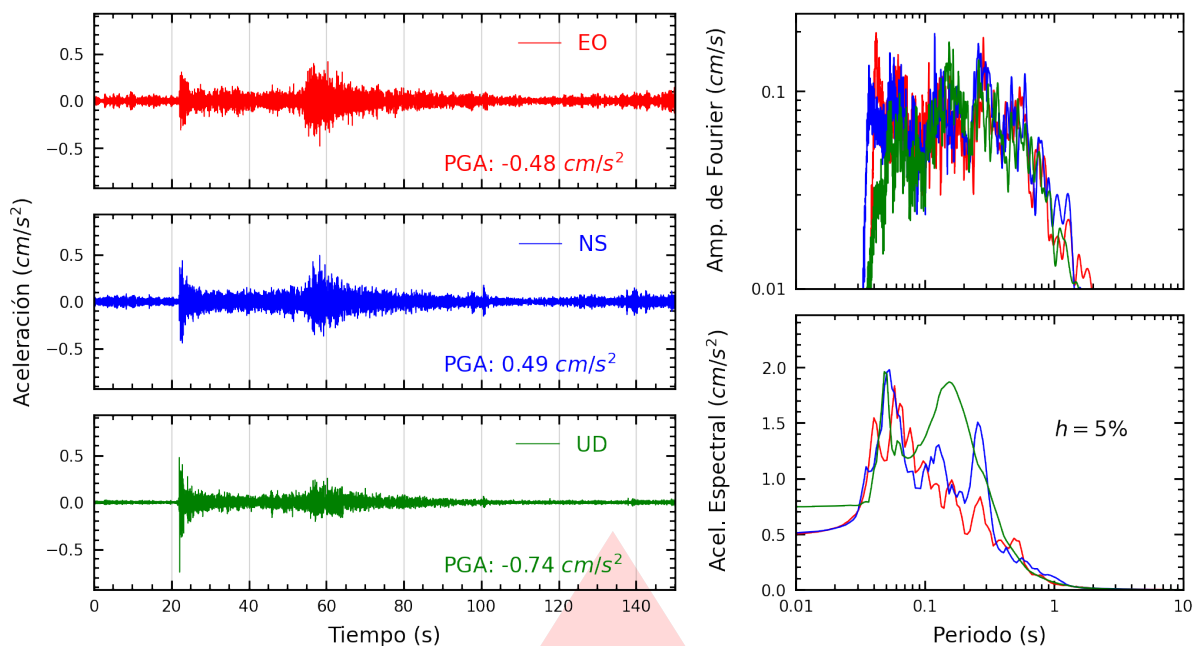
Figura A.5: Registros tiempo-historia, espectros de Fourier y de respuesta en las direcciones EO, NS y vertical de la estación UPTAC. Sismo de Camaná, Camaná - Arequipa del 2026-07-22, 21:38:25 (Hora local)
