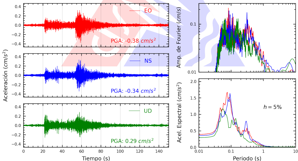
Figura A.6: Registros tiempo-historia, espectros de Fourier y de respuesta en las direcciones EO, NS y vertical de la estación CREY. Sismo de Camaná, Camaná - Arequipa del 2026-07-22, 21:38:25 (Hora local)
