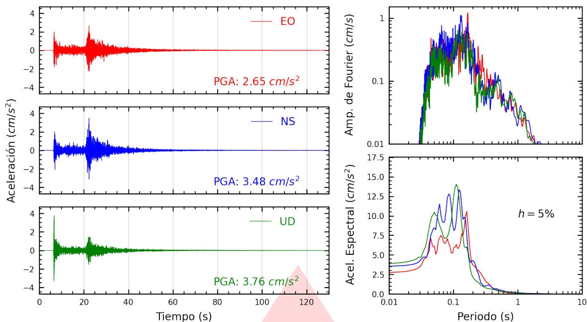
Figura A.1: Registros tiempo-historia, espectros de Fourier y de respuesta en las direcciones EO, NS y vertical de la estación UNSA2. Sismo de Camaná, Camaná - Arequipa del 2026-07-22, 21:38:25 (Hora local)
