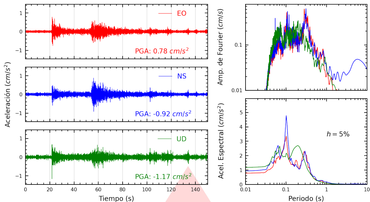
Figura A.3: Registros tiempo-historia, espectros de Fourier y de respuesta en las direcciones EO, NS y vertical de la estación SCTAC. Sismo de Camaná, Camaná - Arequipa del 2026-07-22, 21:38:25 (Hora local)
