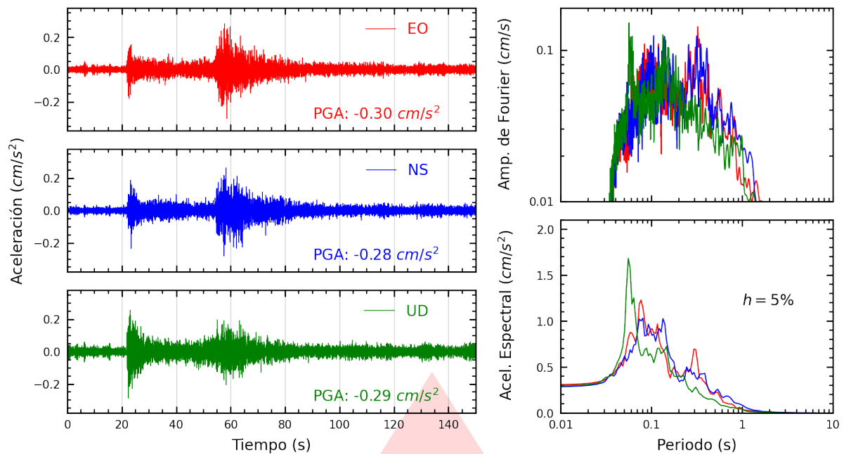
Figura A.7: Registros tiempo-historia, espectros de Fourier y de respuesta en las direcciones EO, NS y vertical de la estación UJBG2. Sismo de Camaná, Camaná - Arequipa del 2026-07-22, 21:38:25 (Hora local)
