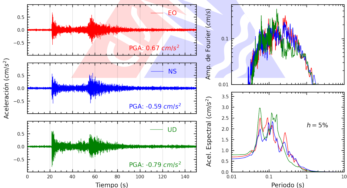
Figura A.4: Registros tiempo-historia, espectros de Fourier y de respuesta en las direcciones EO, NS y vertical de la estación UJBG4. Sismo de Camaná, Camaná - Arequipa del 2026-07-22, 21:38:25 (Hora local)
