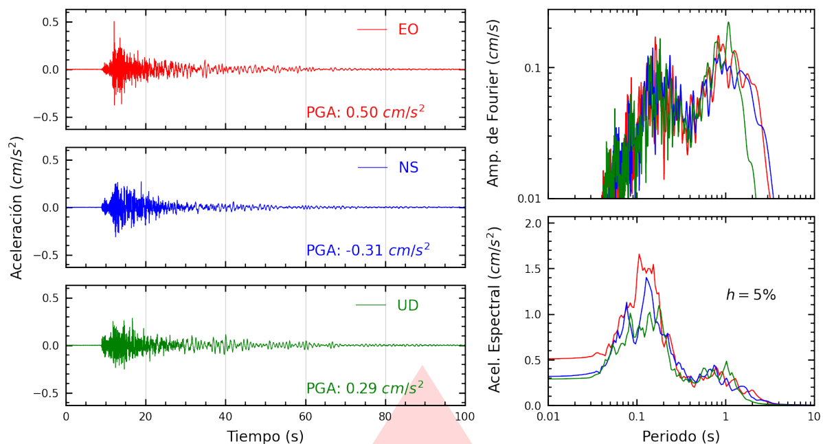
Figura A.1: Registros tiempo-historia, espectros de Fourier y de respuesta en las direcciones EO, NS y vertical de la estación UNCP. Sismo de Chupaca, Chupaca - Junín del 2026-07-23, 16:51:17 (Hora local)
