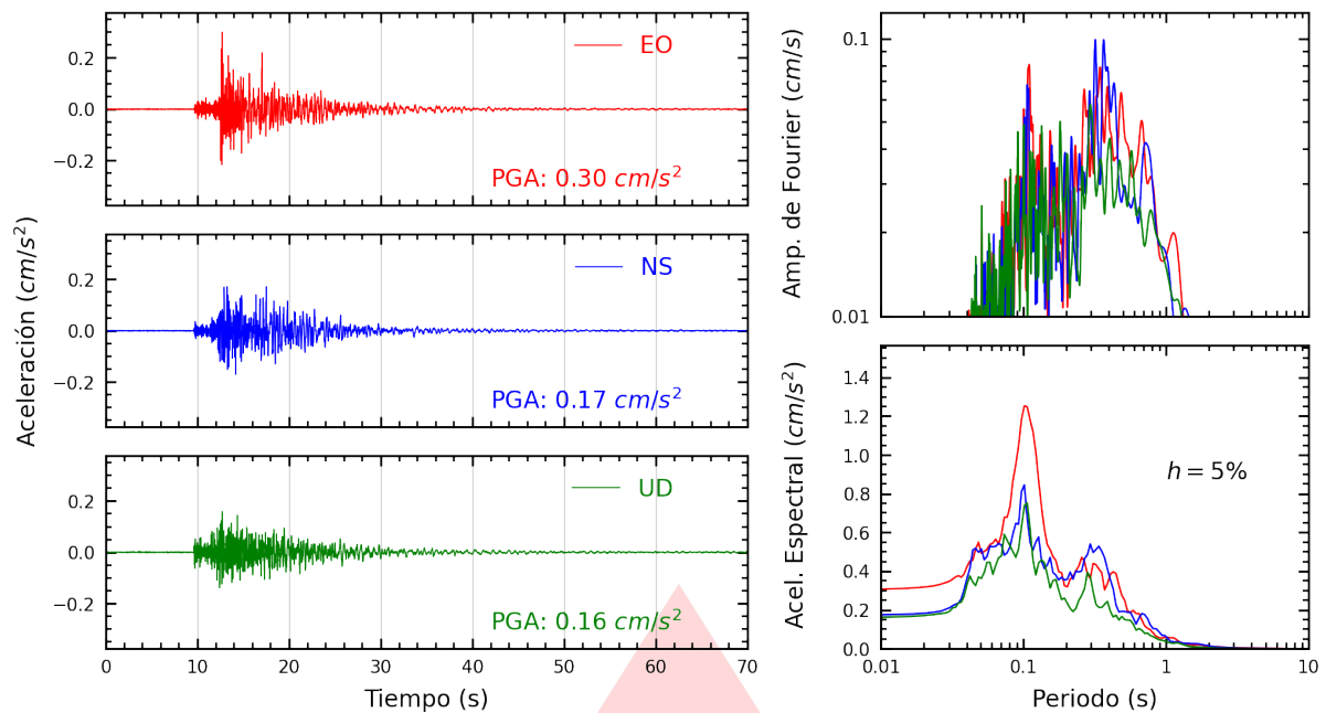
Figura A.1: Registros tiempo-historia, espectros de Fourier y de respuesta en las direcciones EO, NS y vertical de la estación UNCP. Sismo de Chupaca, Chupaca - Junín del 2026-07-27, 21:58:41 (Hora local)
