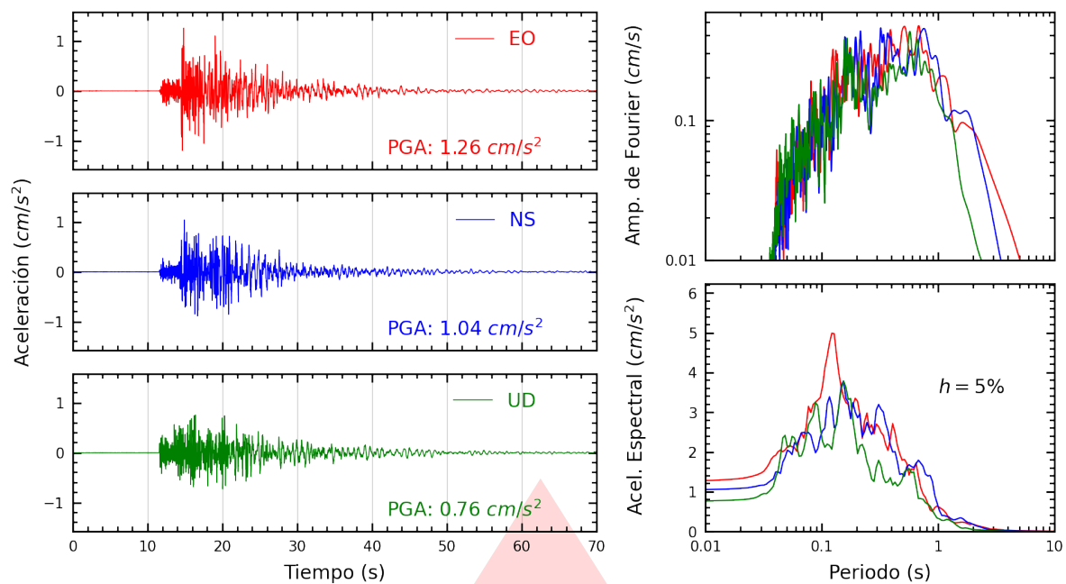
Figura A.1: Registros tiempo-historia, espectros de Fourier y de respuesta en las direcciones EO, NS y vertical de la estación UNCP. Sismo de Chupaca, Chupaca - Junín del 2026-07-29, 22:44:27 (Hora local)
