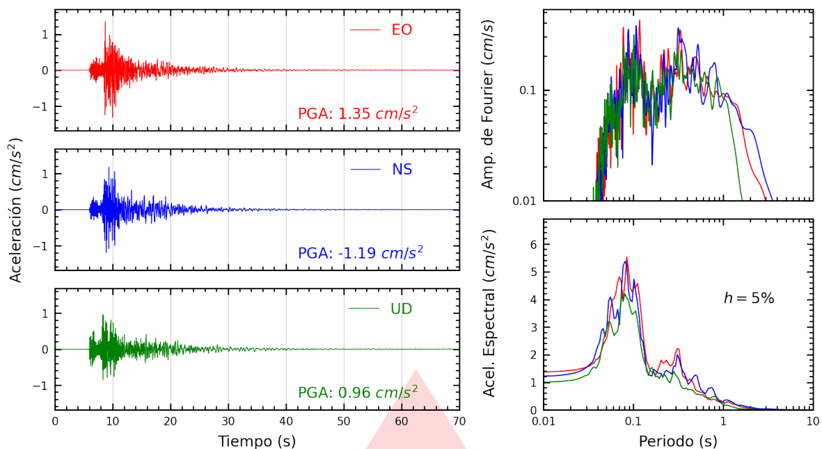
Figura A.1: Registros tiempo-historia, espectros de Fourier y de respuesta en las direcciones EO, NS y vertical de la estación UNCP. Sismo de Chupaca, Chupaca - Junín del 2026-07-31, 04:53:28 (Hora local)
