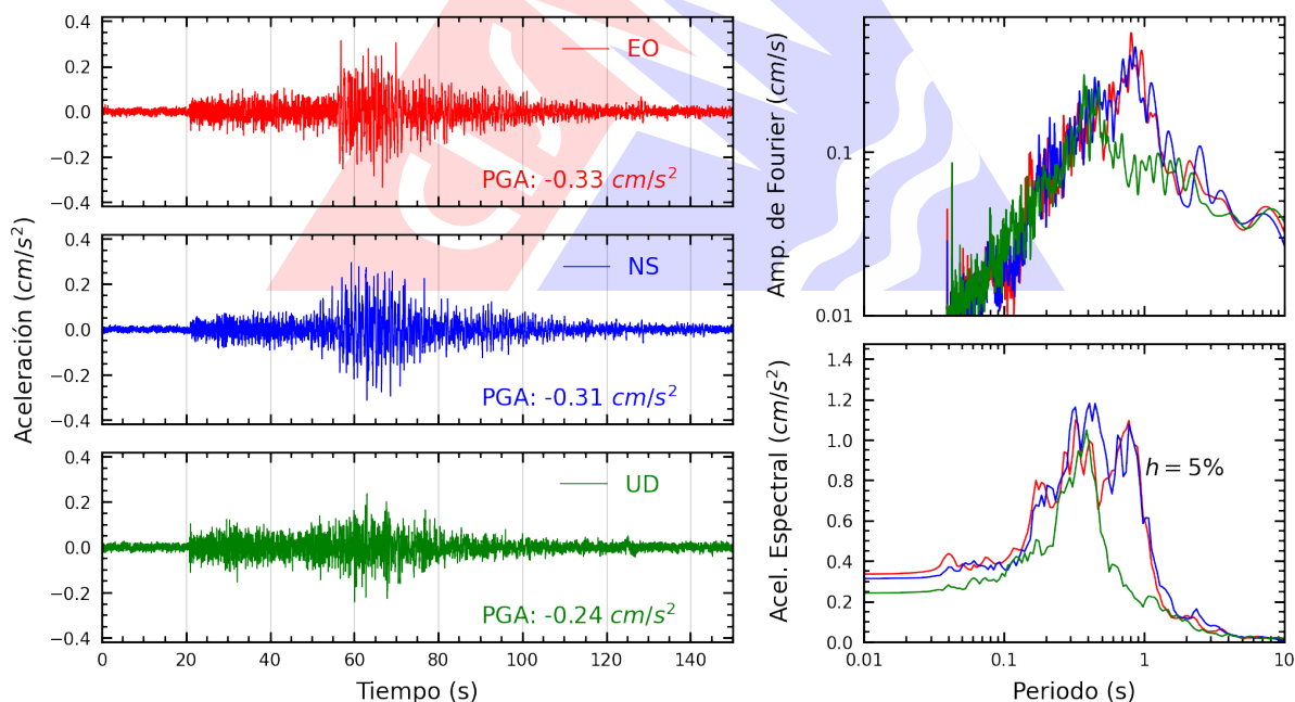
Figura A.28: Registros tiempo-historia, espectros de Fourier y de respuesta en las direcciones EO, NS y vertical de la estación UNMSM. Sismo de Huarney, Huarney - Áncash del 2026-07-11, 02:58:19 (Hora local)
