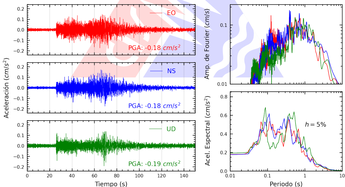
Figura A.34: Registros tiempo-historia, espectros de Fourier y de respuesta en las direcciones EO, NS y vertical de la estación ATARJ. Sismo de Huarney, Huarney - Áncash del 2026-07-11, 02:58:19 (Hora local)
