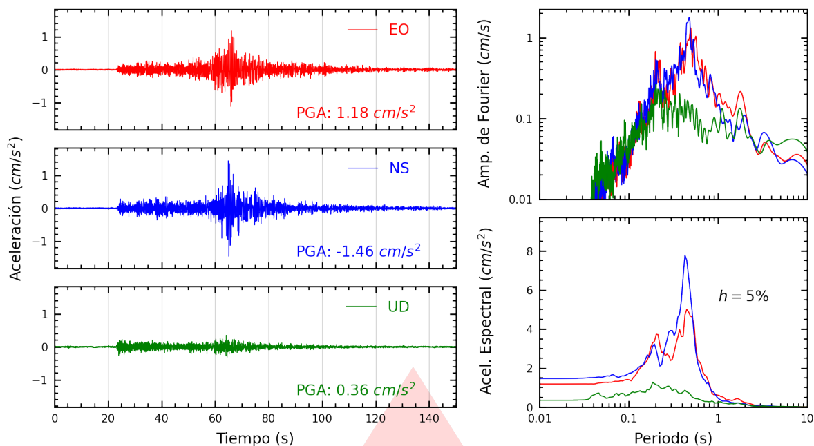
Figura A.3: Registros tiempo-historia, espectros de Fourier y de respuesta en las direcciones EO, NS y vertical de la estación VHAYA. Sismo de Huarney, Huarney - Áncash del 2026-07-11, 02:58:19 (Hora local)
