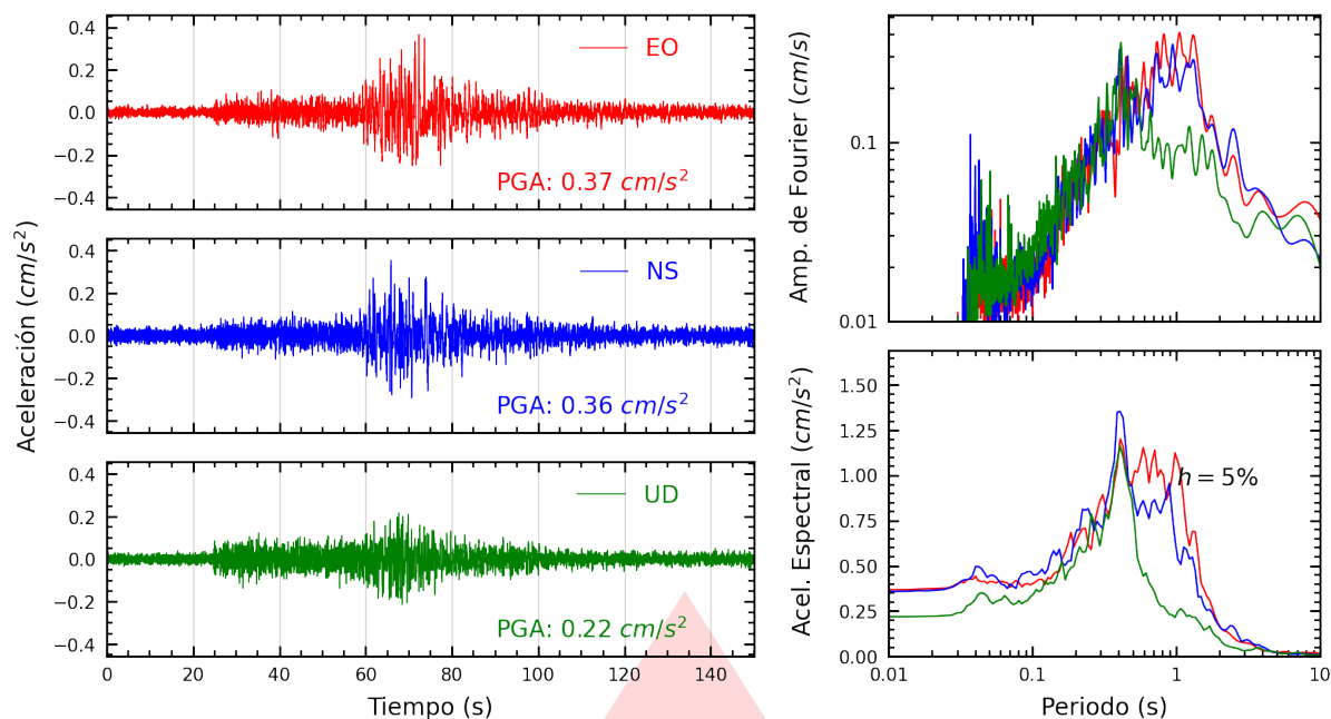
Figura A.25: Registros tiempo-historia, espectros de Fourier y de respuesta en las direcciones EO, NS y vertical de la estación BONDY. Sismo de Huarney, Huarney - Áncash del 2026-07-11, 02:58:19 (Hora local)
