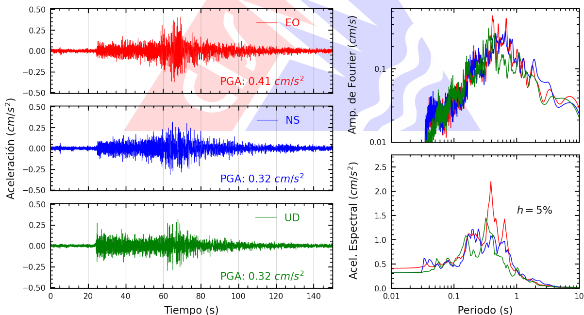
Figura A.20: Registros tiempo-historia, espectros de Fourier y de respuesta en las direcciones EO, NS y vertical de la estación COMAS. Sismo de Huarney, Huarney - Áncash del 2026-07-11, 02:58:19 (Hora local)
