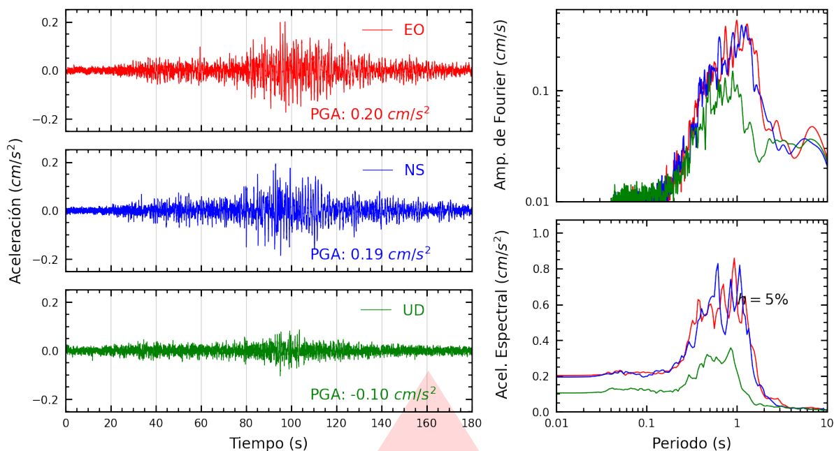
Figura A.33: Registros tiempo-historia, espectros de Fourier y de respuesta en las direcciones EO, NS y vertical de la estación UNTRM. Sismo de Huarney, Huarney - Áncash del 2026-07-11, 02:58:19 (Hora local)
