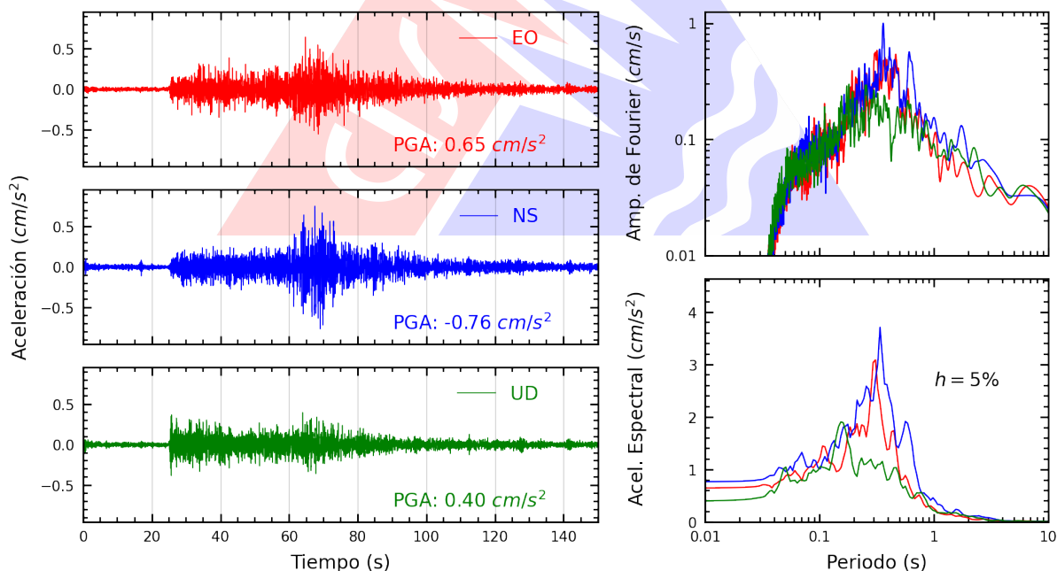
Figura A.8: Registros tiempo-historia, espectros de Fourier y de respuesta en las direcciones EO, NS y vertical de la estación SJLSC. Sismo de Huarney, Huarney - Áncash del 2026-07-11, 02:58:19 (Hora local)
