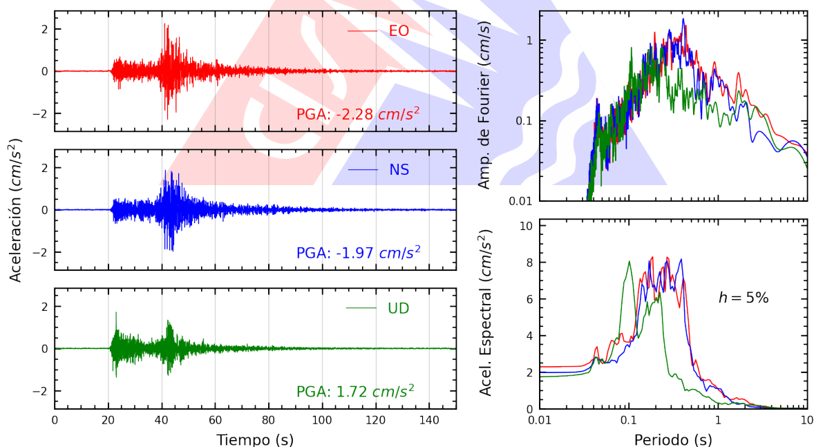
Figura A.2: Registros tiempo-historia, espectros de Fourier y de respuesta en las direcciones EO, NS y vertical de la estación UNAB. Sismo de Huarney, Huarney - Áncash del 2026-07-11, 02:58:19 (Hora local)
