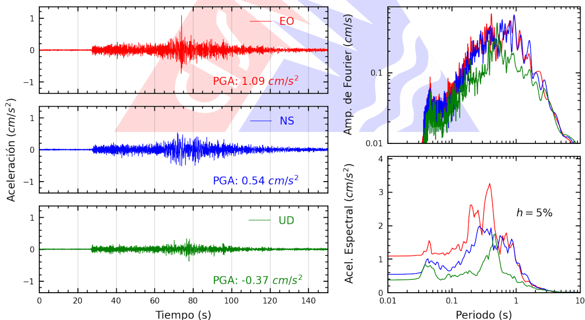
Figura A.4: Registros tiempo-historia, espectros de Fourier y de respuesta en las direcciones EO, NS y vertical de la estación BRISA. Sismo de Huarney, Huarney - Áncash del 2026-07-11, 02:58:19 (Hora local)
