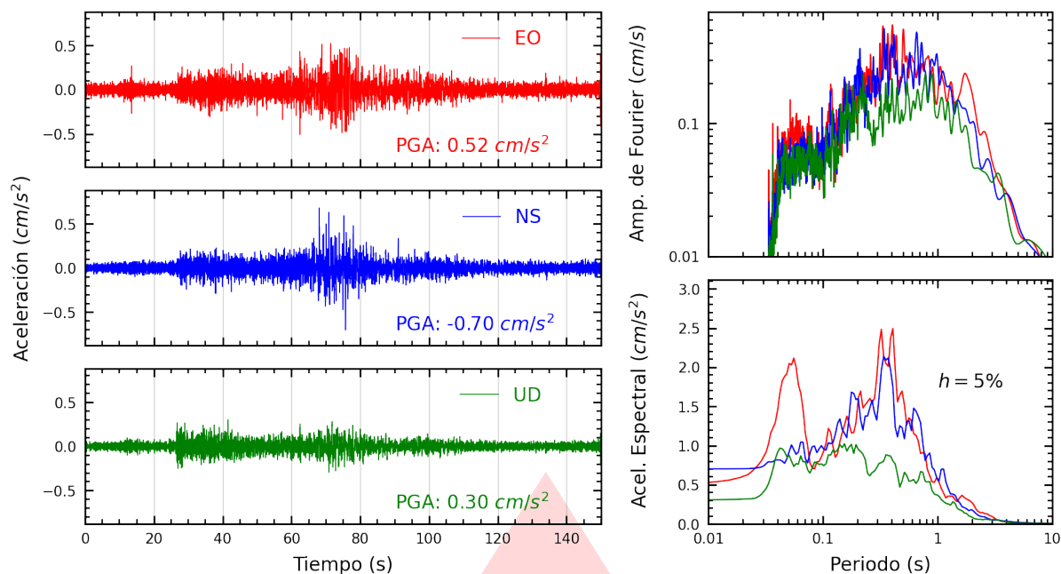
Figura A.9: Registros tiempo-historia, espectros de Fourier y de respuesta en las direcciones EO, NS y vertical de la estación SOBAR. Sismo de Huarney, Huarney - Áncash del 2026-07-11, 02:58:19 (Hora local)
