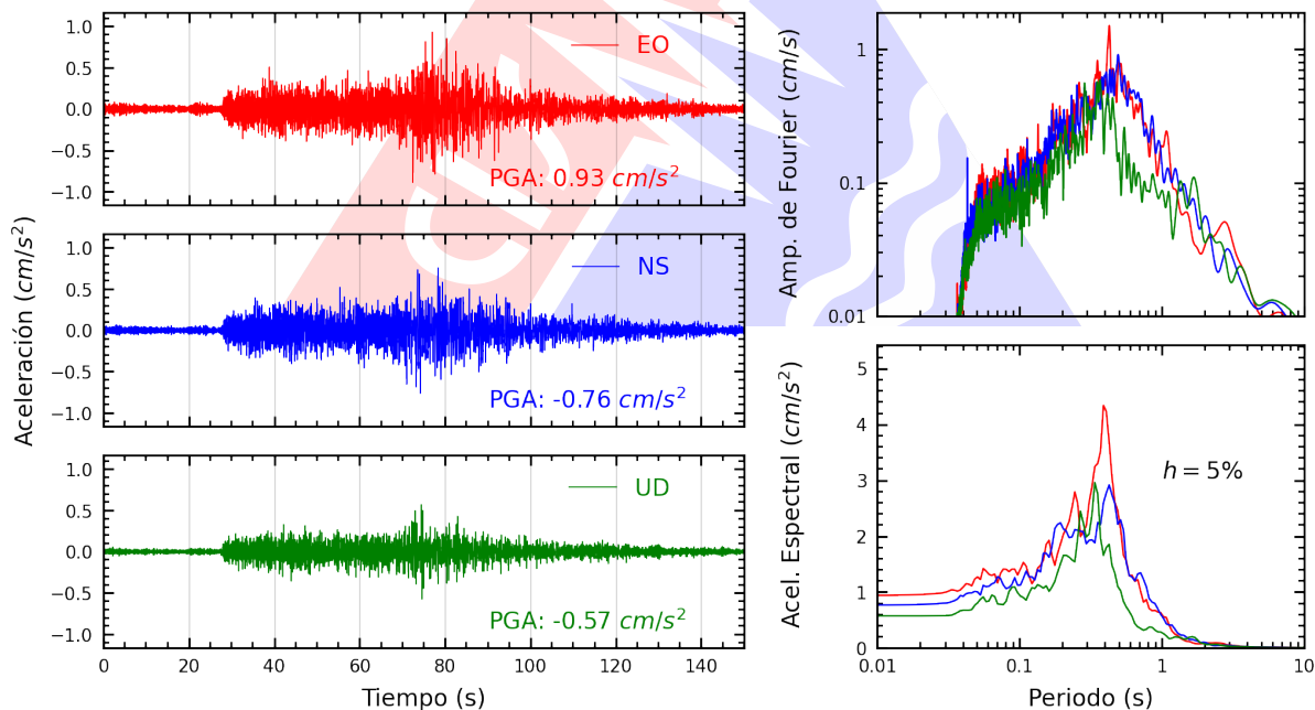
Figura A.6: Registros tiempo-historia, espectros de Fourier y de respuesta en las direcciones EO, NS y vertical de la estación UNTEL. Sismo de Huarmey, Huarmey - Áncash del 2026-07-11, 02:58:19 (Hora local)
