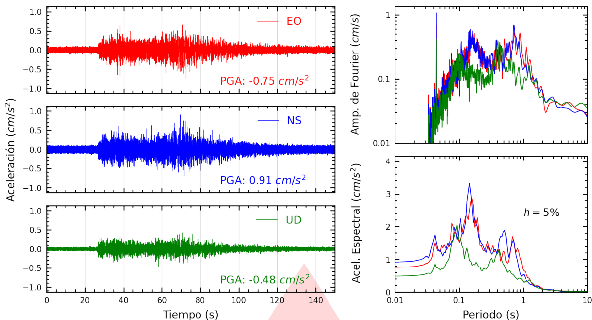
Figura A.7: Registros tiempo-historia, espectros de Fourier y de respuesta en las direcciones EO, NS y vertical de la estación USILM. Sismo de Huarney, Huarney - Áncash del 2026-07-11, 02:58:19 (Hora local)
