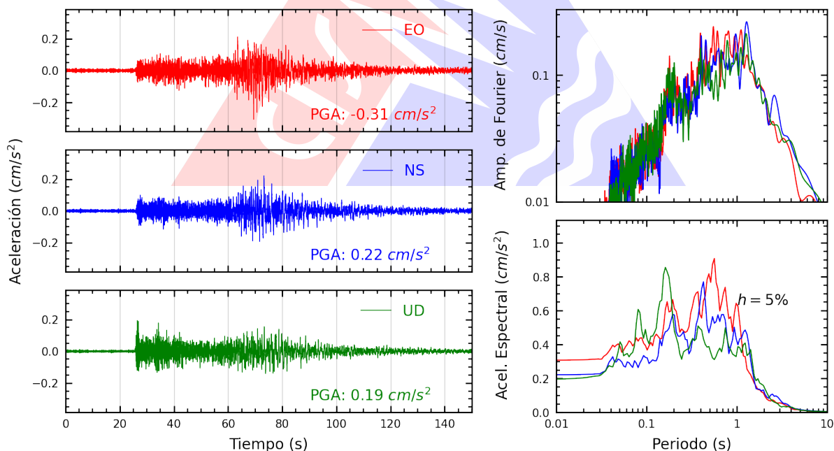
Figura A.30: Registros tiempo-historia, espectros de Fourier y de respuesta en las direcciones EO, NS y vertical de la estación BORJA. Sismo de Huarney, Huarney - Áncash del 2026-07-11, 02:58:19 (Hora local)
