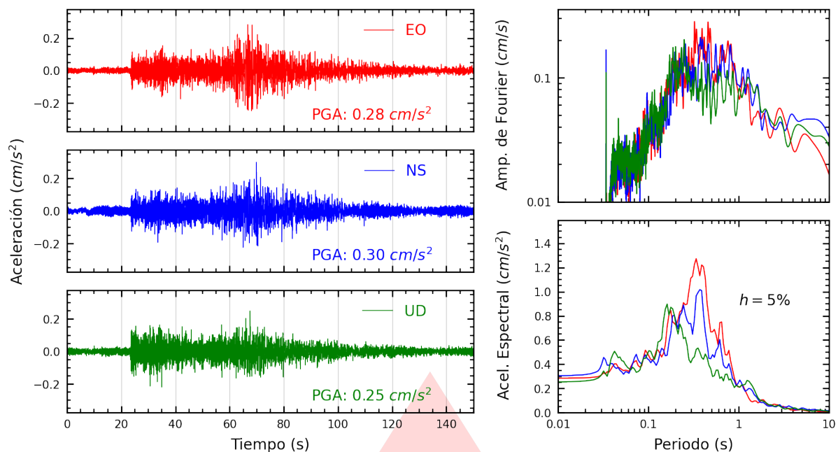
Figura A.31: Registros tiempo-historia, espectros de Fourier y de respuesta en las direcciones EO, NS y vertical de la estación USMP. Sismo de Huarney, Huarney - Áncash del 2026-07-11, 02:58:19 (Hora local)
