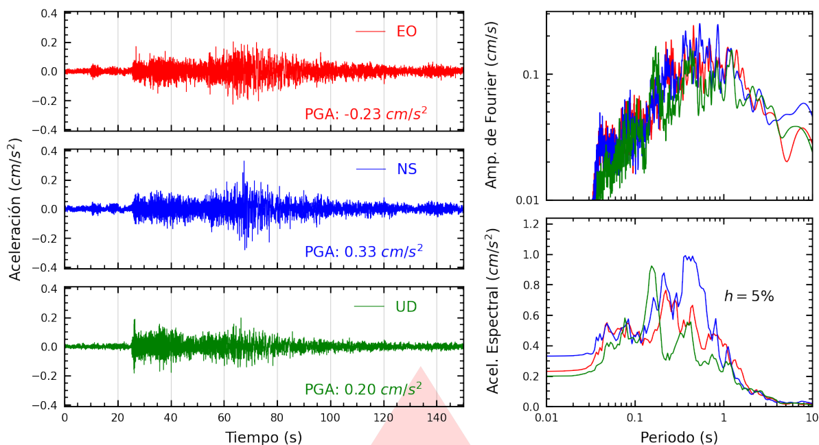
Figura A.29: Registros tiempo-historia, espectros de Fourier y de respuesta en las direcciones EO, NS y vertical de la estación CEPRE. Sismo de Huarney, Huarney - Áncash del 2026-07-11, 02:58:19 (Hora local)
