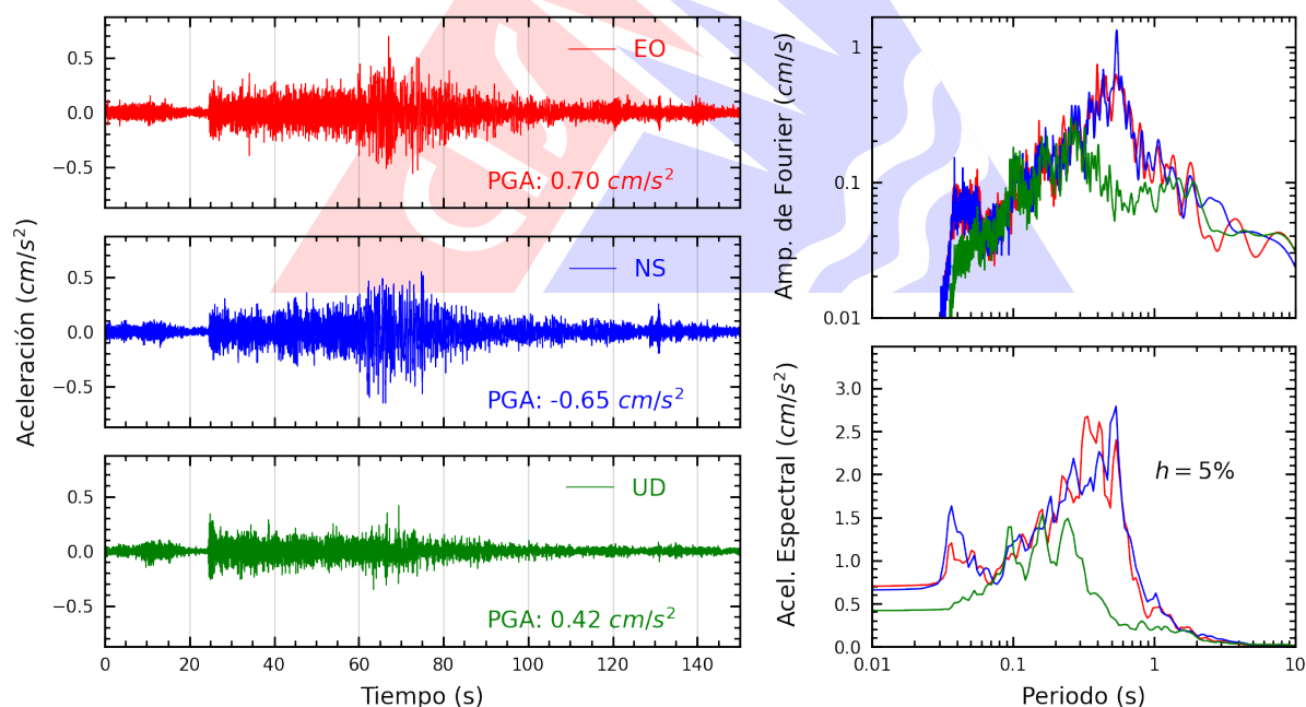
Figura A.10: Registros tiempo-historia, espectros de Fourier y de respuesta en las direcciones EO, NS y vertical de la estación OLIVO. Sismo de Huarney, Huarney - Áncash del 2026-07-11, 02:58:19 (Hora local)
