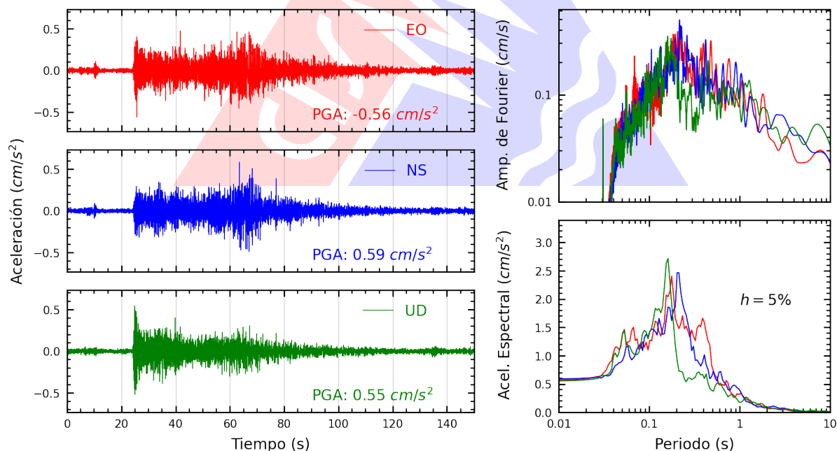
Figura A.14: Registros tiempo-historia, espectros de Fourier y de respuesta en las direcciones EO, NS y vertical de la estación INDEP. Sismo de Huarney, Huarney - Áncash del 2026-07-11, 02:58:19 (Hora local)
