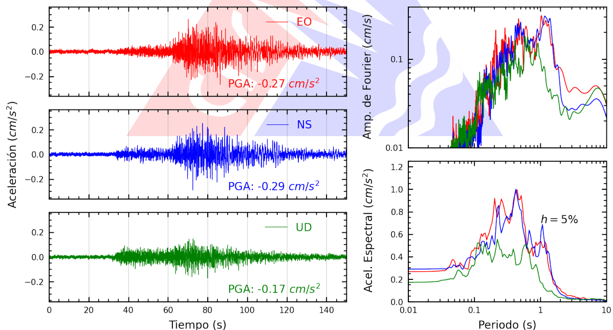
Figura A.32: Registros tiempo-historia, espectros de Fourier y de respuesta en las direcciones EO, NS y vertical de la estación UPAOT. Sismo de Huarney, Huarney - Áncash del 2026-07-11, 02:58:19 (Hora local)
