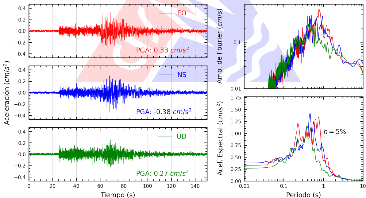
Figura A.22: Registros tiempo-historia, espectros de Fourier y de respuesta en las direcciones EO, NS y vertical de la estación UNFV. Sismo de Huarmey, Huarmey - Áncash del 2026-07-11, 02:58:19 (Hora local)
