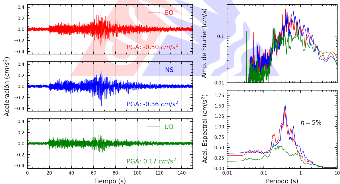
Figura A.26: Registros tiempo-historia, espectros de Fourier y de respuesta en las direcciones EO, NS y vertical de la estación UPCVI. Sismo de Huarney, Huarney - Áncash del 2026-07-11, 02:58:19 (Hora local)
