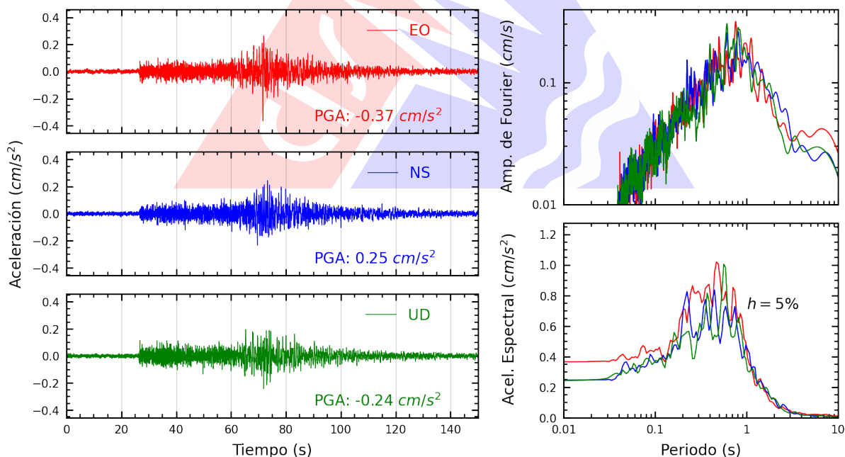
Figura A.24: Registros tiempo-historia, espectros de Fourier y de respuesta en las direcciones EO, NS y vertical de la estación SERVI. Sismo de Huarmey, Huarmey - Áncash del 2026-07-11, 02:58:19 (Hora local)
