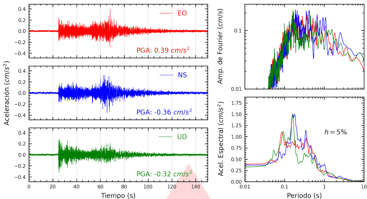
Figura A.21: Registros tiempo-historia, espectros de Fourier y de respuesta en las direcciones EO, NS y vertical de la estación JALVA. Sismo de Huarmey, Huarmey - Áncash del 2026-07-11, 02:58:19 (Hora local)
