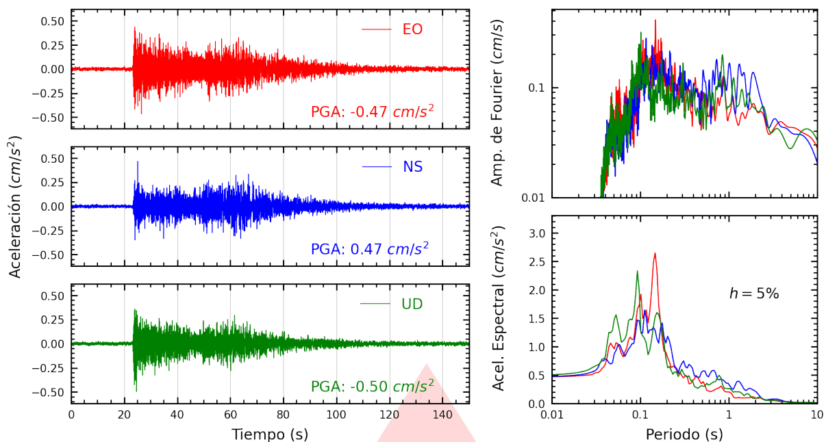
Figura A.17: Registros tiempo-historia, espectros de Fourier y de respuesta en las direcciones EO, NS y vertical de la estación AMORE. Sismo de Huarney, Huarney - Áncash del 2026-07-11, 02:58:19 (Hora local)
