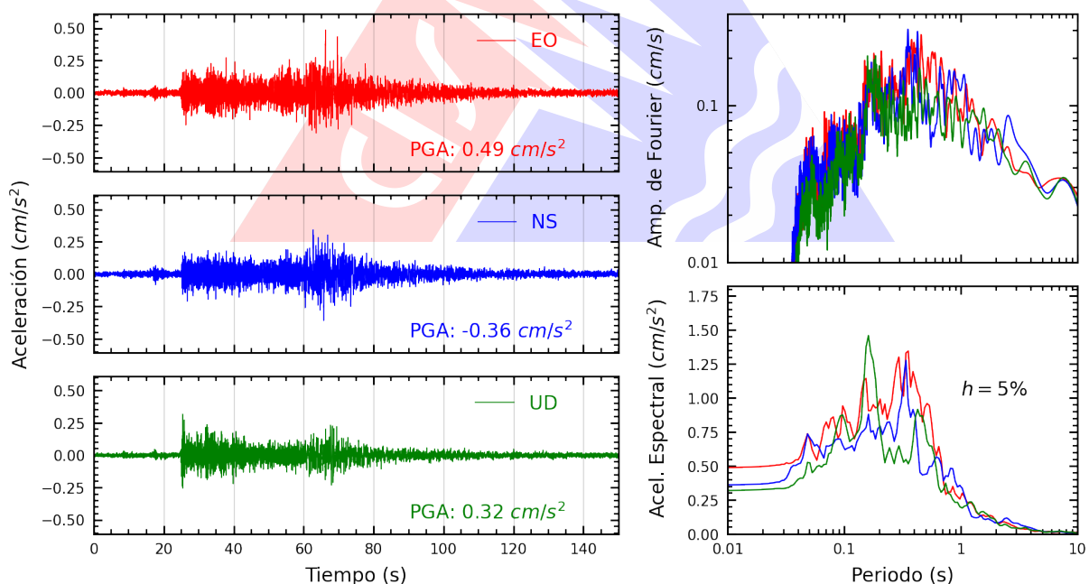
Figura A.18: Registros tiempo-historia, espectros de Fourier y de respuesta en las direcciones EO, NS y vertical de la estación FICPE. Sismo de Huarney, Huarney - Áncash del 2026-07-11, 02:58:19 (Hora local)
