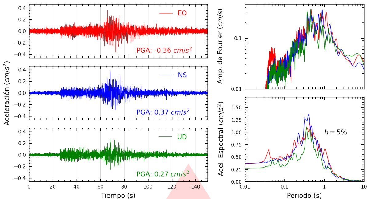
Figura A.23: Registros tiempo-historia, espectros de Fourier y de respuesta en las direcciones EO, NS y vertical de la estación INICT. Sismo de Huarmey, Huarmey - Áncash del 2026-07-11, 02:58:19 (Hora local)
