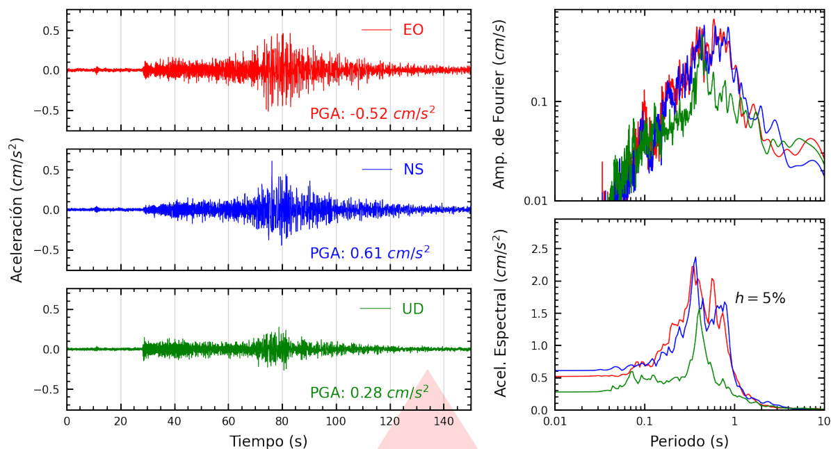
Figura A.13: Registros tiempo-historia, espectros de Fourier y de respuesta en las direcciones EO, NS y vertical de la estación USILP. Sismo de Huarney, Huarney - Áncash del 2026-07-11, 02:58:19 (Hora local)
