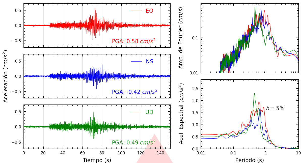
Figura A.15: Registros tiempo-historia, espectros de Fourier y de respuesta en las direcciones EO, NS y vertical de la estación IMCA. Sismo de Huarney, Huarney - Áncash del 2026-07-11, 02:58:19 (Hora local)
