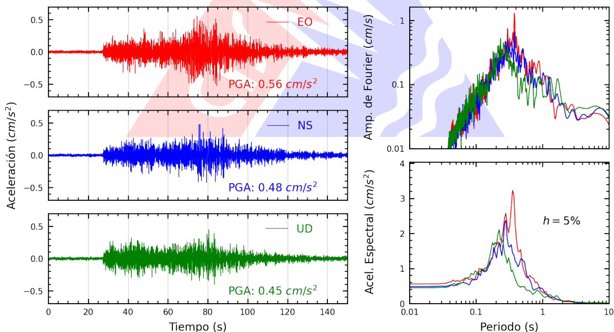
Figura A.16: Registros tiempo-historia, espectros de Fourier y de respuesta en las direcciones EO, NS y vertical de la estación SOVES. Sismo de Huarney, Huarney - Áncash del 2026-07-11, 02:58:19 (Hora local)
