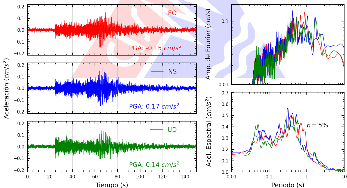
Figura A.36: Registros tiempo-historia, espectros de Fourier y de respuesta en las direcciones EO, NS y vertical de la estación SJLCE. Sismo de Huarney, Huarney - Áncash del 2026-07-11, 02:58:19 (Hora local)
