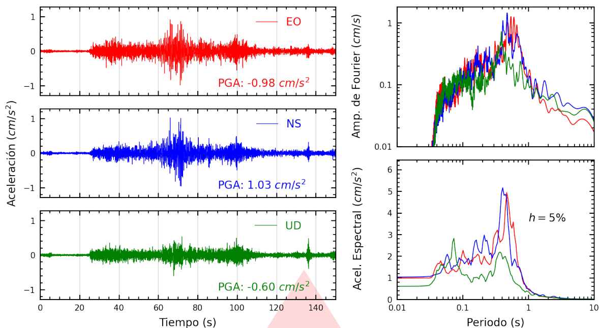
Figura A.5: Registros tiempo-historia, espectros de Fourier y de respuesta en las direcciones EO, NS y vertical de la estación SJLSV. Sismo de Huarmey, Huarmey - Áncash del 2026-07-11, 02:58:19 (Hora local)
