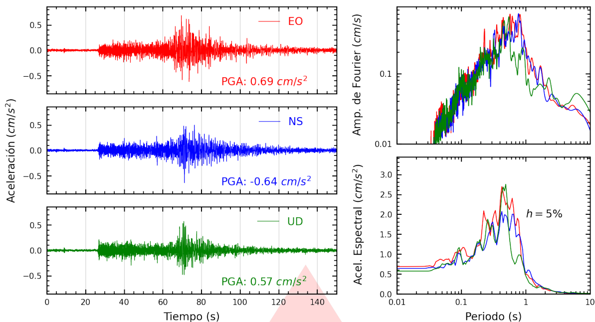
Figura A.11: Registros tiempo-historia, espectros de Fourier y de respuesta en las direcciones EO, NS y vertical de la estación UCVAT. Sismo de Huarney, Huarney - Áncash del 2026-07-11, 02:58:19 (Hora local)
