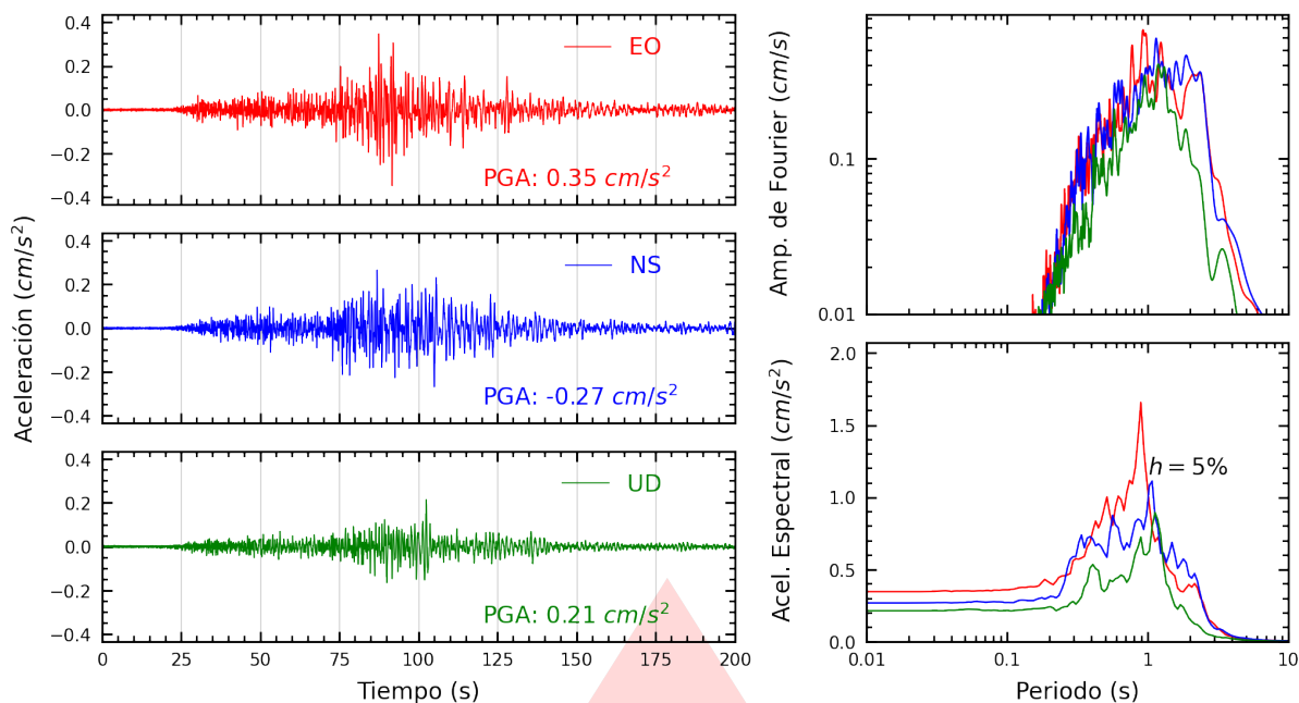
Figura A.27: Registros tiempo-historia, espectros de Fourier y de respuesta en las direcciones EO, NS y vertical de la estación UNC. Sismo de Huarney, Huarney - Áncash del 2026-07-11, 02:58:19 (Hora local)
