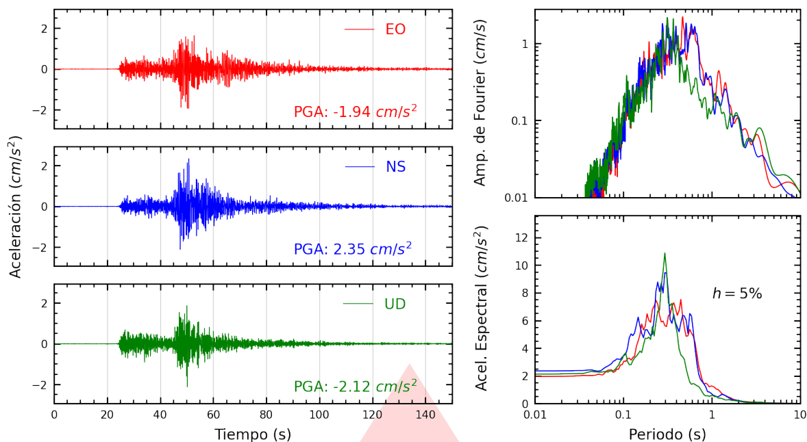
Figura A.1: Registros tiempo-historia, espectros de Fourier y de respuesta en las direcciones EO, NS y vertical de la estación CARAL. Sismo de Huarney, Huarney - Áncash del 2026-07-11, 02:58:19 (Hora local)
