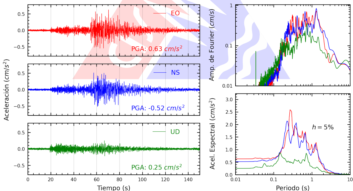
Figura A.12: Registros tiempo-historia, espectros de Fourier y de respuesta en las direcciones EO, NS y vertical de la estación DSML. Sismo de Huarney, Huarney - Áncash del 2026-07-11, 02:58:19 (Hora local)
