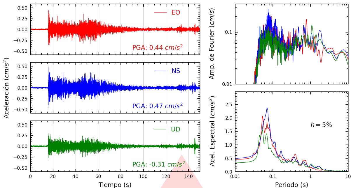
Figura A.19: Registros tiempo-historia, espectros de Fourier y de respuesta en las direcciones EO, NS y vertical de la estación JOSEO. Sismo de Huarney, Huarney - Áncash del 2026-07-11, 02:58:19 (Hora local)
