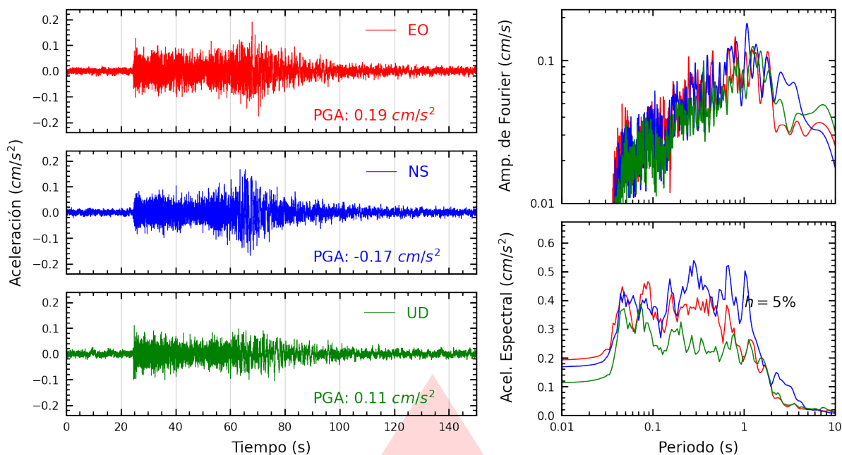
Figura A.35: Registros tiempo-historia, espectros de Fourier y de respuesta en las direcciones EO, NS y vertical de la estación UCSS. Sismo de Huarney, Huarney - Áncash del 2026-07-11, 02:58:19 (Hora local)
