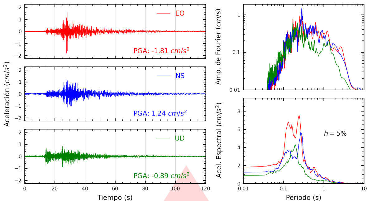
Figura A.1: Registros tiempo-historia, espectros de Fourier y de respuesta en las direcciones EO, NS y vertical de la estación UNICA. Sismo de Ica, Ica - Ica del 2026-07-14, 21:40:25 (Hora local)
