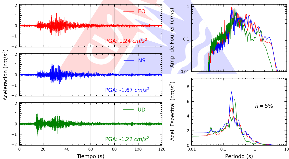
Figura A.2: Registros tiempo-historia, espectros de Fourier y de respuesta en las direcciones EO, NS y vertical de la estación SCICA. Sismo de Ica, Ica - Ica del 2026-07-14, 21:40:25 (Hora local)
