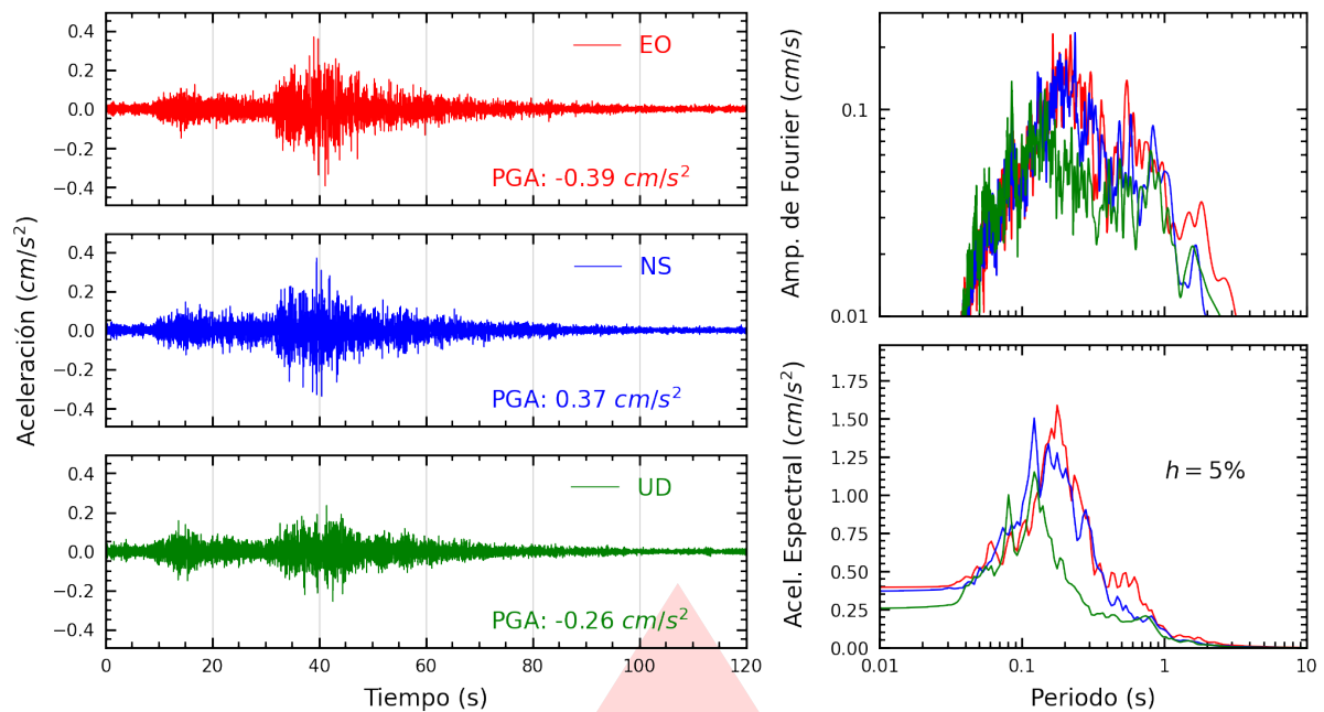
Figura A.3: Registros tiempo-historia, espectros de Fourier y de respuesta en las direcciones EO, NS y vertical de la estación ASIA. Sismo de Ica, Ica - Ica del 2026-07-14, 21:40:25 (Hora local)
