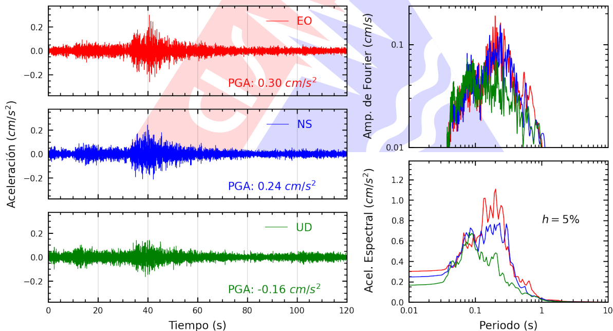
Figura A.2: Registros tiempo-historia, espectros de Fourier y de respuesta en las direcciones EO, NS y vertical de la estación ASIA. Sismo de Ica, Ica - Ica del 2026-07-14, 23:40:17 (Hora local)
