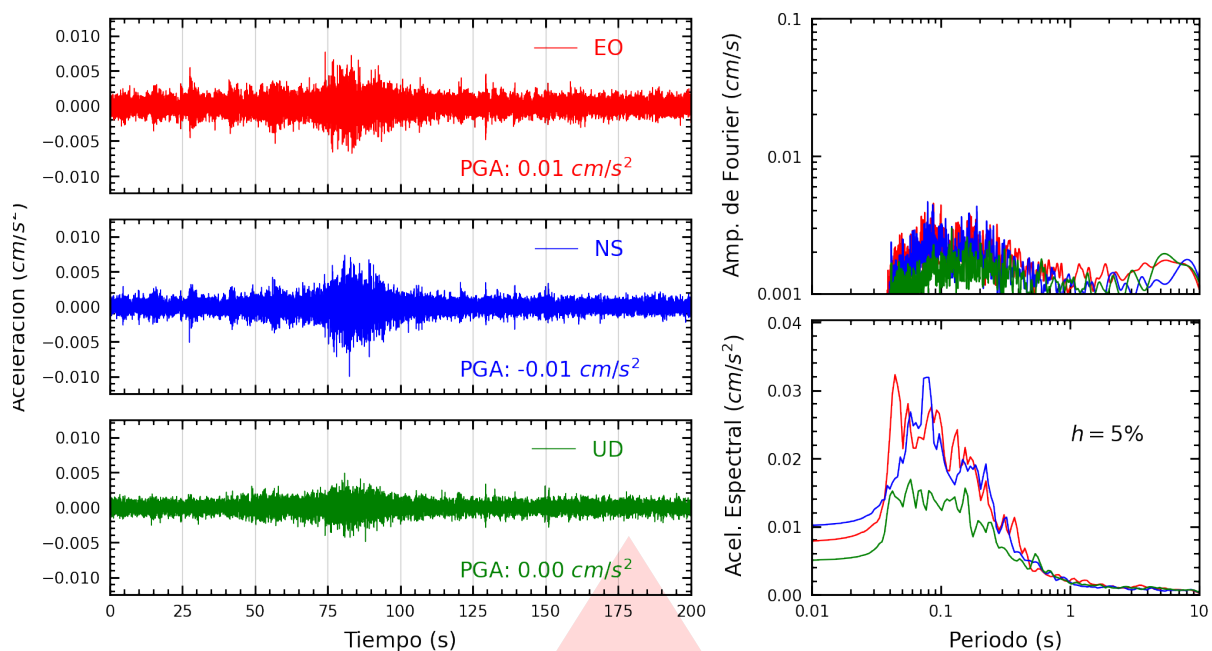
Figura A.1: Registros tiempo-historia, espectros de Fourier y de respuesta en las direcciones EO, NS y vertical de la estación UNSA2. Sismo de Chala, Caravelí - Arequipa del 2026-07-17, 01:41:33 (Hora local)
