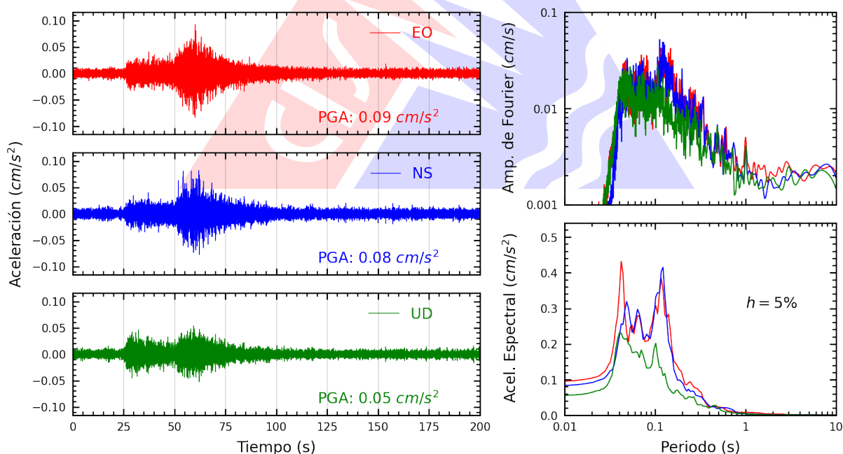
Figura A.22: Registros tiempo-historia, espectros de Fourier y de respuesta en las direcciones EO, NS y vertical de la estación ATARJ. Sismo de Castrovirreyna, Castrovirreyna - Huancavelica del 2026-07-17, 04:16:31 (Hora local)
