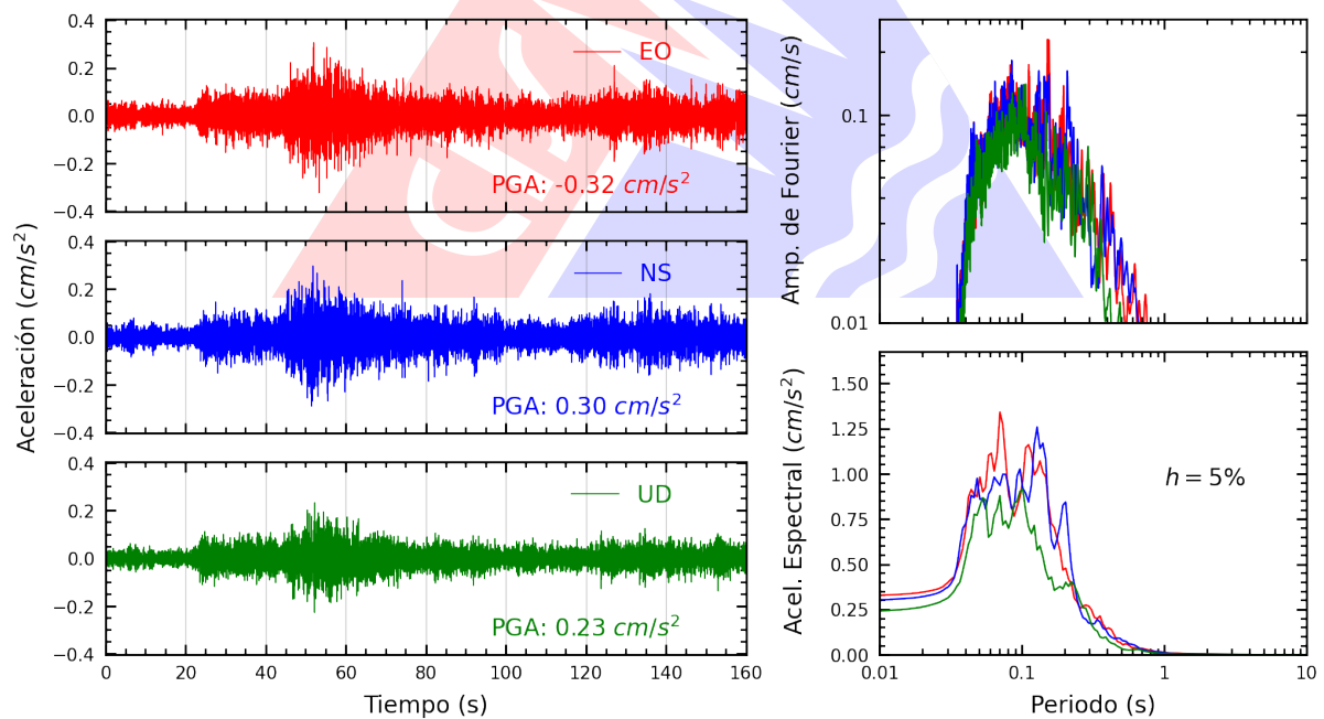
Figura A.4: Registros tiempo-historia, espectros de Fourier y de respuesta en las direcciones EO, NS y vertical de la estación PHERM. Sismo de Castrovirreyna, Castrovirreyna - Huancavelica del 2026-07-17, 04:16:31 (Hora local)
