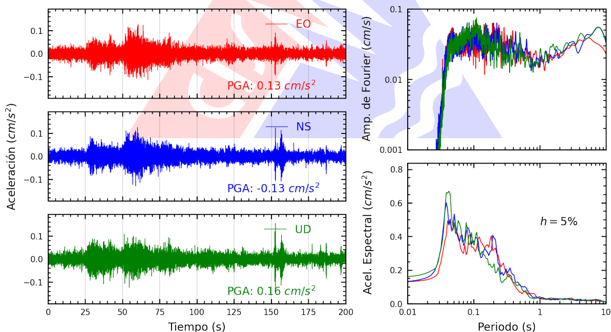
Figura A.12: Registros tiempo-historia, espectros de Fourier y de respuesta en las direcciones EO, NS y vertical de la estación UCVAT. Sismo de Castrovirreyna, Castrovirreyna - Huancavelica del 2026-07-17, 04:16:31 (Hora local)
