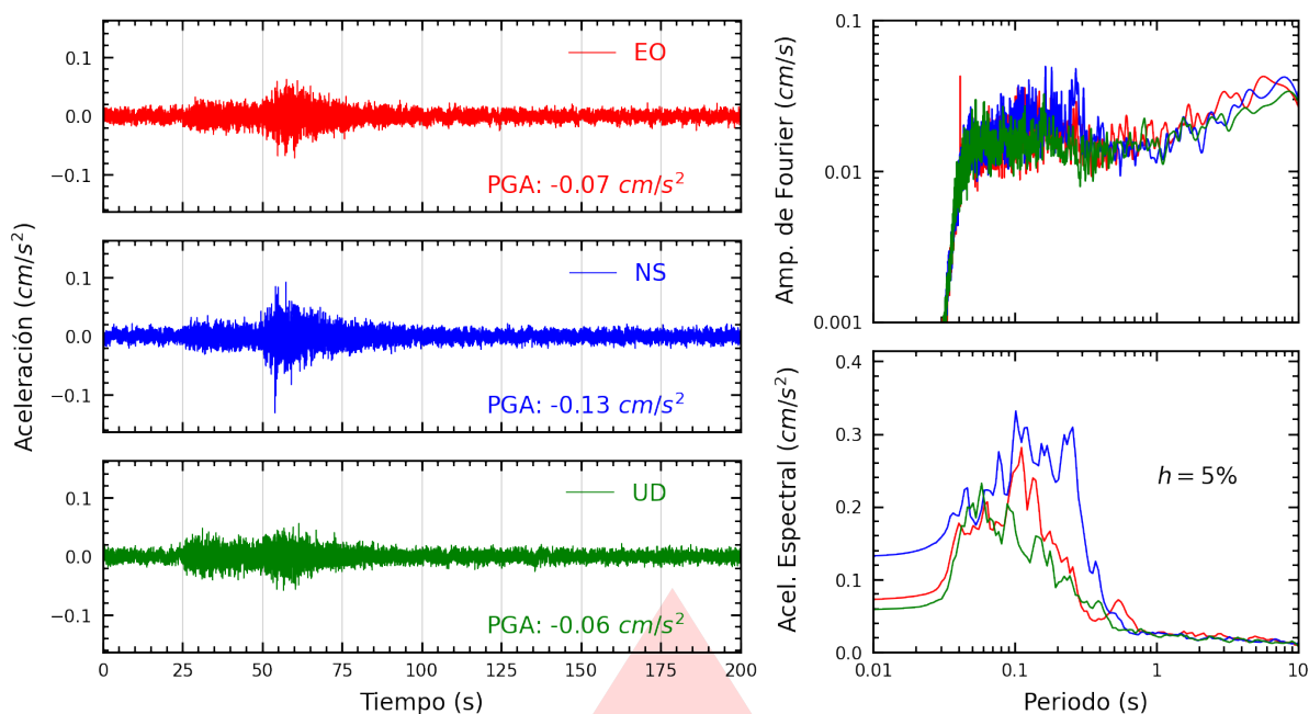
Figura A.15: Registros tiempo-historia, espectros de Fourier y de respuesta en las direcciones EO, NS y vertical de la estación SERVI. Sismo de Castrovirreyna, Castrovirreyna - Huancavelica del 2026-07-17, 04:16:31 (Hora local)
