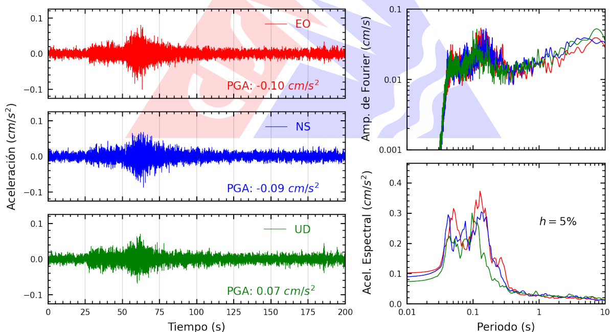
Figura A.20: Registros tiempo-historia, espectros de Fourier y de respuesta en las direcciones EO, NS y vertical de la estación JALVA. Sismo de Castrovirreyna, Castrovirreyna - Huancavelica del 2026-07-17, 04:16:31 (Hora local)
