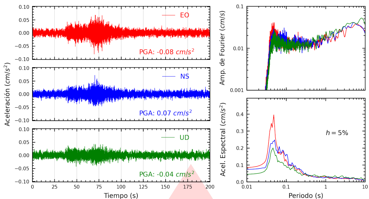
Figura A.23: Registros tiempo-historia, espectros de Fourier y de respuesta en las direcciones EO, NS y vertical de la estación UCSS. Sismo de Castrovirreyna, Castrovirreyna - Huancavelica del 2026-07-17, 04:16:31 (Hora local)
