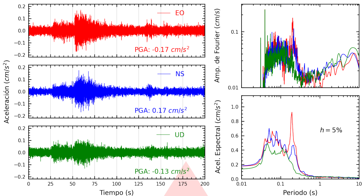
Figura A.11: Registros tiempo-historia, espectros de Fourier y de respuesta en las direcciones EO, NS y vertical de la estación INDEP. Sismo de Castrovirreyna, Castrovirreyna - Huancavelica del 2026-07-17, 04:16:31 (Hora local)
