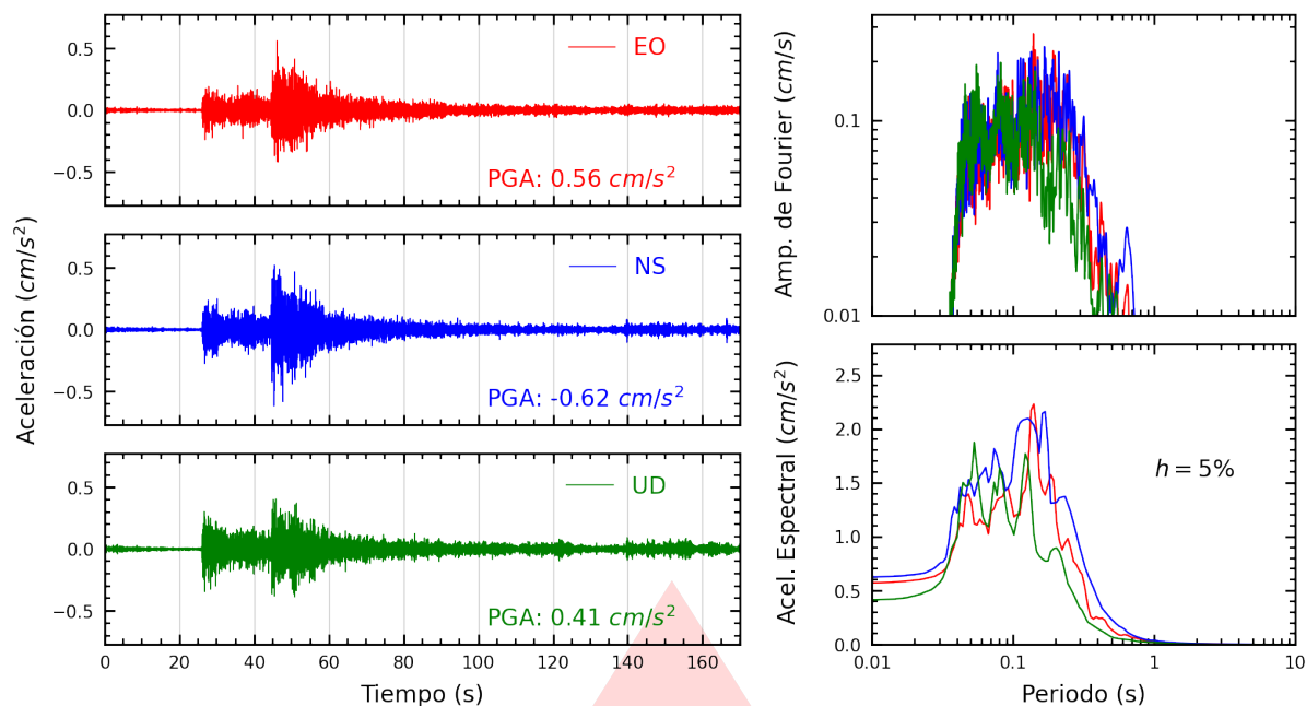
Figura A.1: Registros tiempo-historia, espectros de Fourier y de respuesta en las direcciones EO, NS y vertical de la estación ASIA. Sismo de Castrovirreyna, Castrovirreyna - Huancavelica del 2026-07-17, 04:16:31 (Hora local)
