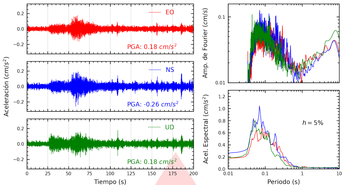
Figura A.7: Registros tiempo-historia, espectros de Fourier y de respuesta en las direcciones EO, NS y vertical de la estación SJLSC. Sismo de Castrovirreyna, Castrovirreyna - Huancavelica del 2026-07-17, 04:16:31 (Hora local)
