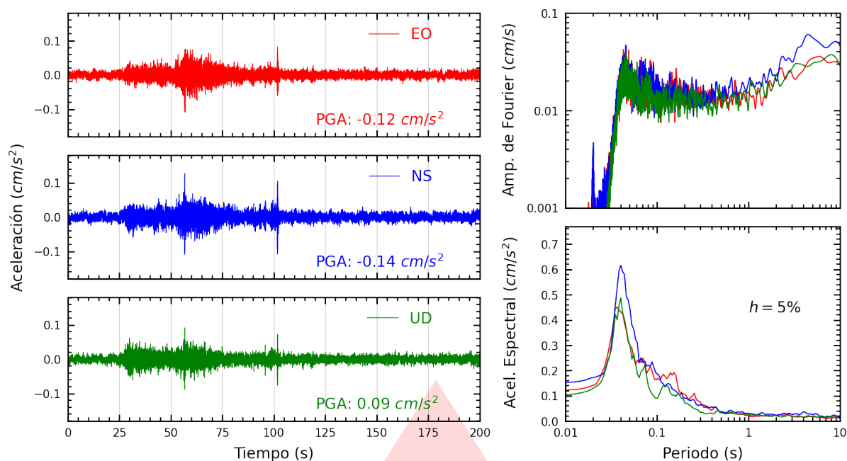
Figura A.13: Registros tiempo-historia, espectros de Fourier y de respuesta en las direcciones EO, NS y vertical de la estación SJLCE. Sismo de Castrovirreyna, Castrovirreyna - Huancavelica del 2026-07-17, 04:16:31 (Hora local)
