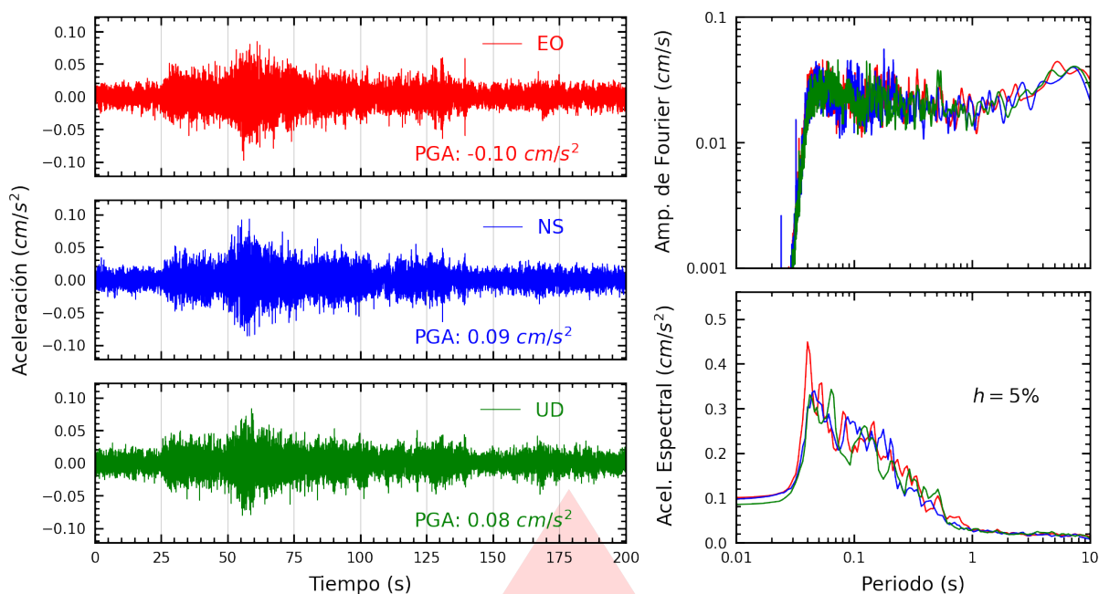
Figura A.21: Registros tiempo-historia, espectros de Fourier y de respuesta en las direcciones EO, NS y vertical de la estación IMCA. Sismo de Castrovirreyna, Castrovirreyna - Huancavelica del 2026-07-17, 04:16:31 (Hora local)
