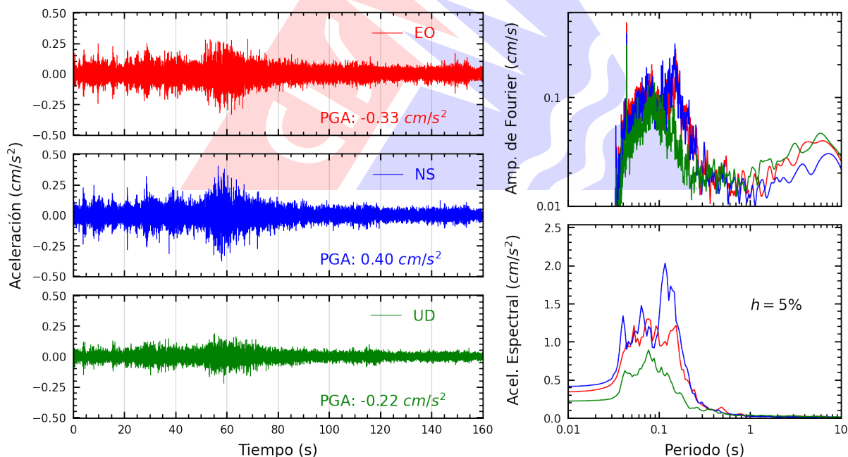
Figura A.2: Registros tiempo-historia, espectros de Fourier y de respuesta en las direcciones EO, NS y vertical de la estación USILM. Sismo de Castrovirreyna, Castrovirreyna - Huancavelica del 2026-07-17, 04:16:31 (Hora local)
