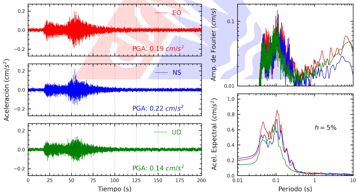
Figura A.8: Registros tiempo-historia, espectros de Fourier y de respuesta en las direcciones EO, NS y vertical de la estación AMORE. Sismo de Castrovirreyna, Castrovirreyna - Huancavelica del 2026-07-17, 04:16:31 (Hora local)
