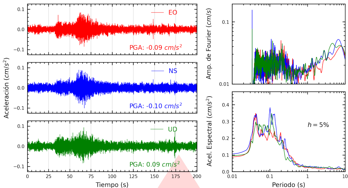
Figura A.19: Registros tiempo-historia, espectros de Fourier y de respuesta en las direcciones EO, NS y vertical de la estación USMP. Sismo de Castrovirreyna, Castrovirreyna - Huancavelica del 2026-07-17, 04:16:31 (Hora local)
