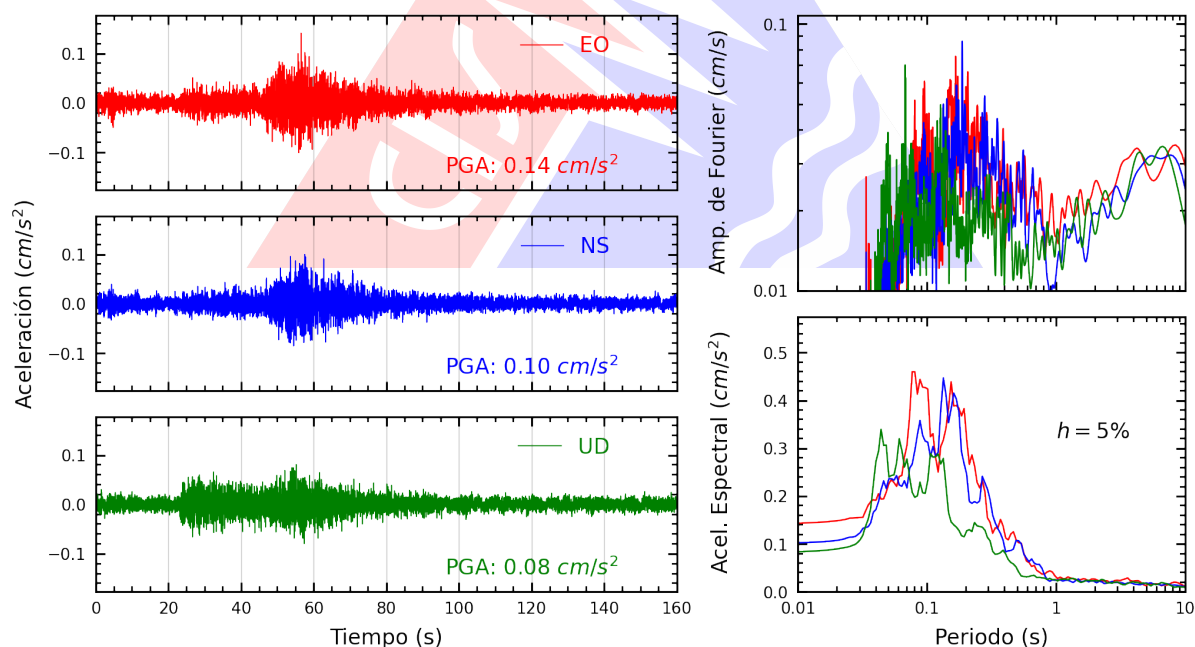
Figura A.14: Registros tiempo-historia, espectros de Fourier y de respuesta en las direcciones EO, NS y vertical de la estación USILP. Sismo de Castrovirreyna, Castrovirreyna - Huancavelica del 2026-07-17, 04:16:31 (Hora local)
