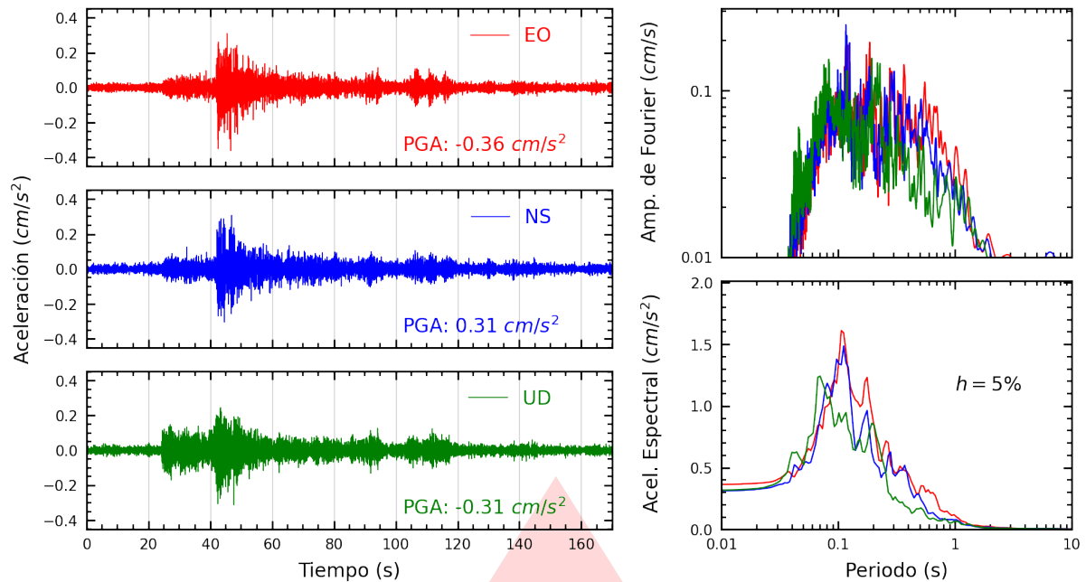
Figura A.3: Registros tiempo-historia, espectros de Fourier y de respuesta en las direcciones EO, NS y vertical de la estación UNICA. Sismo de Castrovirreyna, Castrovirreyna - Huancavelica del 2026-07-17, 04:16:31 (Hora local)
