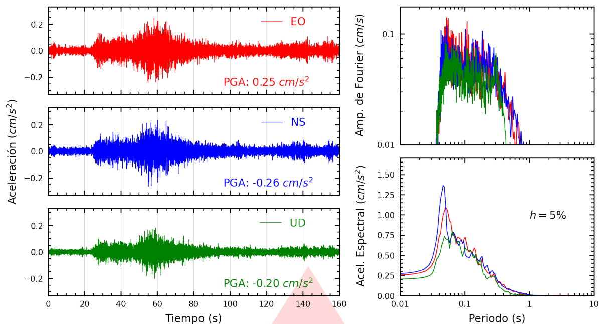
Figura A.5: Registros tiempo-historia, espectros de Fourier y de respuesta en las direcciones EO, NS y vertical de la estación UNTEL. Sismo de Castrovirreyna, Castrovirreyna - Huancavelica del 2026-07-17, 04:16:31 (Hora local)
