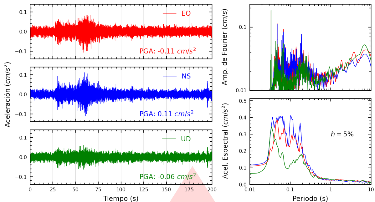
Figura A.17: Registros tiempo-historia, espectros de Fourier y de respuesta en las direcciones EO, NS y vertical de la estación UPCVI. Sismo de Castrovirreyna, Castrovirreyna - Huancavelica del 2026-07-17, 04:16:31 (Hora local)
