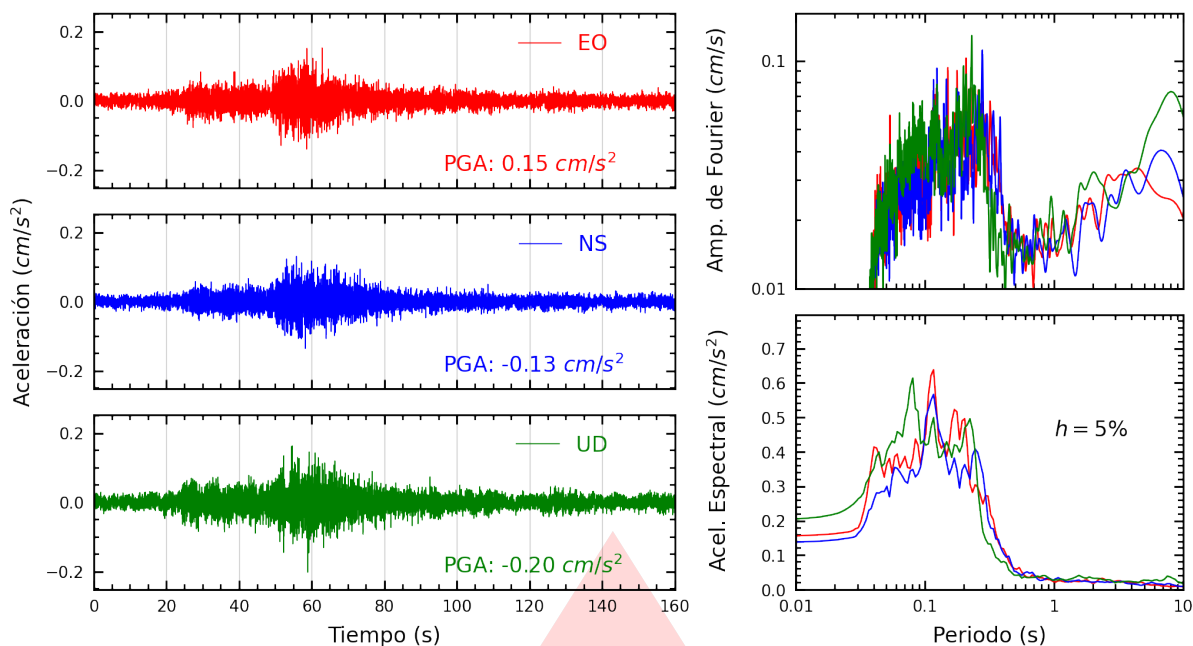
Figura A.9: Registros tiempo-historia, espectros de Fourier y de respuesta en las direcciones EO, NS y vertical de la estación SOVES. Sismo de Castrovirreyna, Castrovirreyna - Huancavelica del 2026-07-17, 04:16:31 (Hora local)
