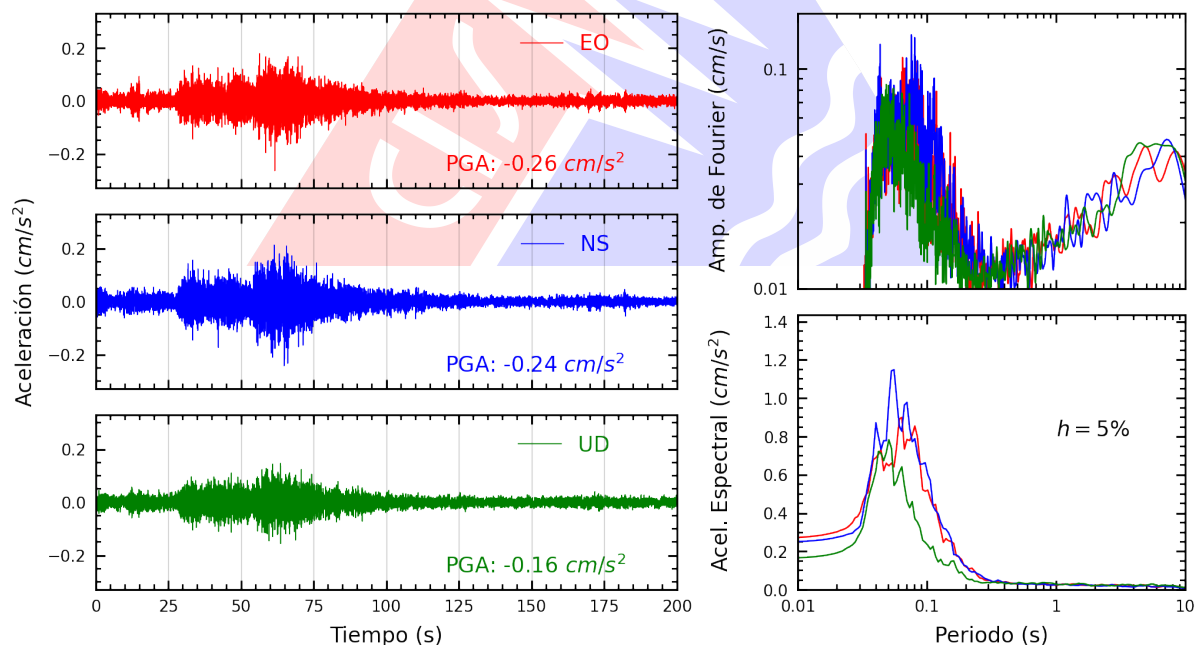
Figura A.6: Registros tiempo-historia, espectros de Fourier y de respuesta en las direcciones EO, NS y vertical de la estación JOSEO. Sismo de Castrovirreyna, Castrovirreyna - Huancavelica del 2026-07-17, 04:16:31 (Hora local)
