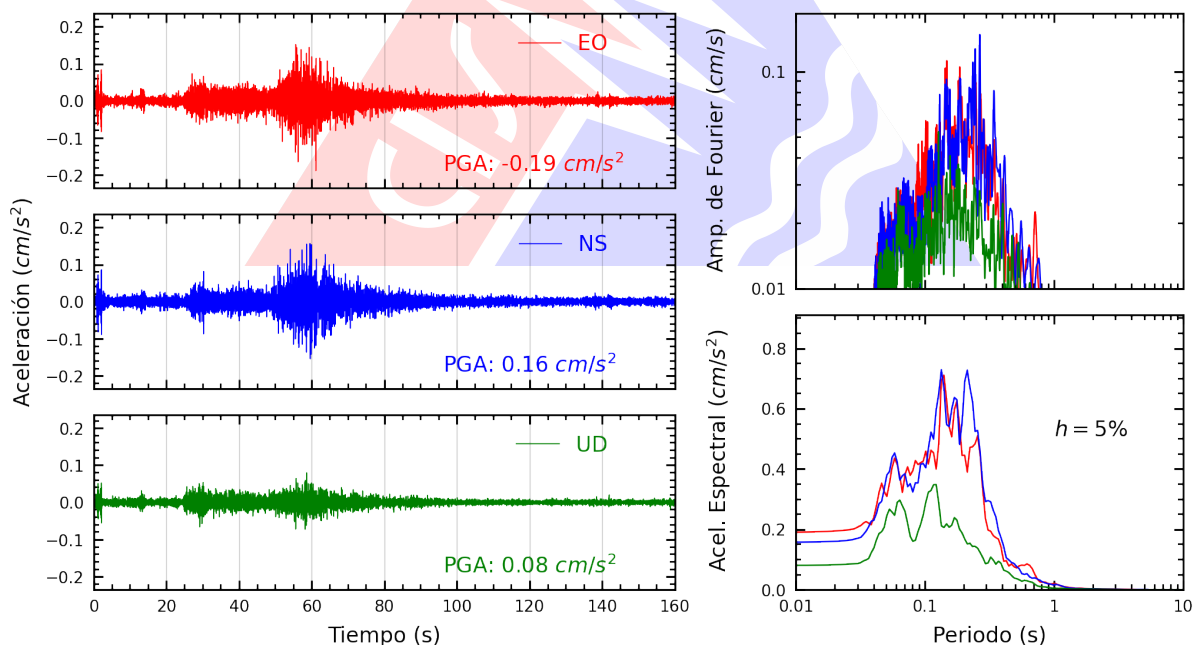
Figura A.10: Registros tiempo-historia, espectros de Fourier y de respuesta en las direcciones EO, NS y vertical de la estación BRIS2. Sismo de Castrovirreyna, Castrovirreyna - Huancavelica del 2026-07-17, 04:16:31 (Hora local)
