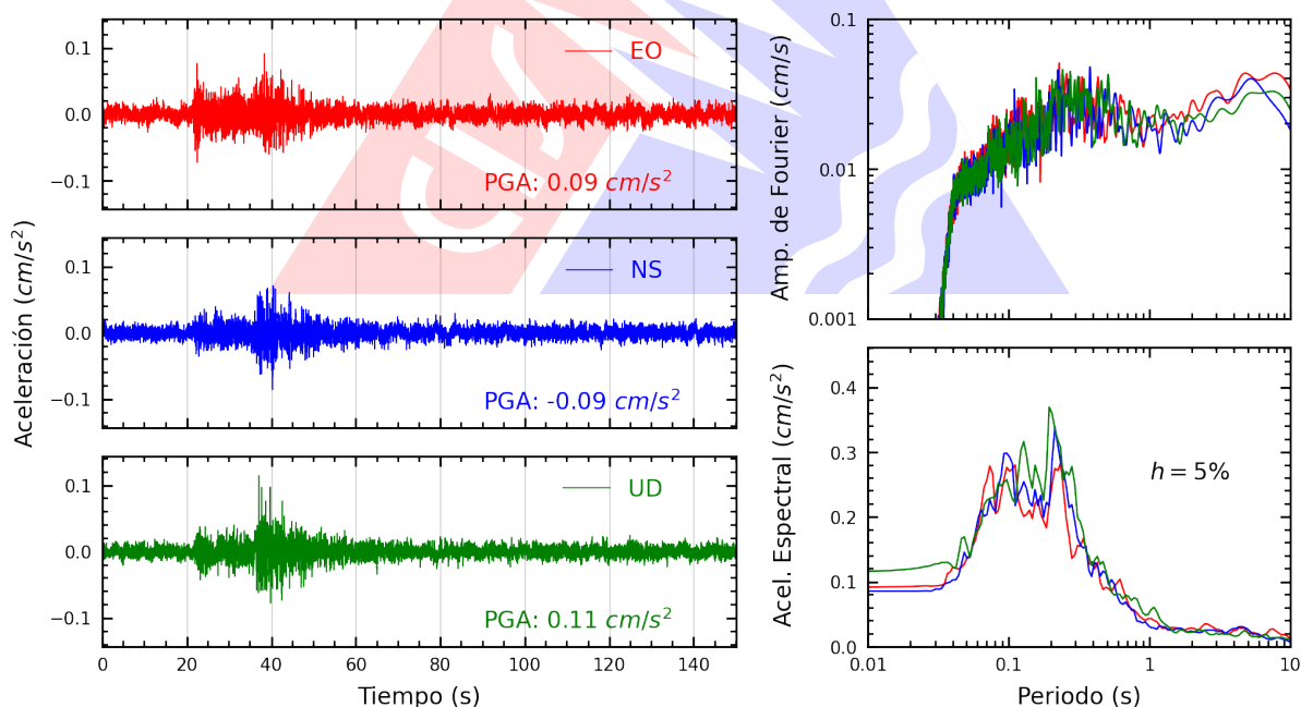
Figura A.16: Registros tiempo-historia, espectros de Fourier y de respuesta en las direcciones EO, NS y vertical de la estación UNSCH. Sismo de Castrovirreyna, Castrovirreyna - Huancavelica del 2026-07-17, 04:16:31 (Hora local)
