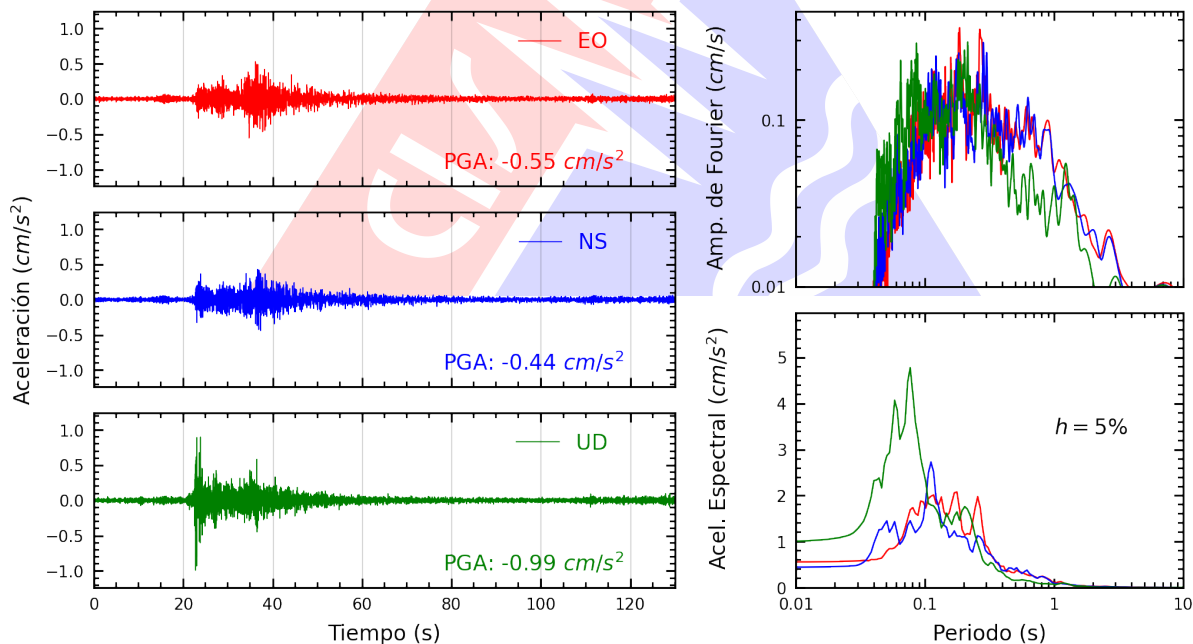
Figura A.2: Registros tiempo-historia, espectros de Fourier y de respuesta en las direcciones EO, NS y vertical de la estación UNICA. Sismo de Ica, Ica - Ica del 2026-07-17, 17:26:25 (Hora local)
