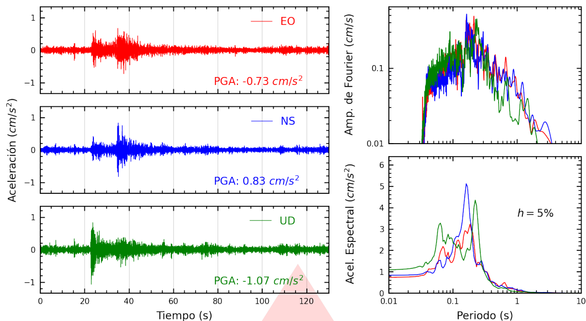
Figura A.1: Registros tiempo-historia, espectros de Fourier y de respuesta en las direcciones EO, NS y vertical de la estación SCICA. Sismo de Ica, Ica - Ica del 2026-07-17, 17:26:25 (Hora local)
