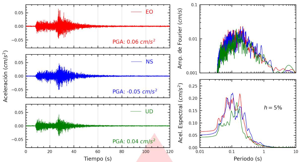
Figura A.1: Registros tiempo-historia, espectros de Fourier y de respuesta en las direcciones EO, NS y vertical de la estación UNSA2. Sismo de Huambo, Caylloma - Arequipa del 2026-07-17, 21:58:55 (Hora local)
