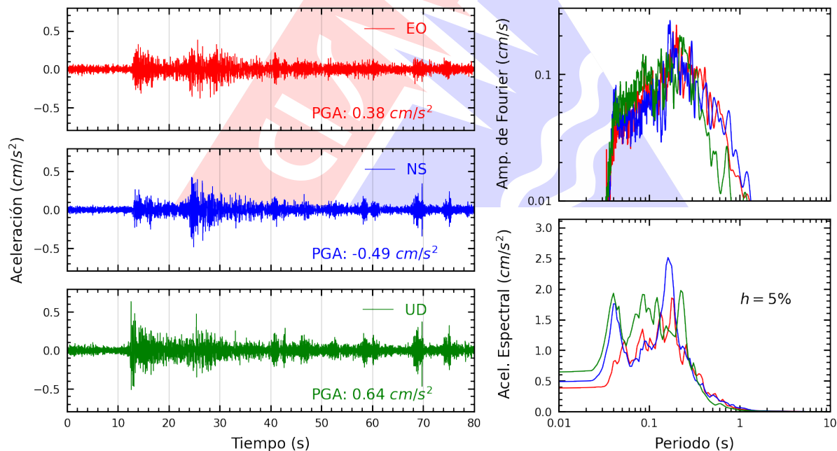
Figura A.2: Registros tiempo-historia, espectros de Fourier y de respuesta en las direcciones EO, NS y vertical de la estación SCICA. Sismo de Ica, Ica - Ica del 2026-07-17, 23:36:54 (Hora local)
