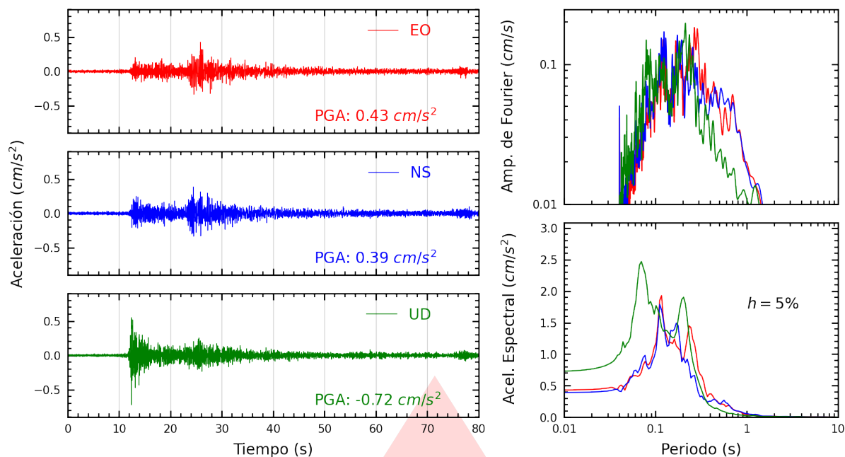
Figura A.1: Registros tiempo-historia, espectros de Fourier y de respuesta en las direcciones EO, NS y vertical de la estación UNICA. Sismo de Ica, Ica - Ica del 2026-07-17, 23:36:54 (Hora local)
