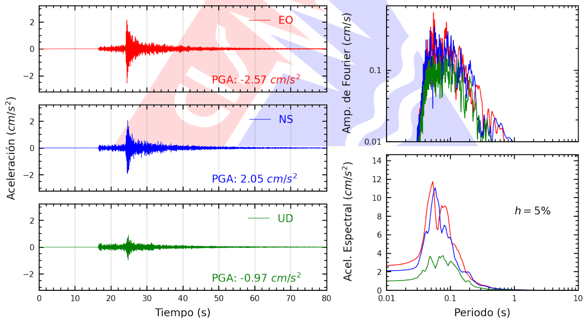
Figura A.2: Registros tiempo-historia, espectros de Fourier y de respuesta en las direcciones EO, NS y vertical de la estación UNSA2. Sismo de Bombón, Islay - Arequipa del 2026-07-18, 09:40:54 (Hora local)
