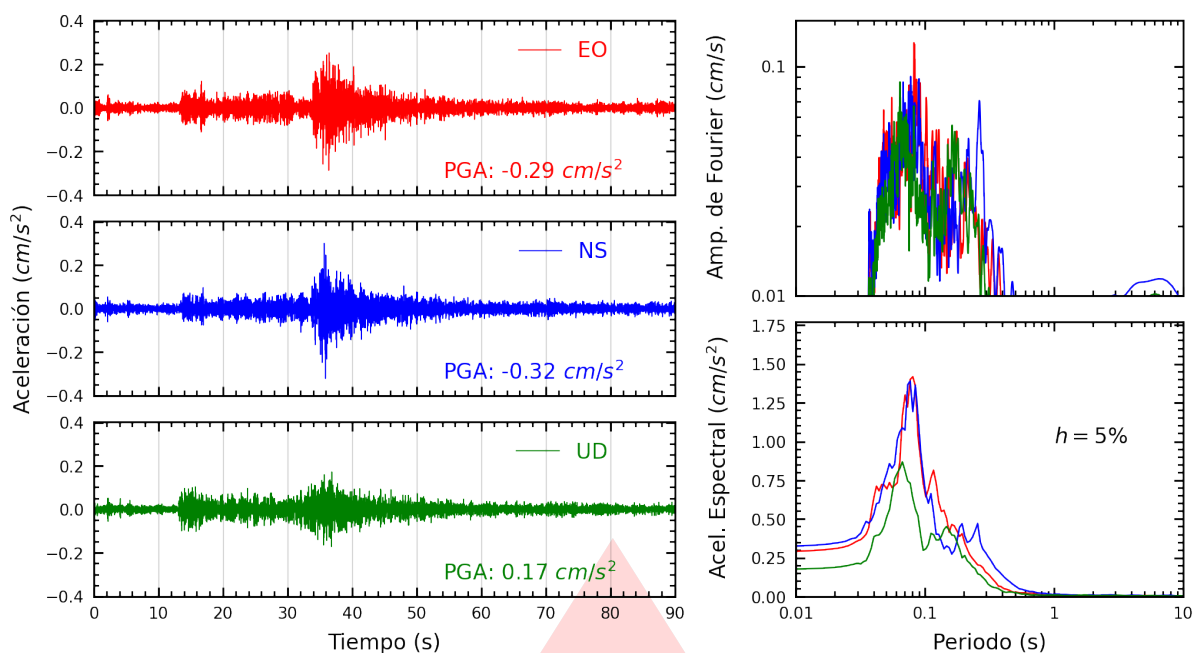
Figura A.3: Registros tiempo-historia, espectros de Fourier y de respuesta en las direcciones EO, NS y vertical de la estación CREY. Sismo de Bombón, Islay - Arequipa del 2026-07-18, 09:40:54 (Hora local)
