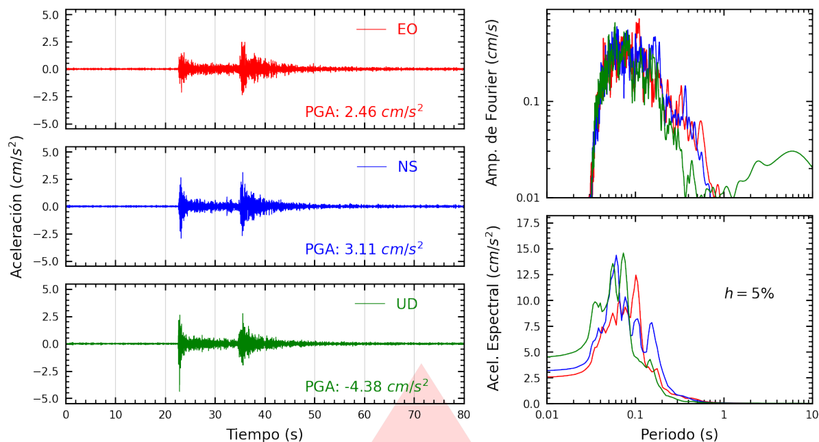
Figura A.1: Registros tiempo-historia, espectros de Fourier y de respuesta en las direcciones EO, NS y vertical de la estación SCARQ. Sismo de Bombón, Islay - Arequipa del 2026-07-18, 09:40:54 (Hora local)
