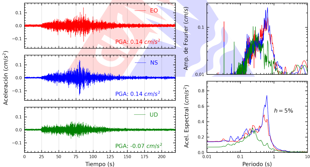
Figura A.4: Registros tiempo-historia, espectros de Fourier y de respuesta en las direcciones EO, NS y vertical de la estación CARAL. Sismo de Chimbote, Santa - Áncash del 2026-07-21, 12:42:55 (Hora local)
