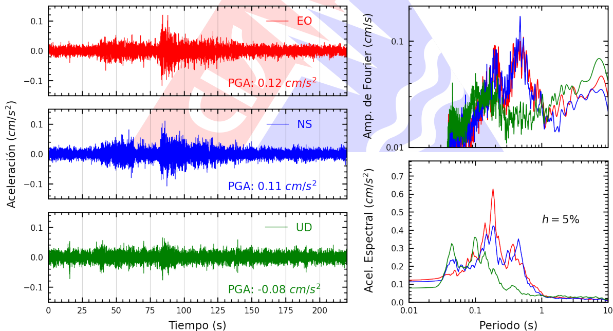
Figura A.6: Registros tiempo-historia, espectros de Fourier y de respuesta en las direcciones EO, NS y vertical de la estación VHAYA. Sismo de Chimbote, Santa - Áncash del 2026-07-21, 12:42:55 (Hora local)
