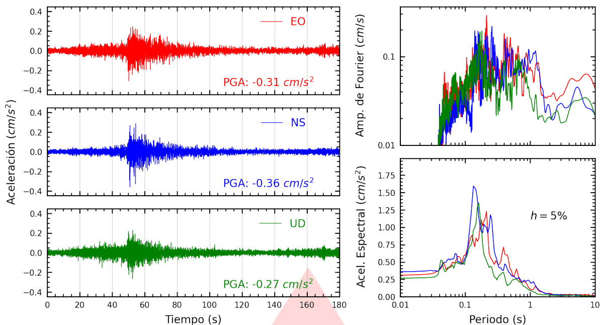
Figura A.1: Registros tiempo-historia, espectros de Fourier y de respuesta en las direcciones EO, NS y vertical de la estación UPAOT. Sismo de Chimbote, Santa - Áncash del 2026-07-21, 12:42:55 (Hora local)
