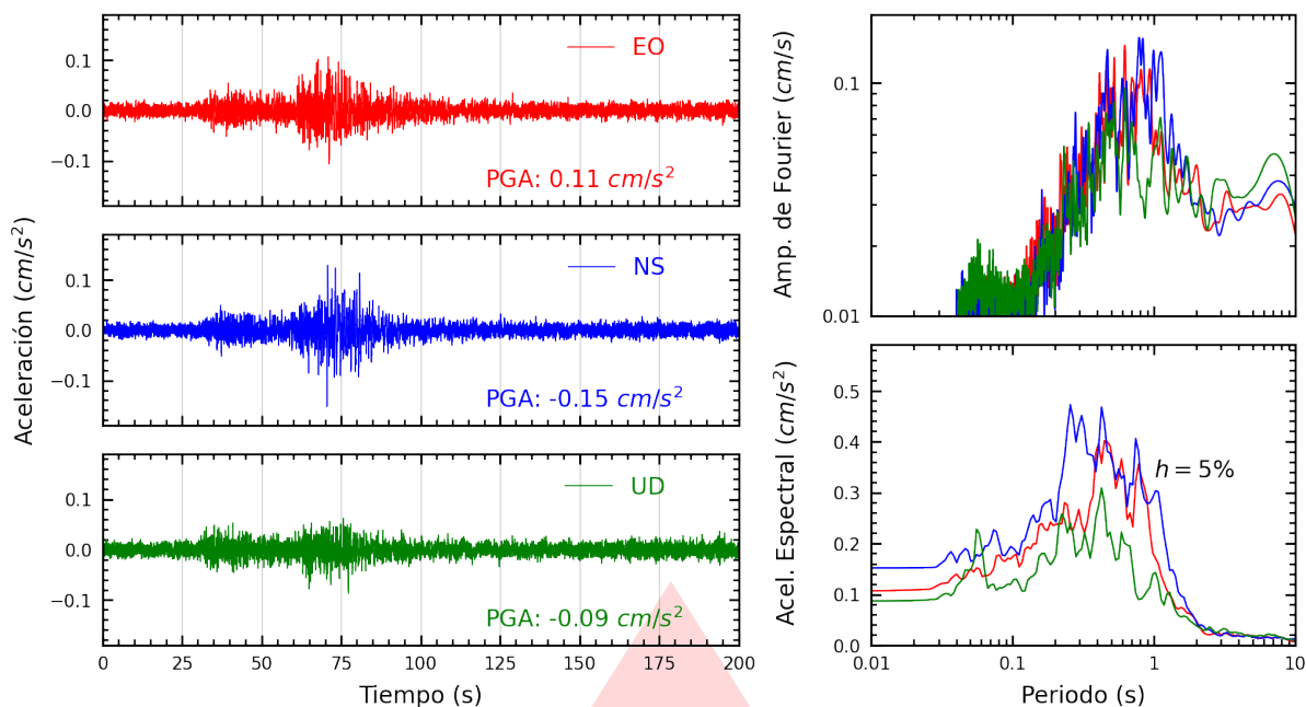
Figura A.3: Registros tiempo-historia, espectros de Fourier y de respuesta en las direcciones EO, NS y vertical de la estación UNASA. Sismo de Chimbote, Santa - Áncash del 2026-07-21, 12:42:55 (Hora local)
