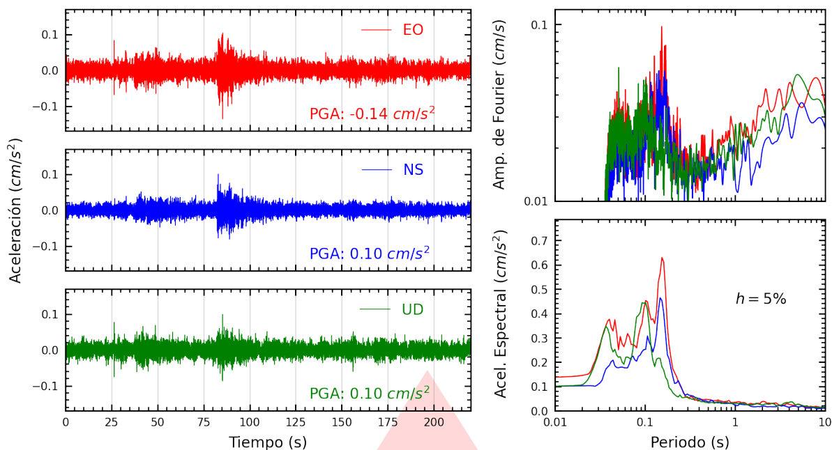
Figura A.5: Registros tiempo-historia, espectros de Fourier y de respuesta en las direcciones EO, NS y vertical de la estación AMORE. Sismo de Chimbote, Santa - Áncash del 2026-07-21, 12:42:55 (Hora local)
