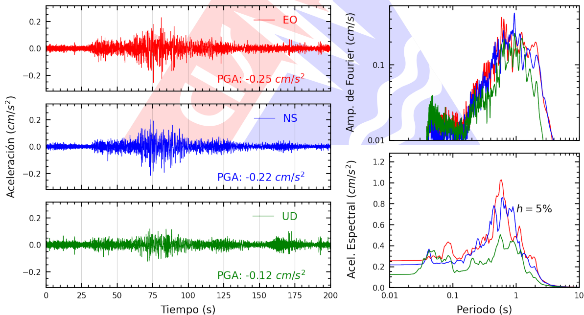
Figura A.2: Registros tiempo-historia, espectros de Fourier y de respuesta en las direcciones EO, NS y vertical de la estación UNC. Sismo de Chimbote, Santa - Áncash del 2026-07-21, 12:42:55 (Hora local)
