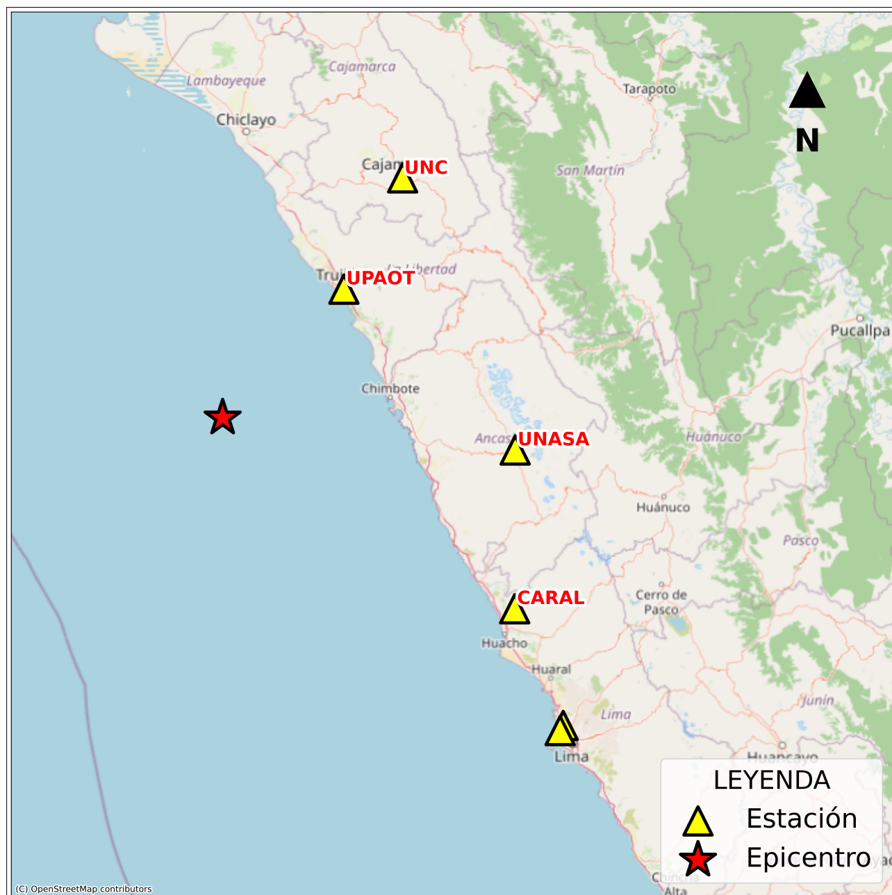
Figura 2: Mapa de ubicación de la(s) estación(es) acelerográfica(s) a nivel nacional correspondiente(s) al Sismo de Chimbote, Santa - Áncash del 21 de julio de 2026 a las 12:42:55 (hora local)
