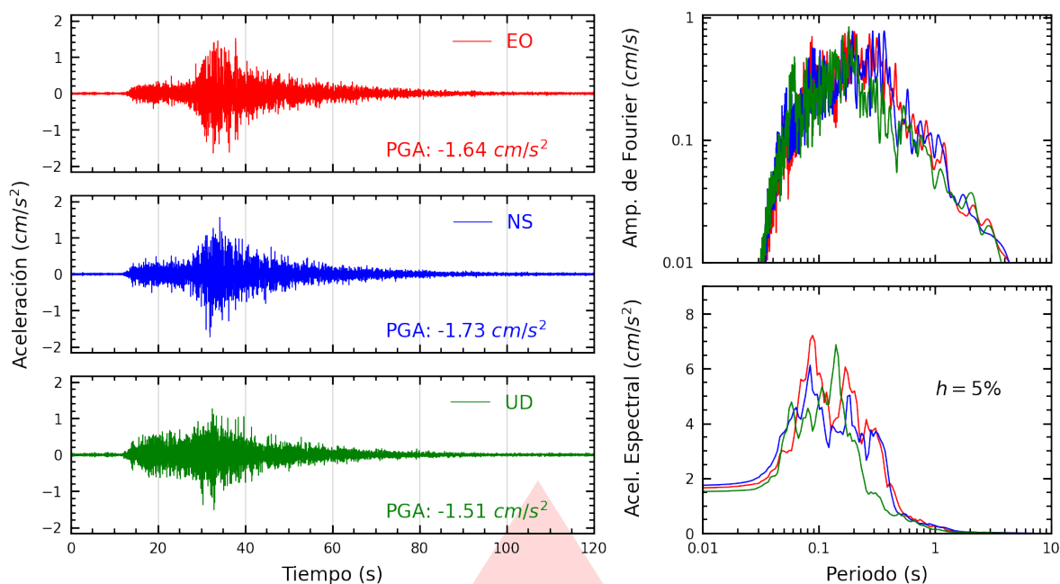
Figura A.3: Registros tiempo-historia, espectros de Fourier y de respuesta en las direcciones EO, NS y vertical de la estación UJBG2. Sismo de Tacna, Tacna - Tacna del 2026-07-21, 21:03:49 (Hora local)
