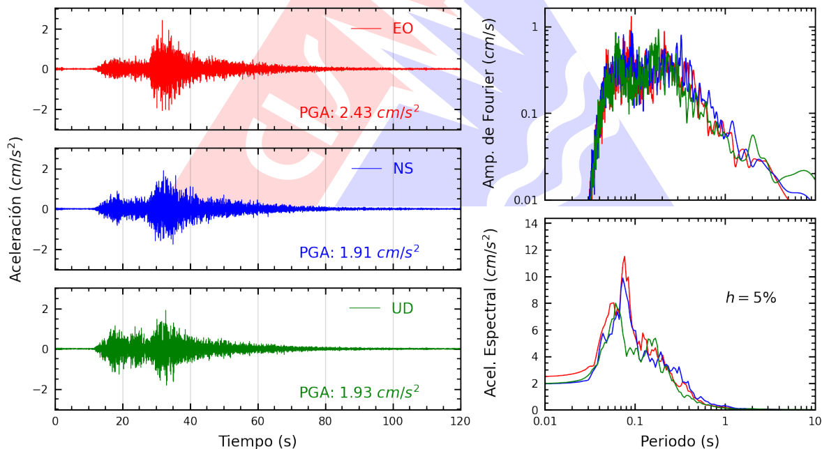
Figura A.2: Registros tiempo-historia, espectros de Fourier y de respuesta en las direcciones EO, NS y vertical de la estación CREY. Sismo de Tacna, Tacna - Tacna del 2026-07-21, 21:03:49 (Hora local)
