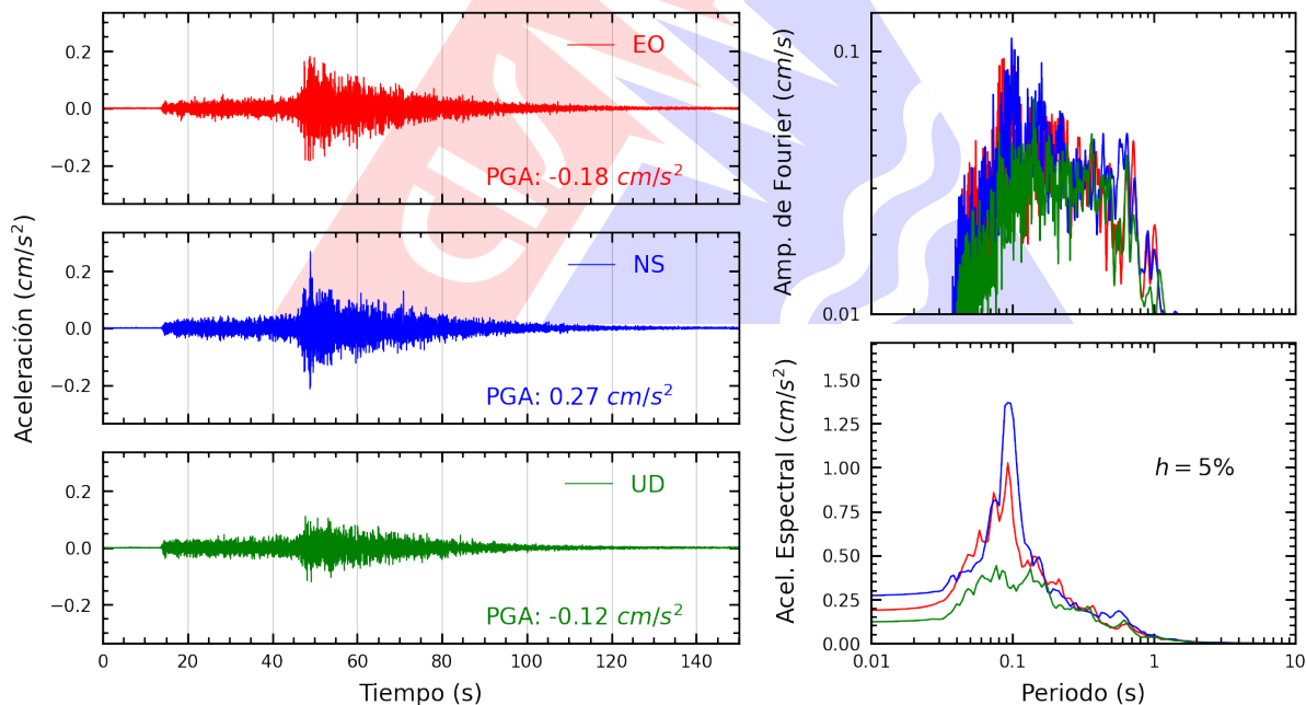
Figura A.4: Registros tiempo-historia, espectros de Fourier y de respuesta en las direcciones EO, NS y vertical de la estación UNSA2. Sismo de Tacna, Tacna - Tacna del 2026-07-21, 21:03:49 (Hora local)
