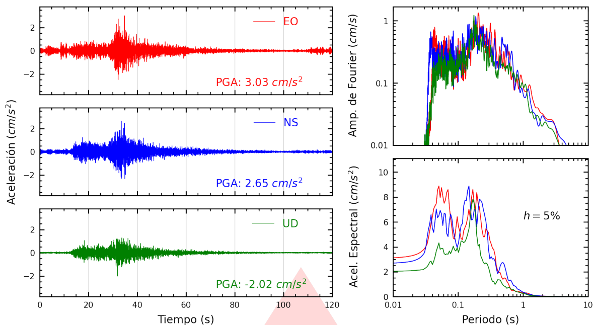
Figura A.1: Registros tiempo-historia, espectros de Fourier y de respuesta en las direcciones EO, NS y vertical de la estación UPTAC. Sismo de Tacna, Tacna - Tacna del 2026-07-21, 21:03:49 (Hora local)
