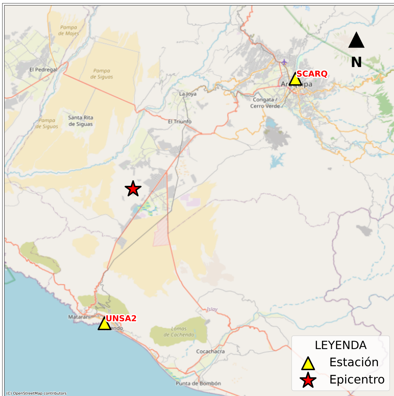
Figura 2: Mapa de ubicación de la(s) estación(es) acelerográfica(s) correspondiente(s) al Sismo de Vitor, Arequipa - Arequipa del 23 de julio de 2026 a las 23:48:06 (hora local)
