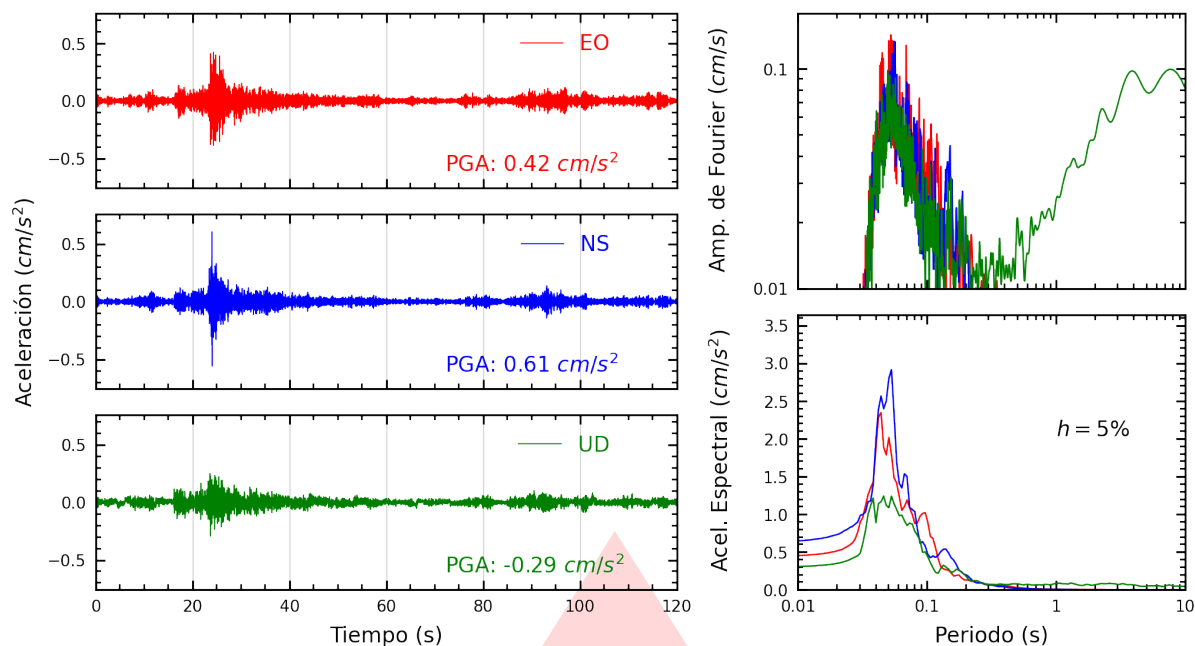
Figura A.1: Registros tiempo-historia, espectros de Fourier y de respuesta en las direcciones EO, NS y vertical de la estación SCARQ. Sismo de Vitor, Arequipa - Arequipa del 2026-07-23, 23:48:06 (Hora local)
