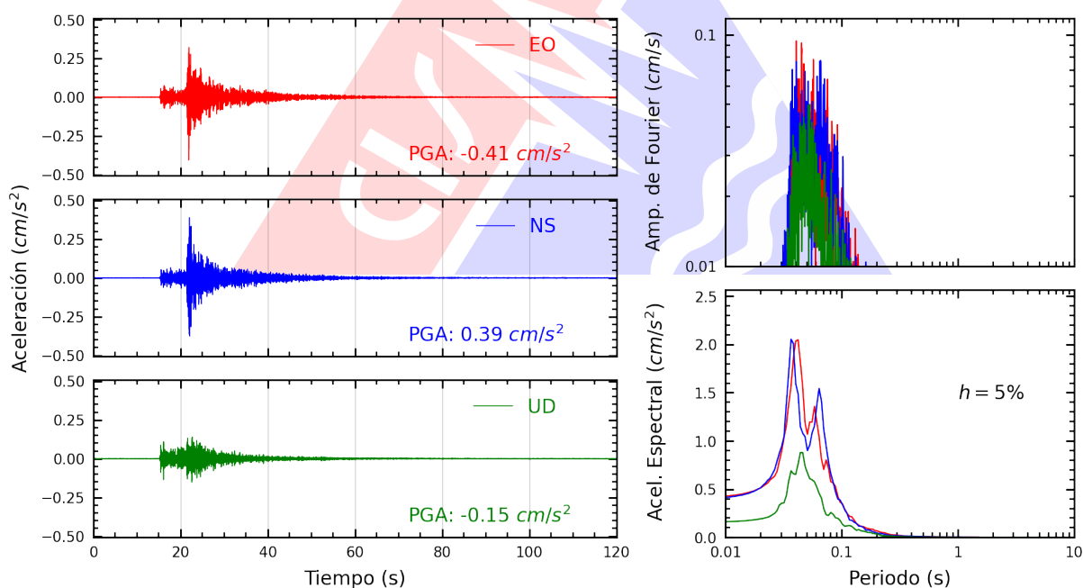
Figura A.2: Registros tiempo-historia, espectros de Fourier y de respuesta en las direcciones EO, NS y vertical de la estación UNSA2. Sismo de Vitor, Arequipa - Arequipa del 2026-07-23, 23:48:06 (Hora local)
