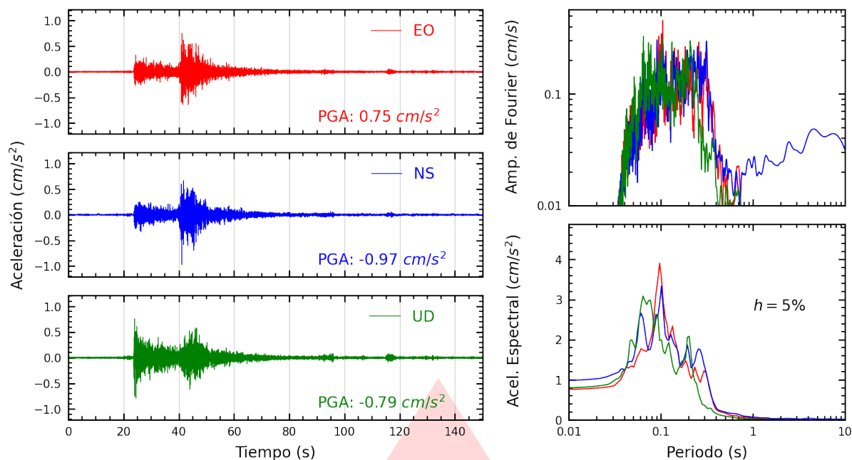
Figura A.1: Registros tiempo-historia, espectros de Fourier y de respuesta en las direcciones EO, NS y vertical de la estación SCTAC. Sismo de Tarata, Tarata - Tacna del 2026-07-24, 02:41:40 (Hora local)
