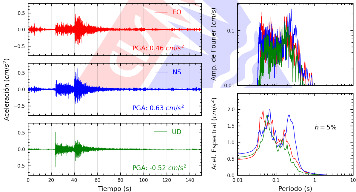
Figura A.4: Registros tiempo-historia, espectros de Fourier y de respuesta en las direcciones EO, NS y vertical de la estación UPTAC. Sismo de Tarata, Tarata - Tacna del 2026-07-24, 02:41:40 (Hora local)
