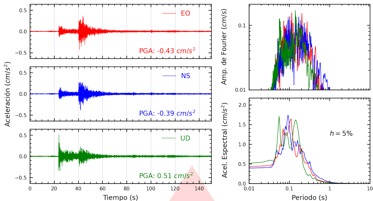
Figura A.5: Registros tiempo-historia, espectros de Fourier y de respuesta en las direcciones EO, NS y vertical de la estación UJBG2. Sismo de Tarata, Tarata - Tacna del 2026-07-24, 02:41:40 (Hora local)
