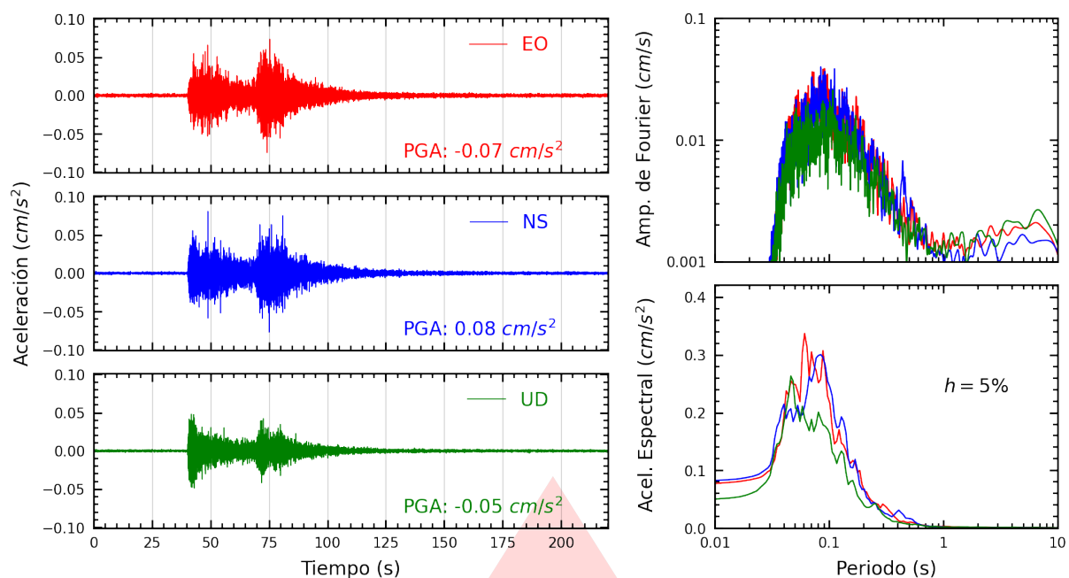
Figura A.7: Registros tiempo-historia, espectros de Fourier y de respuesta en las direcciones EO, NS y vertical de la estación UNSA2. Sismo de Tarata, Tarata - Tacna del 2026-07-24, 02:41:40 (Hora local)
