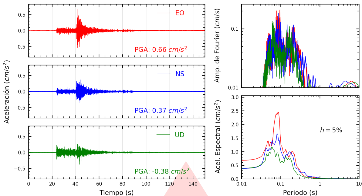
Figura A.3: Registros tiempo-historia, espectros de Fourier y de respuesta en las direcciones EO, NS y vertical de la estación CREY. Sismo de Tarata, Tarata - Tacna del 2026-07-24, 02:41:40 (Hora local)
