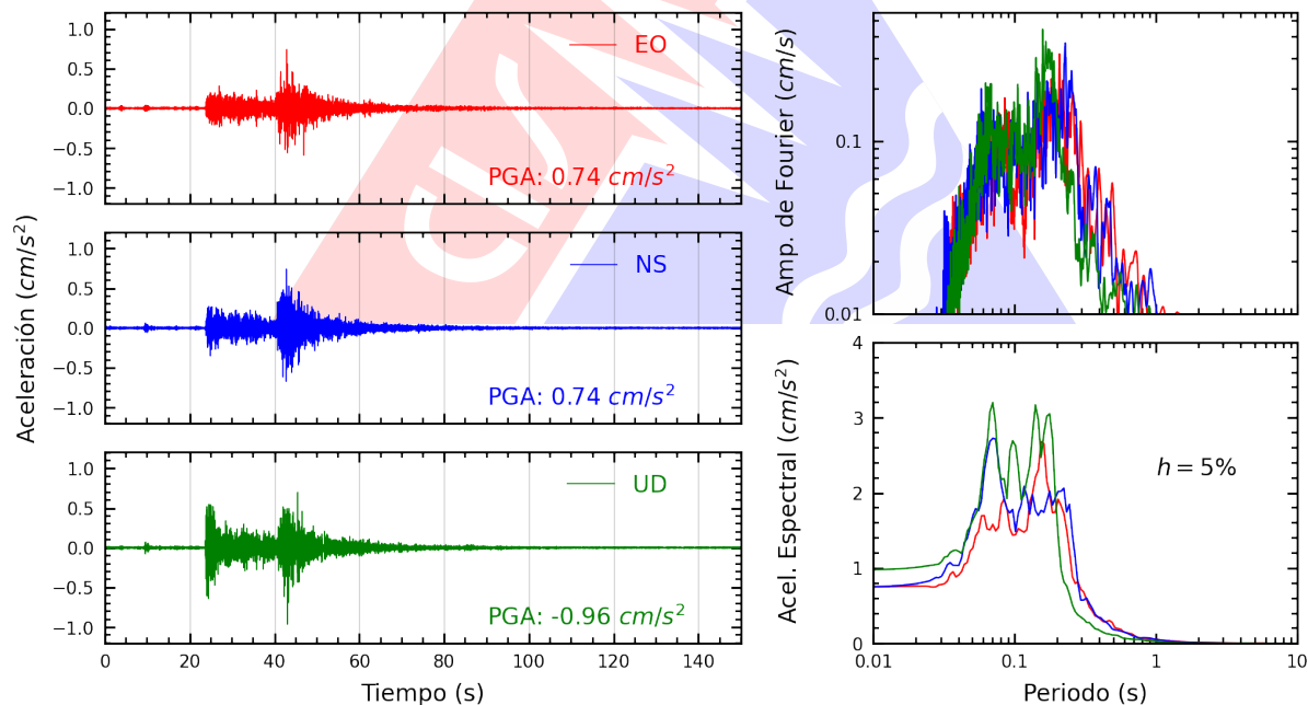
Figura A.2: Registros tiempo-historia, espectros de Fourier y de respuesta en las direcciones EO, NS y vertical de la estación UJB4. Sismo de Tarata, Tarata - Tacna del 2026-07-24, 02:41:40 (Hora local)
