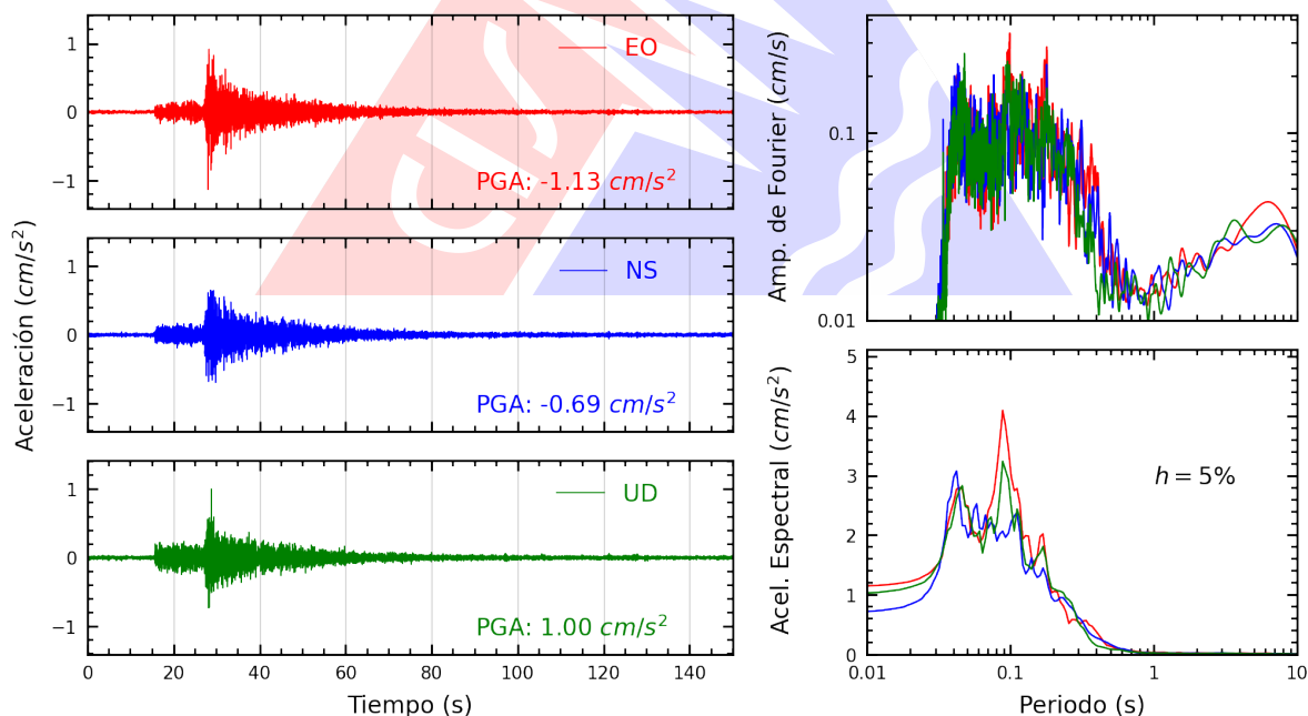
Figura A.20: Registros tiempo-historia, espectros de Fourier y de respuesta en las direcciones EO, NS y vertical de la estación USMP. Sismo de Huacho, Huaura - Lima del 2026-07-24, 21:48:11 (Hora local)
