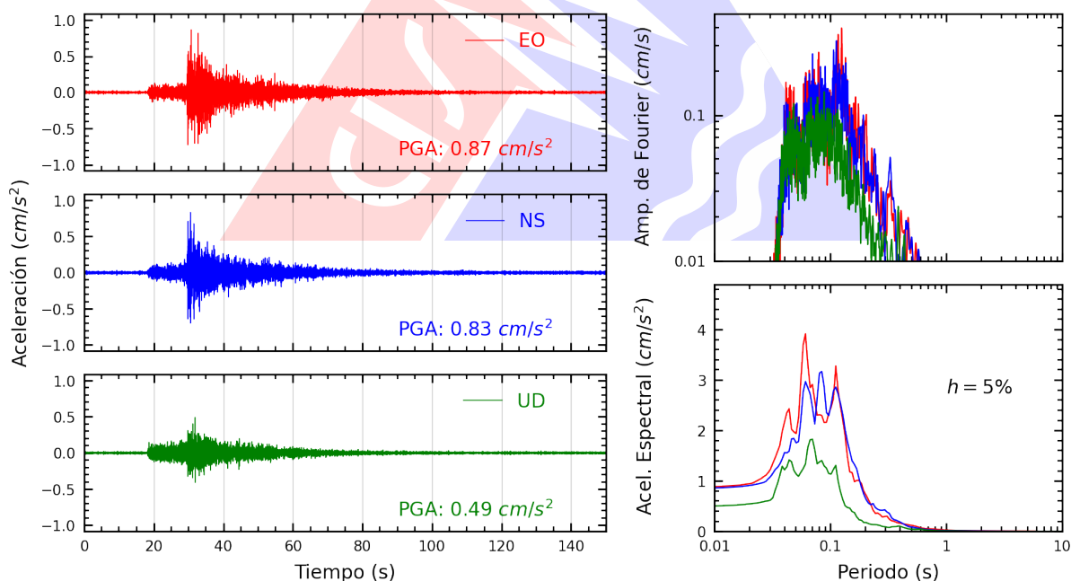
Figura A.30: Registros tiempo-historia, espectros de Fourier y de respuesta en las direcciones EO, NS y vertical de la estación ATARJ. Sismo de Huacho, Huaura - Lima del 2026-07-24, 21:48:11 (Hora local)
