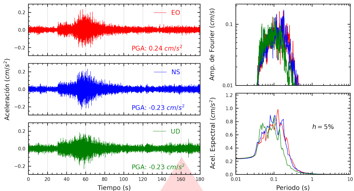
Figura A.41: Registros tiempo-historia, espectros de Fourier y de respuesta en las direcciones EO, NS y vertical de la estación ASIA. Sismo de Huacho, Huaura - Lima del 2026-07-24, 21:48:11 (Hora local)
