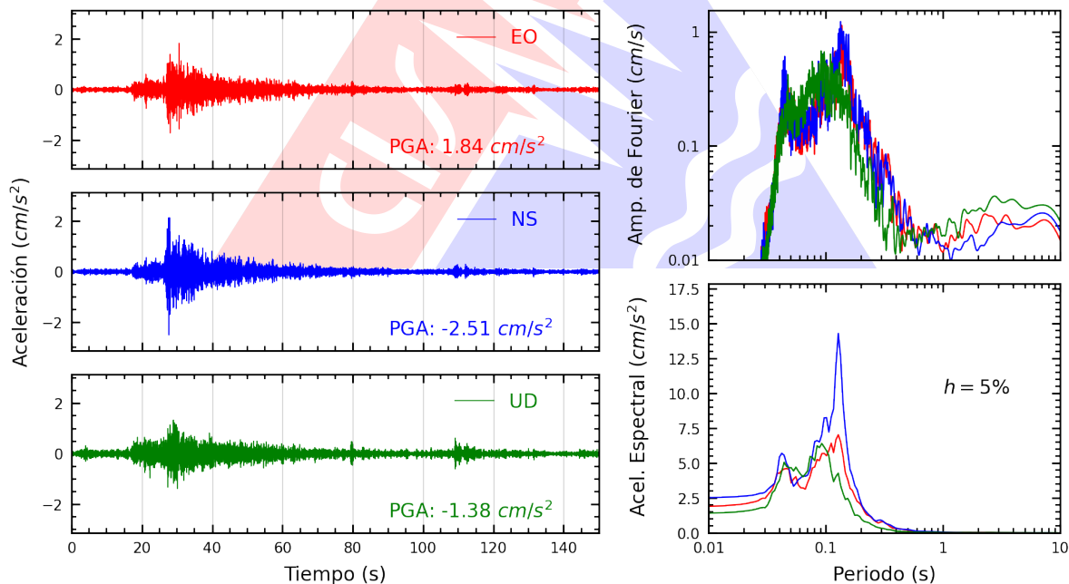
Figura A.8: Registros tiempo-historia, espectros de Fourier y de respuesta en las direcciones EO, NS y vertical de la estación CARAB. Sismo de Huacho, Huaura - Lima del 2026-07-24, 21:48:11 (Hora local)
