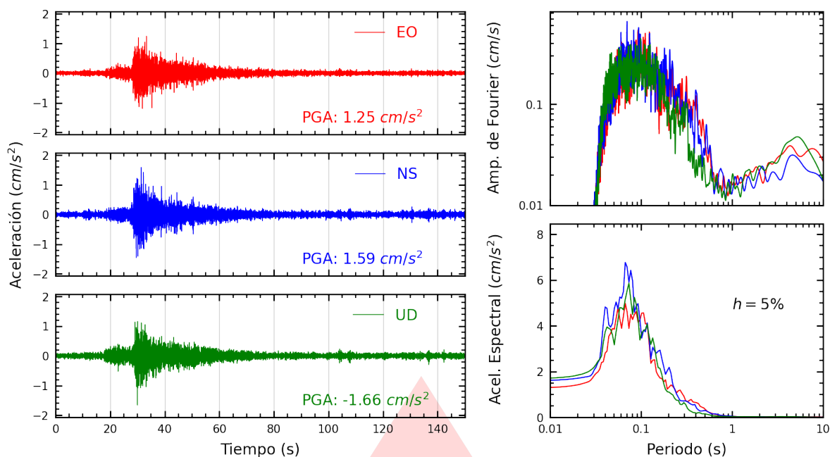
Figura A.15: Registros tiempo-historia, espectros de Fourier y de respuesta en las direcciones EO, NS y vertical de la estación SJLSC. Sismo de Huacho, Huaura - Lima del 2026-07-24, 21:48:11 (Hora local)
