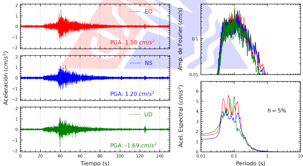
Figura A.14: Registros tiempo-historia, espectros de Fourier y de respuesta en las direcciones EO, NS y vertical de la estación PHERM. Sismo de Huacho, Huaura - Lima del 2026-07-24, 21:48:11 (Hora local)
