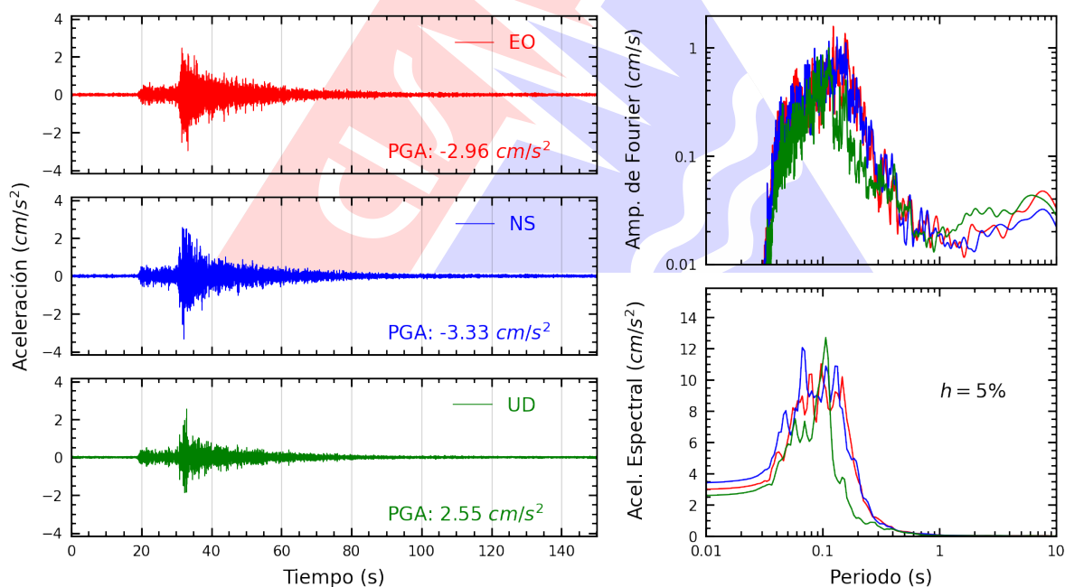
Figura A.4: Registros tiempo-historia, espectros de Fourier y de respuesta en las direcciones EO, NS y vertical de la estación USILM. Sismo de Huacho, Huaura - Lima del 2026-07-24, 21:48:11 (Hora local)
