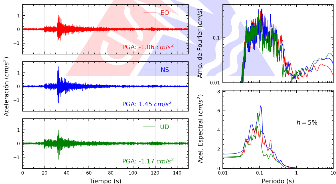
Figura A.18: Registros tiempo-historia, espectros de Fourier y de respuesta en las direcciones EO, NS y vertical de la estación URPE. Sismo de Huacho, Huaura - Lima del 2026-07-24, 21:48:11 (Hora local)
