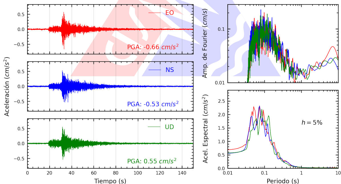
Figura A.36: Registros tiempo-historia, espectros de Fourier y de respuesta en las direcciones EO, NS y vertical de la estación SERVI. Sismo de Huacho, Huaura - Lima del 2026-07-24, 21:48:11 (Hora local)
