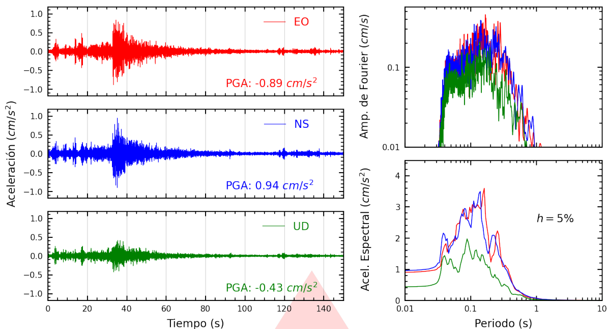
Figura A.27: Registros tiempo-historia, espectros de Fourier y de respuesta en las direcciones EO, NS y vertical de la estación BRISA. Sismo de Huacho, Huaura - Lima del 2026-07-24, 21:48:11 (Hora local)
