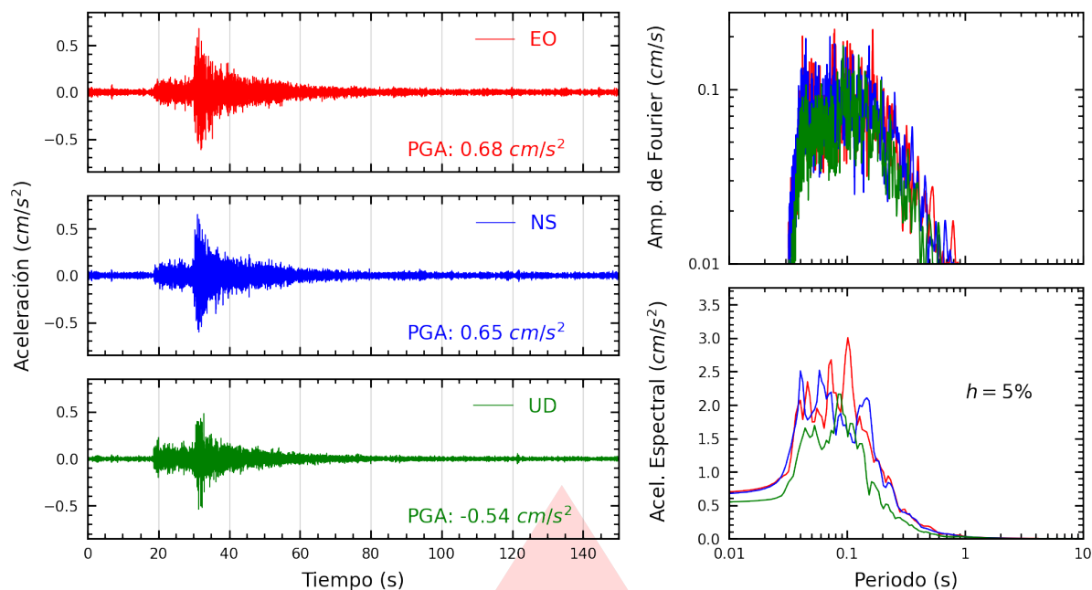
Figura A.33: Registros tiempo-historia, espectros de Fourier y de respuesta en las direcciones EO, NS y vertical de la estación BORJA. Sismo de Huacho, Huaura - Lima del 2026-07-24, 21:48:11 (Hora local)
