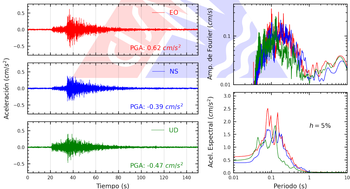
Figura A.38: Registros tiempo-historia, espectros de Fourier y de respuesta en las direcciones EO, NS y vertical de la estación USILP. Sismo de Huacho, Huaura - Lima del 2026-07-24, 21:48:11 (Hora local)
