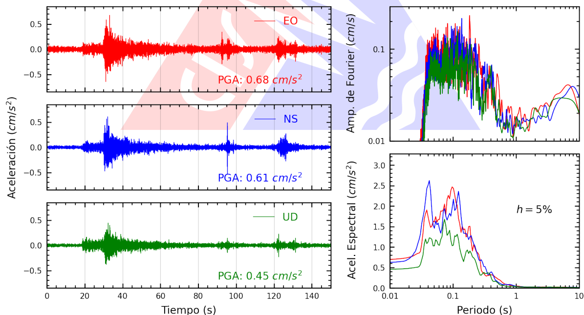
Figura A.34: Registros tiempo-historia, espectros de Fourier y de respuesta en las direcciones EO, NS y vertical de la estación INICT. Sismo de Huacho, Huaura - Lima del 2026-07-24, 21:48:11 (Hora local)
