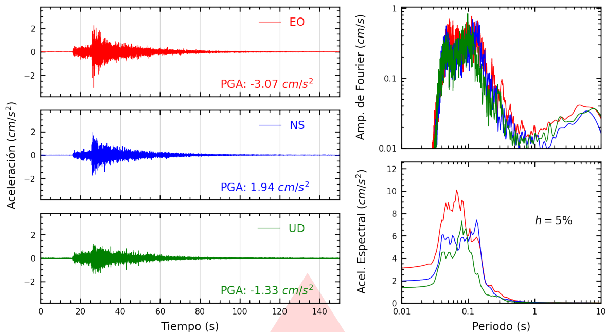
Figura A.5: Registros tiempo-historia, espectros de Fourier y de respuesta en las direcciones EO, NS y vertical de la estación AMORE. Sismo de Huacho, Huaura - Lima del 2026-07-24, 21:48:11 (Hora local)
