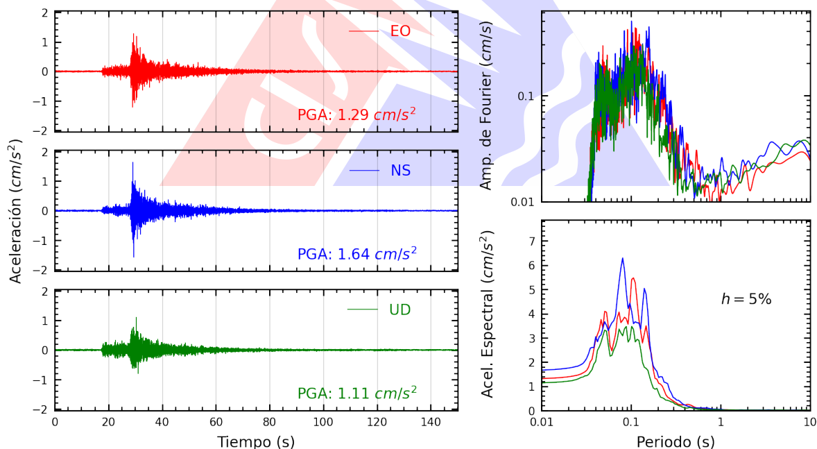
Figura A.16: Registros tiempo-historia, espectros de Fourier y de respuesta en las direcciones EO, NS y vertical de la estación JALVA. Sismo de Huacho, Huaura - Lima del 2026-07-24, 21:48:11 (Hora local)
