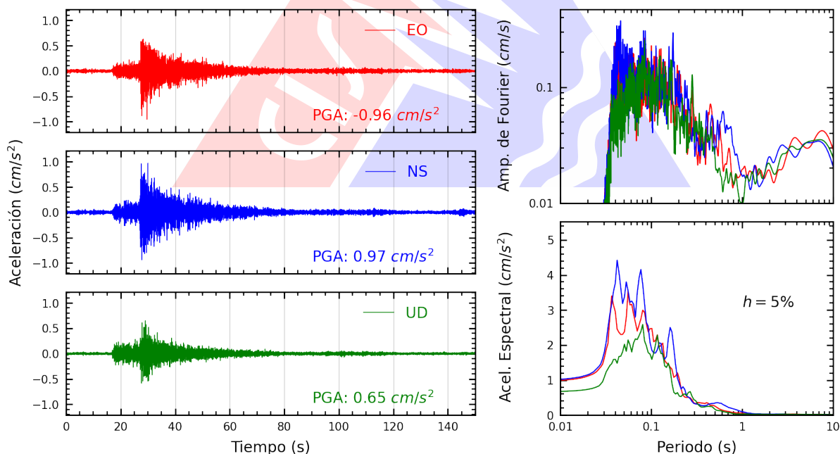
Figura A.24: Registros tiempo-historia, espectros de Fourier y de respuesta en las direcciones EO, NS y vertical de la estación COMAS. Sismo de Huacho, Huaura - Lima del 2026-07-24, 21:48:11 (Hora local)
