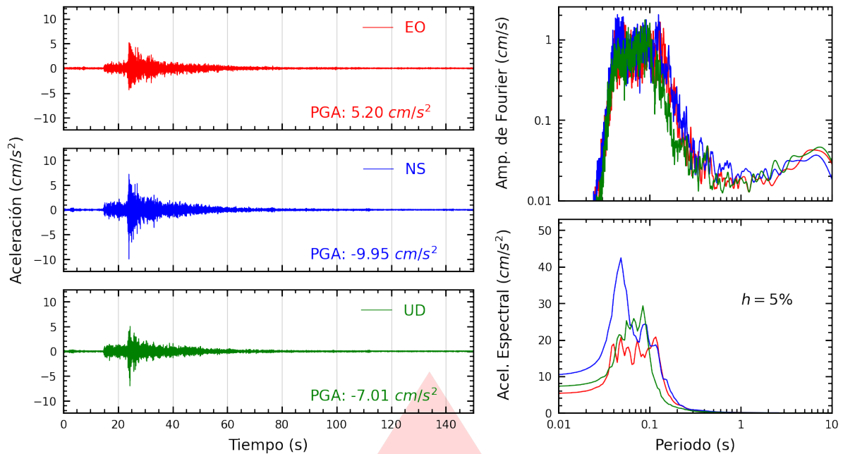
Figura A.1: Registros tiempo-historia, espectros de Fourier y de respuesta en las direcciones EO, NS y vertical de la estación SROSA. Sismo de Huacho, Huaura - Lima del 2026-07-24, 21:48:11 (Hora local)
