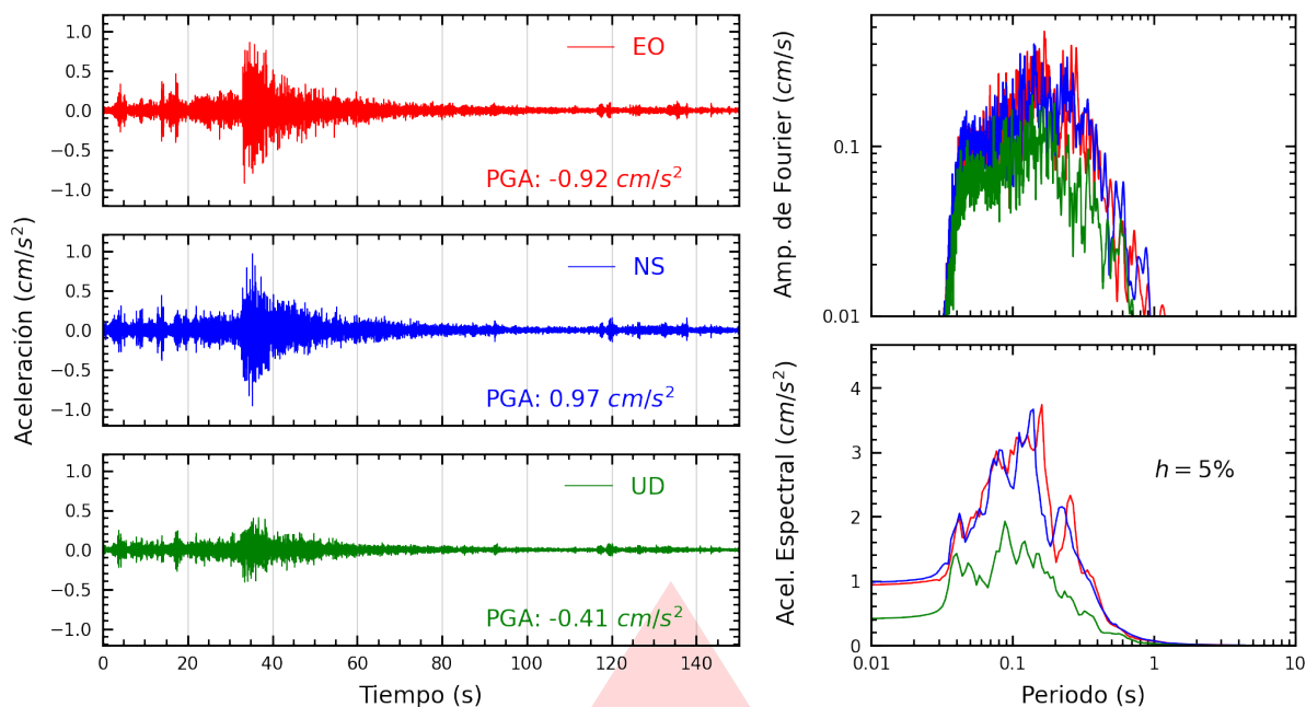
Figura A.25: Registros tiempo-historia, espectros de Fourier y de respuesta en las direcciones EO, NS y vertical de la estación BRIS2. Sismo de Huacho, Huaura - Lima del 2026-07-24, 21:48:11 (Hora local)
