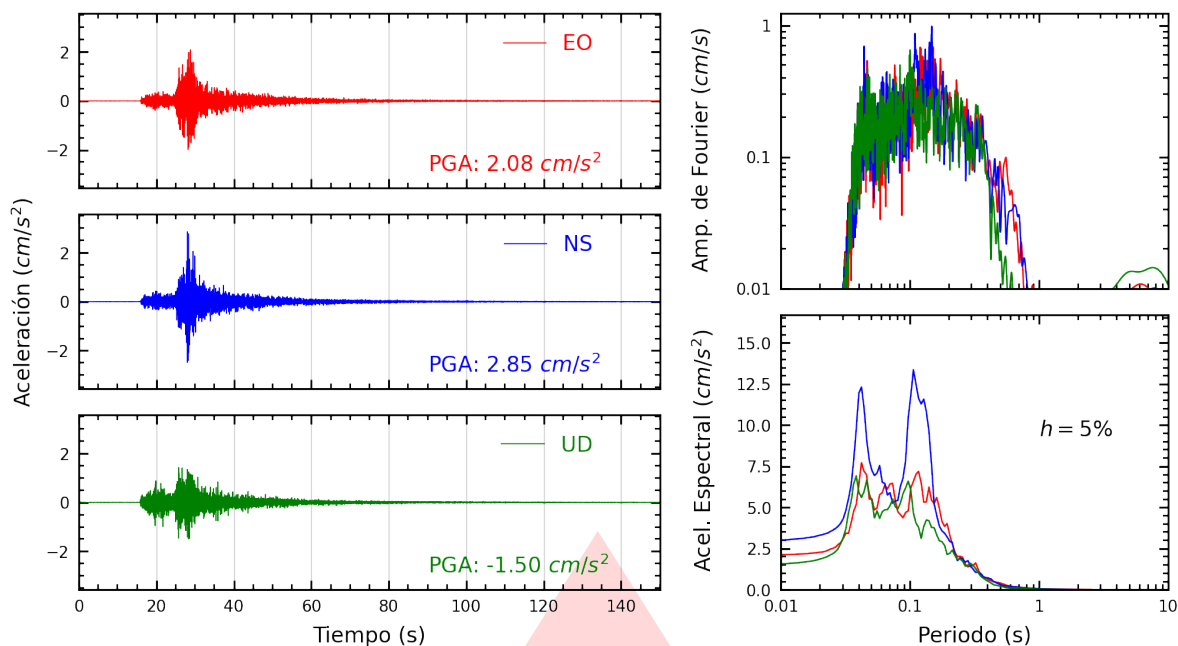
Figura A.7: Registros tiempo-historia, espectros de Fourier y de respuesta en las direcciones EO, NS y vertical de la estación CARAL. Sismo de Huacho, Huaura - Lima del 2026-07-24, 21:48:11 (Hora local)
