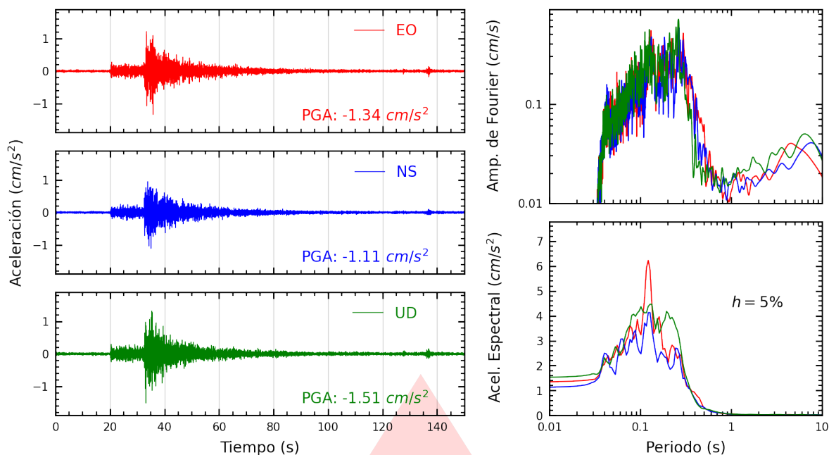
Figura A.17: Registros tiempo-historia, espectros de Fourier y de respuesta en las direcciones EO, NS y vertical de la estación SOVES. Sismo de Huacho, Huaura - Lima del 2026-07-24, 21:48:11 (Hora local)
