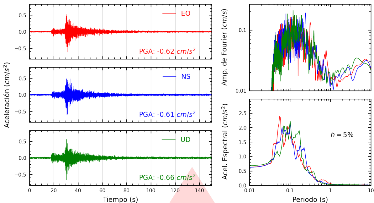
Figura A.37: Registros tiempo-historia, espectros de Fourier y de respuesta en las direcciones EO, NS y vertical de la estación UNFV. Sismo de Huacho, Huaura - Lima del 2026-07-24, 21:48:11 (Hora local)
