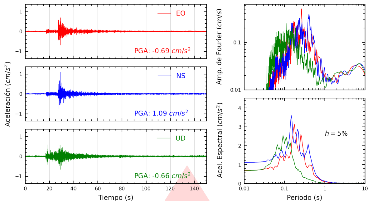
Figura A.21: Registros tiempo-historia, espectros de Fourier y de respuesta en las direcciones EO, NS y vertical de la estación ACAPU. Sismo de Huacho, Huaura - Lima del 2026-07-24, 21:48:11 (Hora local)
