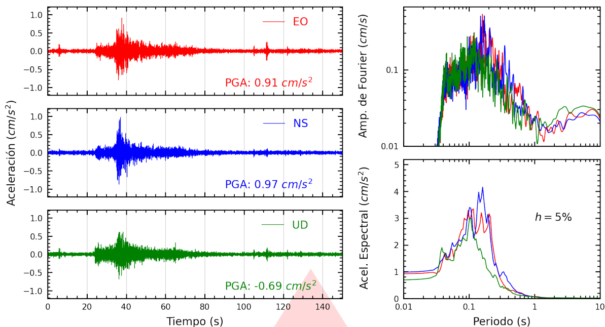
Figura A.23: Registros tiempo-historia, espectros de Fourier y de respuesta en las direcciones EO, NS y vertical de la estación PRADO. Sismo de Huacho, Huaura - Lima del 2026-07-24, 21:48:11 (Hora local)
