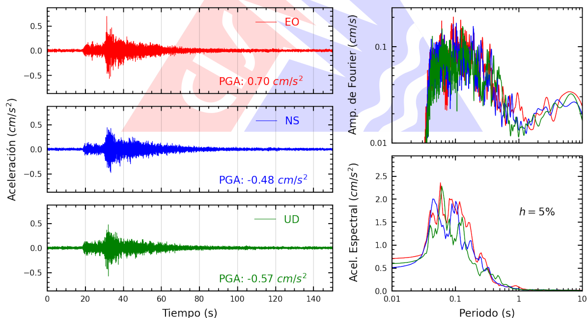
Figura A.32: Registros tiempo-historia, espectros de Fourier y de respuesta en las direcciones EO, NS y vertical de la estación IMCA. Sismo de Huacho, Huaura - Lima del 2026-07-24, 21:48:11 (Hora local)
