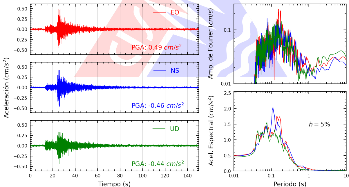
Figura A.40: Registros tiempo-historia, espectros de Fourier y de respuesta en las direcciones EO, NS y vertical de la estación UNMSM. Sismo de Huacho, Huaura - Lima del 2026-07-24, 21:48:11 (Hora local)
