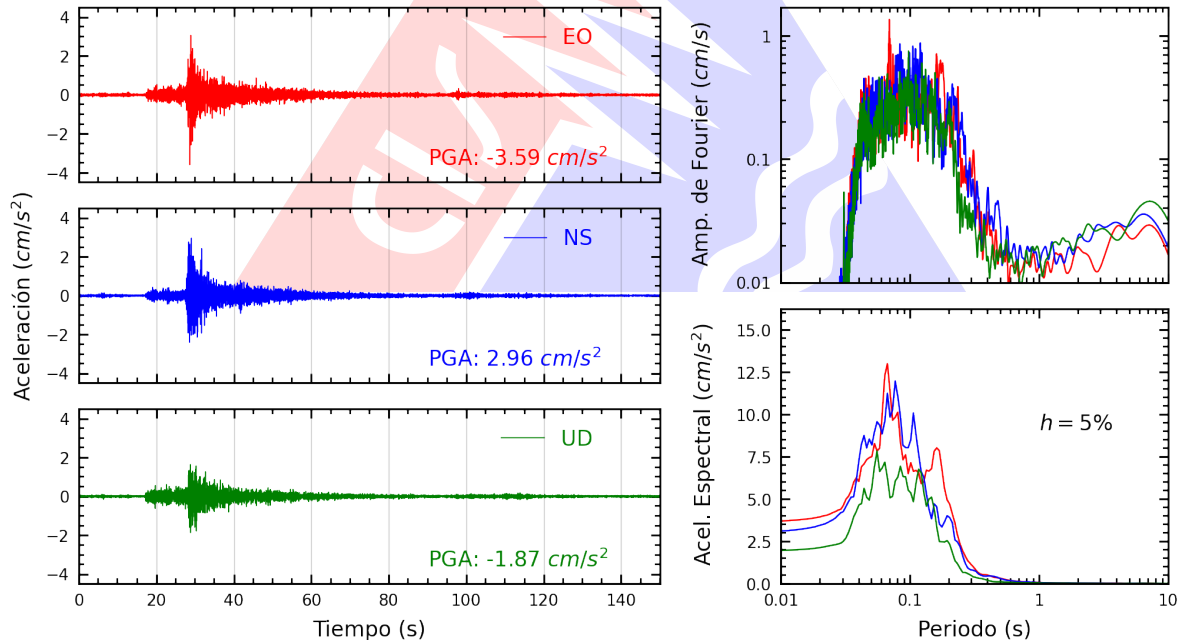
Figura A.2: Registros tiempo-historia, espectros de Fourier y de respuesta en las direcciones EO, NS y vertical de la estación INDEP. Sismo de Huacho, Huaura - Lima del 2026-07-24, 21:48:11 (Hora local)
