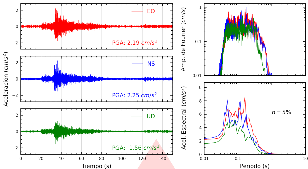
Figura A.9: Registros tiempo-historia, espectros de Fourier y de respuesta en las direcciones EO, NS y vertical de la estación UNTEL. Sismo de Huacho, Huaura - Lima del 2026-07-24, 21:48:11 (Hora local)
