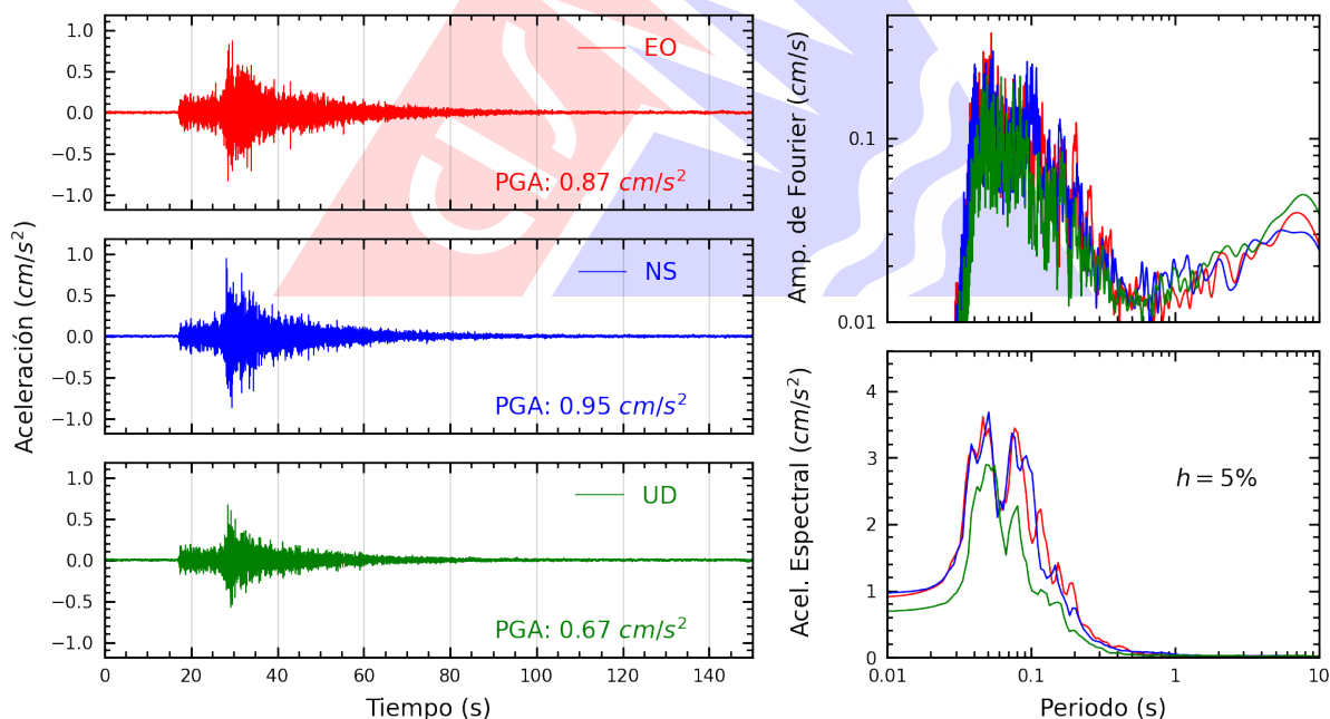
Figura A.26: Registros tiempo-historia, espectros de Fourier y de respuesta en las direcciones EO, NS y vertical de la estación UCSS. Sismo de Huacho, Huaura - Lima del 2026-07-24, 21:48:11 (Hora local)
