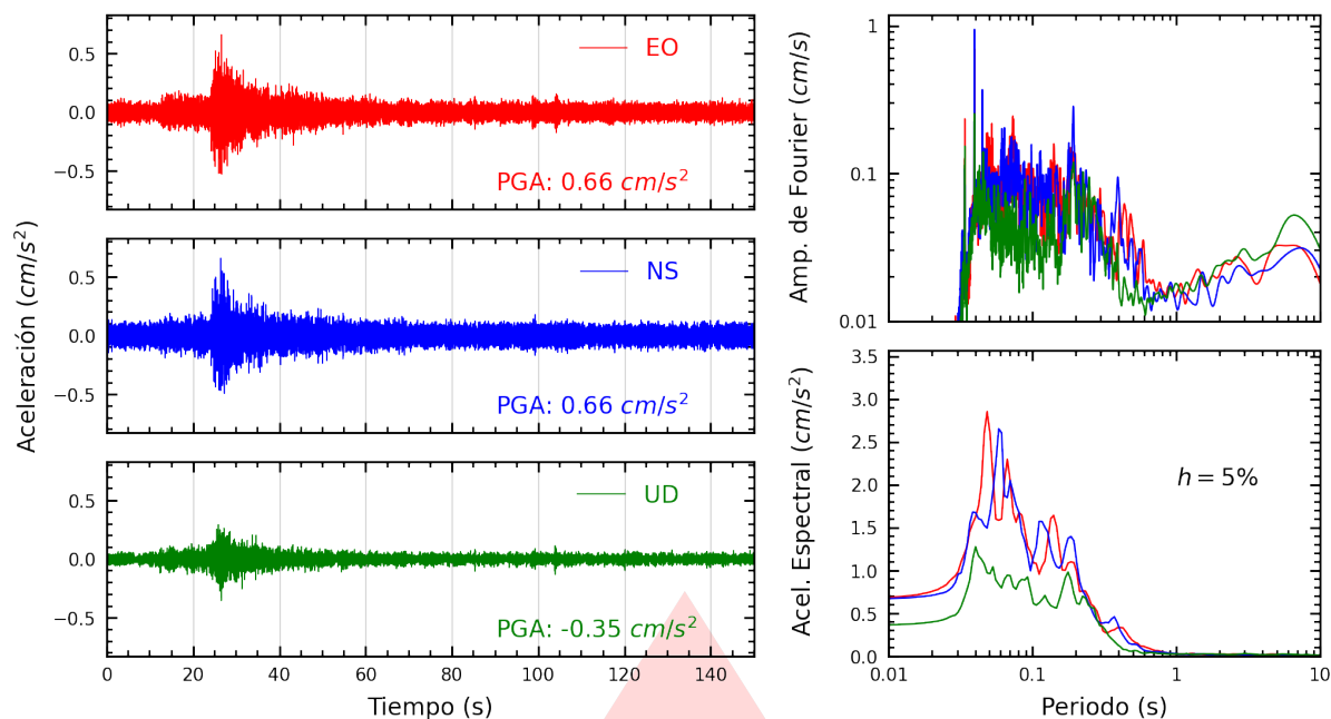
Figura A.35: Registros tiempo-historia, espectros de Fourier y de respuesta en las direcciones EO, NS y vertical de la estación UPCVI. Sismo de Huacho, Huaura - Lima del 2026-07-24, 21:48:11 (Hora local)
