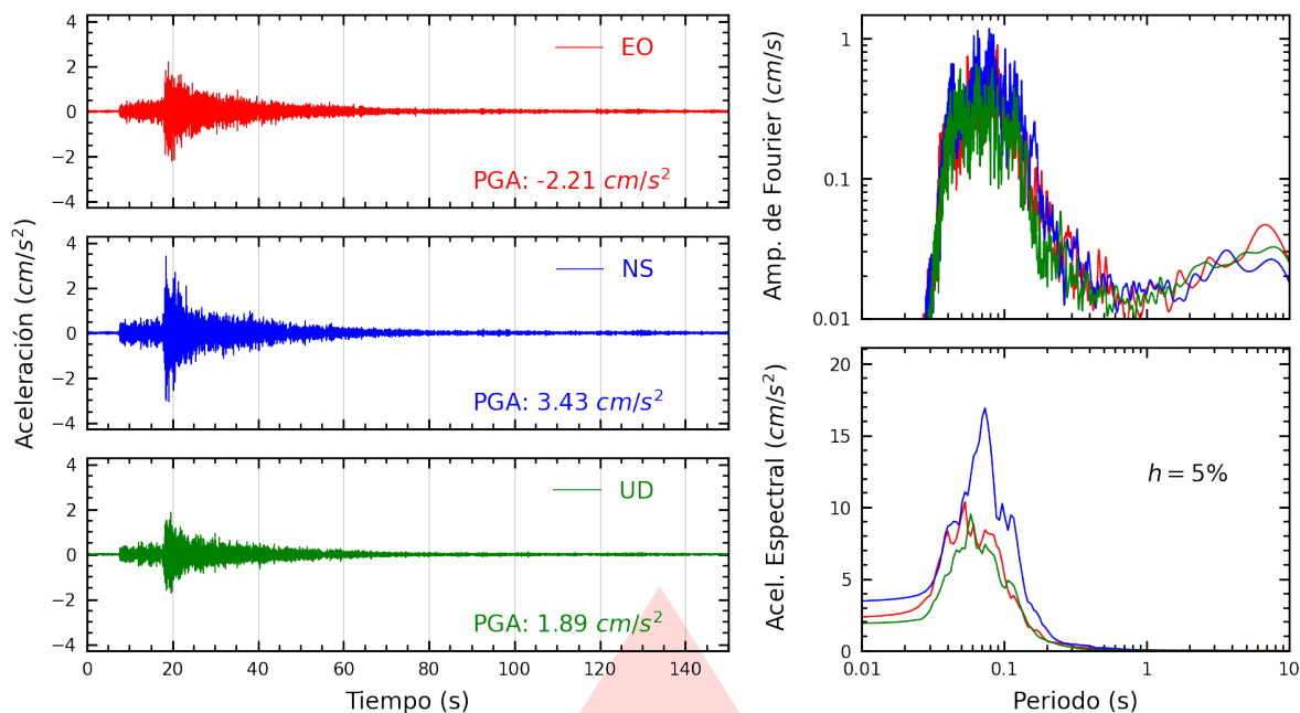
Figura A.3: Registros tiempo-historia, espectros de Fourier y de respuesta en las direcciones EO, NS y vertical de la estación JOSEO. Sismo de Huacho, Huaura - Lima del 2026-07-24, 21:48:11 (Hora local)
