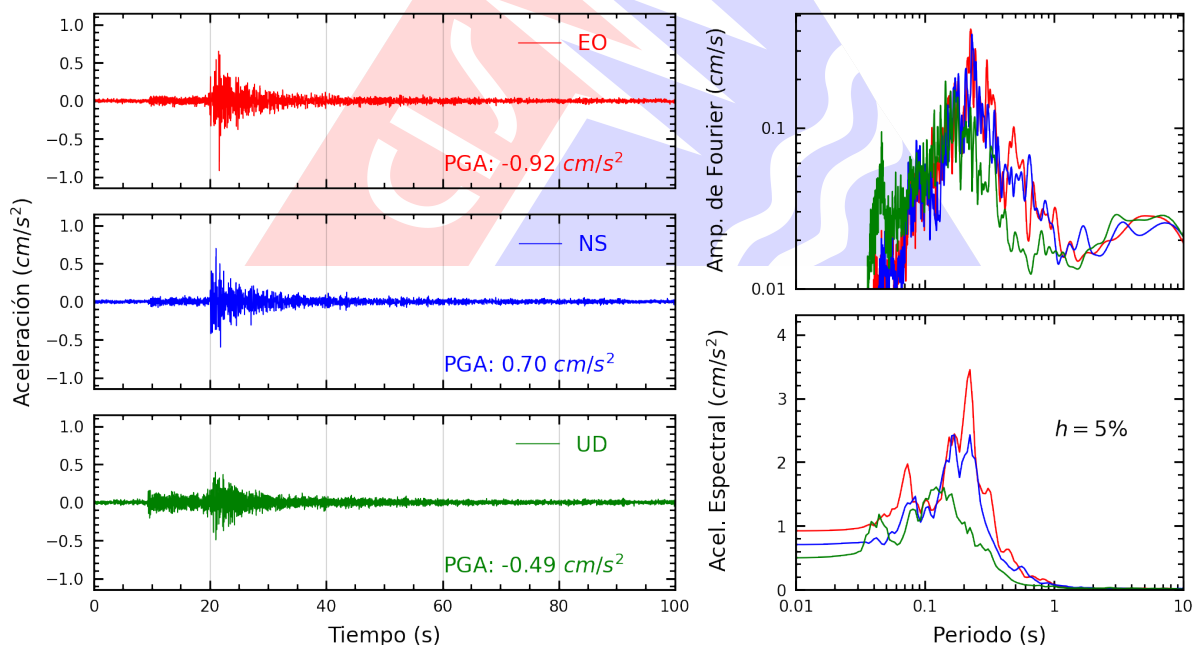
Figura A.28: Registros tiempo-historia, espectros de Fourier y de respuesta en las direcciones EO, NS y vertical de la estación DSMI. Sismo de Huacho, Huaura - Lima del 2026-07-24, 21:48:11 (Hora local)
