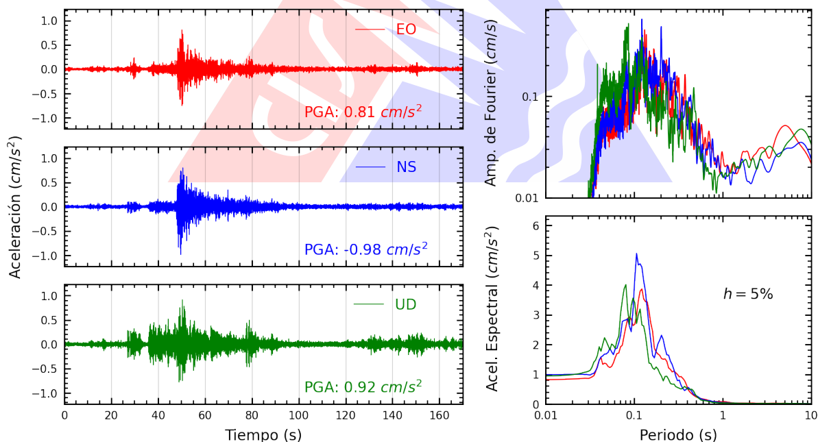
Figura A.22: Registros tiempo-historia, espectros de Fourier y de respuesta en las direcciones EO, NS y vertical de la estación SOCHO. Sismo de Huacho, Huaura - Lima del 2026-07-24, 21:48:11 (Hora local)
