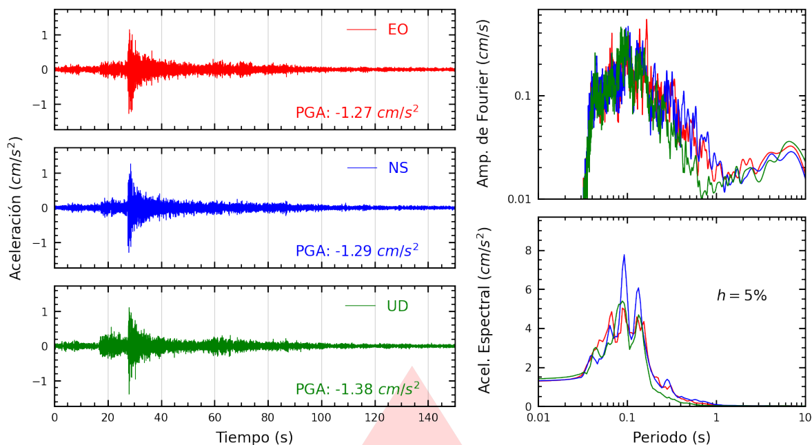
Figura A.19: Registros tiempo-historia, espectros de Fourier y de respuesta en las direcciones EO, NS y vertical de la estación MADRE. Sismo de Huacho, Huaura - Lima del 2026-07-24, 21:48:11 (Hora local)
