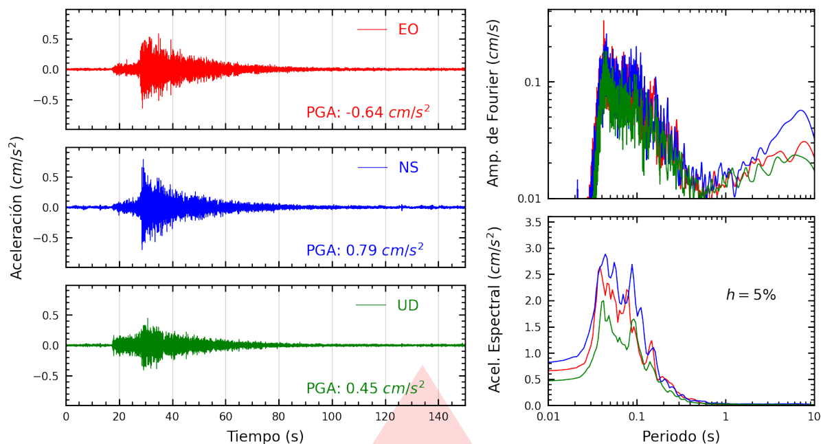
Figura A.31: Registros tiempo-historia, espectros de Fourier y de respuesta en las direcciones EO, NS y vertical de la estación SJLCE. Sismo de Huacho, Huaura - Lima del 2026-07-24, 21:48:11 (Hora local)
