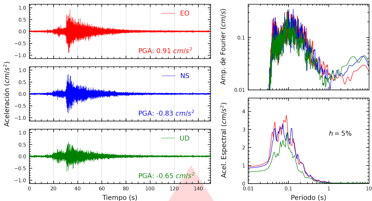
Figura A.29: Registros tiempo-historia, espectros de Fourier y de respuesta en las direcciones EO, NS y vertical de la estación UCVAT. Sismo de Huacho, Huaura - Lima del 2026-07-24, 21:48:11 (Hora local)
