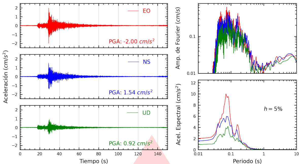
Figura A.11: Registros tiempo-historia, espectros de Fourier y de respuesta en las direcciones EO, NS y vertical de la estación FICPE. Sismo de Huacho, Huaura - Lima del 2026-07-24, 21:48:11 (Hora local)
