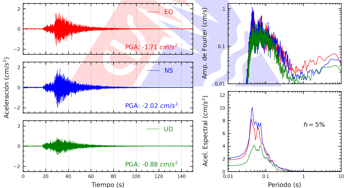
Figura A.10: Registros tiempo-historia, espectros de Fourier y de respuesta en las direcciones EO, NS y vertical de la estación UNAB. Sismo de Huacho, Huaura - Lima del 2026-07-24, 21:48:11 (Hora local)
