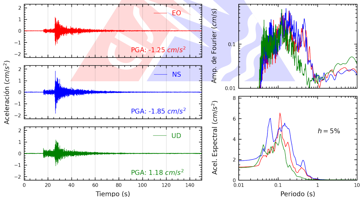
Figura A.12: Registros tiempo-historia, espectros de Fourier y de respuesta en las direcciones EO, NS y vertical de la estación VHAYA. Sismo de Huacho, Huaura - Lima del 2026-07-24, 21:48:11 (Hora local)
