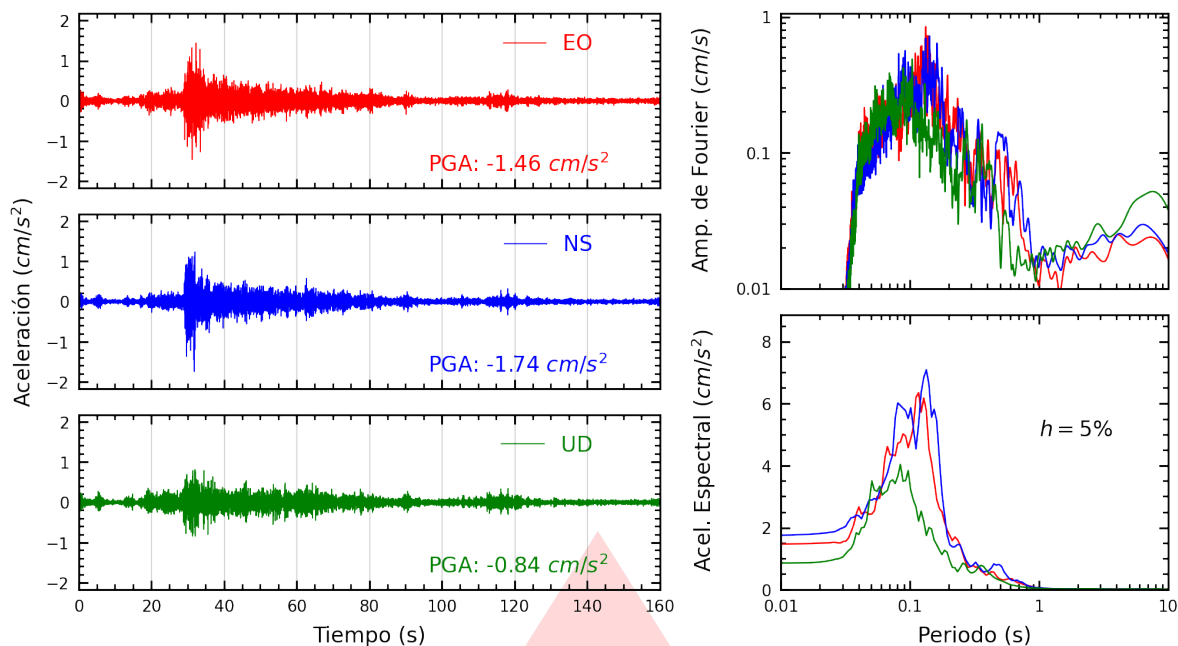
Figura A.13: Registros tiempo-historia, espectros de Fourier y de respuesta en las direcciones EO, NS y vertical de la estación SJLSV. Sismo de Huacho, Huaura - Lima del 2026-07-24, 21:48:11 (Hora local)
