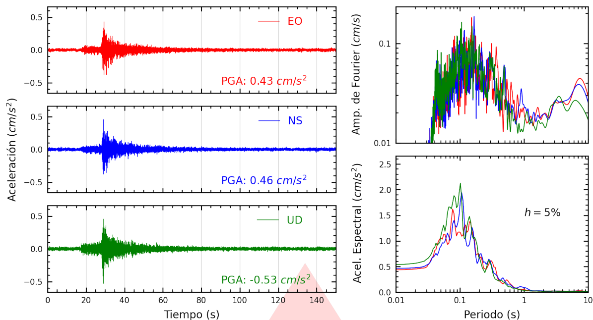
Figura A.39: Registros tiempo-historia, espectros de Fourier y de respuesta en las direcciones EO, NS y vertical de la estación BONDY. Sismo de Huacho, Huaura - Lima del 2026-07-24, 21:48:11 (Hora local)
