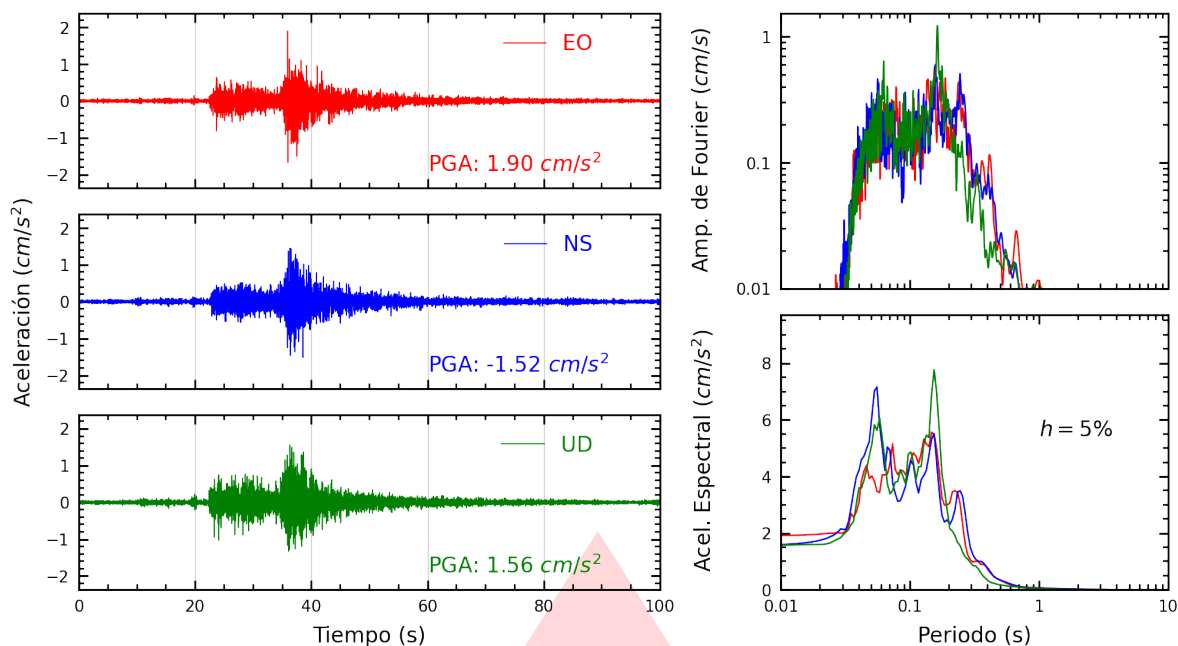
Figura A.3: Registros tiempo-historia, espectros de Fourier y de respuesta en las direcciones EO, NS y vertical de la estación UJBG4. Sismo de Ilo, Ilo - Moquegua del 2026-07-25, 13:58:43 (Hora local)
