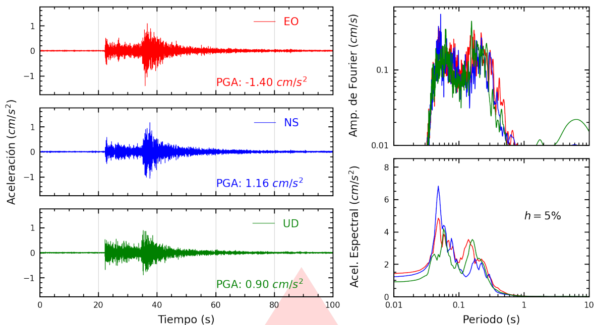
Figura A.5: Registros tiempo-historia, espectros de Fourier y de respuesta en las direcciones EO, NS y vertical de la estación CREY. Sismo de Ilo, Ilo - Moquegua del 2026-07-25, 13:58:43 (Hora local)
