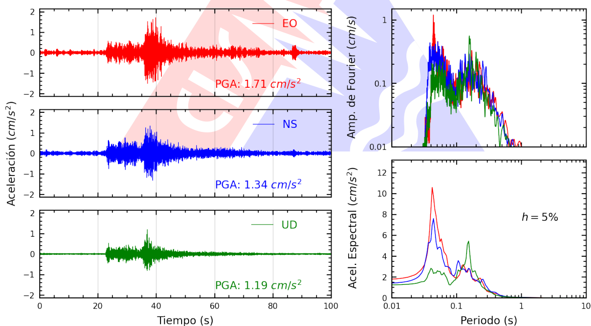
Figura A.4: Registros tiempo-historia, espectros de Fourier y de respuesta en las direcciones EO, NS y vertical de la estación UPTAC. Sismo de Ilo, Ilo - Moquegua del 2026-07-25, 13:58:43 (Hora local)
