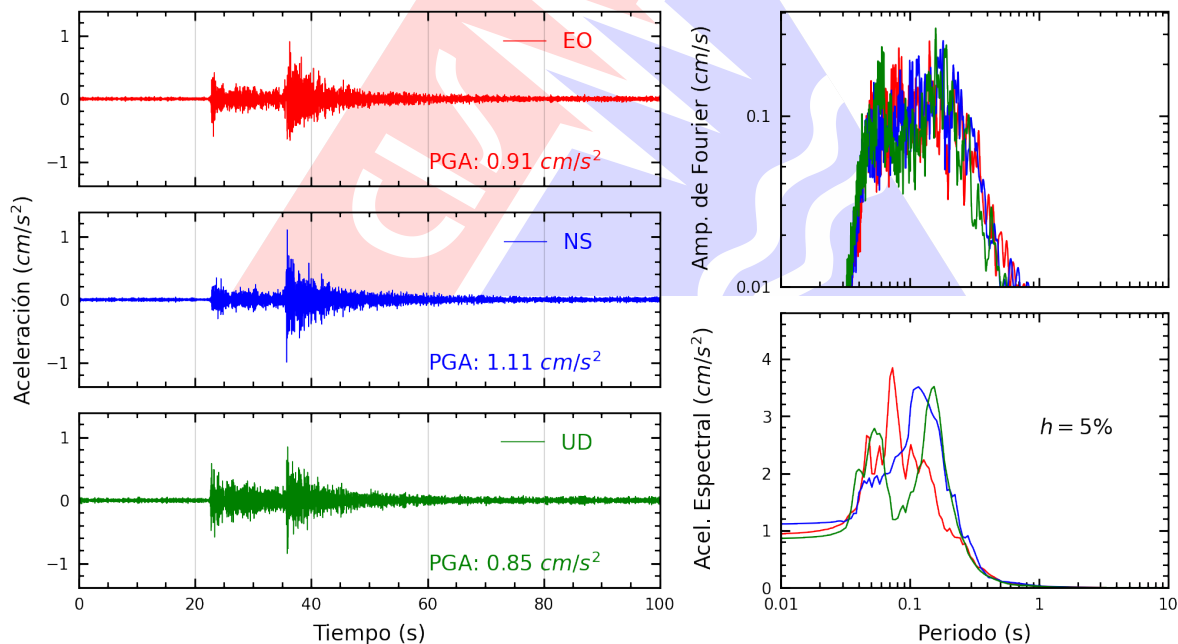
Figura A.6: Registros tiempo-historia, espectros de Fourier y de respuesta en las direcciones EO, NS y vertical de la estación UJB2. Sismo de Ilo, Ilo - Moquegua del 2026-07-25, 13:58:43 (Hora local)
