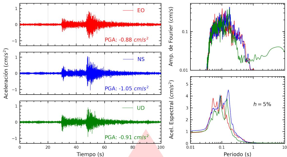
Figura A.7: Registros tiempo-historia, espectros de Fourier y de respuesta en las direcciones EO, NS y vertical de la estación SCARQ. Sismo de Ilo, Ilo - Moquegua del 2026-07-25, 13:58:43 (Hora local)
