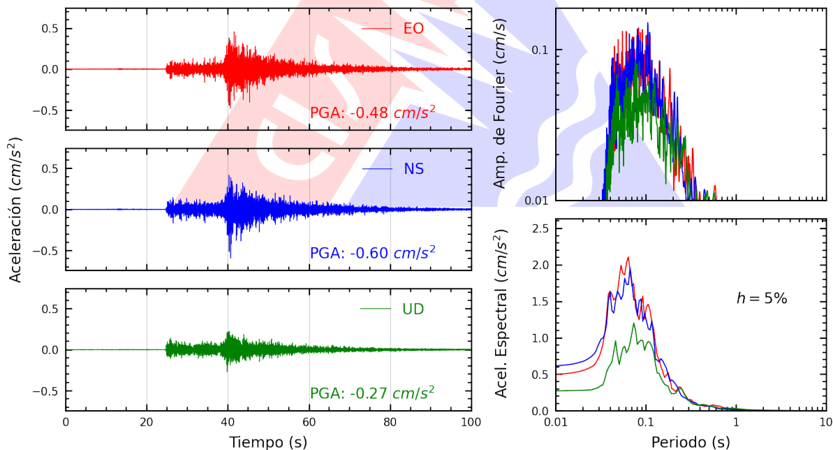
Figura A.8: Registros tiempo-historia, espectros de Fourier y de respuesta en las direcciones EO, NS y vertical de la estación UNSA2. Sismo de Ilo, Ilo - Moquegua del 2026-07-25, 13:58:43 (Hora local)
