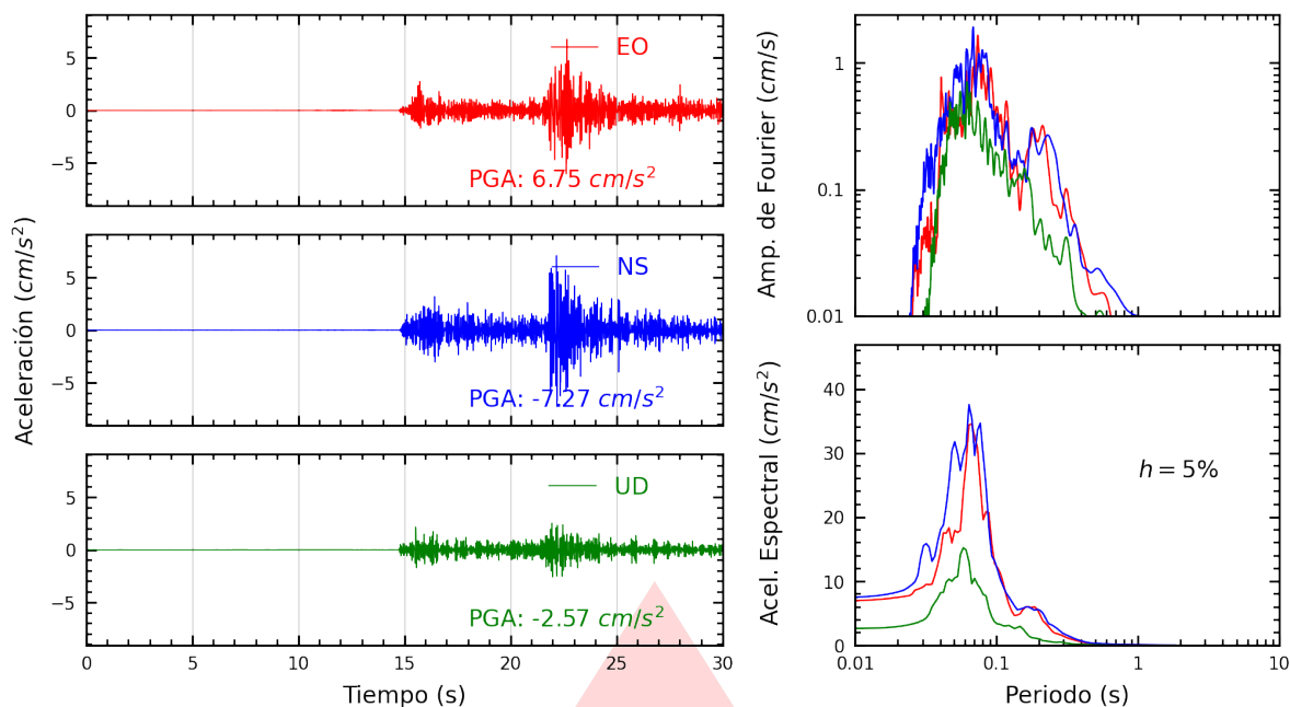
Figura A.1: Registros tiempo-historia, espectros de Fourier y de respuesta en las direcciones EO, NS y vertical de la estación UNAM. Sismo de Ilo, Ilo - Moquegua del 2026-07-25, 13:58:43 (Hora local)
