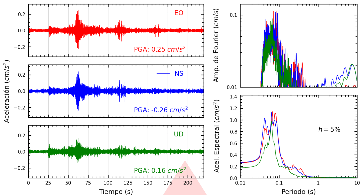
Figura A.1: Registros tiempo-historia, espectros de Fourier y de respuesta en las direcciones EO, NS y vertical de la estación CREY. Sismo de Santa Lucía, Lampa - Puno del 2026-07-30, 19:04:06 (Hora local)
