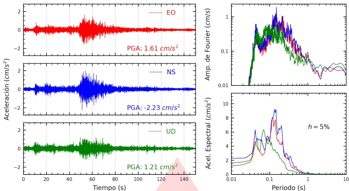
Figura A.9: Registros tiempo-historia, espectros de Fourier y de respuesta en las direcciones EO, NS y vertical de la estación CARAB. Sismo de Aucayacu, Leoncio Prado - Huánuco del 2026-08-02, 20:42:22 (Hora local)
