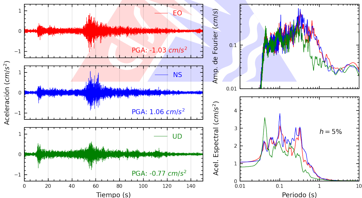
Figura A.32: Registros tiempo-historia, espectros de Fourier y de respuesta en las direcciones EO, NS y vertical de la estación MADRE. Sismo de Aucayacu, Leoncio Prado - Huánuco del 2026-08-02, 20:42:22 (Hora local)
