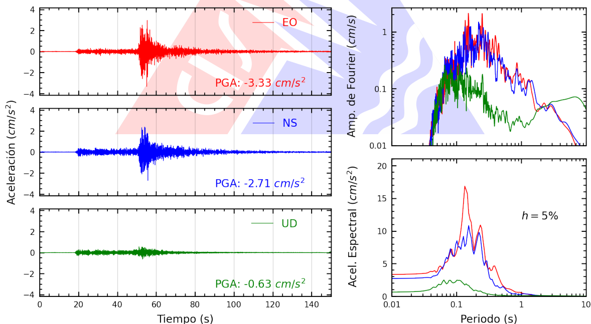
Figura A.6: Registros tiempo-historia, espectros de Fourier y de respuesta en las direcciones EO, NS y vertical de la estación UNAAA. Sismo de Aucayacu, Leoncio Prado - Huánuco del 2026-08-02, 20:42:22 (Hora local)
