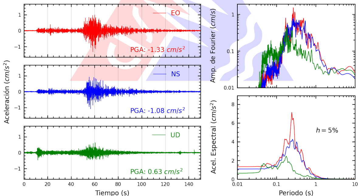
Figura A.24: Registros tiempo-historia, espectros de Fourier y de respuesta en las direcciones EO, NS y vertical de la estación ACAPU. Sismo de Aucayacu, Leoncio Prado - Huánuco del 2026-08-02, 20:42:22 (Hora local)
