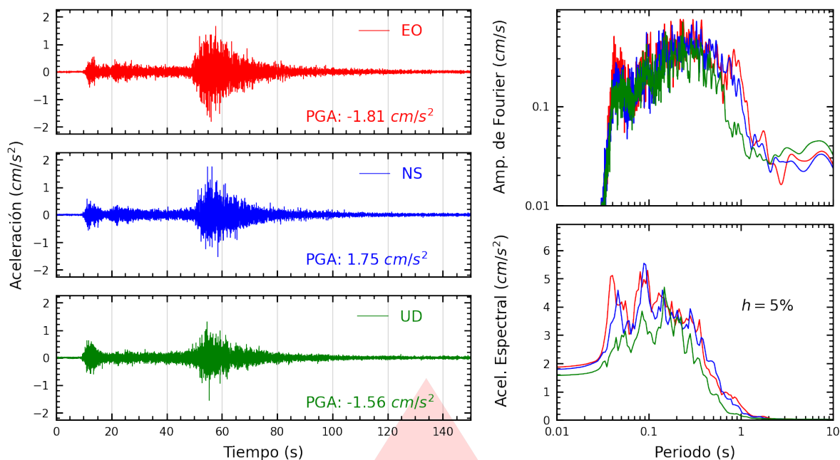
Figura A.15: Registros tiempo-historia, espectros de Fourier y de respuesta en las direcciones EO, NS y vertical de la estación UCVAT. Sismo de Aucayacu, Leoncio Prado - Huánuco del 2026-08-02, 20:42:22 (Hora local)
