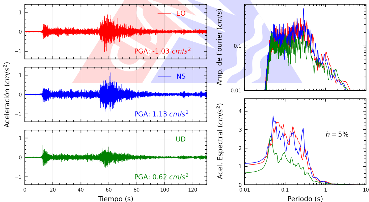
Figura A.28: Registros tiempo-historia, espectros de Fourier y de respuesta en las direcciones EO, NS y vertical de la estación PACHA. Sismo de Aucayacu, Leoncio Prado - Huánuco del 2026-08-02, 20:42:22 (Hora local)
