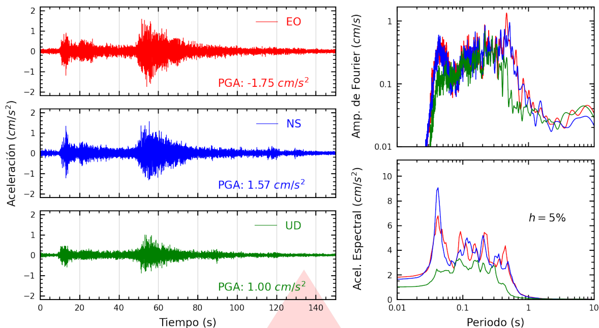
Figura A.17: Registros tiempo-historia, espectros de Fourier y de respuesta en las direcciones EO, NS y vertical de la estación OLIVO. Sismo de Aucayacu, Leoncio Prado - Huánuco del 2026-08-02, 20:42:22 (Hora local)
