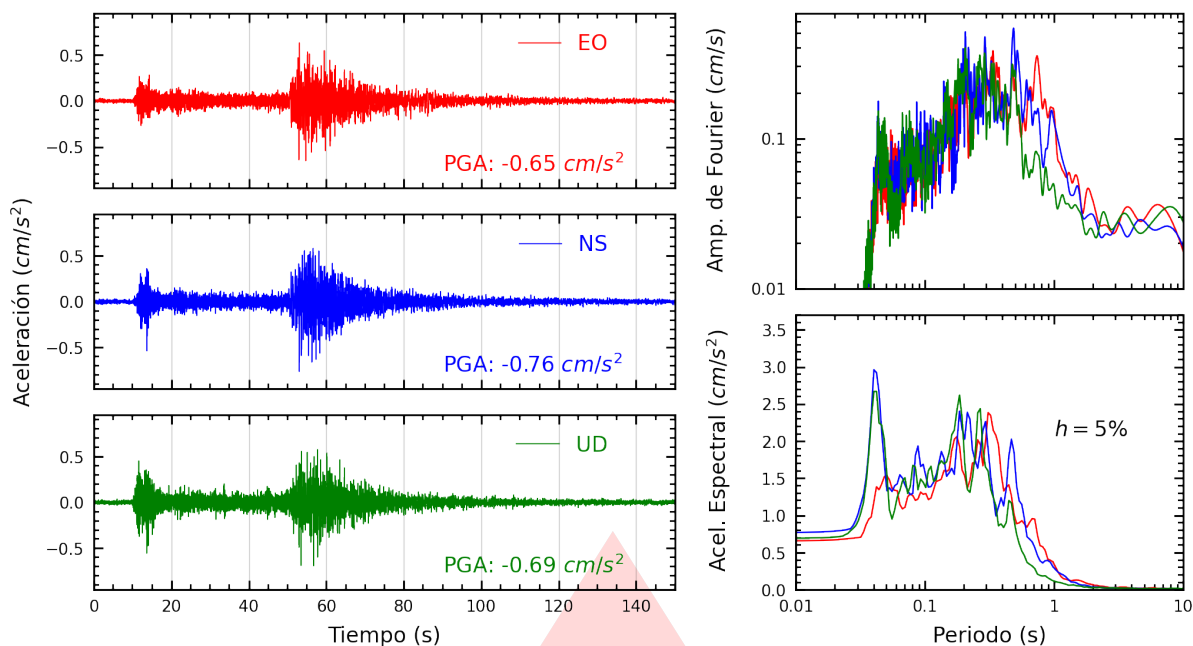
Figura A.41: Registros tiempo-historia, espectros de Fourier y de respuesta en las direcciones EO, NS y vertical de la estación UNFV. Sismo de Aucayacu, Leoncio Prado - Huánuco del 2026-08-02, 20:42:22 (Hora local)
