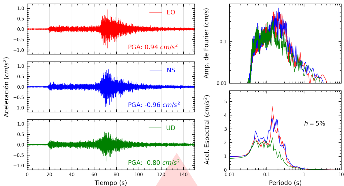
Figura A.35: Registros tiempo-historia, espectros de Fourier y de respuesta en las direcciones EO, NS y vertical de la estación ASIA. Sismo de Aucayacu, Leoncio Prado - Huánuco del 2026-08-02, 20:42:22 (Hora local)
