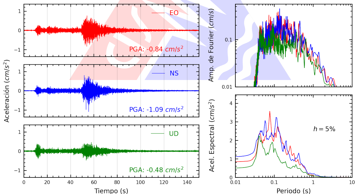
Figura A.30: Registros tiempo-historia, espectros de Fourier y de respuesta en las direcciones EO, NS y vertical de la estación ATARJ. Sismo de Aucayacu, Leoncio Prado - Huánuco del 2026-08-02, 20:42:22 (Hora local)
