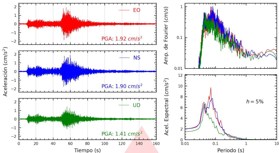
Figura A.13: Registros tiempo-historia, espectros de Fourier y de respuesta en las direcciones EO, NS y vertical de la estación JOSEO. Sismo de Aucayacu, Leoncio Prado - Huánuco del 2026-08-02, 20:42:22 (Hora local)
