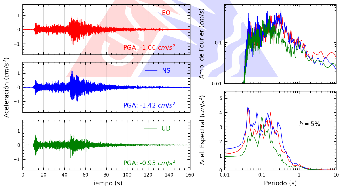
Figura A.22: Registros tiempo-historia, espectros de Fourier y de respuesta en las direcciones EO, NS y vertical de la estación UNAB. Sismo de Aucayacu, Leoncio Prado - Huánuco del 2026-08-02, 20:42:22 (Hora local)
