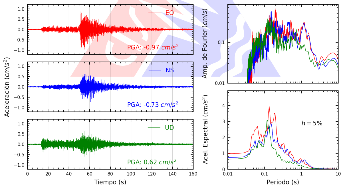
Figura A.34: Registros tiempo-historia, espectros de Fourier y de respuesta en las direcciones EO, NS y vertical de la estación UPAOT. Sismo de Aucayacu, Leoncio Prado - Huánuco del 2026-08-02, 20:42:22 (Hora local)
