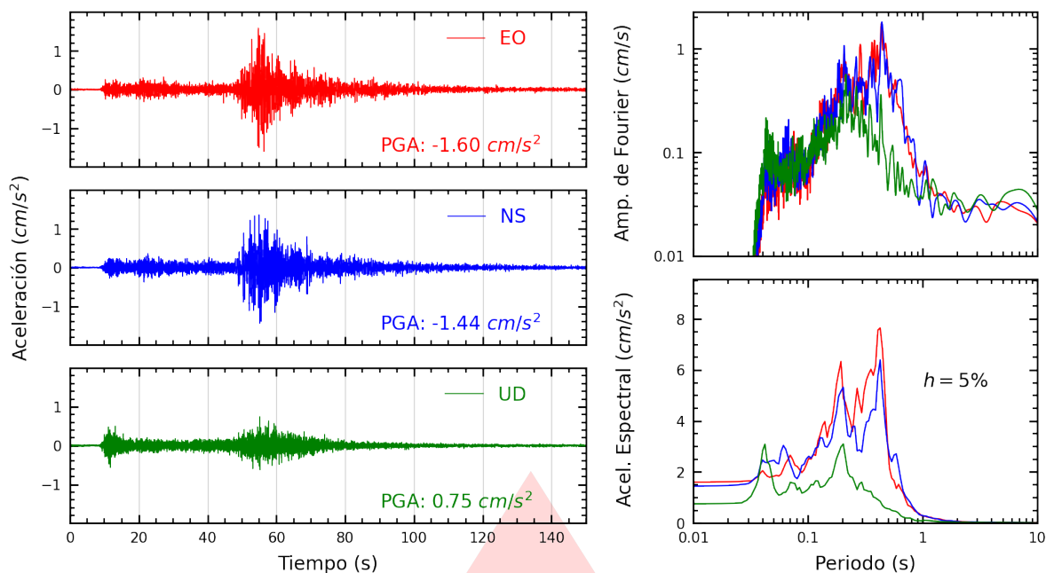
Figura A.21: Registros tiempo-historia, espectros de Fourier y de respuesta en las direcciones EO, NS y vertical de la estación VHAYA. Sismo de Aucayacu, Leoncio Prado - Huánuco del 2026-08-02, 20:42:22 (Hora local)
