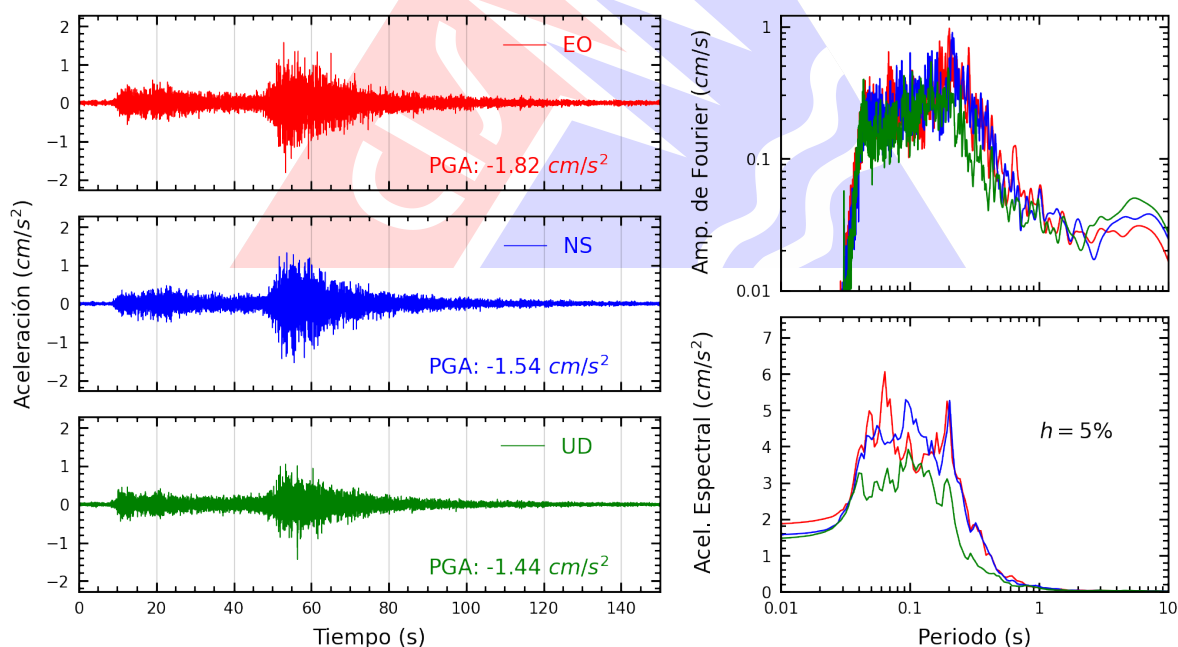
Figura A.14: Registros tiempo-historia, espectros de Fourier y de respuesta en las direcciones EO, NS y vertical de la estación INDEP. Sismo de Aucayacu, Leoncio Prado - Huánuco del 2026-08-02, 20:42:22 (Hora local)
