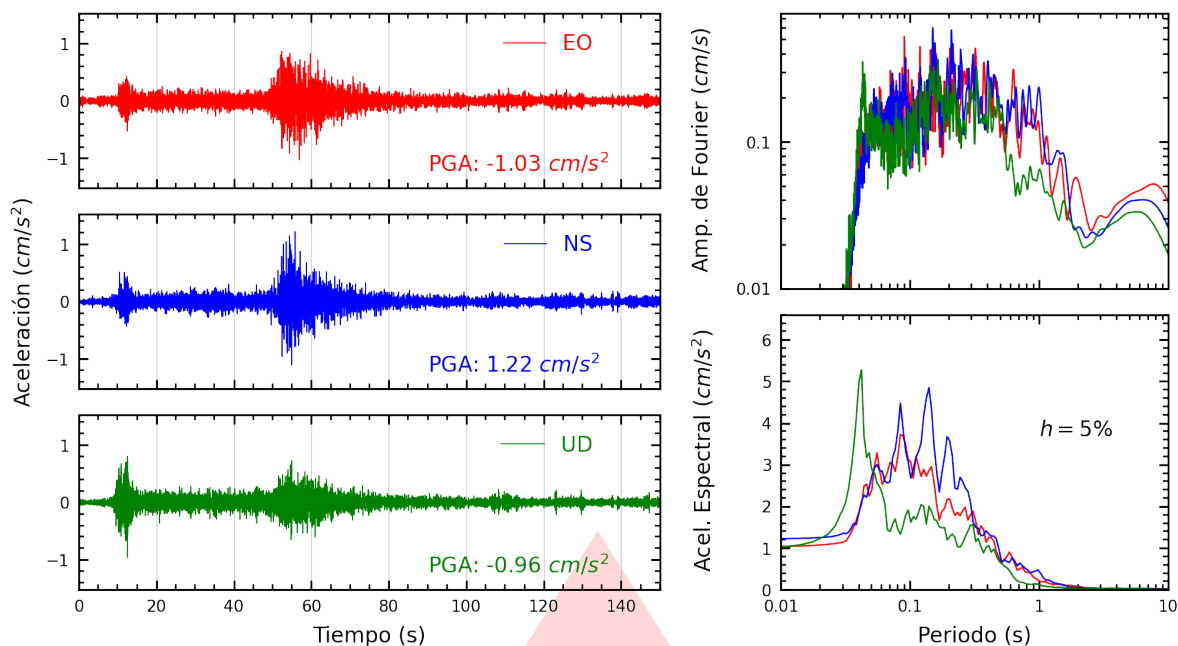
Figura A.27: Registros tiempo-historia, espectros de Fourier y de respuesta en las direcciones EO, NS y vertical de la estación UPCSM. Sismo de Aucayacu, Leoncio Prado - Huánuco del 2026-08-02, 20:42:22 (Hora local)
