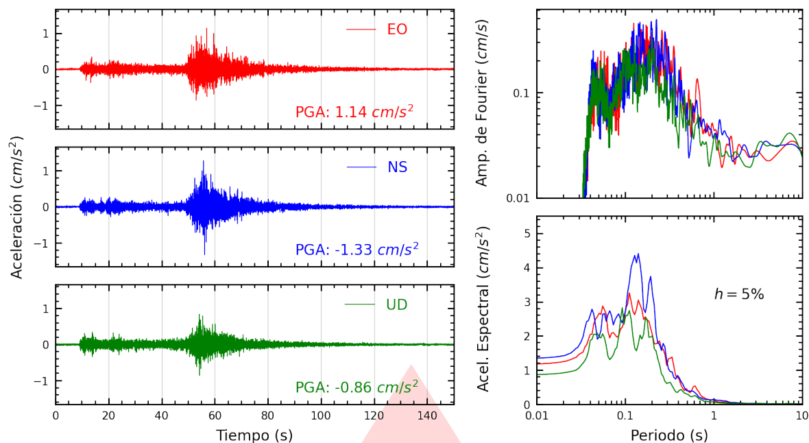
Figura A.25: Registros tiempo-historia, espectros de Fourier y de respuesta en las direcciones EO, NS y vertical de la estación JALVA. Sismo de Aucayacu, Leoncio Prado - Huánuco del 2026-08-02, 20:42:22 (Hora local)
