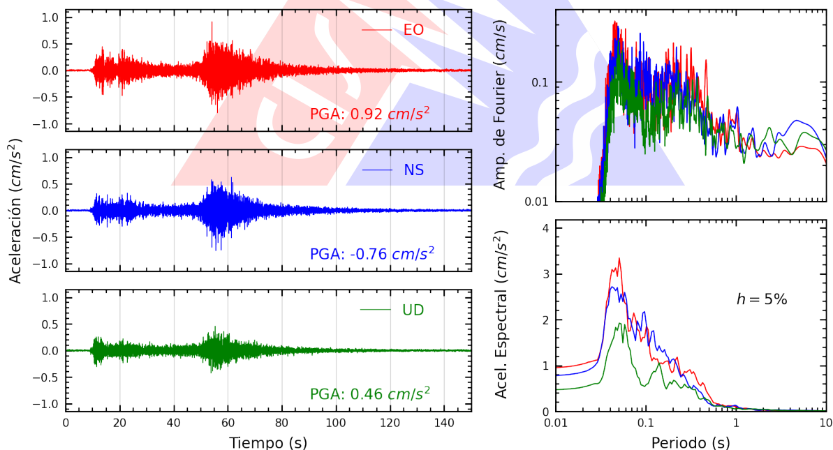
Figura A.36: Registros tiempo-historia, espectros de Fourier y de respuesta en las direcciones EO, NS y vertical de la estación UCSS. Sismo de Aucayacu, Leoncio Prado - Huánuco del 2026-08-02, 20:42:22 (Hora local)
