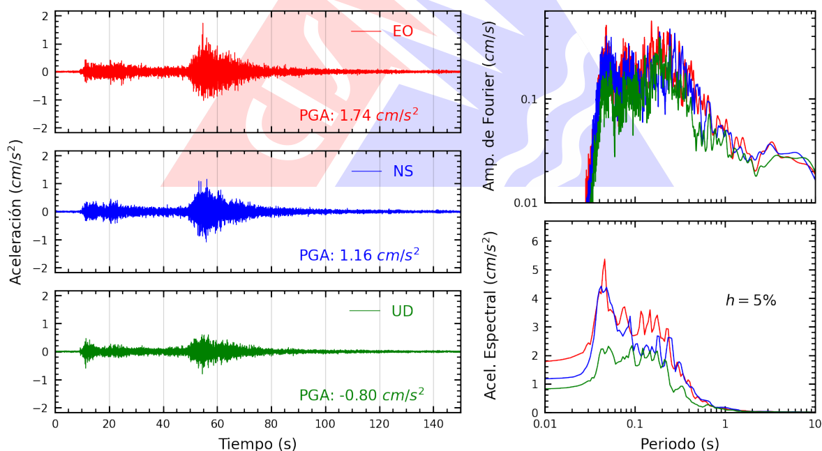
Figura A.18: Registros tiempo-historia, espectros de Fourier y de respuesta en las direcciones EO, NS y vertical de la estación FICPE. Sismo de Aucayacu, Leoncio Prado - Huánuco del 2026-08-02, 20:42:22 (Hora local)
