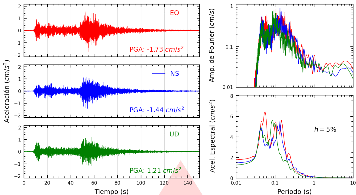
Figura A.19: Registros tiempo-historia, espectros de Fourier y de respuesta en las direcciones EO, NS y vertical de la estación AMORE. Sismo de Aucayacu, Leoncio Prado - Huánuco del 2026-08-02, 20:42:22 (Hora local)
