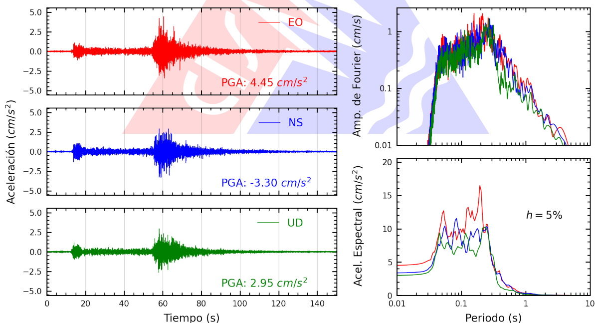
Figura A.2: Registros tiempo-historia, espectros de Fourier y de respuesta en las direcciones EO, NS y vertical de la estación PHERM. Sismo de Aucayacu, Leoncio Prado - Huánuco del 2026-08-02, 20:42:22 (Hora local)
