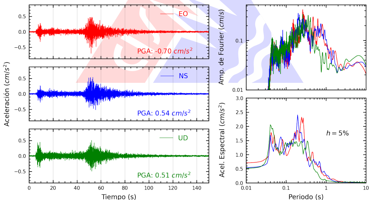
Figura A.42: Registros tiempo-historia, espectros de Fourier y de respuesta en las direcciones EO, NS y vertical de la estación UNMSM. Sismo de Aucayacu, Leoncio Prado - Huánuco del 2026-08-02, 20:42:22 (Hora local)
