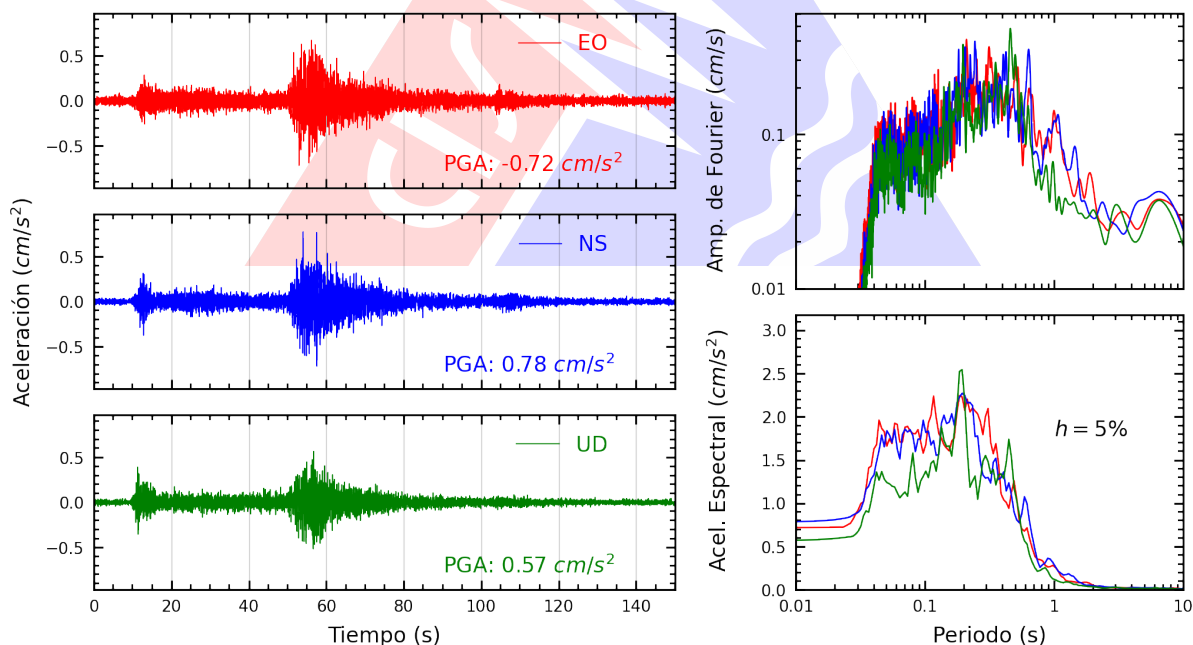
Figura A.40: Registros tiempo-historia, espectros de Fourier y de respuesta en las direcciones EO, NS y vertical de la estación INICT. Sismo de Aucayacu, Leoncio Prado - Huánuco del 2026-08-02, 20:42:22 (Hora local)
