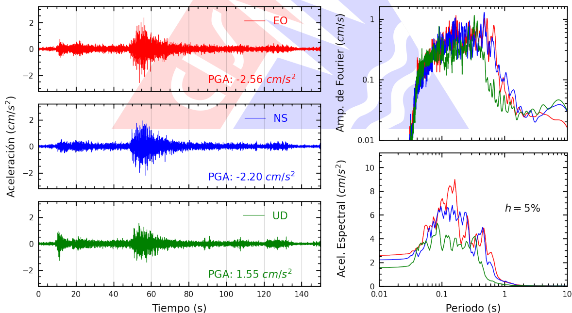
Figura A.8: Registros tiempo-historia, espectros de Fourier y de respuesta en las direcciones EO, NS y vertical de la estación SJLSV. Sismo de Aucayacu, Leoncio Prado - Huánuco del 2026-08-02, 20:42:22 (Hora local)
