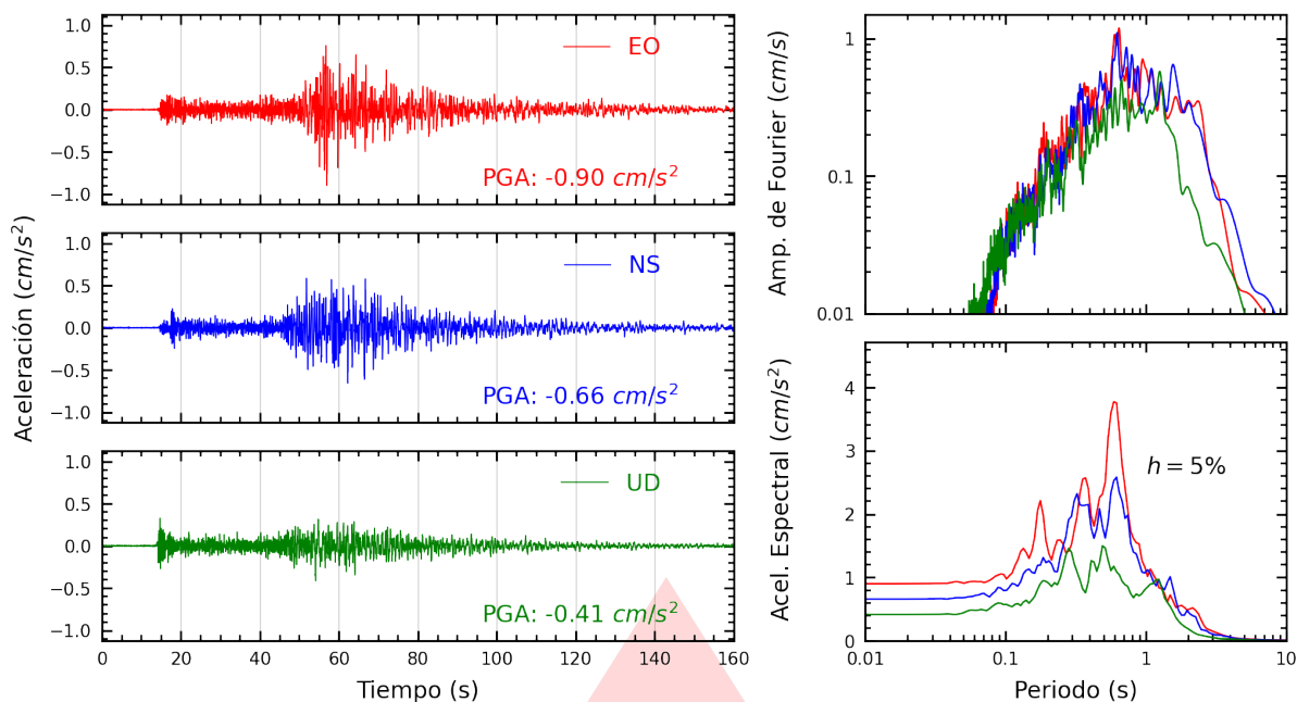
Figura A.37: Registros tiempo-historia, espectros de Fourier y de respuesta en las direcciones EO, NS y vertical de la estación UNC. Sismo de Aucayacu, Leoncio Prado - Huánuco del 2026-08-02, 20:42:22 (Hora local)
