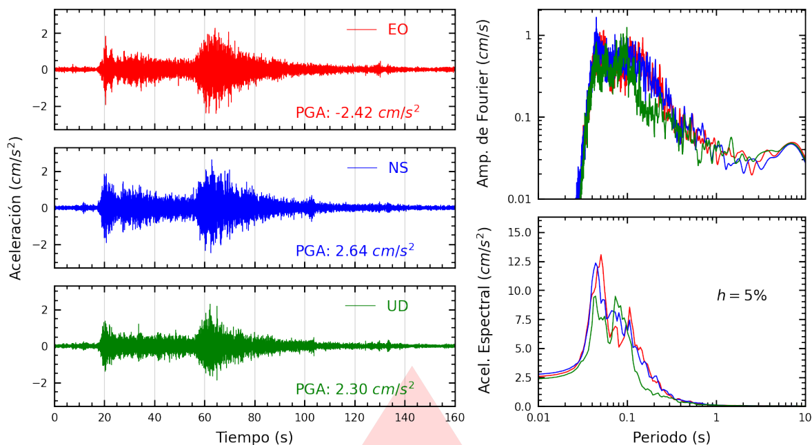
Figura A.7: Registros tiempo-historia, espectros de Fourier y de respuesta en las direcciones EO, NS y vertical de la estación SROSA. Sismo de Aucayacu, Leoncio Prado - Huánuco del 2026-08-02, 20:42:22 (Hora local)
