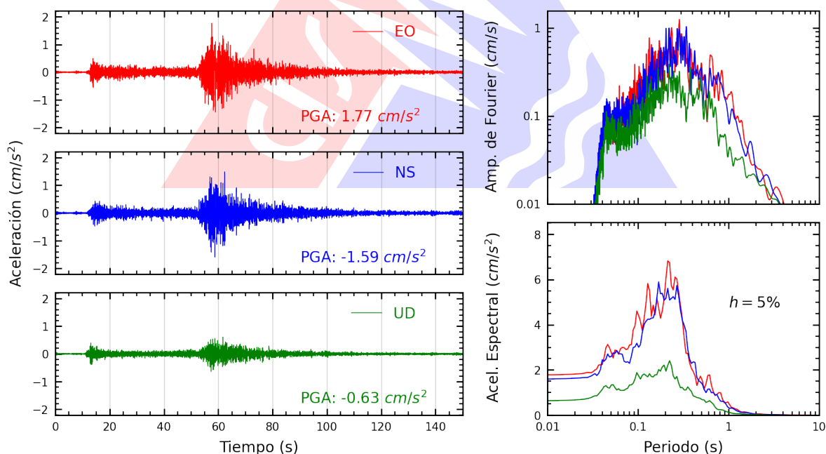
Figura A.16: Registros tiempo-historia, espectros de Fourier y de respuesta en las direcciones EO, NS y vertical de la estación BRIS2. Sismo de Aucayacu, Leoncio Prado - Huánuco del 2026-08-02, 20:42:22 (Hora local)
