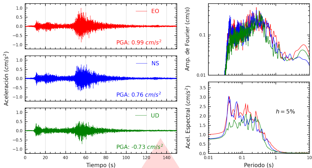
Figura A.33: Registros tiempo-historia, espectros de Fourier y de respuesta en las direcciones EO, NS y vertical de la estación COMAS. Sismo de Aucayacu, Leoncio Prado - Huánuco del 2026-08-02, 20:42:22 (Hora local)
