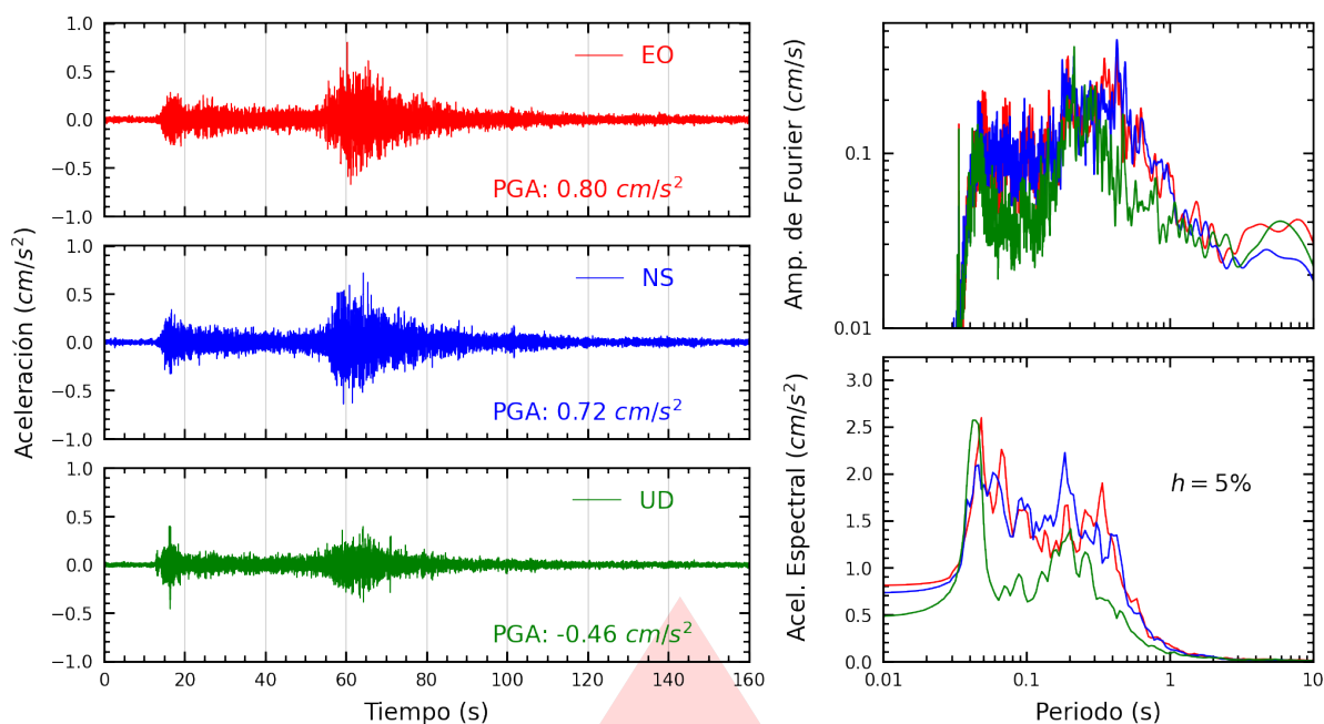
Figura A.39: Registros tiempo-historia, espectros de Fourier y de respuesta en las direcciones EO, NS y vertical de la estación UPCVI. Sismo de Aucayacu, Leoncio Prado - Huánuco del 2026-08-02, 20:42:22 (Hora local)
