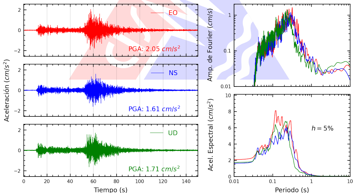
Figura A.10: Registros tiempo-historia, espectros de Fourier y de respuesta en las direcciones EO, NS y vertical de la estación SOVES. Sismo de Aucayacu, Leoncio Prado - Huánuco del 2026-08-02, 20:42:22 (Hora local)
