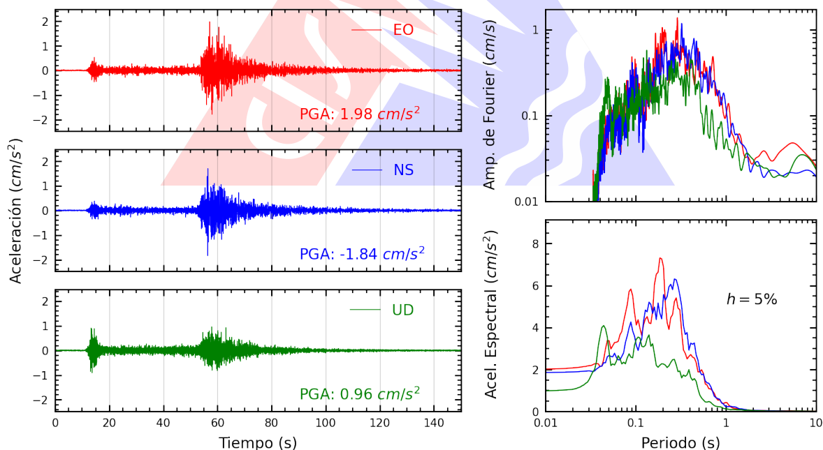
Figura A.12: Registros tiempo-historia, espectros de Fourier y de respuesta en las direcciones EO, NS y vertical de la estación USILP. Sismo de Aucayacu, Leoncio Prado - Huánuco del 2026-08-02, 20:42:22 (Hora local)
