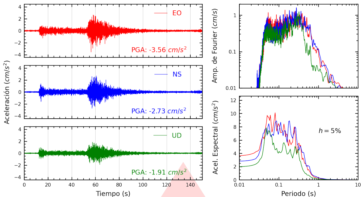
Figura A.5: Registros tiempo-historia, espectros de Fourier y de respuesta en las direcciones EO, NS y vertical de la estación UNTEL. Sismo de Aucayacu, Leoncio Prado - Huánuco del 2026-08-02, 20:42:22 (Hora local)
