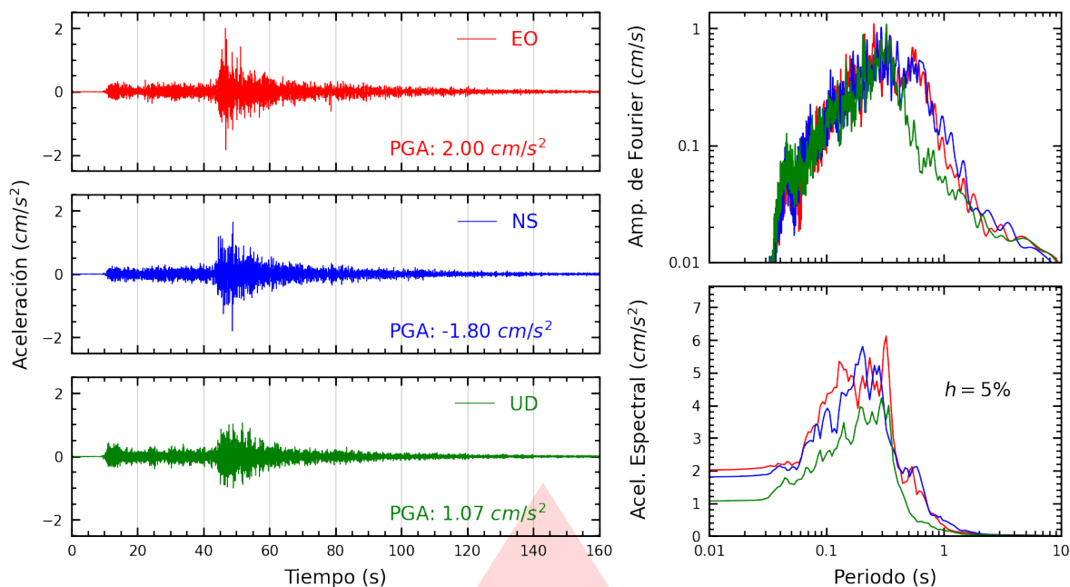
Figura A.11: Registros tiempo-historia, espectros de Fourier y de respuesta en las direcciones EO, NS y vertical de la estación CARAL. Sismo de Aucayacu, Leoncio Prado - Huánuco del 2026-08-02, 20:42:22 (Hora local)
