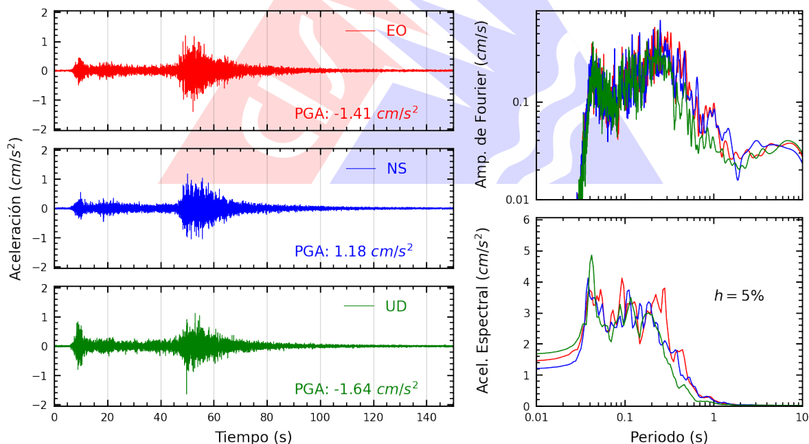
Figura A.20: Registros tiempo-historia, espectros de Fourier y de respuesta en las direcciones EO, NS y vertical de la estación USMP. Sismo de Aucayacu, Leoncio Prado - Huánuco del 2026-08-02, 20:42:22 (Hora local)
