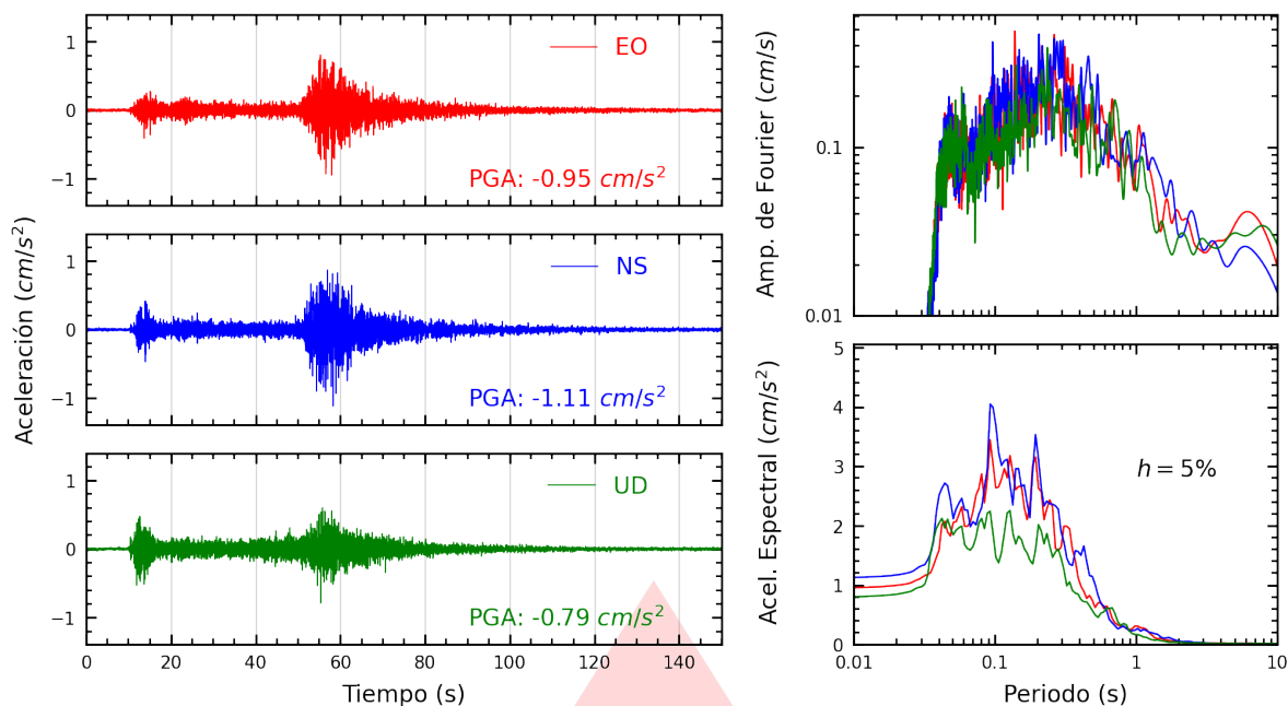
Figura A.29: Registros tiempo-historia, espectros de Fourier y de respuesta en las direcciones EO, NS y vertical de la estación SERVI. Sismo de Aucayacu, Leoncio Prado - Huánuco del 2026-08-02, 20:42:22 (Hora local)
