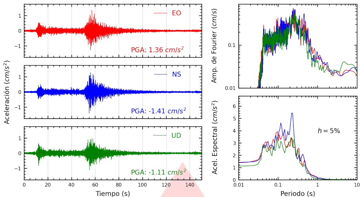
Figura A.23: Registros tiempo-historia, espectros de Fourier y de respuesta en las direcciones EO, NS y vertical de la estación URPE. Sismo de Aucayacu, Leoncio Prado - Huánuco del 2026-08-02, 20:42:22 (Hora local)
