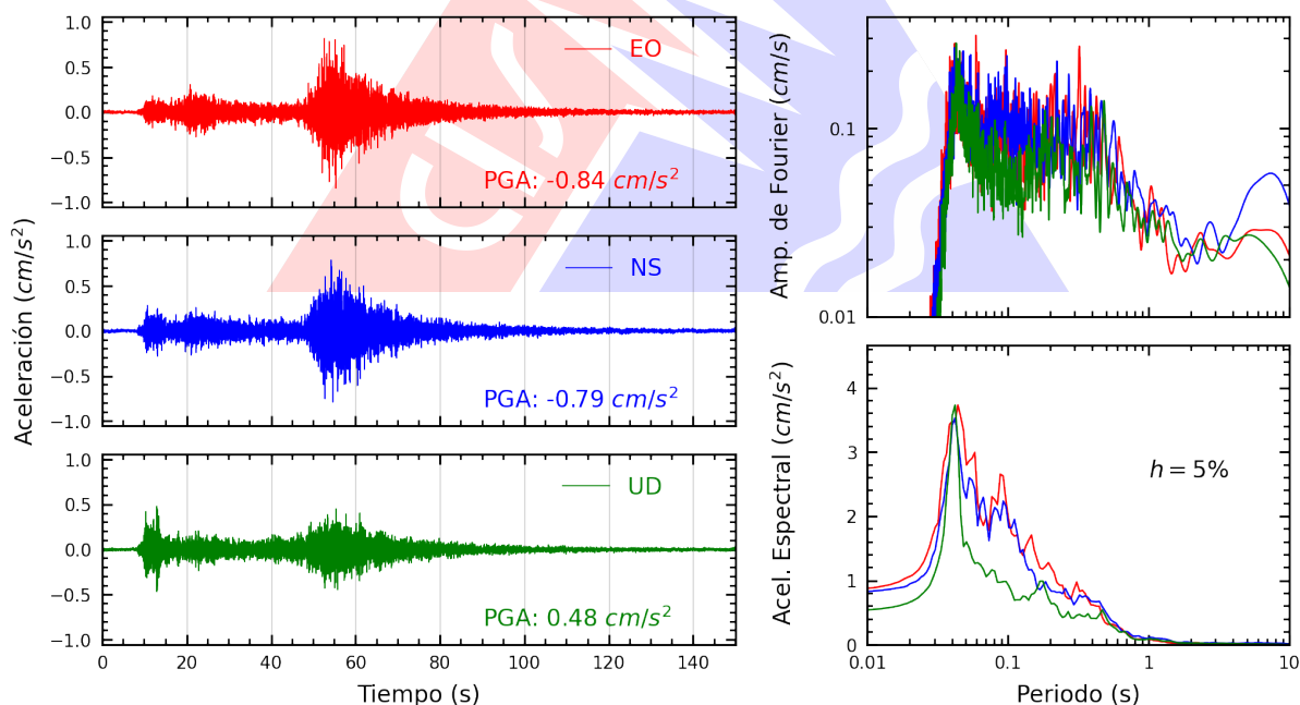
Figura A.38: Registros tiempo-historia, espectros de Fourier y de respuesta en las direcciones EO, NS y vertical de la estación SJLCE. Sismo de Aucayacu, Leoncio Prado - Huánuco del 2026-08-02, 20:42:22 (Hora local)
