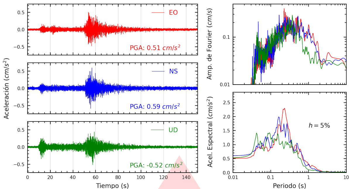
Figura A.43: Registros tiempo-historia, espectros de Fourier y de respuesta en las direcciones EO, NS y vertical de la estación BONDY. Sismo de Aucayacu, Leoncio Prado - Huánuco del 2026-08-02, 20:42:22 (Hora local)
