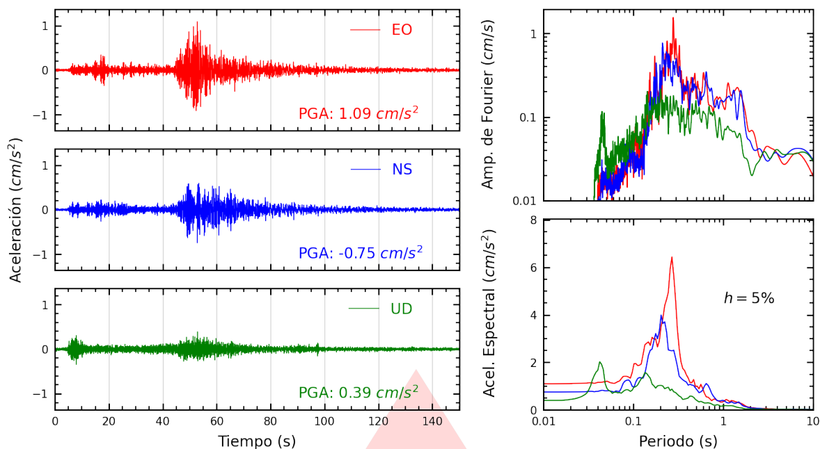
Figura A.31: Registros tiempo-historia, espectros de Fourier y de respuesta en las direcciones EO, NS y vertical de la estación DSML. Sismo de Aucayacu, Leoncio Prado - Huánuco del 2026-08-02, 20:42:22 (Hora local)
