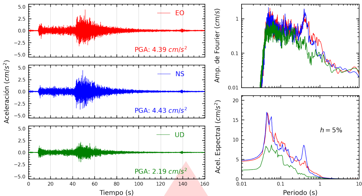
Figura A.3: Registros tiempo-historia, espectros de Fourier y de respuesta en las direcciones EO, NS y vertical de la estación USP. Sismo de Aucayacu, Leoncio Prado - Huánuco del 2026-08-02, 20:42:22 (Hora local)
