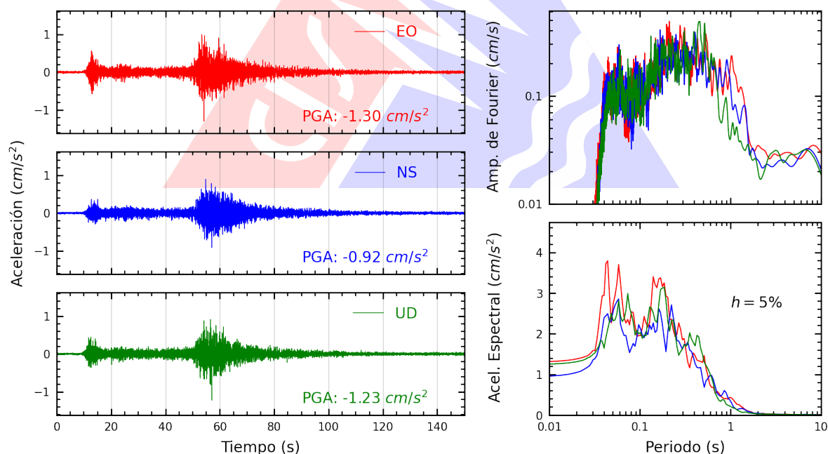
Figura A.26: Registros tiempo-historia, espectros de Fourier y de respuesta en las direcciones EO, NS y vertical de la estación IMCA. Sismo de Aucayacu, Leoncio Prado - Huánuco del 2026-08-02, 20:42:22 (Hora local)
