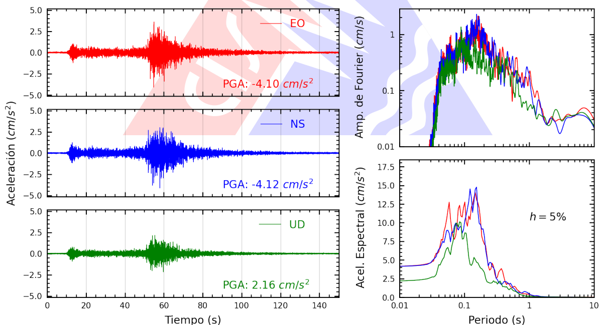
Figura A.4: Registros tiempo-historia, espectros de Fourier y de respuesta en las direcciones EO, NS y vertical de la estación USILM. Sismo de Aucayacu, Leoncio Prado - Huánuco del 2026-08-02, 20:42:22 (Hora local)
