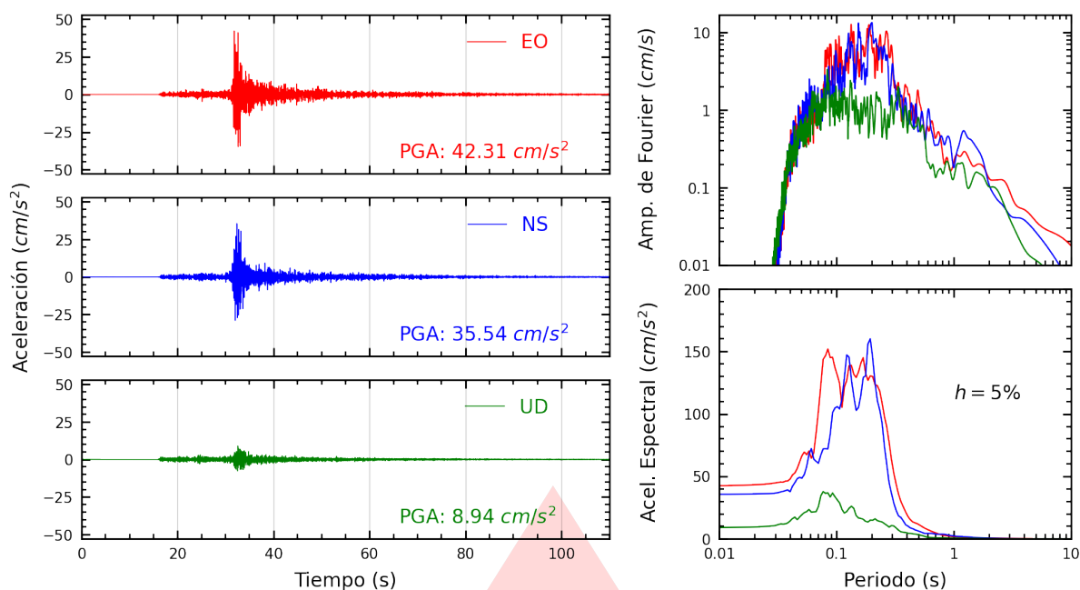
Figura A.1: Registros tiempo-historia, espectros de Fourier y de respuesta en las direcciones EO, NS y vertical de la estación UNAS. Sismo de Aucayacu, Leoncio Prado - Huánuco del 2026-08-02, 20:42:22 (Hora local)
