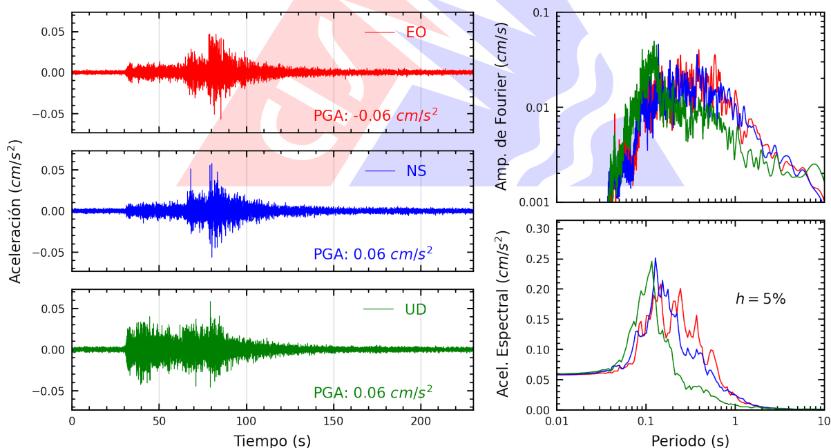
Figura A.2: Registros tiempo-historia, espectros de Fourier y de respuesta en las direcciones EO, NS y vertical de la estación UNIA. Sismo de Saposoa, Huallaga - San Martín del 2026-08-04, 22:40:45 (Hora local)
