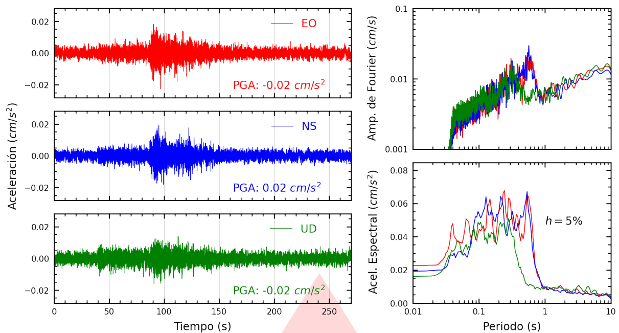
Figura A.3: Registros tiempo-historia, espectros de Fourier y de respuesta en las direcciones EO, NS y vertical de la estación CARAL. Sismo de Saposoa, Hualлага - San Martín del 2026-08-04, 22:40:45 (Hora local)
