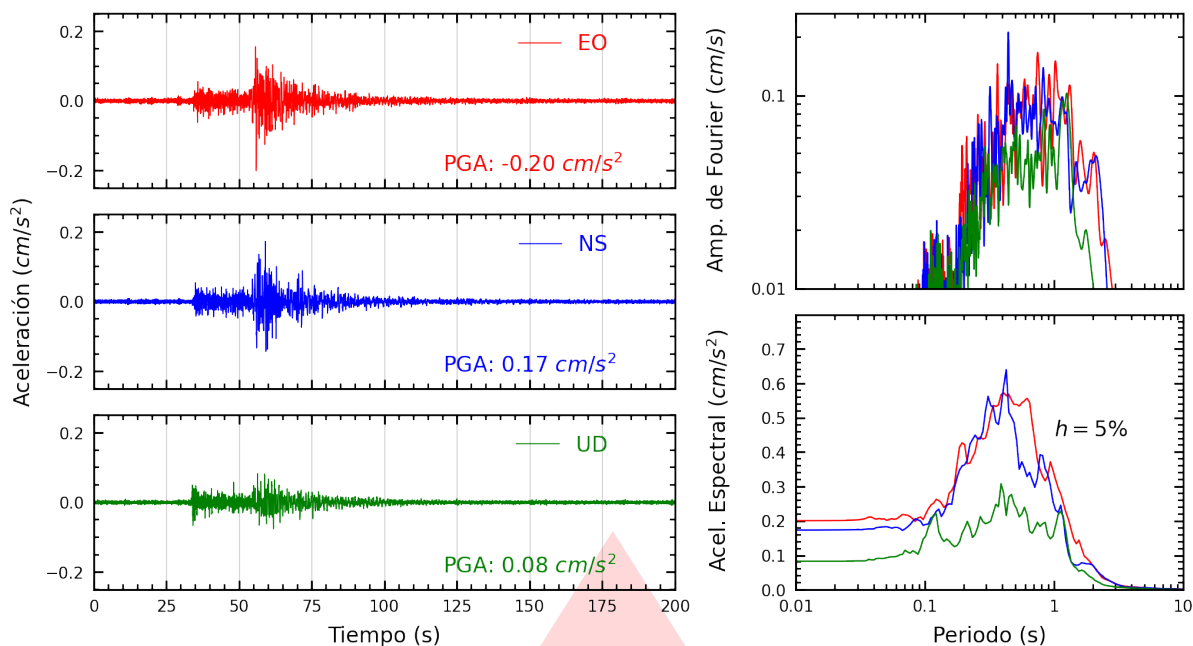
Figura A.1: Registros tiempo-historia, espectros de Fourier y de respuesta en las direcciones EO, NS y vertical de la estación UNC. Sismo de Saposoa, Huallaga - San Martín del 2026-08-04, 22:40:45 (Hora local)
