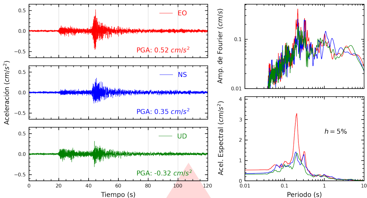
Figura A.17: Registros tiempo-historia, espectros de Fourier y de respuesta en las direcciones EO, NS y vertical de la estación SERVI. Sismo de Chupaca, Chupaca - Junín del 2026-08-06, 13:57:18 (Hora local)
