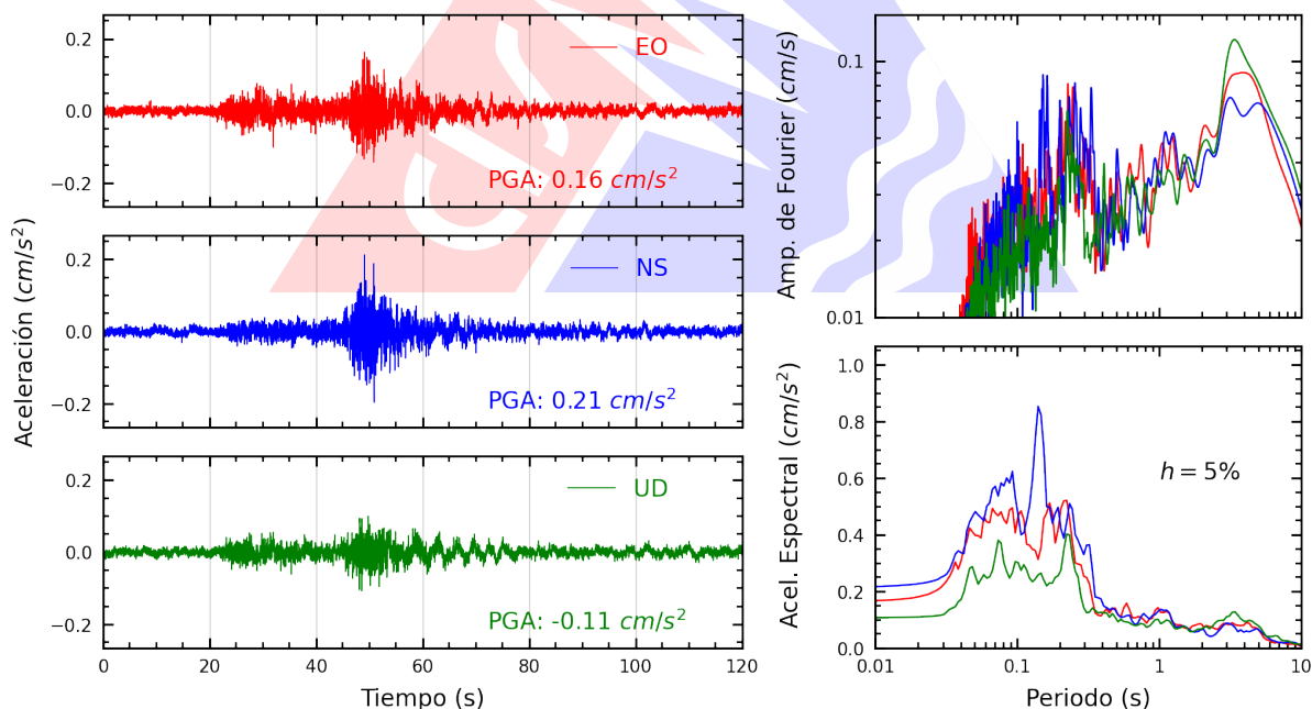
Figura A.32: Registros tiempo-historia, espectros de Fourier y de respuesta en las direcciones EO, NS y vertical de la estación UCSS. Sismo de Chupaca, Chupaca - Junín del 2026-08-06, 13:57:18 (Hora local)
