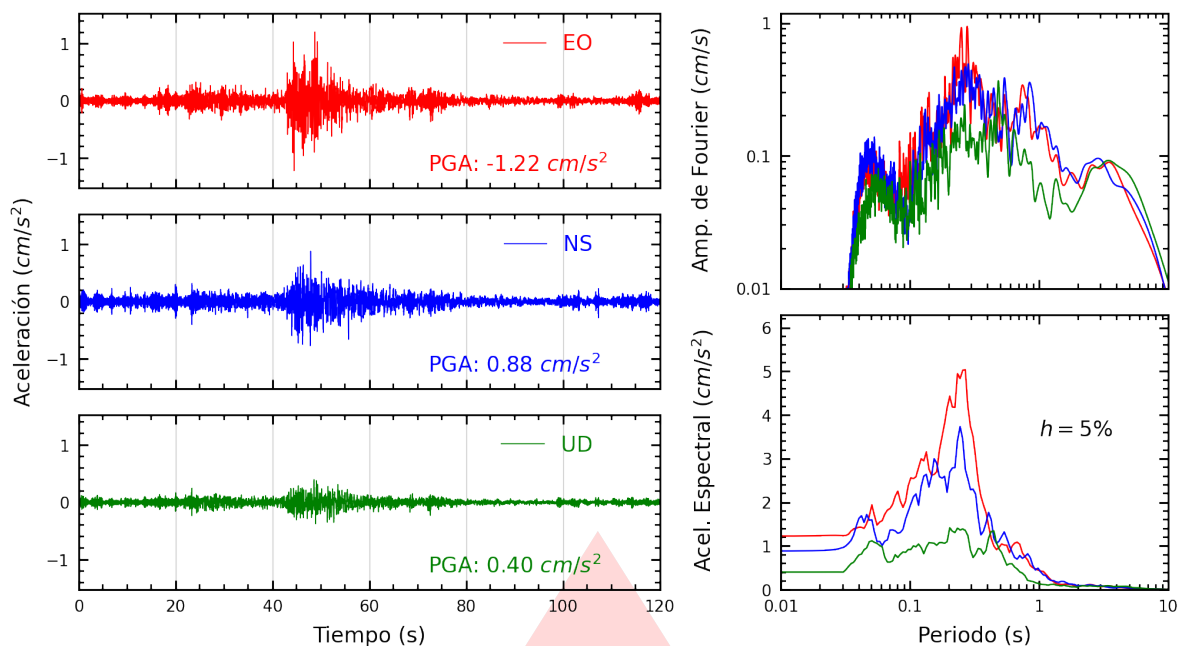
Figura A.5: Registros tiempo-historia, espectros de Fourier y de respuesta en las direcciones EO, NS y vertical de la estación BRIS2. Sismo de Chupaca, Chupaca - Junín del 2026-08-06, 13:57:18 (Hora local)
