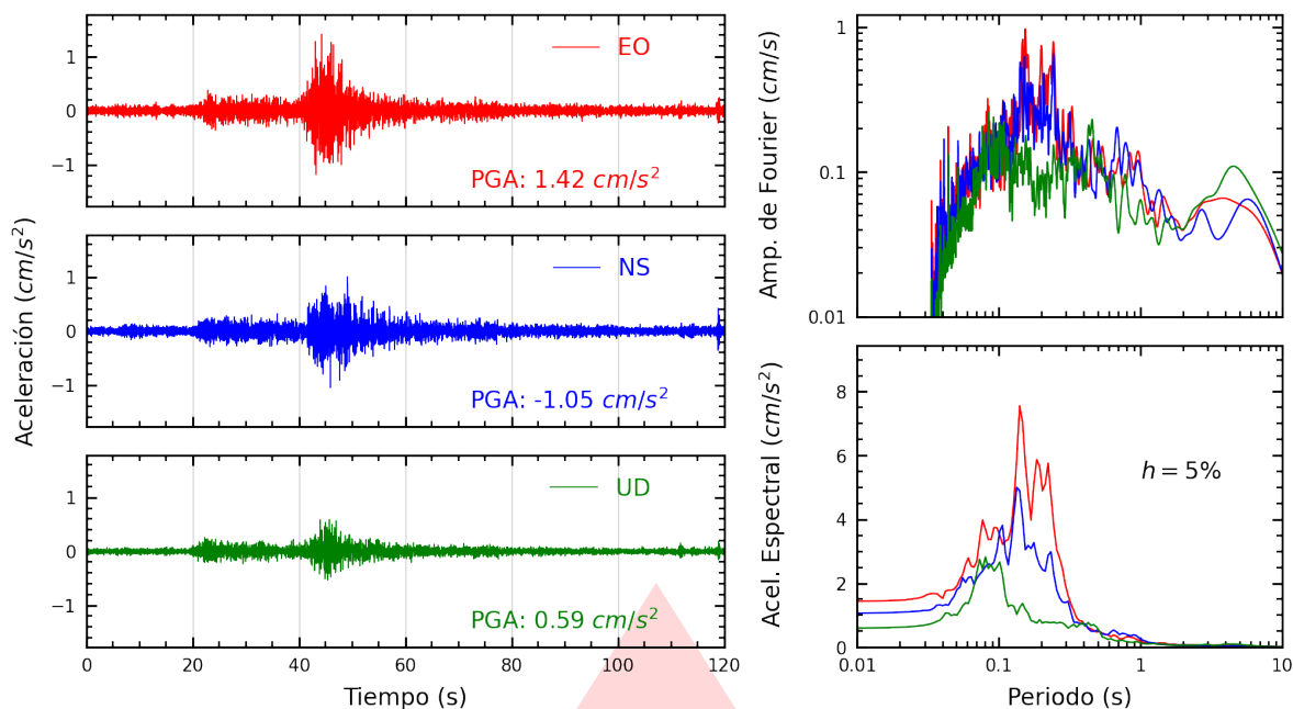
Figura A.3: Registros tiempo-historia, espectros de Fourier y de respuesta en las direcciones EO, NS y vertical de la estación USILM. Sismo de Chupaca, Chupaca - Junín del 2026-08-06, 13:57:18 (Hora local)
