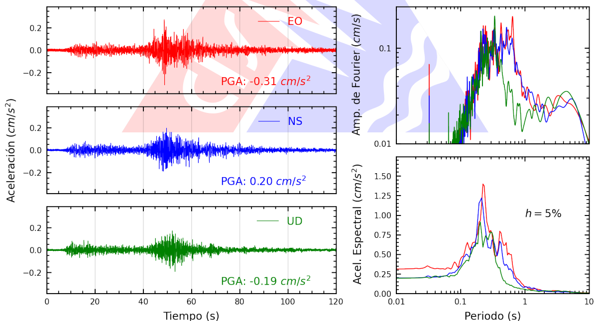
Figura A.30: Registros tiempo-historia, espectros de Fourier y de respuesta en las direcciones EO, NS y vertical de la estación CARAL. Sismo de Chupaca, Chupaca - Junín del 2026-08-06, 13:57:18 (Hora local)
