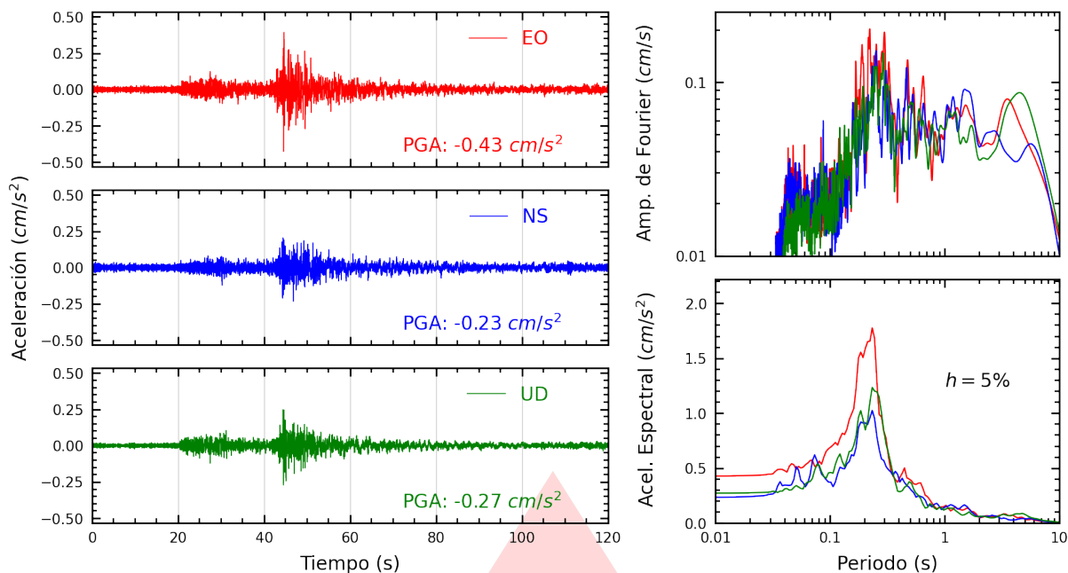
Figura A.21: Registros tiempo-historia, espectros de Fourier y de respuesta en las direcciones EO, NS y vertical de la estación BORJA. Sismo de Chupaca, Chupaca - Junín del 2026-08-06, 13:57:18 (Hora local)
