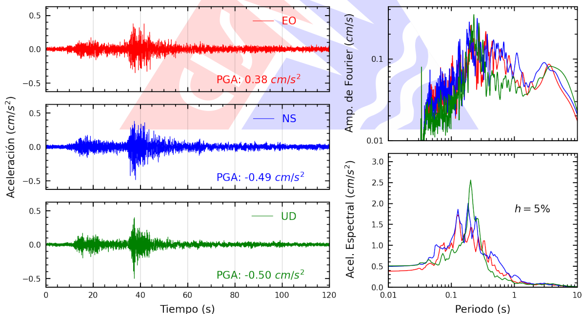
Figura A.18: Registros tiempo-historia, espectros de Fourier y de respuesta en las direcciones EO, NS y vertical de la estación UPCVI. Sismo de Chupaca, Chupaca - Junín del 2026-08-06, 13:57:18 (Hora local)
