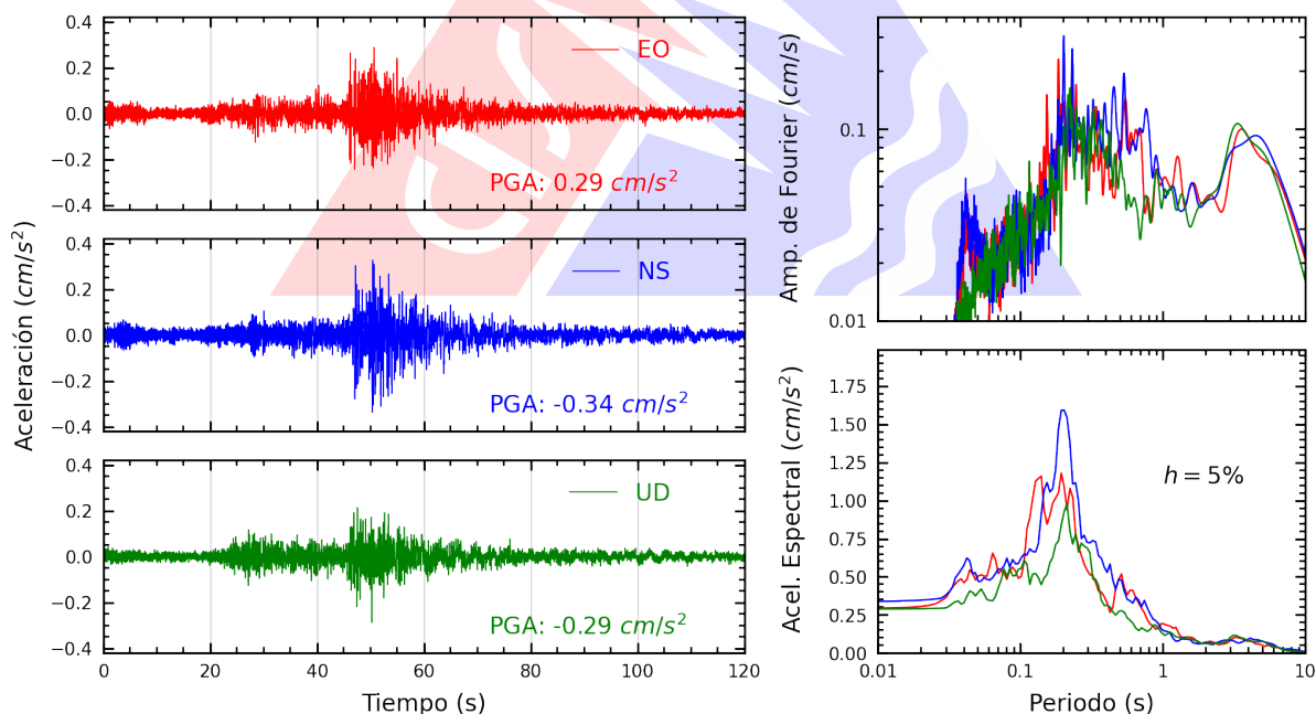
Figura A.28: Registros tiempo-historia, espectros de Fourier y de respuesta en las direcciones EO, NS y vertical de la estación COMAS. Sismo de Chupaca, Chupaca - Junín del 2026-08-06, 13:57:18 (Hora local)
