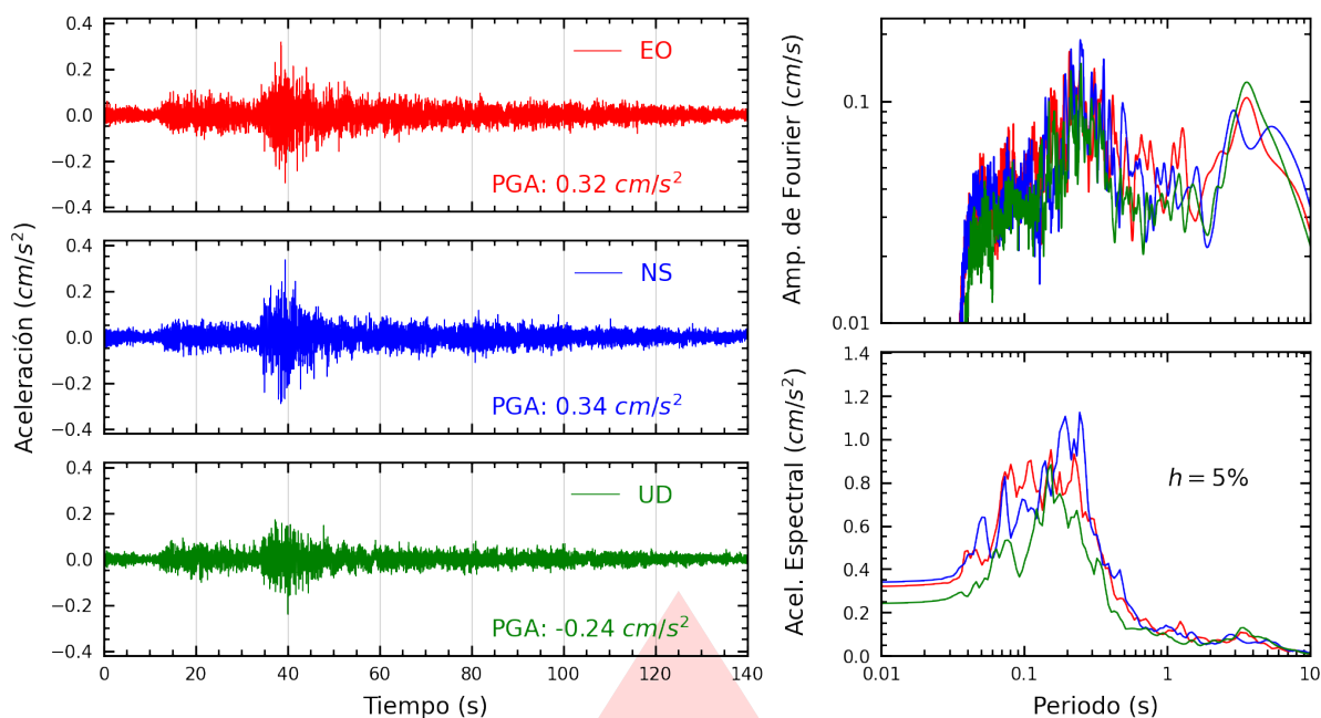
Figura A.29: Registros tiempo-historia, espectros de Fourier y de respuesta en las direcciones EO, NS y vertical de la estación FICPE. Sismo de Chupaca, Chupaca - Junín del 2026-08-06, 13:57:18 (Hora local)
