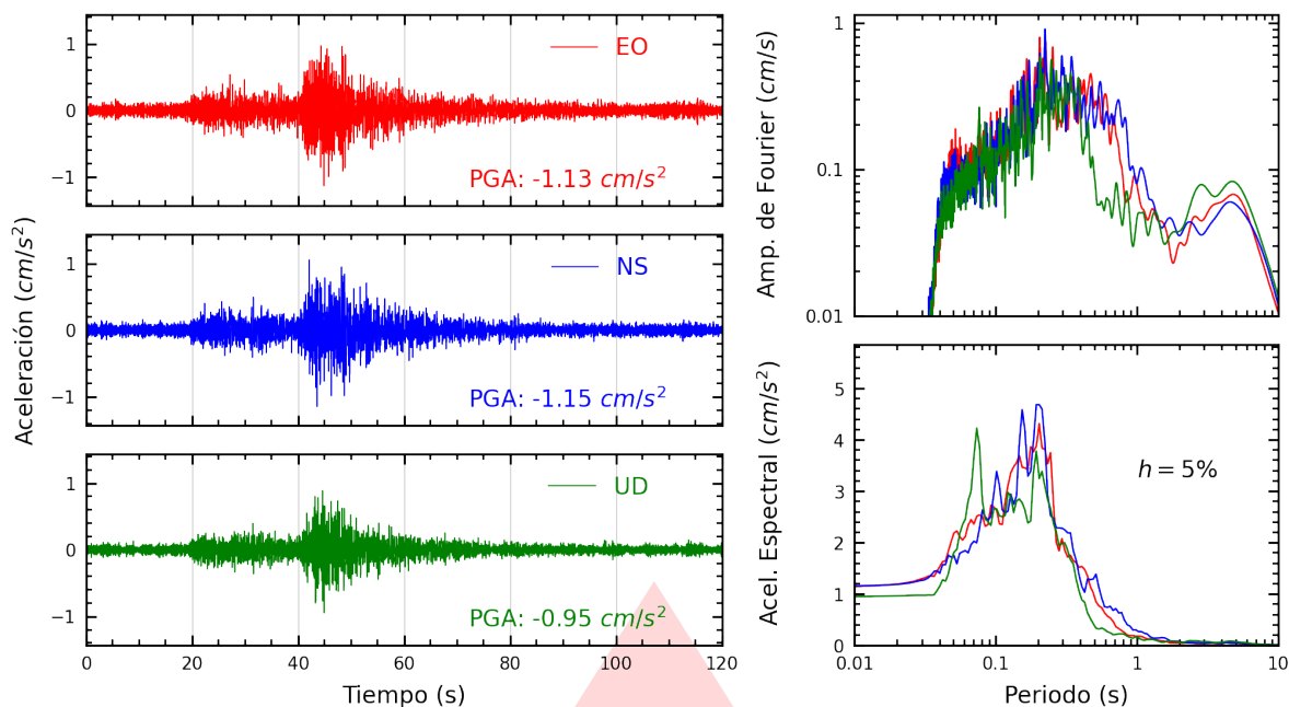
Figura A.7: Registros tiempo-historia, espectros de Fourier y de respuesta en las direcciones EO, NS y vertical de la estación UNTEL. Sismo de Chupaca, Chupaca - Junín del 2026-08-06, 13:57:18 (Hora local)
