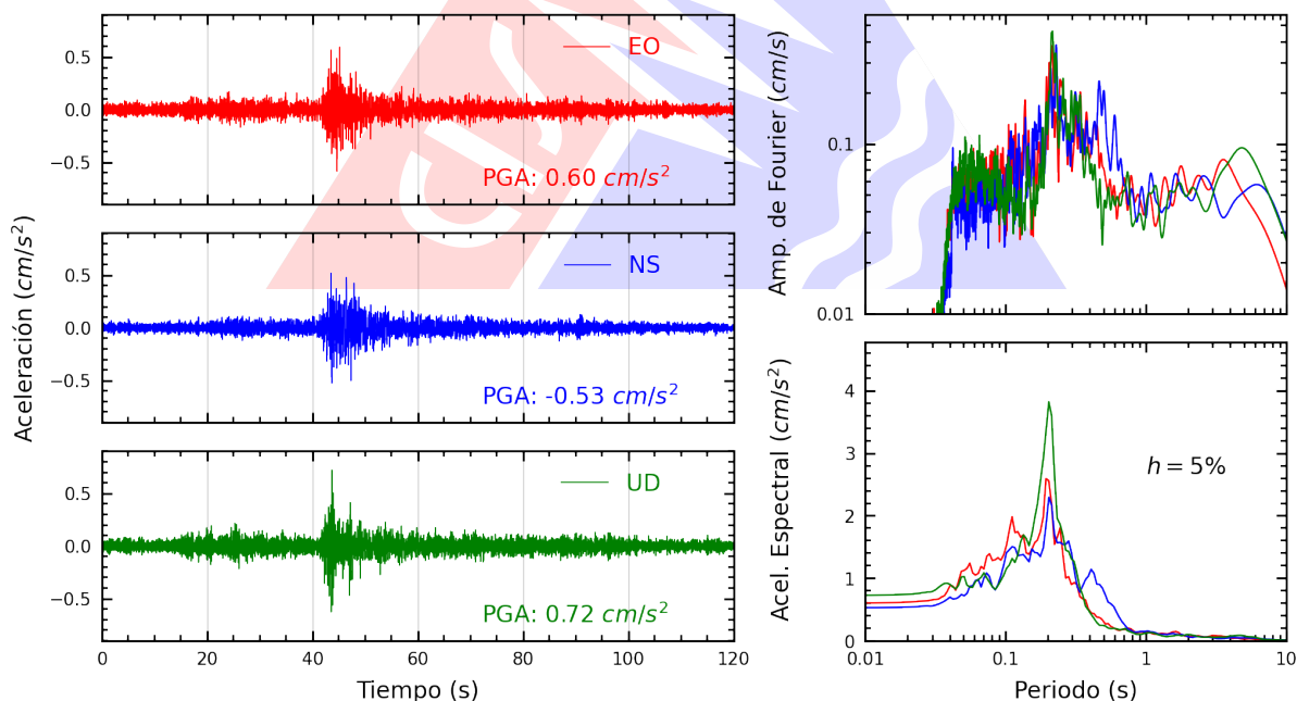
Figura A.14: Registros tiempo-historia, espectros de Fourier y de respuesta en las direcciones EO, NS y vertical de la estación URPE. Sismo de Chupaca, Chupaca - Junín del 2026-08-06, 13:57:18 (Hora local)
