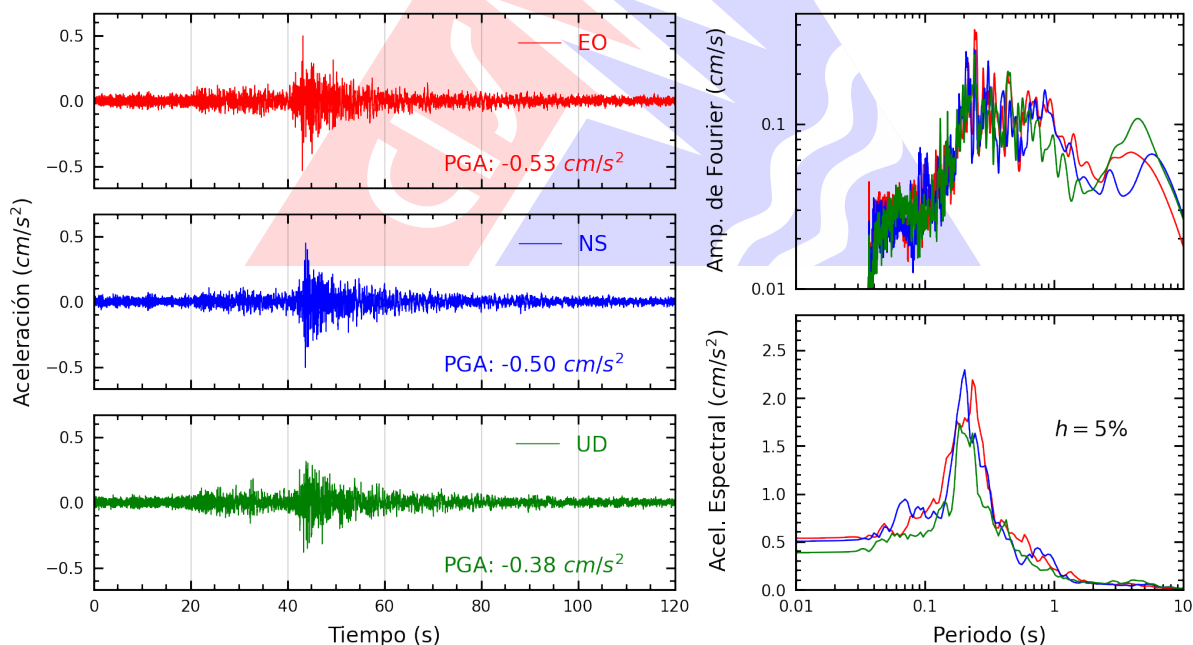
Figura A.16: Registros tiempo-historia, espectros de Fourier y de respuesta en las direcciones EO, NS y vertical de la estación IMCA. Sismo de Chupaca, Chupaca - Junín del 2026-08-06, 13:57:18 (Hora local)
