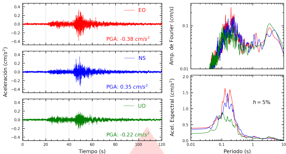
Figura A.27: Registros tiempo-historia, espectros de Fourier y de respuesta en las direcciones EO, NS y vertical de la estación JALVA. Sismo de Chupaca, Chupaca - Junín del 2026-08-06, 13:57:18 (Hora local)
