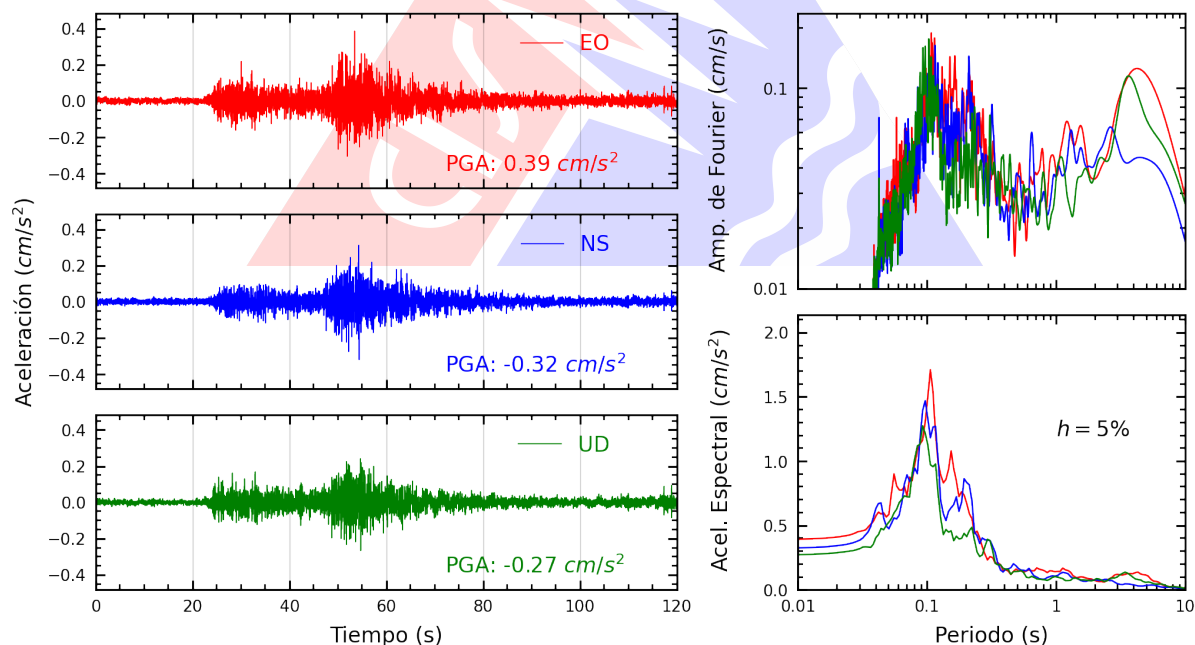
Figura A.26: Registros tiempo-historia, espectros de Fourier y de respuesta en las direcciones EO, NS y vertical de la estación AMORE. Sismo de Chupaca, Chupaca - Junín del 2026-08-06, 13:57:18 (Hora local)
