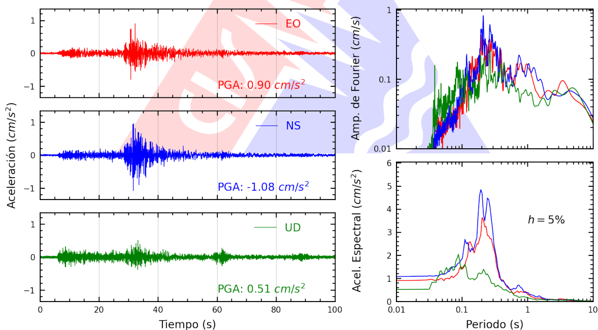
Figura A.8: Registros tiempo-historia, espectros de Fourier y de respuesta en las direcciones EO, NS y vertical de la estación SOCHO. Sismo de Chupaca, Chupaca - Junín del 2026-08-06, 13:57:18 (Hora local)
