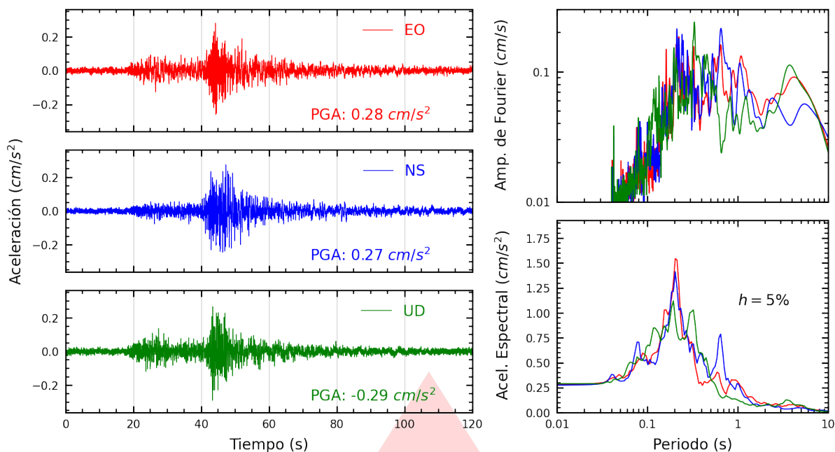
Figura A.31: Registros tiempo-historia, espectros de Fourier y de respuesta en las direcciones EO, NS y vertical de la estación UNMSM. Sismo de Chupaca, Chupaca - Junín del 2026-08-06, 13:57:18 (Hora local)
