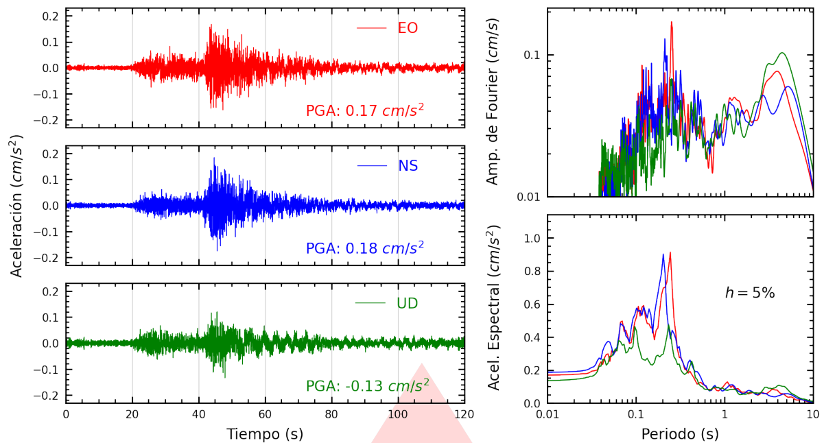
Figura A.33: Registros tiempo-historia, espectros de Fourier y de respuesta en las direcciones EO, NS y vertical de la estación ATARJ. Sismo de Chupaca, Chupaca - Junín del 2026-08-06, 13:57:18 (Hora local)
