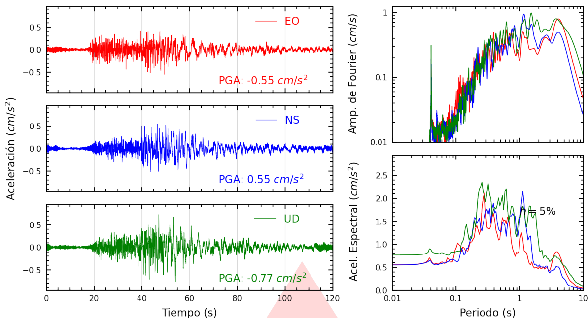
Figura A.13: Registros tiempo-historia, espectros de Fourier y de respuesta en las direcciones EO, NS y vertical de la estación UNSCH. Sismo de Chupaca, Chupaca - Junín del 2026-08-06, 13:57:18 (Hora local)
