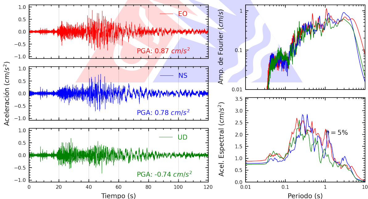
Figura A.12: Registros tiempo-historia, espectros de Fourier y de respuesta en las direcciones EO, NS y vertical de la estación SCAYA. Sismo de Chupaca, Chupaca - Junín del 2026-08-06, 13:57:18 (Hora local)
