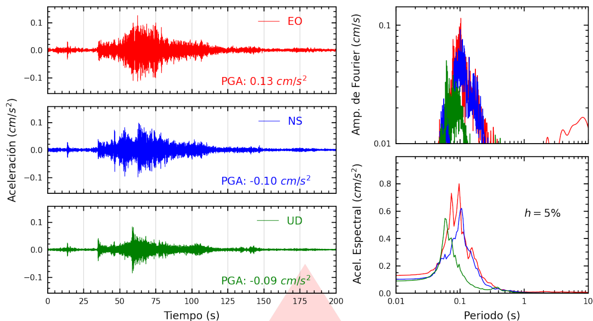
Figura A.1: Registros tiempo-historia, espectros de Fourier y de respuesta en las direcciones EO, NS y vertical de la estación UNAS. Sismo de Contamana, Ucayali - Loreto del 2026-08-07, 00:01:47 (Hora local)
