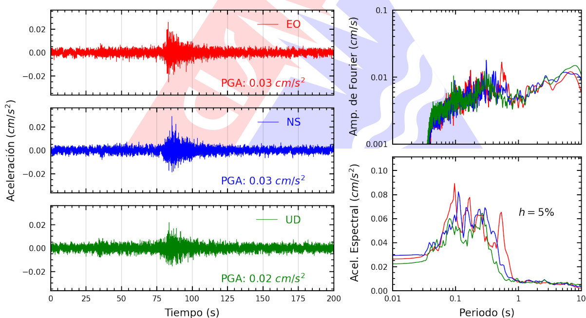
Figura A.2: Registros tiempo-historia, espectros de Fourier y de respuesta en las direcciones EO, NS y vertical de la estación CARAL. Sismo de Contamana, Ucayali - Loreto del 2026-08-07, 00:01:47 (Hora local)
