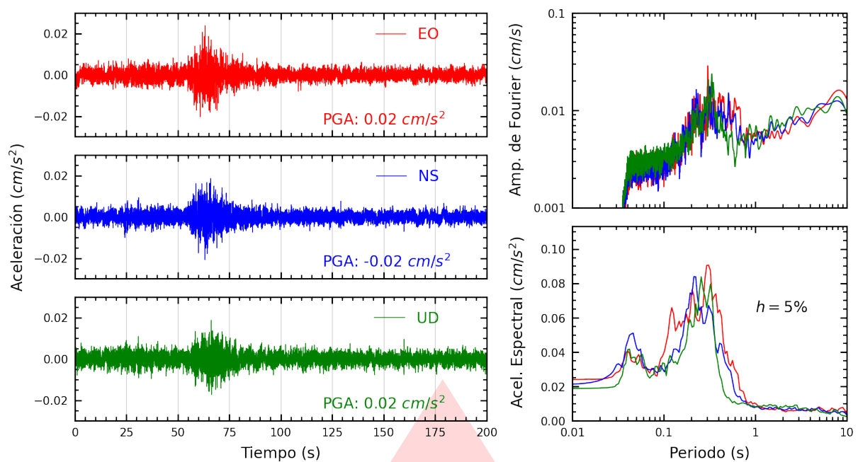
Figura A.1: Registros tiempo-historia, espectros de Fourier y de respuesta en las direcciones EO, NS y vertical de la estación CARAL. Sismo de Huasicancha, Huancayo - Junín del 2026-08-07, 07:10:33 (Hora local)
