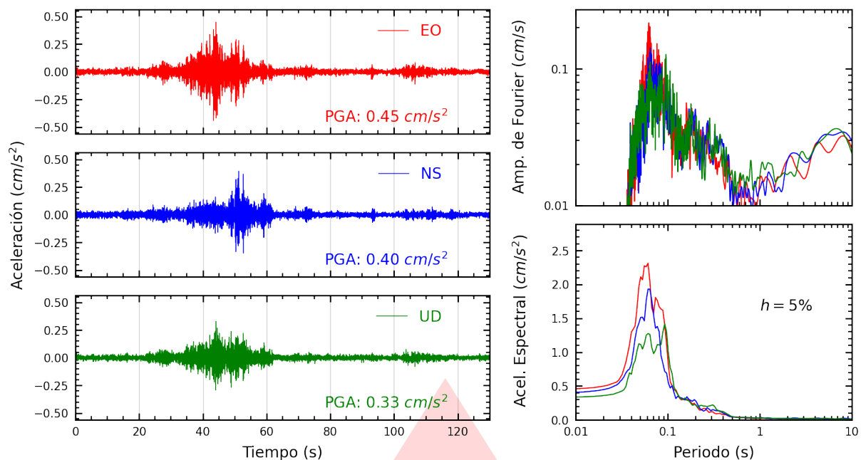
Figura A.1: Registros tiempo-historia, espectros de Fourier y de respuesta en las direcciones EO, NS y vertical de la estación UNTRM. Sismo de Andoas, Datem del Marañón - Loreto del 2026-08-07, 08:27:32 (Hora local)
