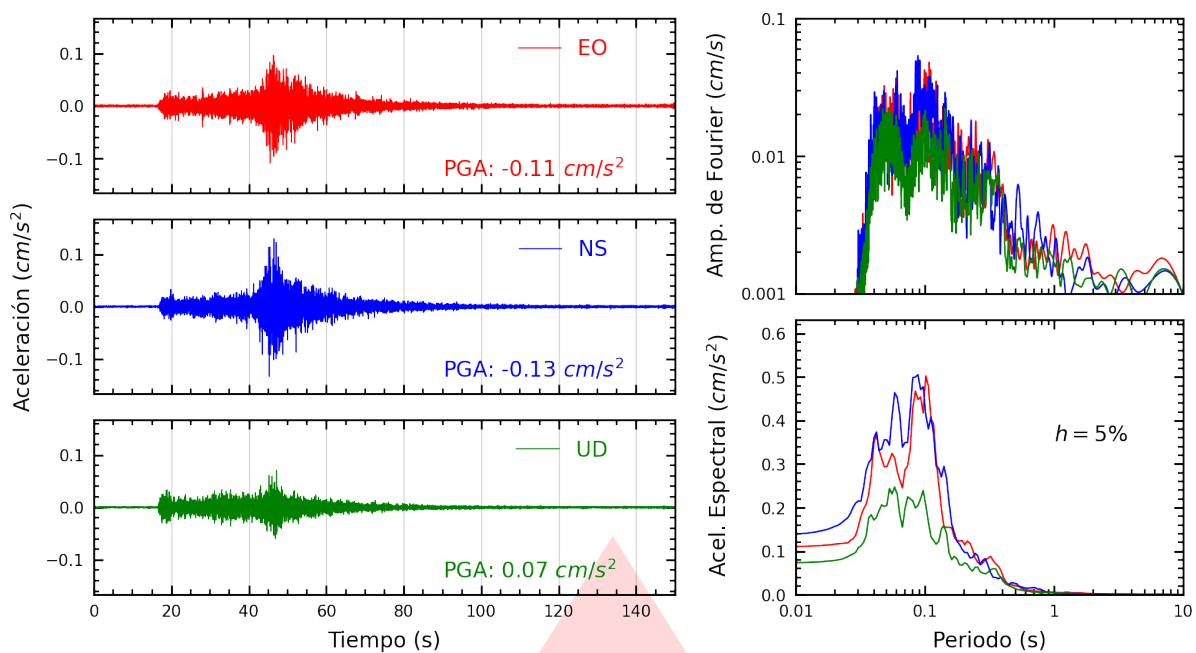
Figura A.1: Registros tiempo-historia, espectros de Fourier y de respuesta en las direcciones EO, NS y vertical de la estación UNSA2. Sismo de Tuti, Caylloma - Arequipa del 2026-08-07, 09:47:13 (Hora local)
