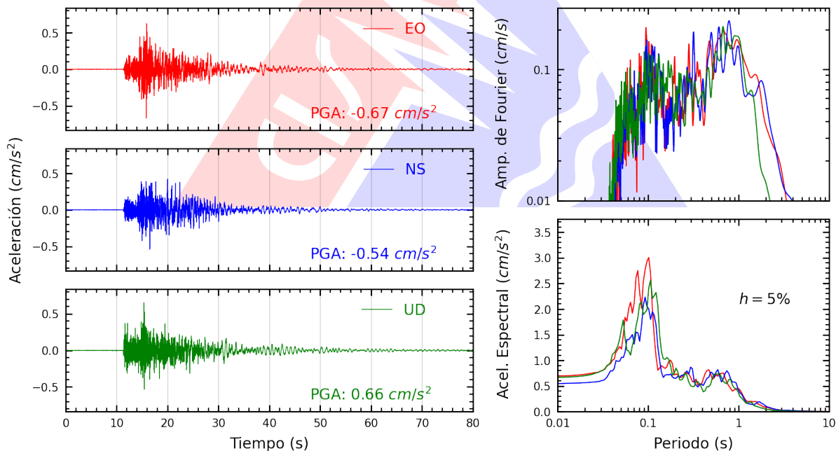
Figura A.2: Registros tiempo-historia, espectros de Fourier y de respuesta en las direcciones EO, NS y vertical de la estación UNCP. Sismo de Chupaca, Chupaca - Junín del 2026-08-07, 19:06:33 (Hora local)
