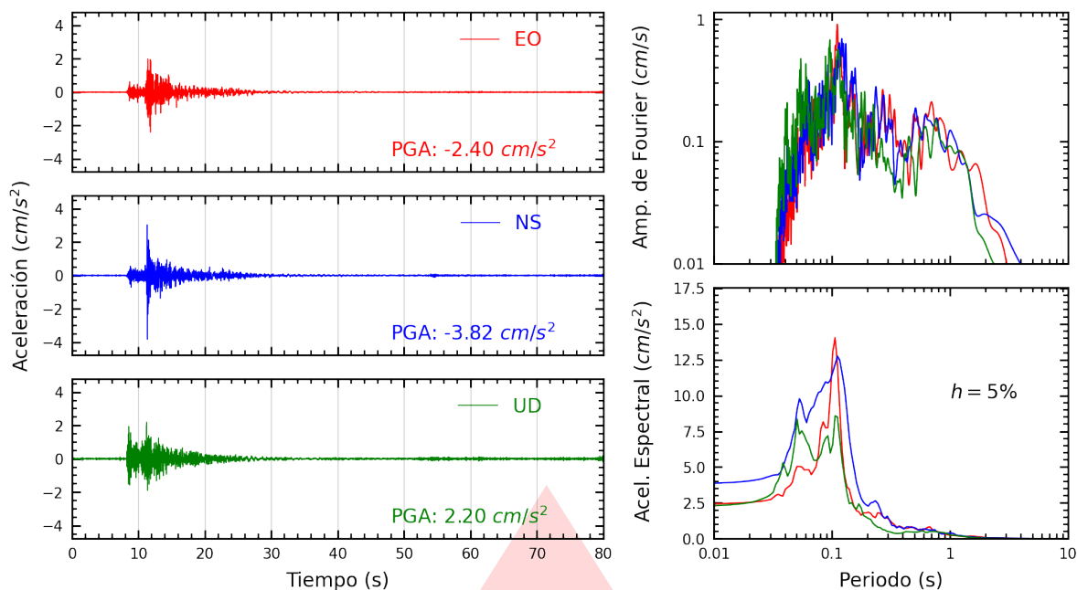
Figura A.1: Registros tiempo-historia, espectros de Fourier y de respuesta en las direcciones EO, NS y vertical de la estación SCHYO. Sismo de Chupaca, Chupaca - Junín del 2026-08-07, 19:06:33 (Hora local)
