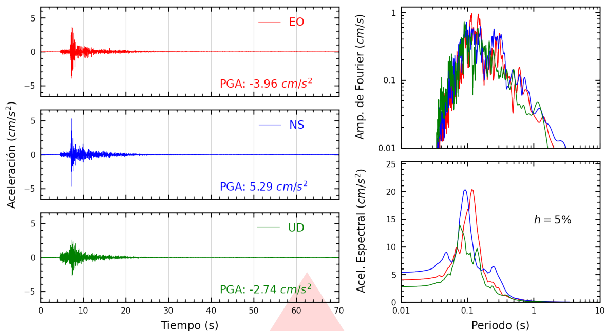
Figura A.1: Registros tiempo-historia, espectros de Fourier y de respuesta en las direcciones EO, NS y vertical de la estación SCHYO. Sismo de Chupaca, Chupaca - Junín del 2026-08-09, 03:26:40 (Hora local)
