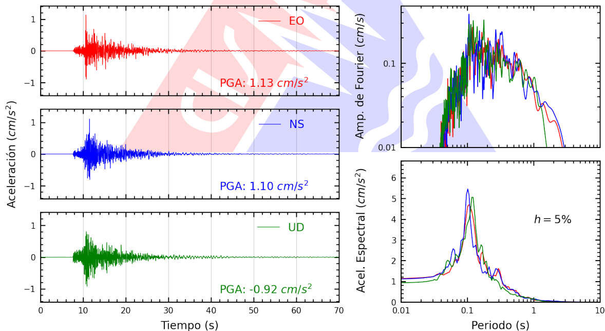
Figura A.2: Registros tiempo-historia, espectros de Fourier y de respuesta en las direcciones EO, NS y vertical de la estación UNCP. Sismo de Chupaca, Chupaca - Junín del 2026-08-09, 03:26:40 (Hora local)
