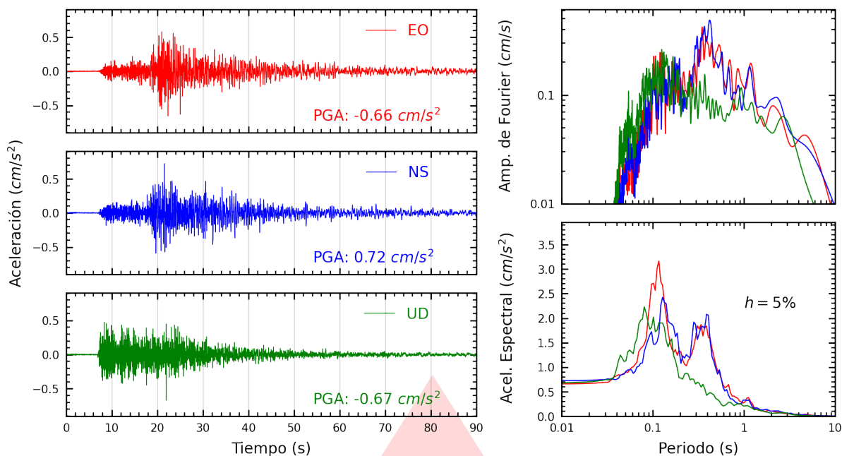
Figura A.1: Registros tiempo-historia, espectros de Fourier y de respuesta en las direcciones EO, NS y vertical de la estación SCPIU. Sismo de Sechura, Sechura - Piura del 2026-08-11, 03:00:28 (Hora local)
