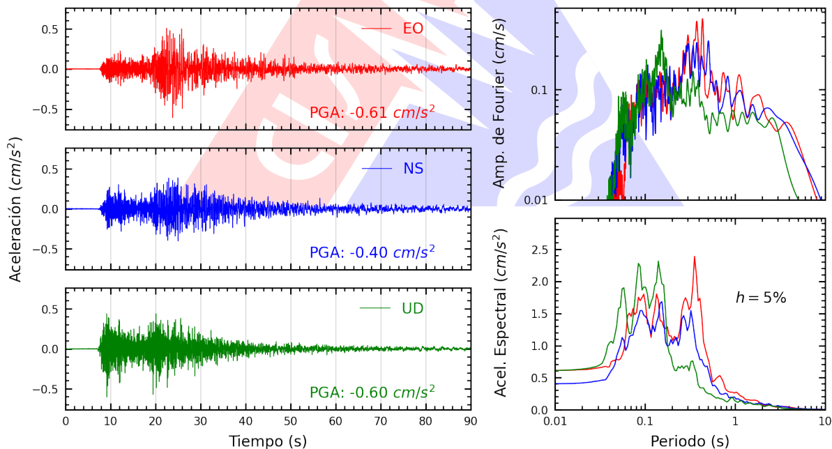
Figura A.2: Registros tiempo-historia, espectros de Fourier y de respuesta en las direcciones EO, NS y vertical de la estación UPAOP. Sismo de Sechura, Sechura - Piura del 2026-08-11, 03:00:28 (Hora local)
