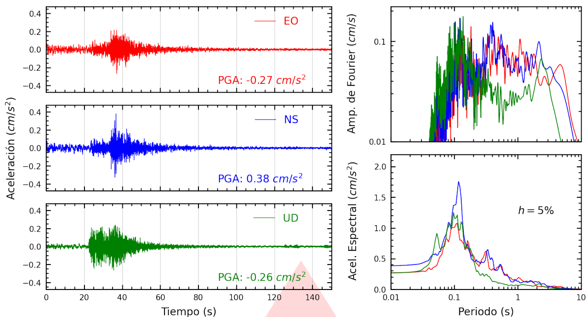
Figura A.1: Registros tiempo-historia, espectros de Fourier y de respuesta en las direcciones EO, NS y vertical de la estación SCPIU. Sismo de Sechura, Sechura - Piura del 2026-08-11, 03:02:05 (Hora local)
