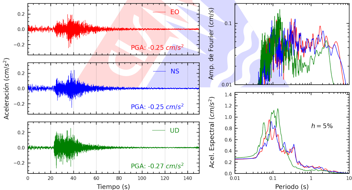
Figura A.2: Registros tiempo-historia, espectros de Fourier y de respuesta en las direcciones EO, NS y vertical de la estación UPAOP. Sismo de Sechura, Sechura - Piura del 2026-08-11, 03:02:05 (Hora local)
