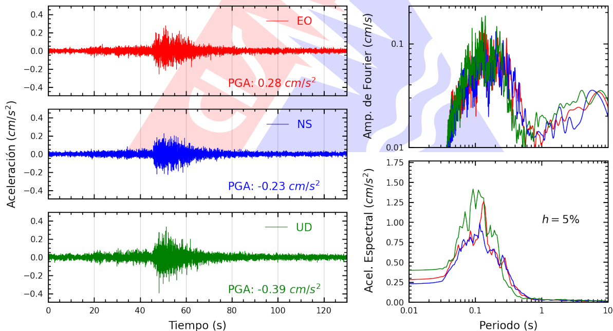
Figura A.8: Registros tiempo-historia, espectros de Fourier y de respuesta en las direcciones EO, NS y vertical de la estación SOVES. Sismo de Panao, Pachitea - Huánuco del 2026-08-11, 23:06:55 (Hora local)
