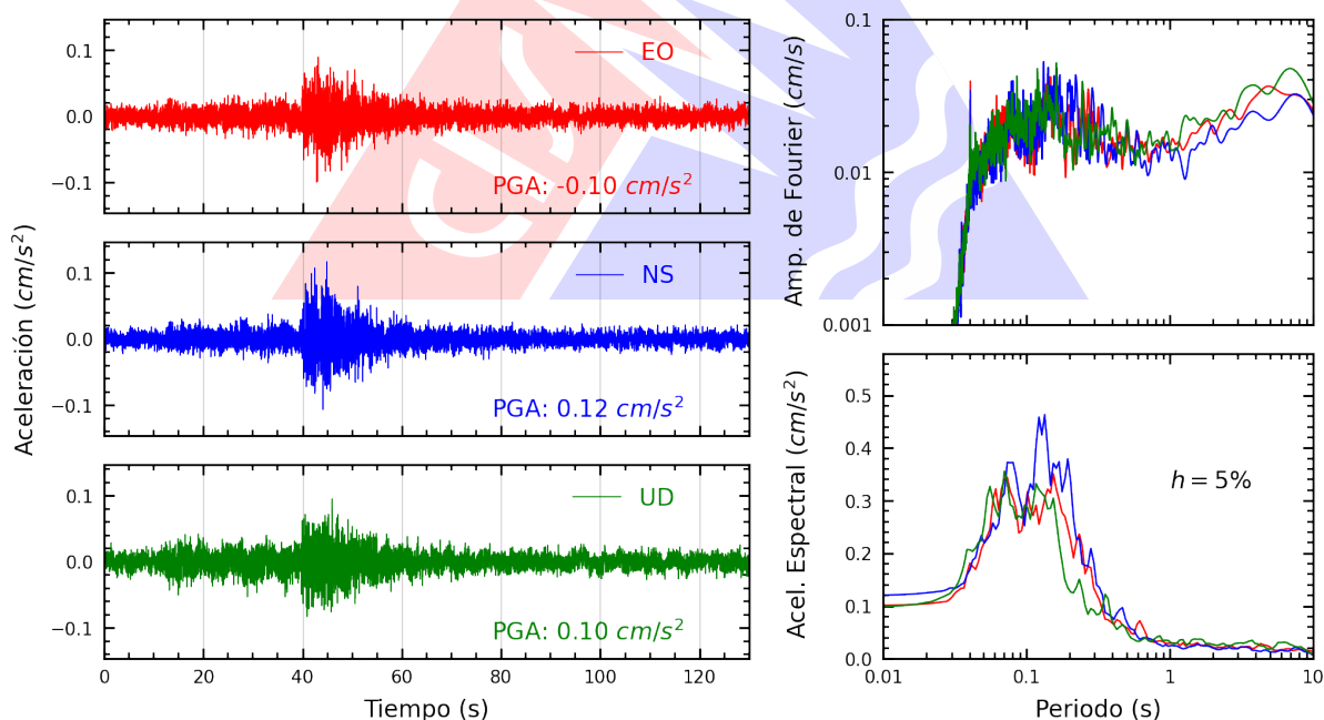
Figura A.20: Registros tiempo-historia, espectros de Fourier y de respuesta en las direcciones EO, NS y vertical de la estación UNMSM. Sismo de Panao, Pachitea - Huánuco del 2026-08-11, 23:06:55 (Hora local)
