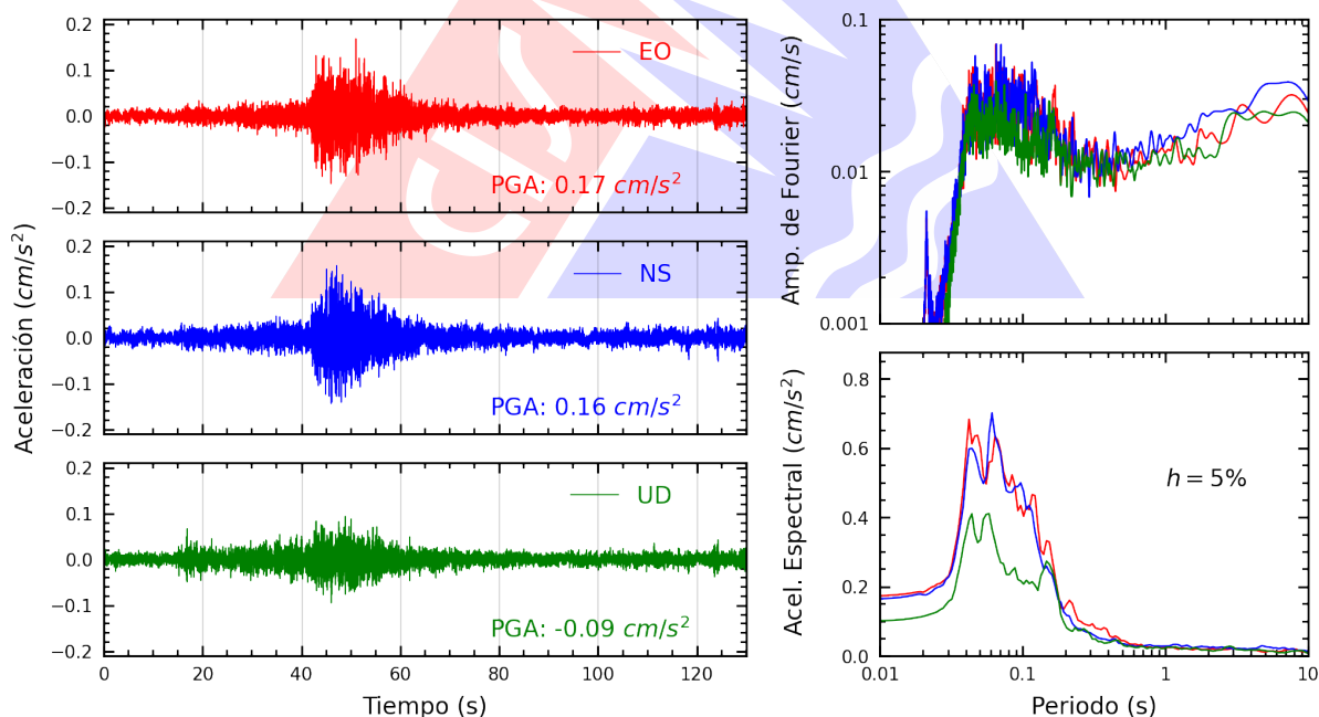
Figura A.18: Registros tiempo-historia, espectros de Fourier y de respuesta en las direcciones EO, NS y vertical de la estación SJLCE. Sismo de Panao, Pachitea - Huánuco del 2026-08-11, 23:06:55 (Hora local)
