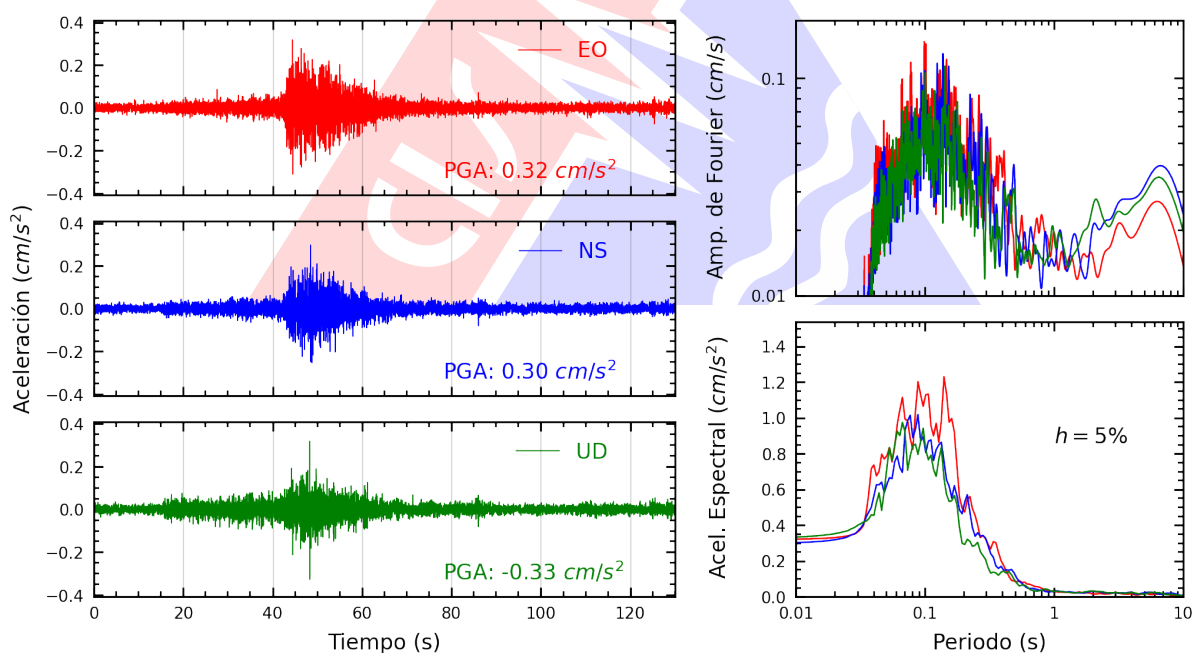
Figura A.10: Registros tiempo-historia, espectros de Fourier y de respuesta en las direcciones EO, NS y vertical de la estación UCVAT. Sismo de Panao, Pachitea - Huánuco del 2026-08-11, 23:06:55 (Hora local)
