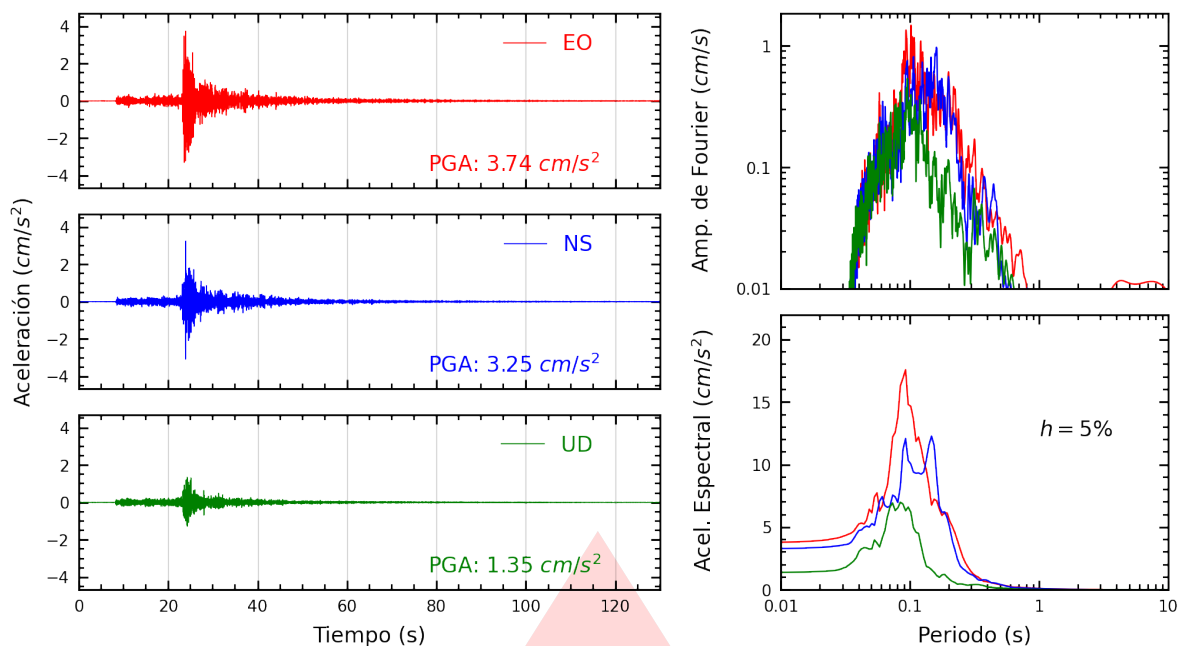
Figura A.1: Registros tiempo-historia, espectros de Fourier y de respuesta en las direcciones EO, NS y vertical de la estación UNAS. Sismo de Panao, Pachitea - Huánuco del 2026-08-11, 23:06:55 (Hora local)
