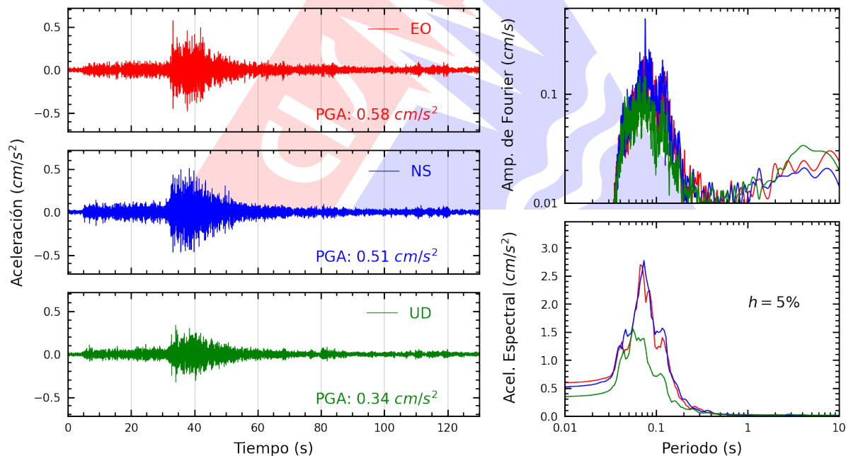
Figura A.4: Registros tiempo-historia, espectros de Fourier y de respuesta en las direcciones EO, NS y vertical de la estación JOSEO. Sismo de Panao, Pachitea - Huánuco del 2026-08-11, 23:06:55 (Hora local)
