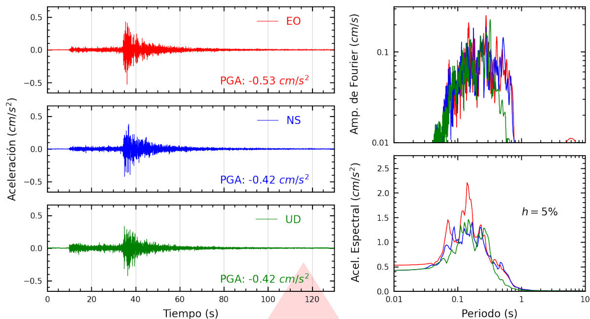
Figura A.5: Registros tiempo-historia, espectros de Fourier y de respuesta en las direcciones EO, NS y vertical de la estación CARAL. Sismo de Panao, Pachitea - Huánuco del 2026-08-11, 23:06:55 (Hora local)
