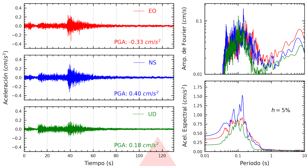
Figura A.7: Registros tiempo-historia, espectros de Fourier y de respuesta en las direcciones EO, NS y vertical de la estación UNAB. Sismo de Panao, Pachitea - Huánuco del 2026-08-11, 23:06:55 (Hora local)
