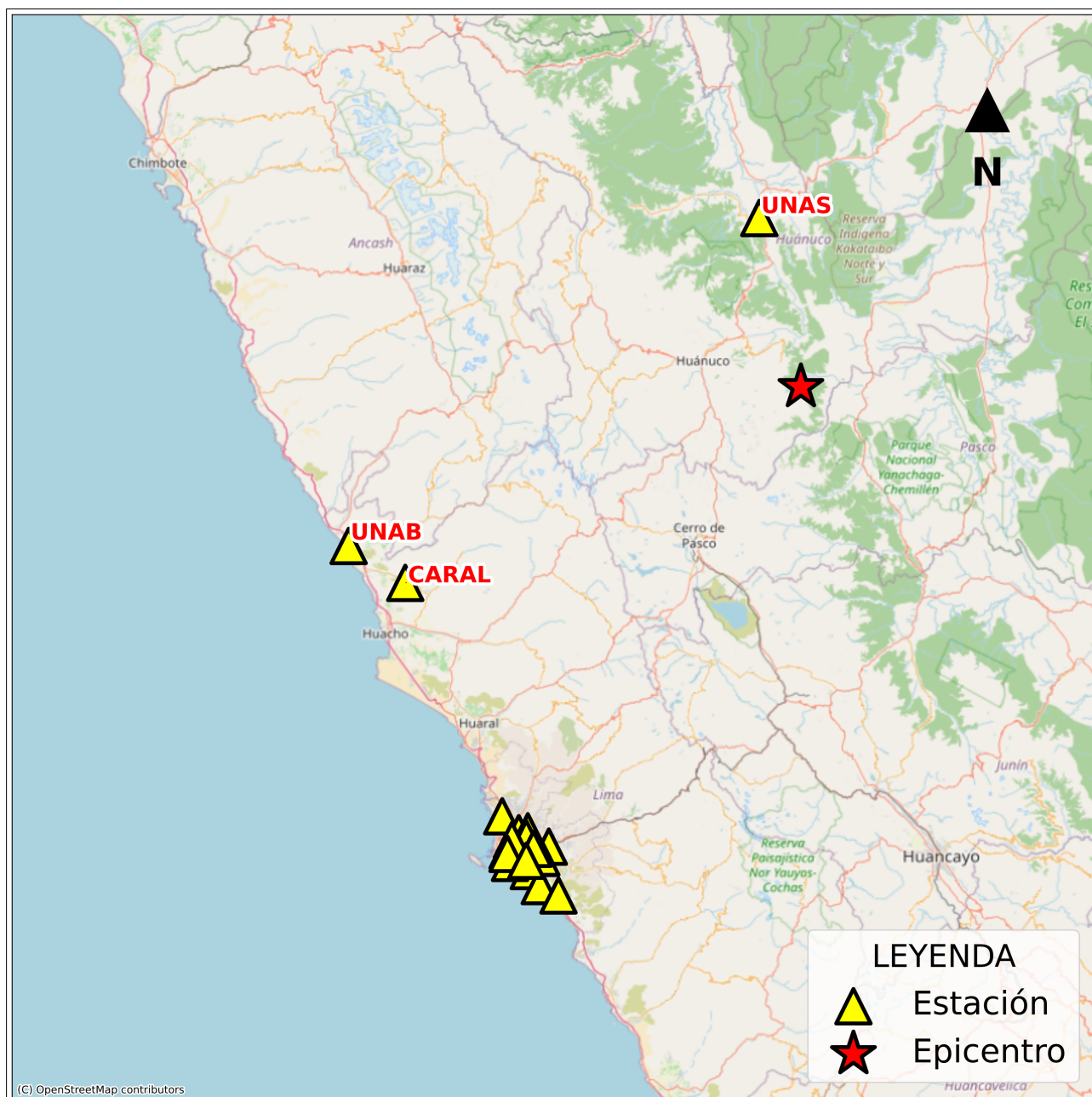
Figura 2: Mapa de ubicación de la(s) estación(es) acelerográfica(s) a nivel nacional correspondiente(s) al Sismo de Panao, Pachitea - Huánuco del 11 de agosto de 2026 a las 23:06:55 (hora local)
