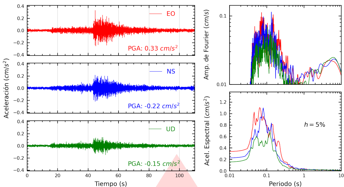
Figura A.9: Registros tiempo-historia, espectros de Fourier y de respuesta en las direcciones EO, NS y vertical de la estación FICPE. Sismo de Panao, Pachitea - Huánuco del 2026-08-11, 23:06:55 (Hora local)
