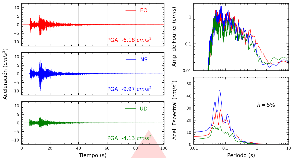
Figura A.27: Registros tiempo-historia, espectros de Fourier y de respuesta en las direcciones EO, NS y vertical de la estación UPCVI. Sismo de Lurín, Lima - Lima del 2026-08-19, 05:28:02 (Hora local)
