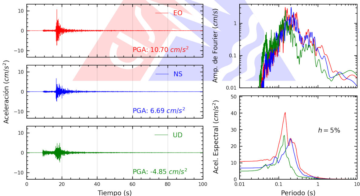
Figura A.24: Registros tiempo-historia, espectros de Fourier y de respuesta en las direcciones EO, NS y vertical de la estación DSMI. Sismo de Lurín, Lima - Lima del 2026-08-19, 05:28:02 (Hora local)
