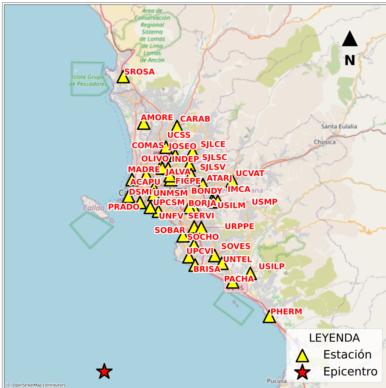
Figura 3: Mapa de ubicación de la(s) estación(es) acelerográfica(s) en Lima Metropolitana correspondiente(s) al Sismo de Lurín, Lima - Lima del 19 de agosto de 2026 a las 05:28:02 (hora local)
