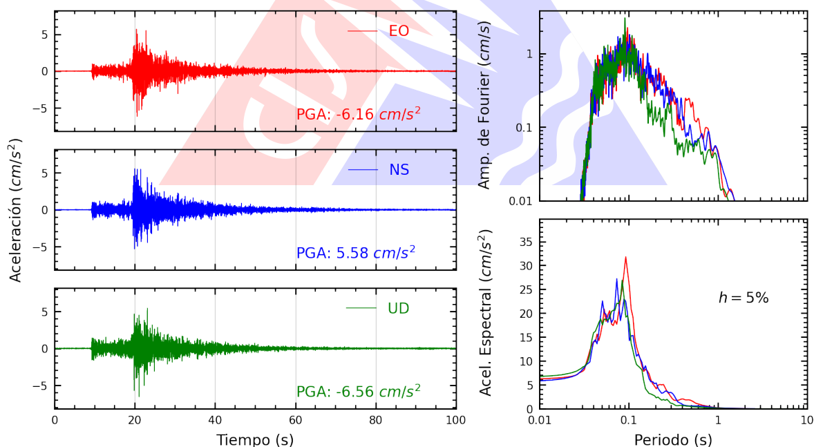
Figura A.38: Registros tiempo-historia, espectros de Fourier y de respuesta en las direcciones EO, NS y vertical de la estación ASIA. Sismo de Lurín, Lima - Lima del 2026-08-19, 05:28:02 (Hora local)
