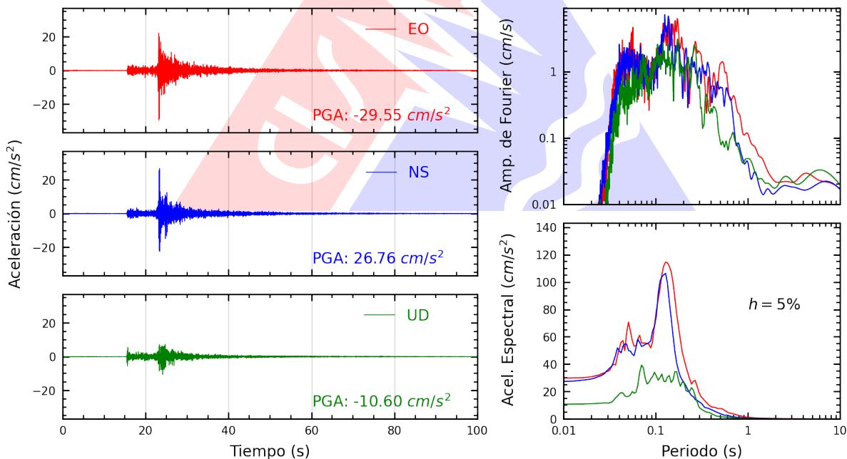
Figura A.4: Registros tiempo-historia, espectros de Fourier y de respuesta en las direcciones EO, NS y vertical de la estación OLIVO. Sismo de Lurín, Lima - Lima del 2026-08-19, 05:28:02 (Hora local)
