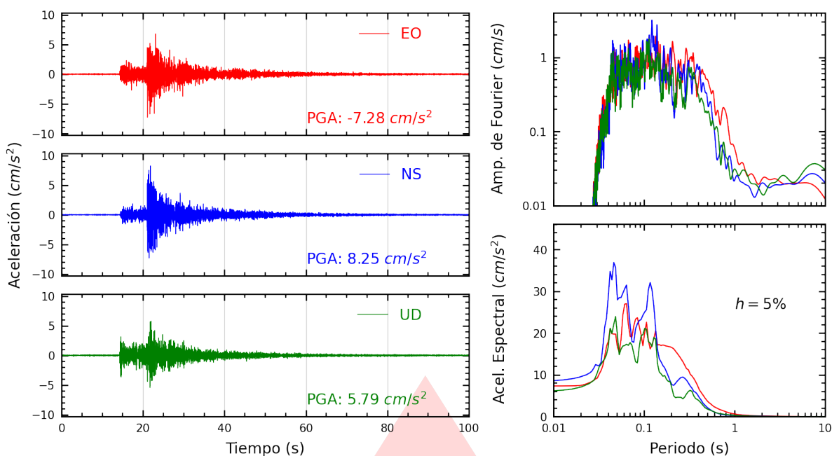
Figura A.33: Registros tiempo-historia, espectros de Fourier y de respuesta en las direcciones EO, NS y vertical de la estación URPE. Sismo de Lurín, Lima - Lima del 2026-08-19, 05:28:02 (Hora local)
