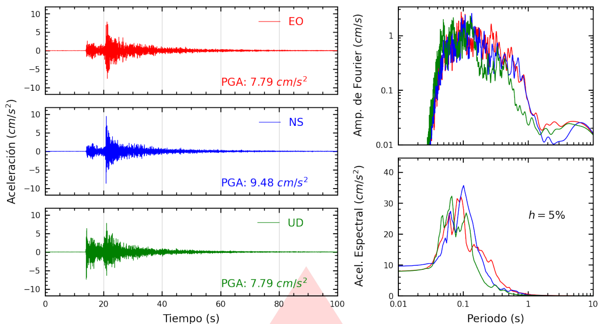
Figura A.29: Registros tiempo-historia, espectros de Fourier y de respuesta en las direcciones EO, NS y vertical de la estación USILP. Sismo de Lurín, Lima - Lima del 2026-08-19, 05:28:02 (Hora local)
