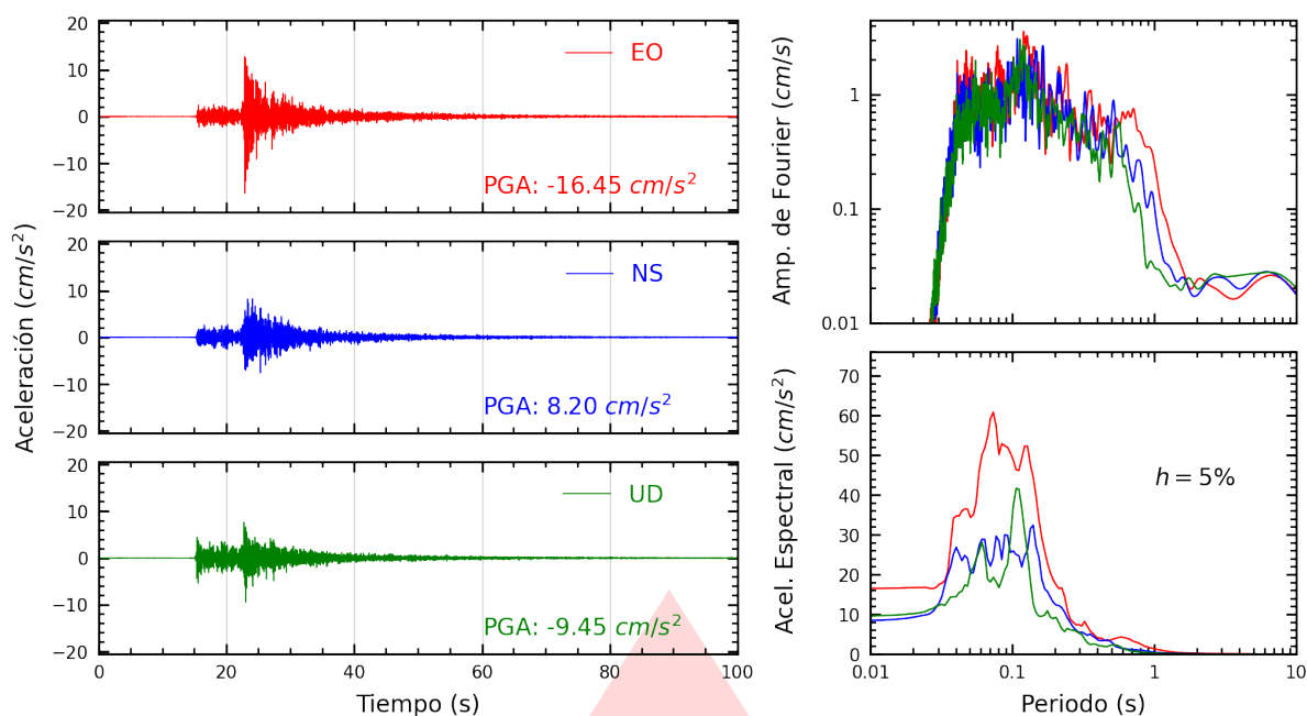
Figura A.15: Registros tiempo-historia, espectros de Fourier y de respuesta en las direcciones EO, NS y vertical de la estación UCVAT. Sismo de Lurín, Lima - Lima del 2026-08-19, 05:28:02 (Hora local)
