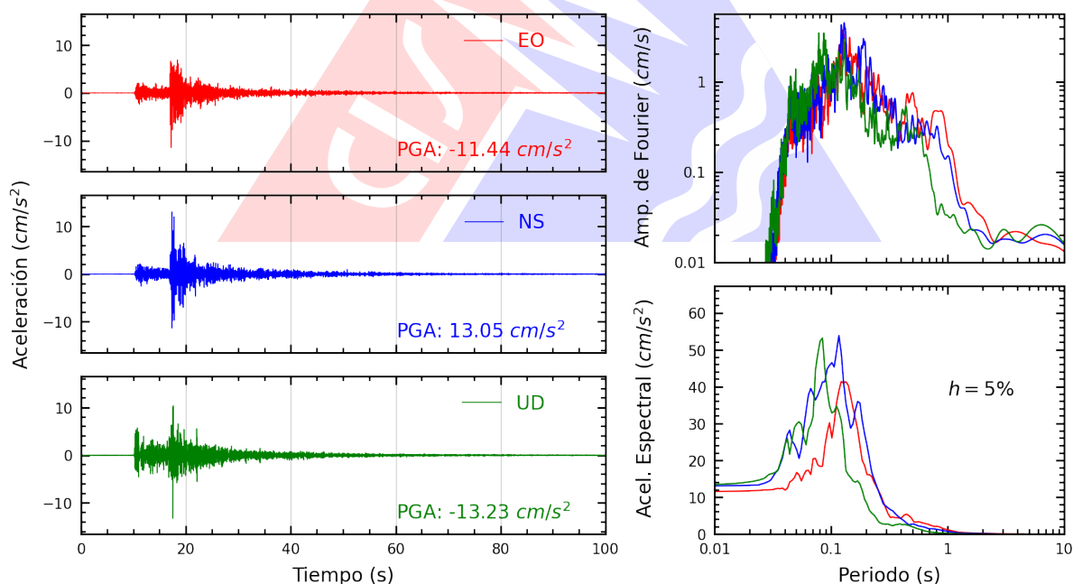
Figura A.16: Registros tiempo-historia, espectros de Fourier y de respuesta en las direcciones EO, NS y vertical de la estación SOCHO. Sismo de Lurín, Lima - Lima del 2026-08-19, 05:28:02 (Hora local)
