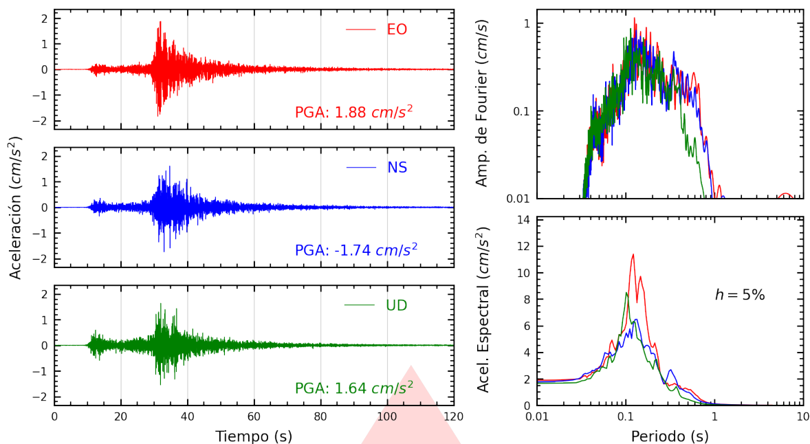
Figura A.41: Registros tiempo-historia, espectros de Fourier y de respuesta en las direcciones EO, NS y vertical de la estación CARAL. Sismo de Lurín, Lima - Lima del 2026-08-19, 05:28:02 (Hora local)
