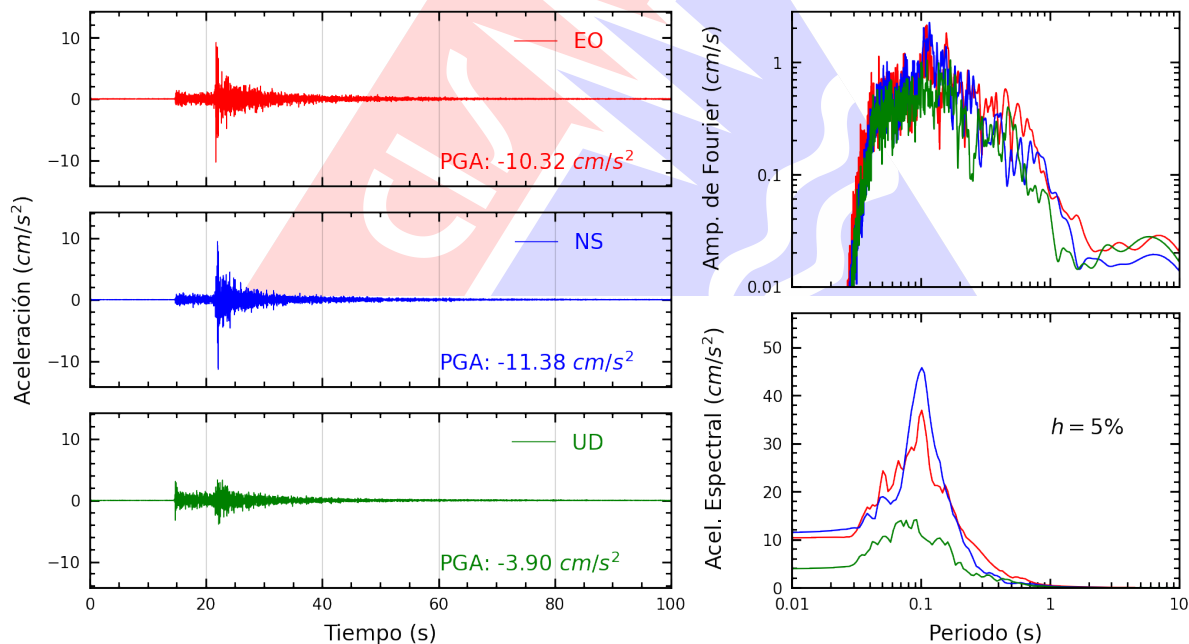
Figura A.20: Registros tiempo-historia, espectros de Fourier y de respuesta en las direcciones EO, NS y vertical de la estación INICT. Sismo de Lurín, Lima - Lima del 2026-08-19, 05:28:02 (Hora local)
