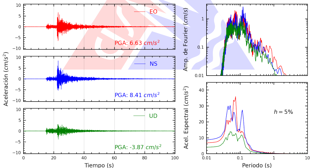
Figura A.32: Registros tiempo-historia, espectros de Fourier y de respuesta en las direcciones EO, NS y vertical de la estación ATARJ. Sismo de Lurín, Lima - Lima del 2026-08-19, 05:28:02 (Hora local)
