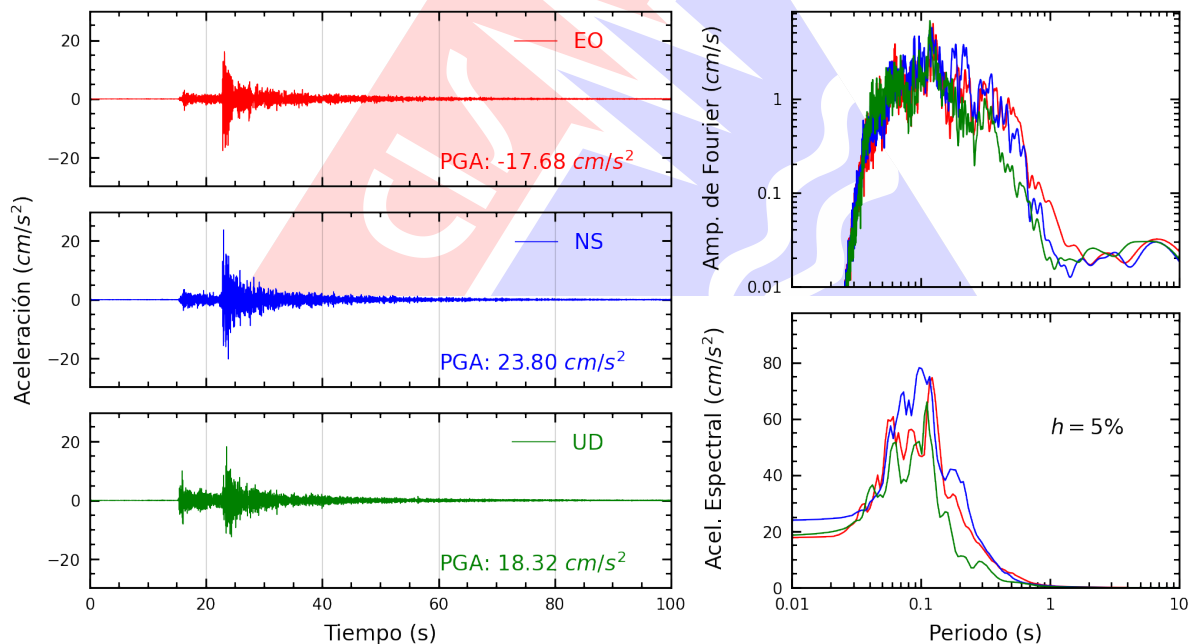
Figura A.6: Registros tiempo-historia, espectros de Fourier y de respuesta en las direcciones EO, NS y vertical de la estación SJLSC. Sismo de Lurín, Lima - Lima del 2026-08-19, 05:28:02 (Hora local)
