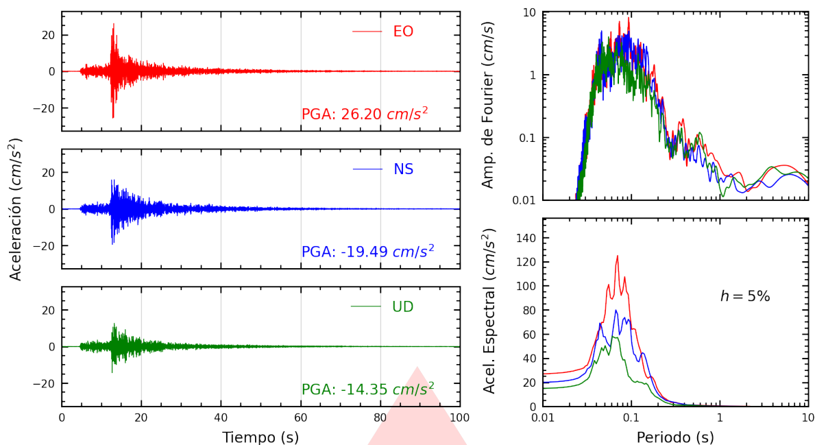
Figura A.5: Registros tiempo-historia, espectros de Fourier y de respuesta en las direcciones EO, NS y vertical de la estación JOSEO. Sismo de Lurín, Lima - Lima del 2026-08-19, 05:28:02 (Hora local)
