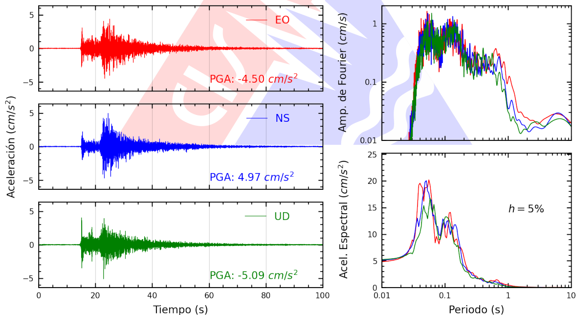
Figura A.40: Registros tiempo-historia, espectros de Fourier y de respuesta en las direcciones EO, NS y vertical de la estación IMCA. Sismo de Lurín, Lima - Lima del 2026-08-19, 05:28:02 (Hora local)
