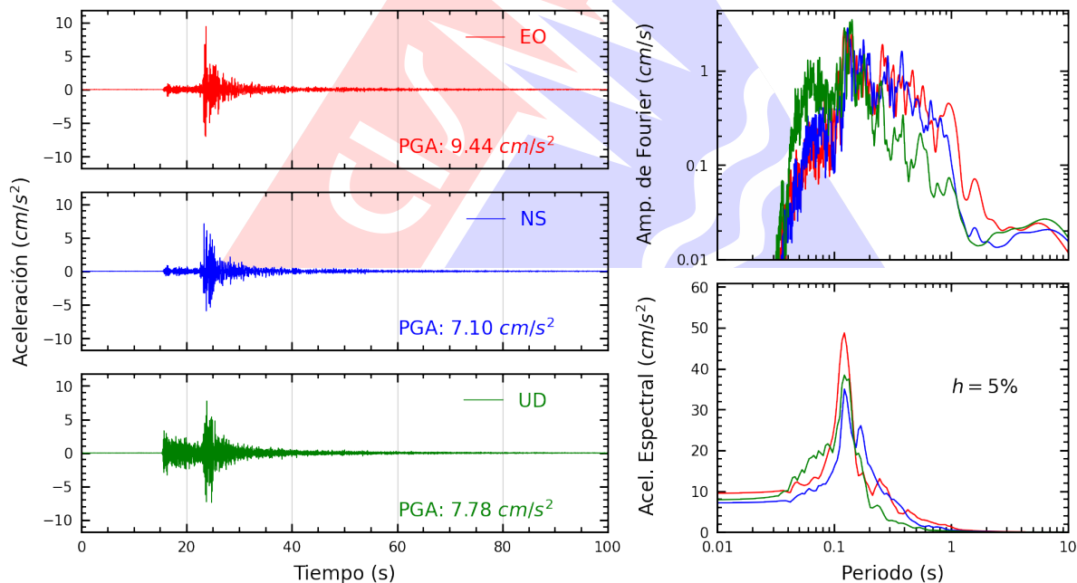
Figura A.30: Registros tiempo-historia, espectros de Fourier y de respuesta en las direcciones EO, NS y vertical de la estación ACAPU. Sismo de Lurín, Lima - Lima del 2026-08-19, 05:28:02 (Hora local)
