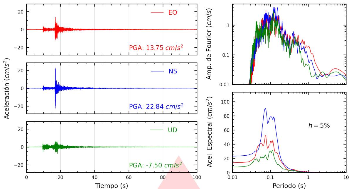
Figura A.7: Registros tiempo-historia, espectros de Fourier y de respuesta en las direcciones EO, NS y vertical de la estación UPCSM. Sismo de Lurín, Lima - Lima del 2026-08-19, 05:28:02 (Hora local)
