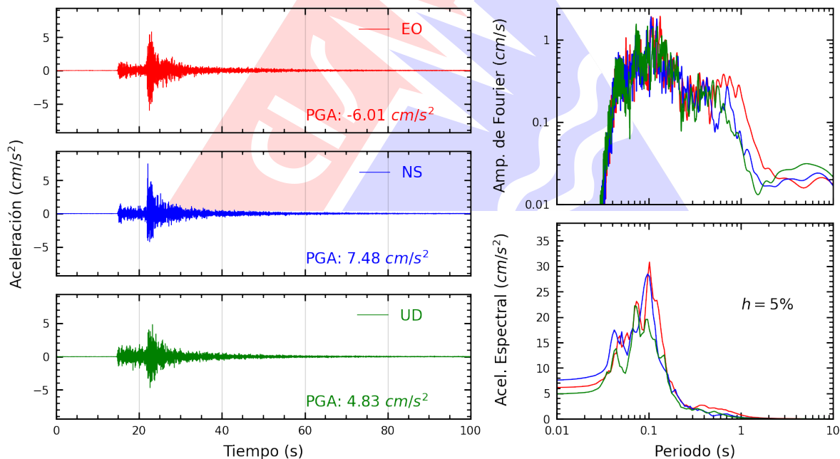
Figura A.36: Registros tiempo-historia, espectros de Fourier y de respuesta en las direcciones EO, NS y vertical de la estación UNFV. Sismo de Lurín, Lima - Lima del 2026-08-19, 05:28:02 (Hora local)
