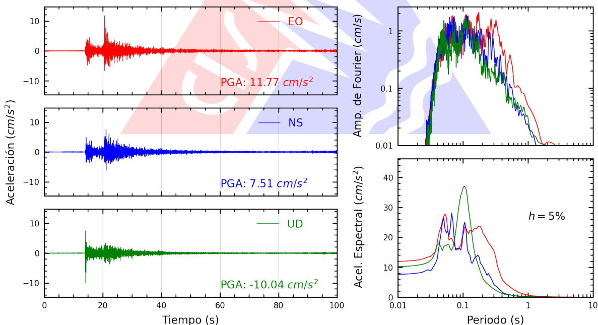
Figura A.18: Registros tiempo-historia, espectros de Fourier y de respuesta en las direcciones EO, NS y vertical de la estación PACHA. Sismo de Lurín, Lima - Lima del 2026-08-19, 05:28:02 (Hora local)
