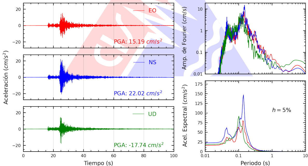
Figura A.8: Registros tiempo-historia, espectros de Fourier y de respuesta en las direcciones EO, NS y vertical de la estación CARAB. Sismo de Lurín, Lima - Lima del 2026-08-19, 05:28:02 (Hora local)
