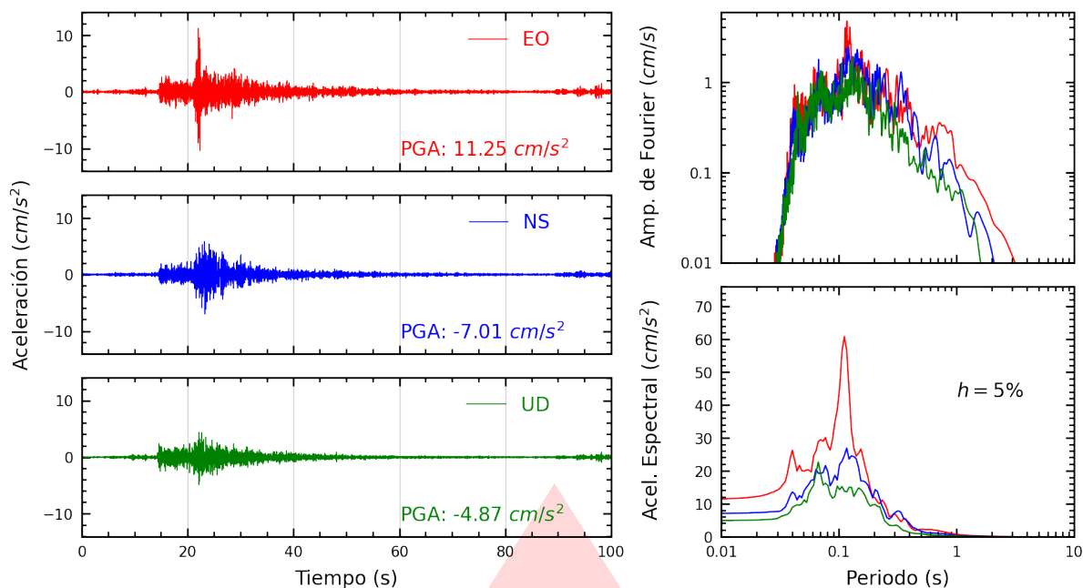
Figura A.21: Registros tiempo-historia, espectros de Fourier y de respuesta en las direcciones EO, NS y vertical de la estación SOBAR. Sismo de Lurín, Lima - Lima del 2026-08-19, 05:28:02 (Hora local)
