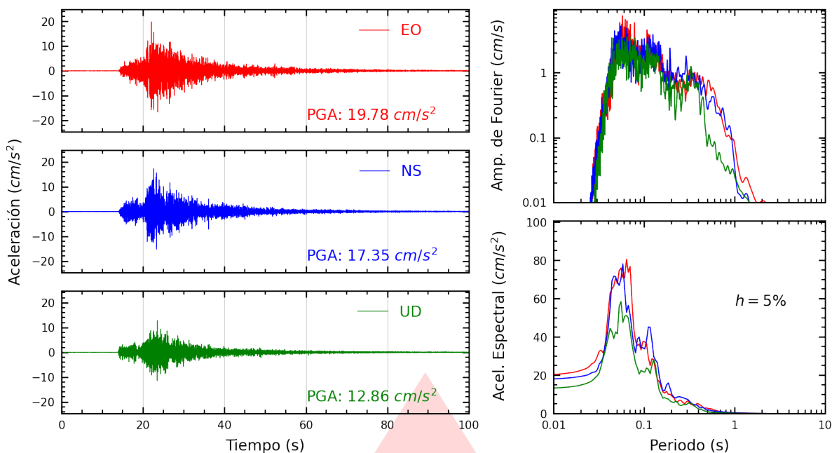
Figura A.11: Registros tiempo-historia, espectros de Fourier y de respuesta en las direcciones EO, NS y vertical de la estación UNTEL. Sismo de Lurín, Lima - Lima del 2026-08-19, 05:28:02 (Hora local)
