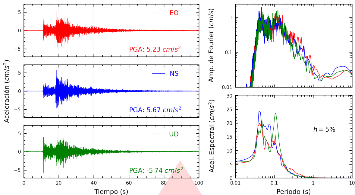
Figura A.39: Registros tiempo-historia, espectros de Fourier y de respuesta en las direcciones EO, NS y vertical de la estación USMP. Sismo de Lurín, Lima - Lima del 2026-08-19, 05:28:02 (Hora local)
