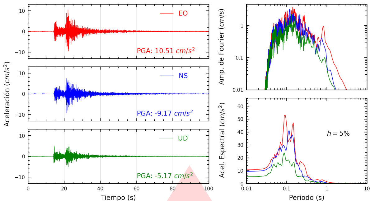
Figura A.25: Registros tiempo-historia, espectros de Fourier y de respuesta en las direcciones EO, NS y vertical de la estación BRISA. Sismo de Lurín, Lima - Lima del 2026-08-19, 05:28:02 (Hora local)
