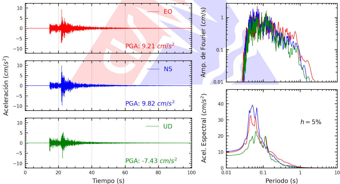
Figura A.28: Registros tiempo-historia, espectros de Fourier y de respuesta en las direcciones EO, NS y vertical de la estación BORJA. Sismo de Lurín, Lima - Lima del 2026-08-19, 05:28:02 (Hora local)
