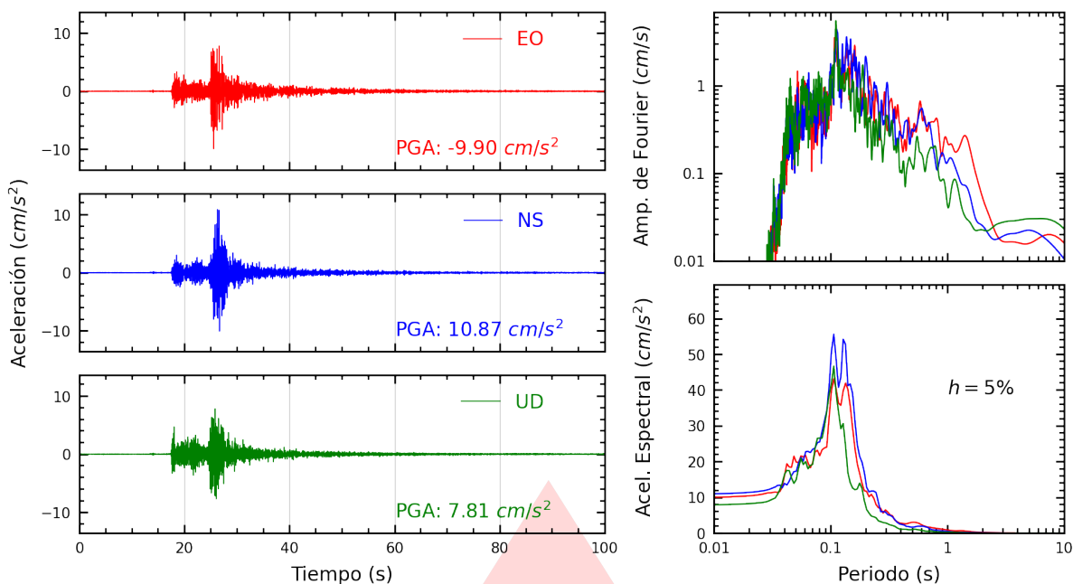
Figura A.23: Registros tiempo-historia, espectros de Fourier y de respuesta en las direcciones EO, NS y vertical de la estación PRADO. Sismo de Lurín, Lima - Lima del 2026-08-19, 05:28:02 (Hora local)
