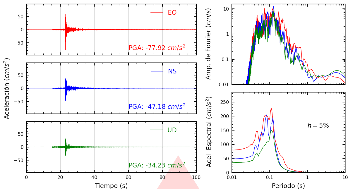
Figura A.1: Registros tiempo-historia, espectros de Fourier y de respuesta en las direcciones EO, NS y vertical de la estación INDEP. Sismo de Lurín, Lima - Lima del 2026-08-19, 05:28:02 (Hora local)
