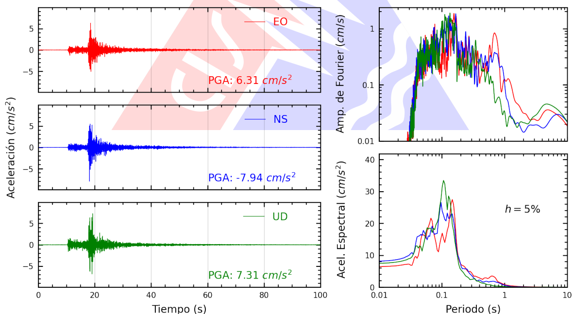
Figura A.34: Registros tiempo-historia, espectros de Fourier y de respuesta en las direcciones EO, NS y vertical de la estación UNMSM. Sismo de Lurín, Lima - Lima del 2026-08-19, 05:28:02 (Hora local)
