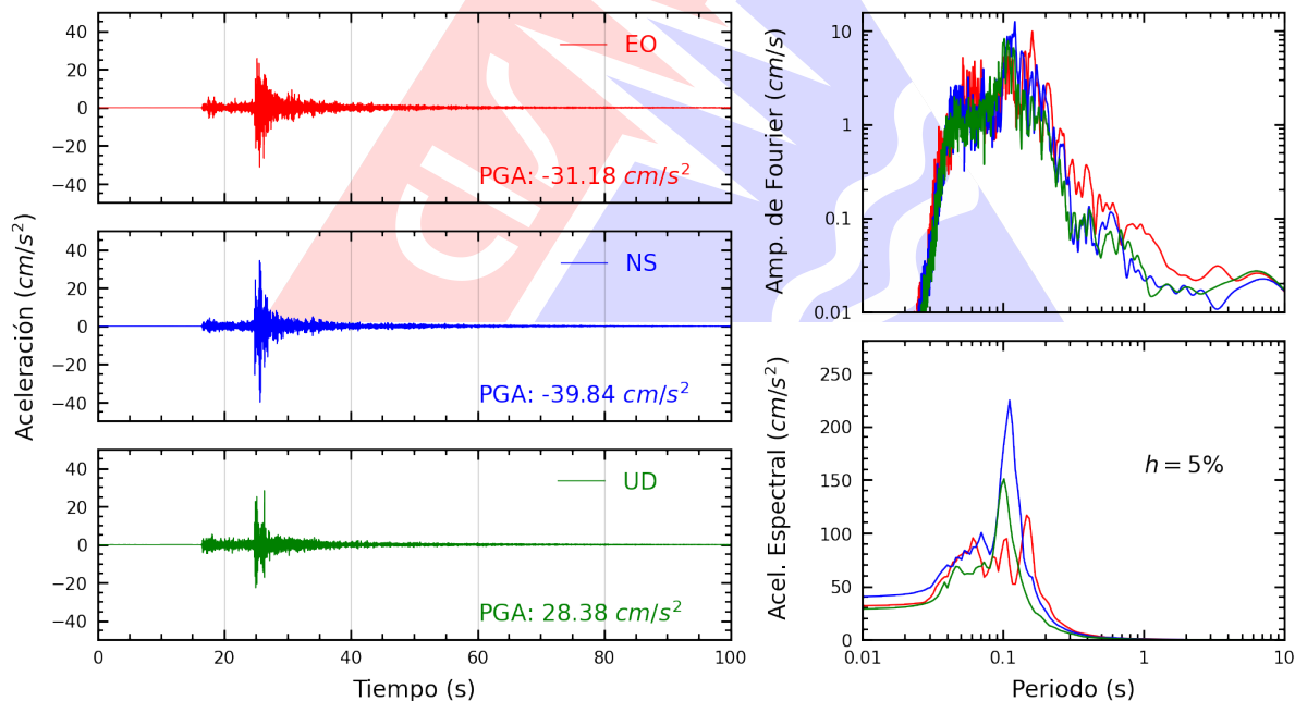
Figura A.2: Registros tiempo-historia, espectros de Fourier y de respuesta en las direcciones EO, NS y vertical de la estación AMORE. Sismo de Lurín, Lima - Lima del 2026-08-19, 05:28:02 (Hora local)
