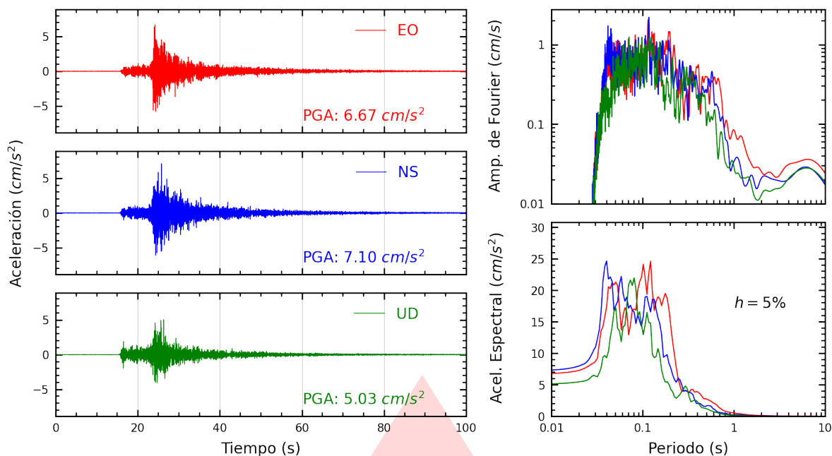
Figura A.37: Registros tiempo-historia, espectros de Fourier y de respuesta en las direcciones EO, NS y vertical de la estación COMAS. Sismo de Lurín, Lima - Lima del 2026-08-19, 05:28:02 (Hora local)
