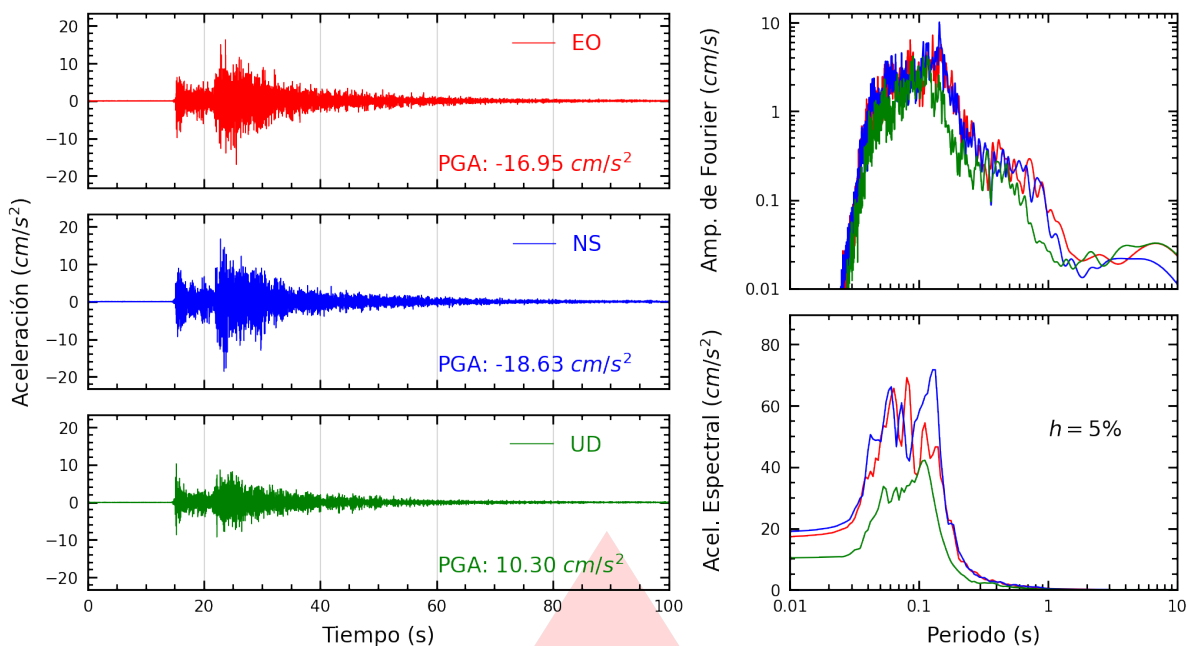
Figura A.13: Registros tiempo-historia, espectros de Fourier y de respuesta en las direcciones EO, NS y vertical de la estación USILM. Sismo de Lurín, Lima - Lima del 2026-08-19, 05:28:02 (Hora local)
