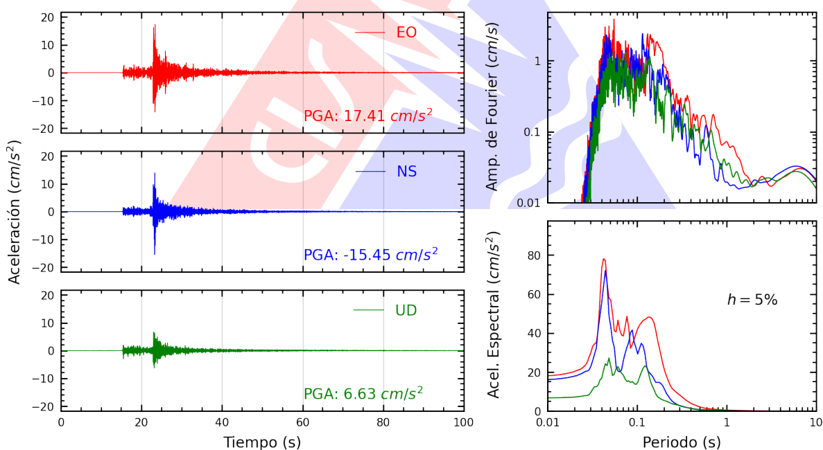
Figura A.14: Registros tiempo-historia, espectros de Fourier y de respuesta en las direcciones EO, NS y vertical de la estación UCSS. Sismo de Lurín, Lima - Lima del 2026-08-19, 05:28:02 (Hora local)
