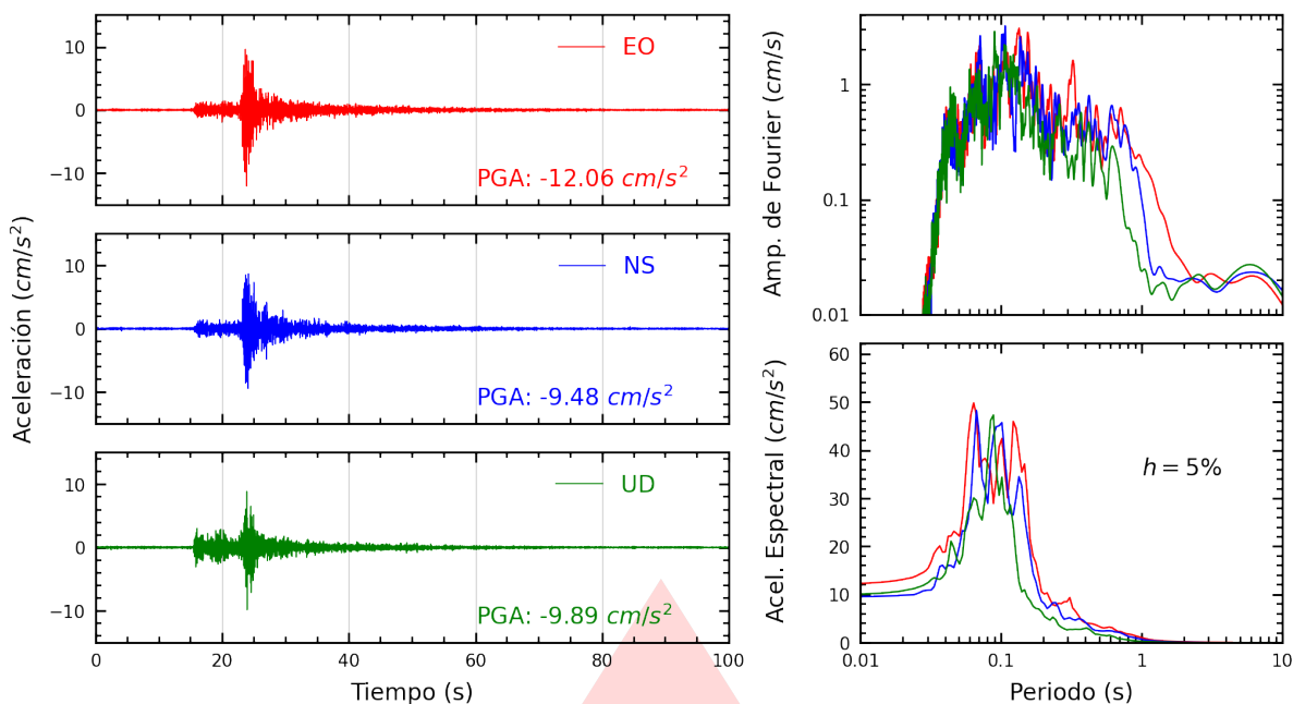
Figura A.17: Registros tiempo-historia, espectros de Fourier y de respuesta en las direcciones EO, NS y vertical de la estación MADRE. Sismo de Lurín, Lima - Lima del 2026-08-19, 05:28:02 (Hora local)
