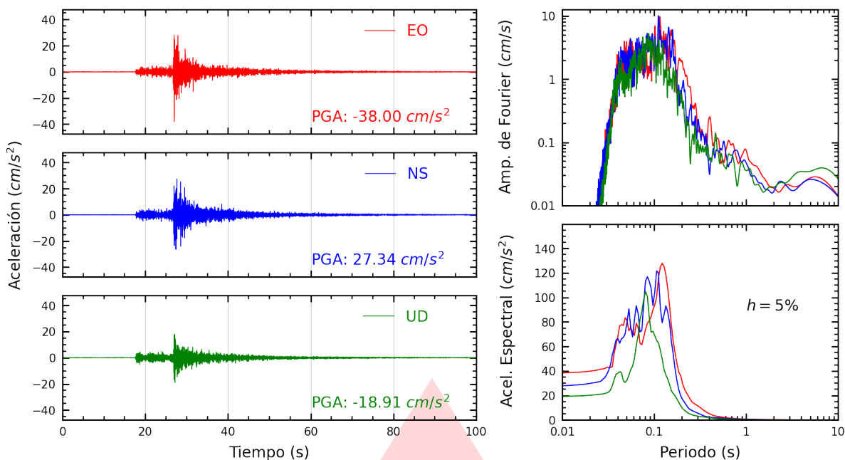
Figura A.3: Registros tiempo-historia, espectros de Fourier y de respuesta en las direcciones EO, NS y vertical de la estación SROSA. Sismo de Lurín, Lima - Lima del 2026-08-19, 05:28:02 (Hora local)
