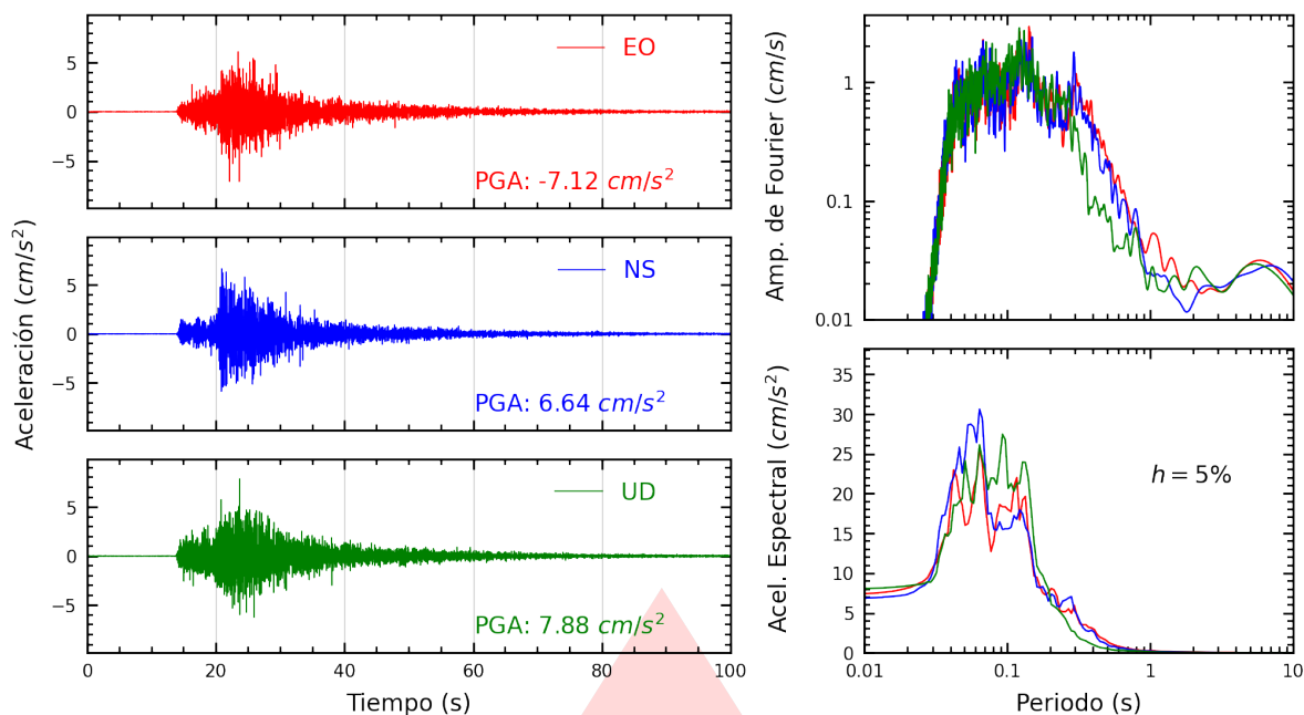
Figura A.35: Registros tiempo-historia, espectros de Fourier y de respuesta en las direcciones EO, NS y vertical de la estación SOVES. Sismo de Lurín, Lima - Lima del 2026-08-19, 05:28:02 (Hora local)
