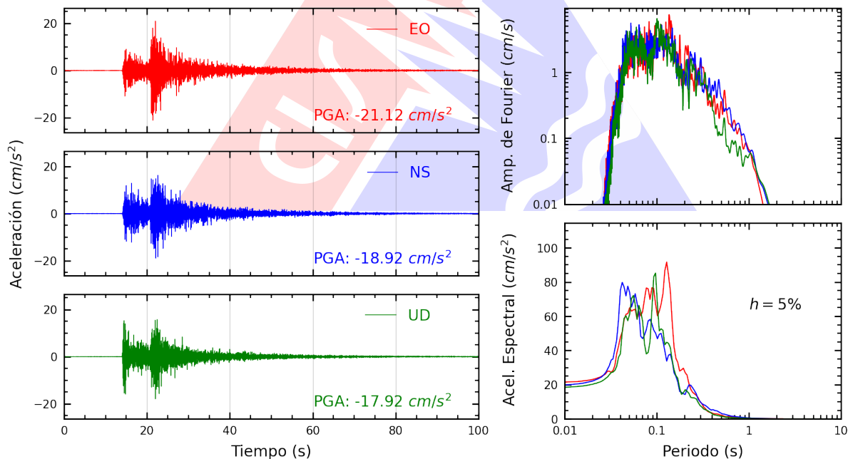
Figura A.10: Registros tiempo-historia, espectros de Fourier y de respuesta en las direcciones EO, NS y vertical de la estación PHERM. Sismo de Lurín, Lima - Lima del 2026-08-19, 05:28:02 (Hora local)
