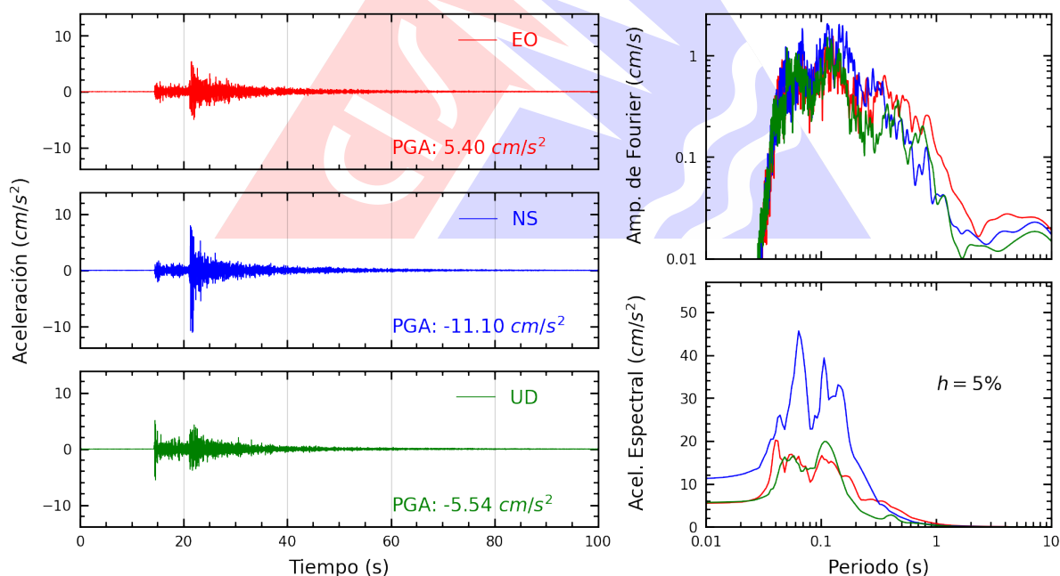
Figura A.22: Registros tiempo-historia, espectros de Fourier y de respuesta en las direcciones EO, NS y vertical de la estación SERVI. Sismo de Lurín, Lima - Lima del 2026-08-19, 05:28:02 (Hora local)
