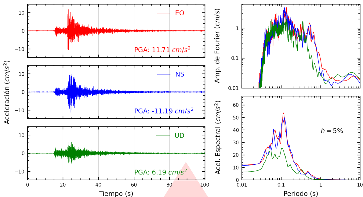
Figura A.19: Registros tiempo-historia, espectros de Fourier y de respuesta en las direcciones EO, NS y vertical de la estación SJLSV. Sismo de Lurín, Lima - Lima del 2026-08-19, 05:28:02 (Hora local)
