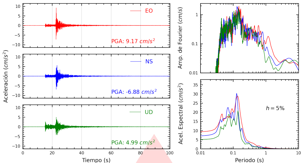
Figura A.31: Registros tiempo-historia, espectros de Fourier y de respuesta en las direcciones EO, NS y vertical de la estación BONDY. Sismo de Lurín, Lima - Lima del 2026-08-19, 05:28:02 (Hora local)
