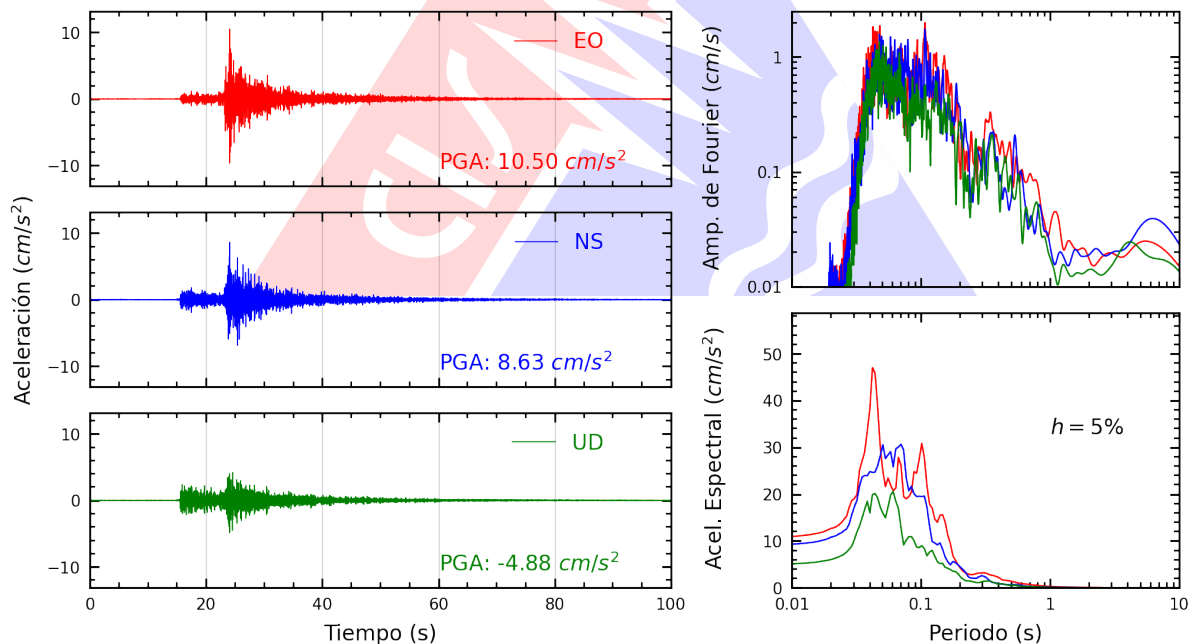
Figura A.26: Registros tiempo-historia, espectros de Fourier y de respuesta en las direcciones EO, NS y vertical de la estación SJLCE. Sismo de Lurín, Lima - Lima del 2026-08-19, 05:28:02 (Hora local)
