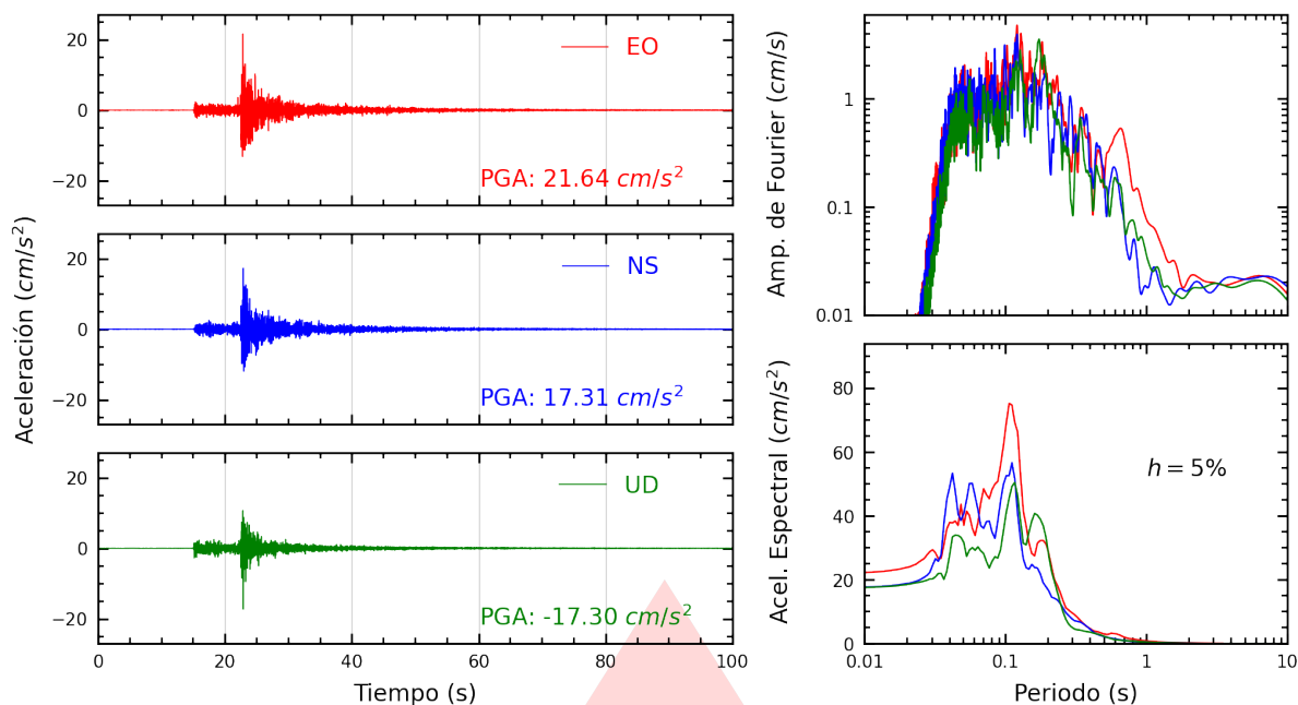
Figura A.9: Registros tiempo-historia, espectros de Fourier y de respuesta en las direcciones EO, NS y vertical de la estación FICPE. Sismo de Lurín, Lima - Lima del 2026-08-19, 05:28:02 (Hora local)
