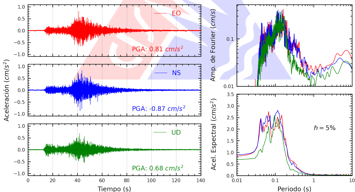
Figura A.42: Registros tiempo-historia, espectros de Fourier y de respuesta en las direcciones EO, NS y vertical de la estación UNAB. Sismo de Lurín, Lima - Lima del 2026-08-19, 05:28:02 (Hora local)
