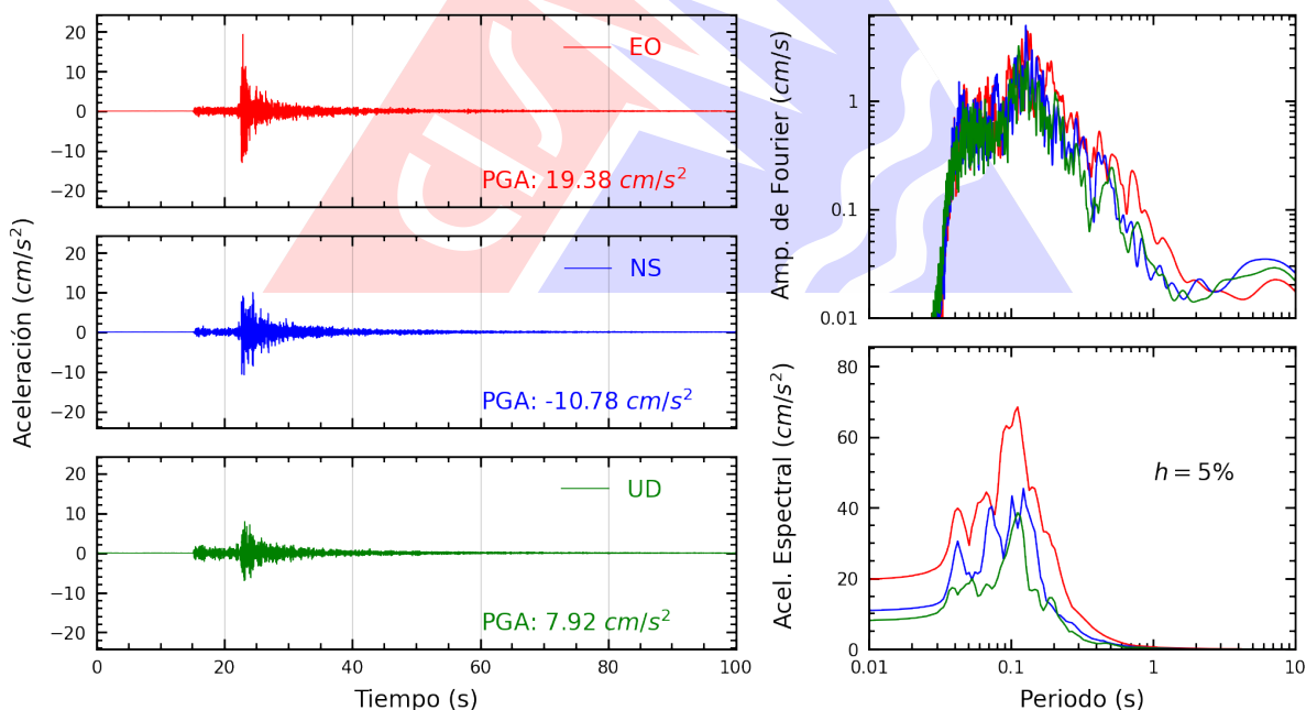
Figura A.12: Registros tiempo-historia, espectros de Fourier y de respuesta en las direcciones EO, NS y vertical de la estación JALVA. Sismo de Lurín, Lima - Lima del 2026-08-19, 05:28:02 (Hora local)
