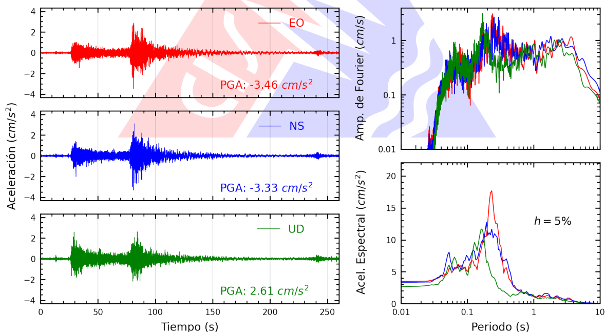
Figura A.22: Registros tiempo-historia, espectros de Fourier y de respuesta en las direcciones EO, NS y vertical de la estación UJBG4. Sismo de Coracora, Parinacochas - Ayacucho del 2026-08-20, 13:00:16 (Hora local)
