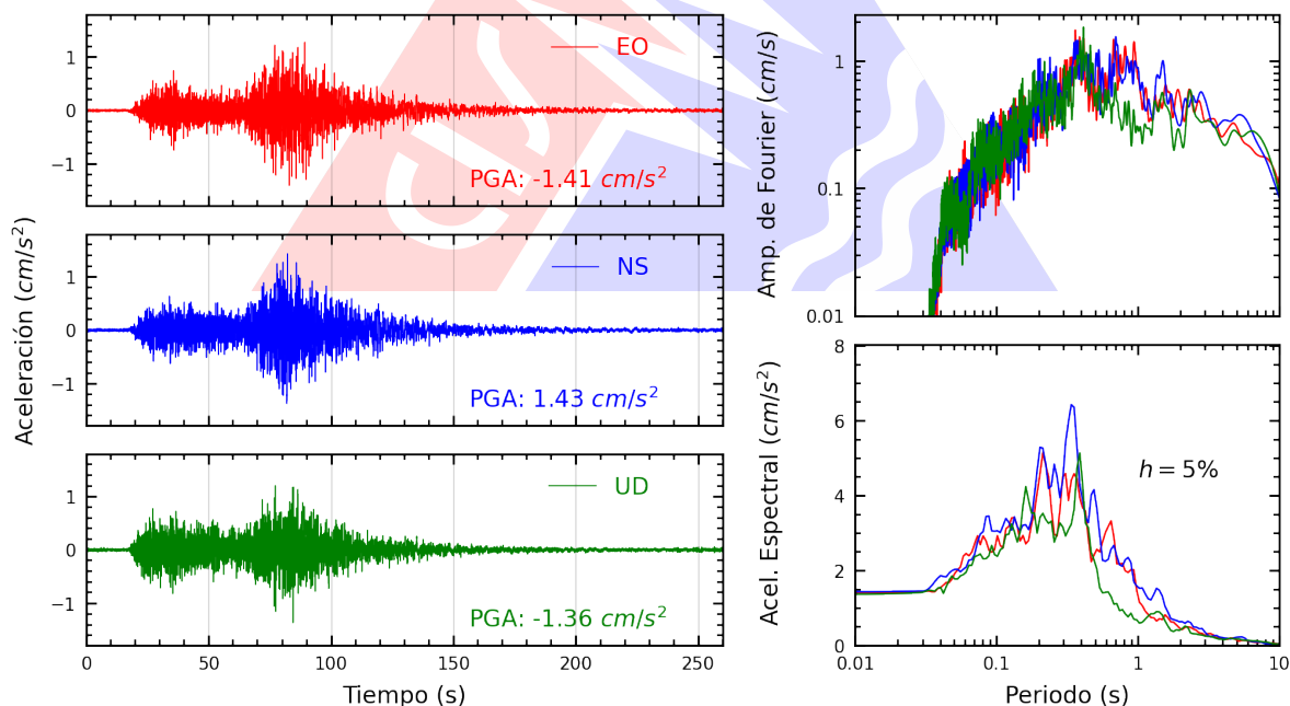
Figura A.50: Registros tiempo-historia, espectros de Fourier y de respuesta en las direcciones EO, NS y vertical de la estación UNFV. Sismo de Coracora, Parinacochas - Ayacucho del 2026-08-20, 13:00:16 (Hora local)
