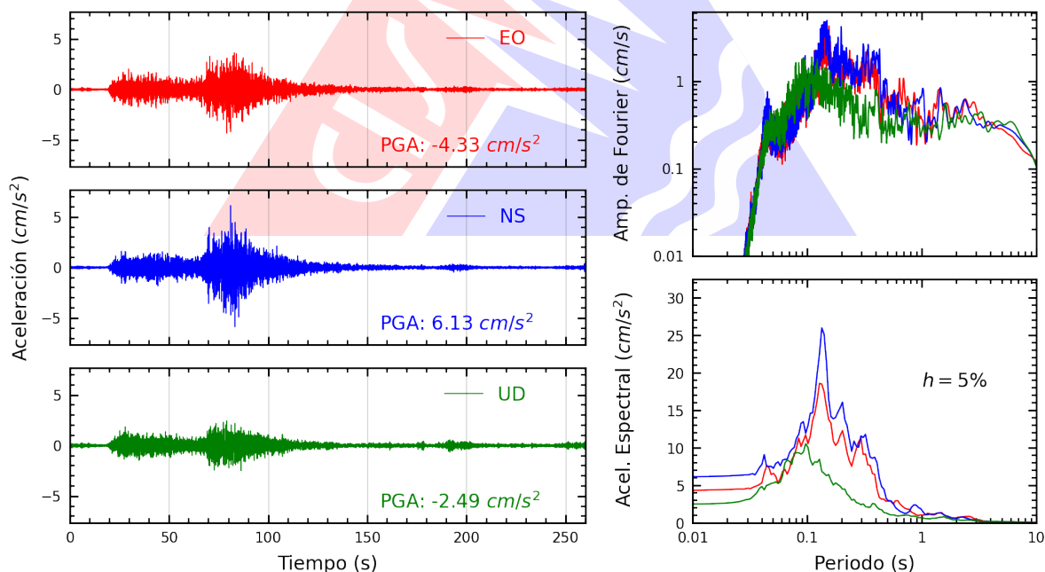
Figura A.8: Registros tiempo-historia, espectros de Fourier y de respuesta en las direcciones EO, NS y vertical de la estación CARAB. Sismo de Coracora, Parinacochas - Ayacucho del 2026-08-20, 13:00:16 (Hora local)
