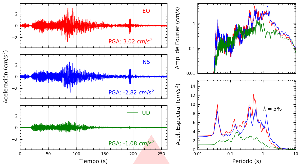
Figura A.29: Registros tiempo-historia, espectros de Fourier y de respuesta en las direcciones EO, NS y vertical de la estación DHNPE. Sismo de Coracora, Parinacochas - Ayacucho del 2026-08-20, 13:00:16 (Hora local)
