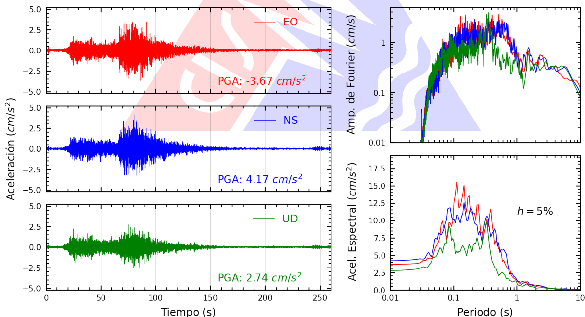
Figura A.16: Registros tiempo-historia, espectros de Fourier y de respuesta en las direcciones EO, NS y vertical de la estación SJLSV. Sismo de Coracora, Parinacochas - Ayacucho del 2026-08-20, 13:00:16 (Hora local)
