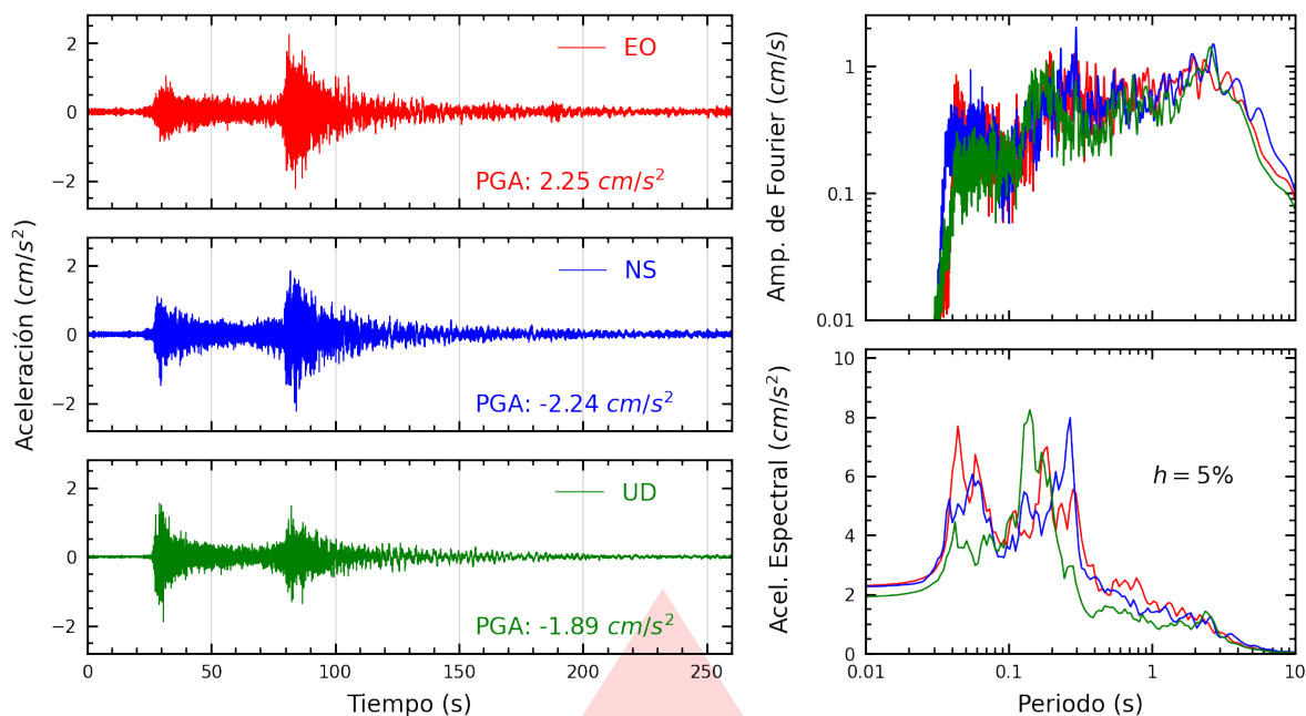
Figura A.37: Registros tiempo-historia, espectros de Fourier y de respuesta en las direcciones EO, NS y vertical de la estación UPTAC. Sismo de Coracora, Parinacochas - Ayacucho del 2026-08-20, 13:00:16 (Hora local)
