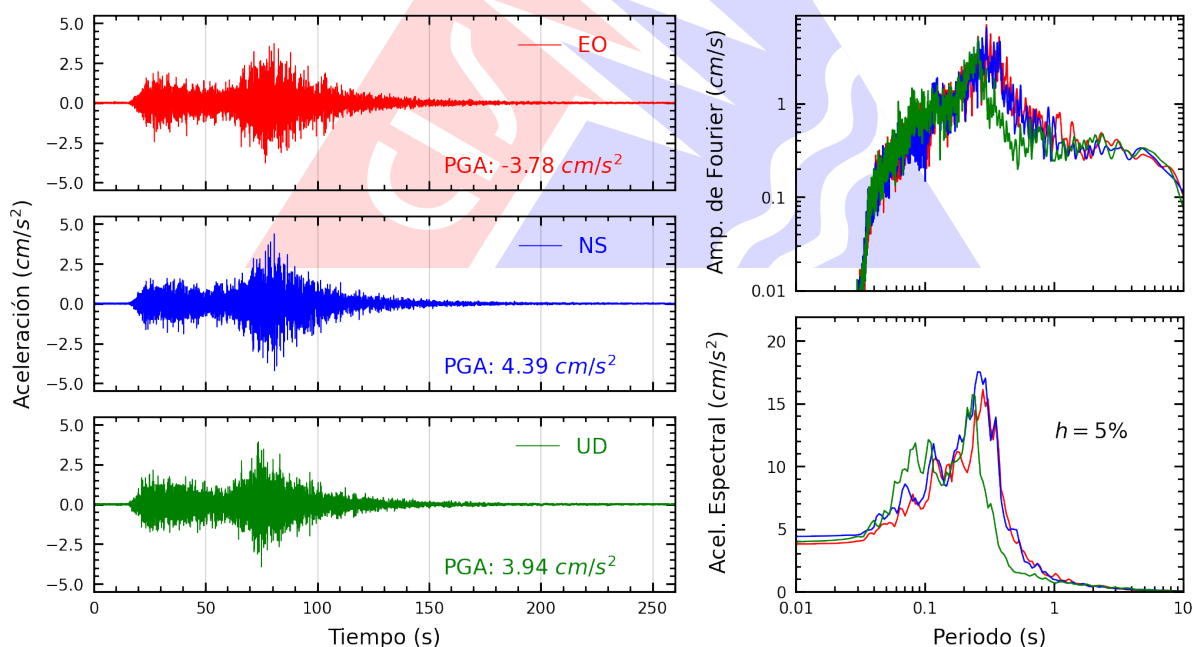
Figura A.14: Registros tiempo-historia, espectros de Fourier y de respuesta en las direcciones EO, NS y vertical de la estación SOVES. Sismo de Coracora, Parinacochas - Ayacucho del 2026-08-20, 13:00:16 (Hora local)
