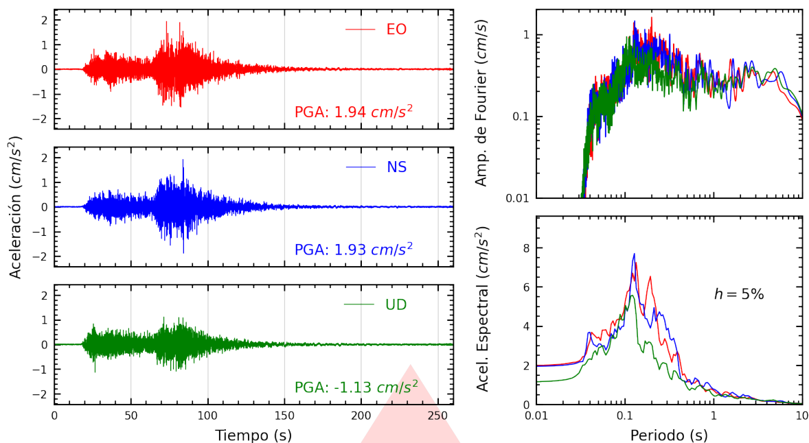
Figura A.41: Registros tiempo-historia, espectros de Fourier y de respuesta en las direcciones EO, NS y vertical de la estación JALVA. Sismo de Coracora, Parinacochas - Ayacucho del 2026-08-20, 13:00:16 (Hora local)
