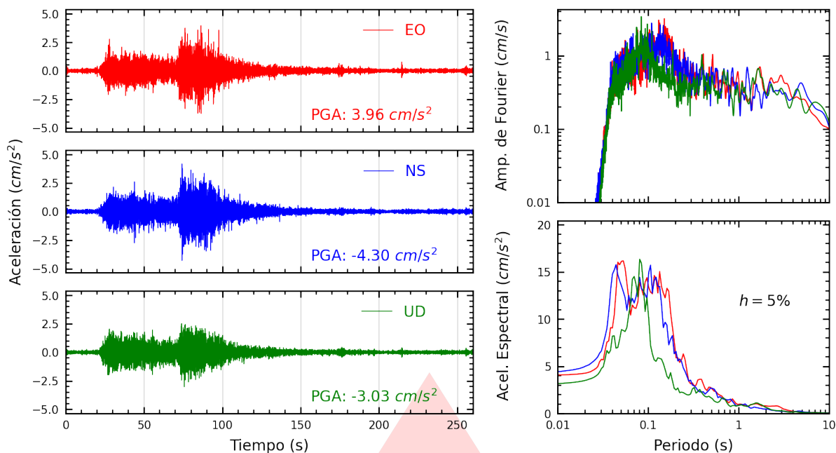
Figura A.15: Registros tiempo-historia, espectros de Fourier y de respuesta en las direcciones EO, NS y vertical de la estación SROSA. Sismo de Coracora, Parinacochas - Ayacucho del 2026-08-20, 13:00:16 (Hora local)
