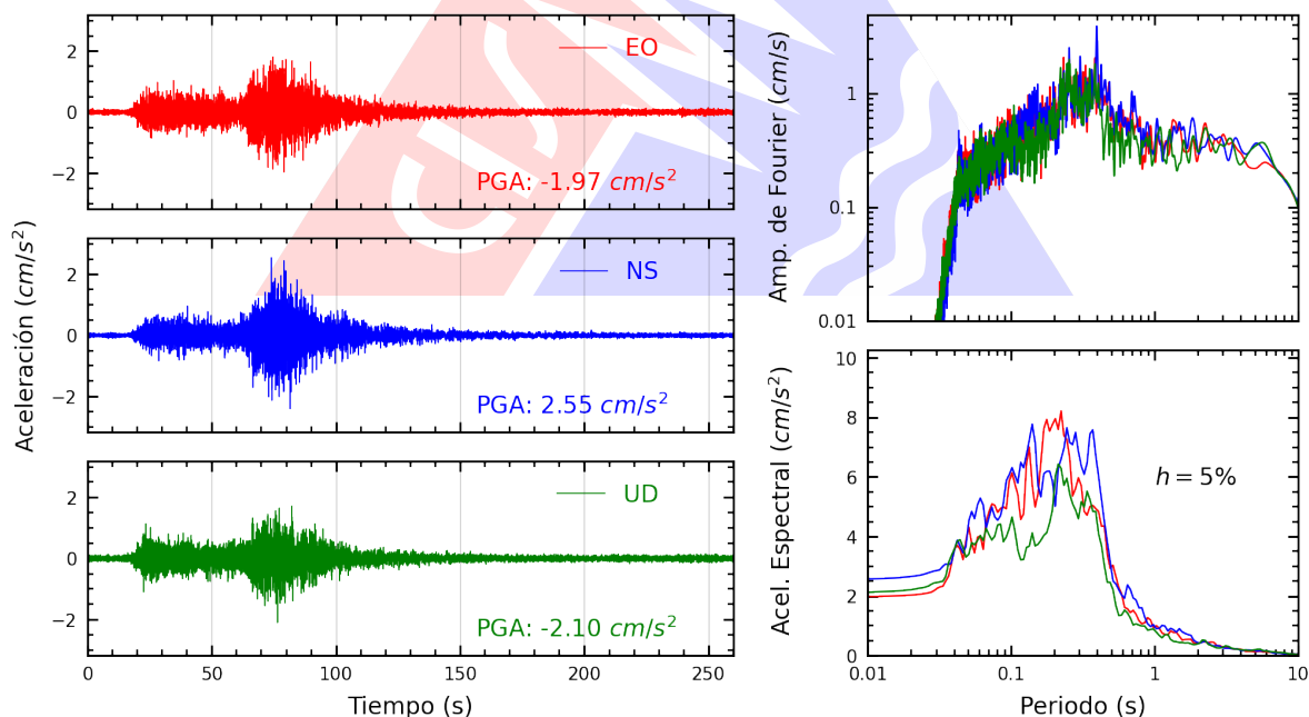
Figura A.34: Registros tiempo-historia, espectros de Fourier y de respuesta en las direcciones EO, NS y vertical de la estación URPE. Sismo de Coracora, Parinacochas - Ayacucho del 2026-08-20, 13:00:16 (Hora local)
