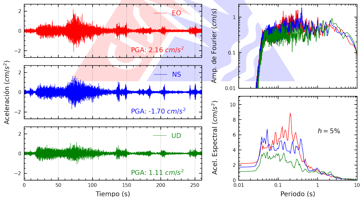
Figura A.40: Registros tiempo-historia, espectros de Fourier y de respuesta en las direcciones EO, NS y vertical de la estación PACHA. Sismo de Coracora, Parinacochas - Ayacucho del 2026-08-20, 13:00:16 (Hora local)
