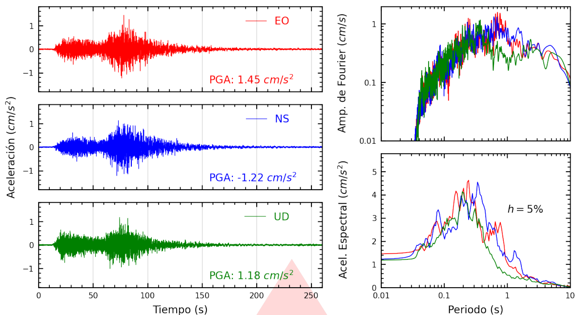
Figura A.49: Registros tiempo-historia, espectros de Fourier y de respuesta en las direcciones EO, NS y vertical de la estación UNMSM. Sismo de Coracora, Parinacochas - Ayacucho del 2026-08-20, 13:00:16 (Hora local)
