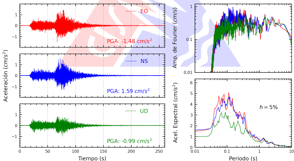
Figura A.46: Registros tiempo-historia, espectros de Fourier y de respuesta en las direcciones EO, NS y vertical de la estación ATARJ. Sismo de Coracora, Parinacochas - Ayacucho del 2026-08-20, 13:00:16 (Hora local)
