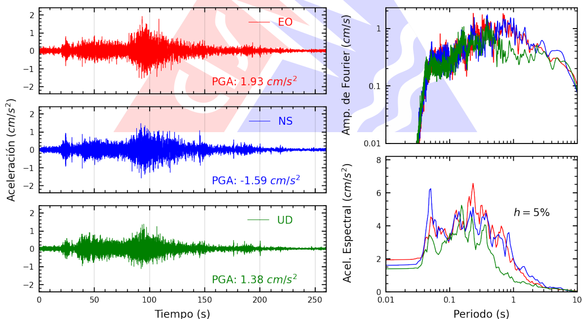
Figura A.42: Registros tiempo-historia, espectros de Fourier y de respuesta en las direcciones EO, NS y vertical de la estación UPCSM. Sismo de Coracora, Parinacochas - Ayacucho del 2026-08-20, 13:00:16 (Hora local)
