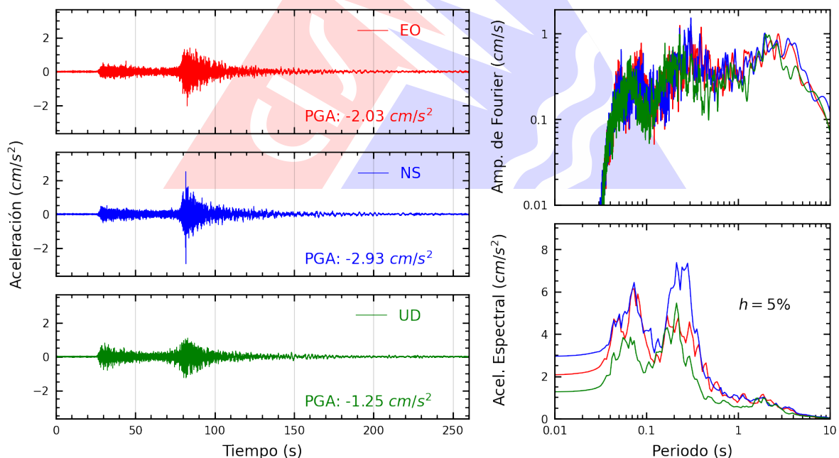
Figura A.30: Registros tiempo-historia, espectros de Fourier y de respuesta en las direcciones EO, NS y vertical de la estación CREY. Sismo de Coracora, Parinacochas - Ayacucho del 2026-08-20, 13:00:16 (Hora local)
