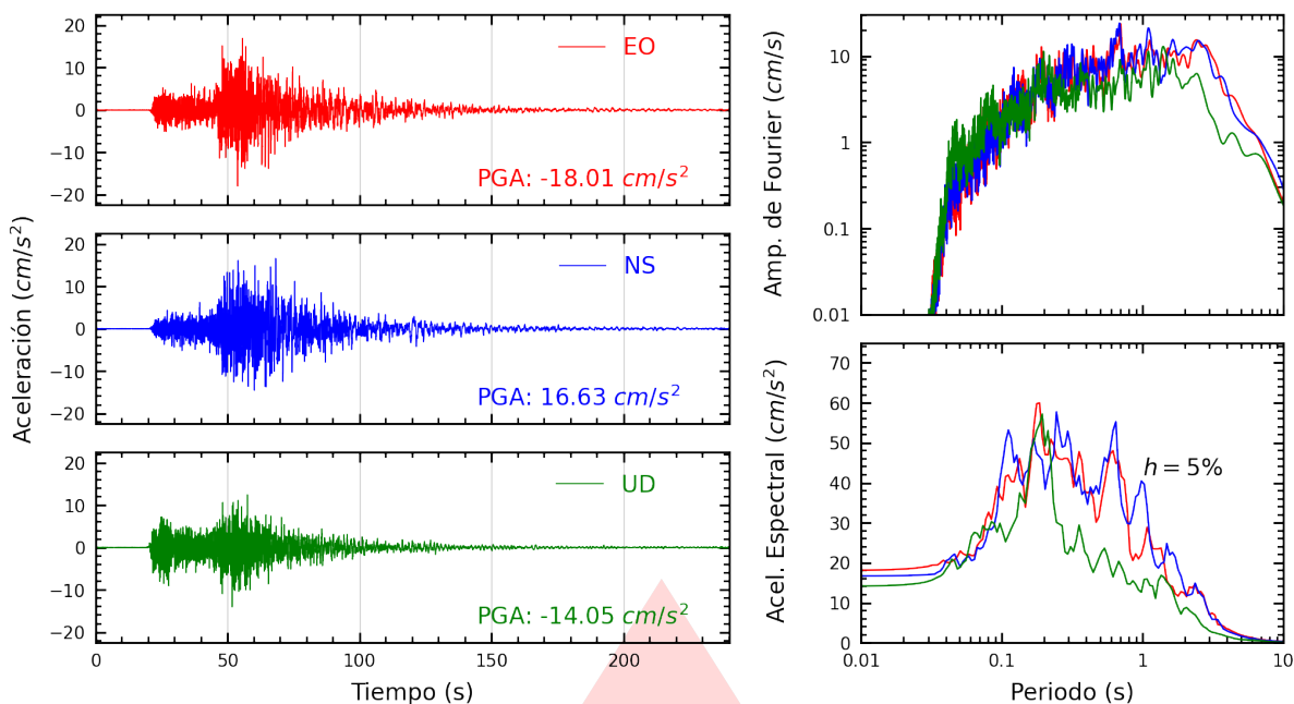
Figura A.3: Registros tiempo-historia, espectros de Fourier y de respuesta en las direcciones EO, NS y vertical de la estación UNICA. Sismo de Coracora, Parinacochas - Ayacucho del 2026-08-20, 13:00:16 (Hora local)
