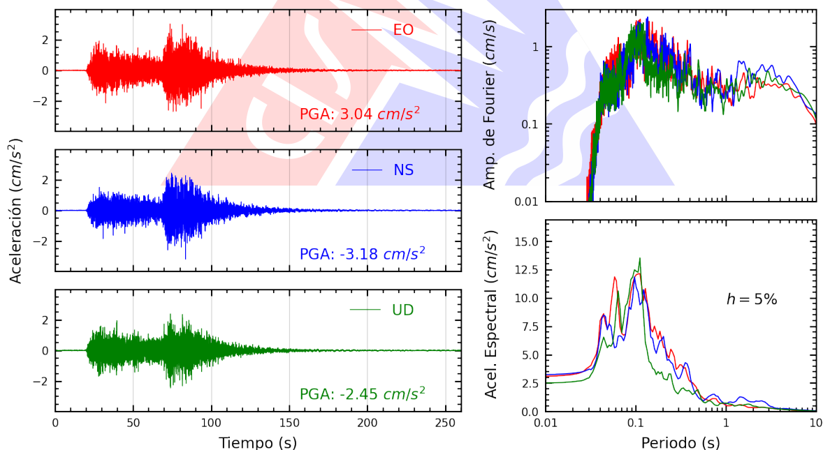
Figura A.26: Registros tiempo-historia, espectros de Fourier y de respuesta en las direcciones EO, NS y vertical de la estación AMORE. Sismo de Coracora, Parinacochas - Ayacucho del 2026-08-20, 13:00:16 (Hora local)
