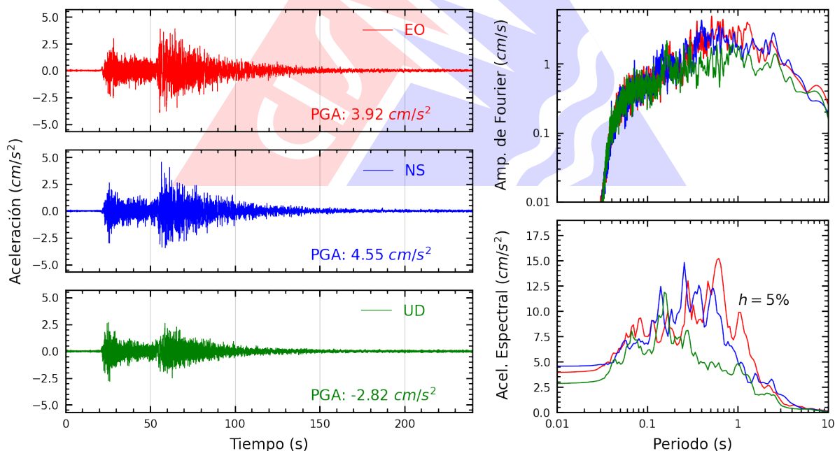
Figura A.12: Registros tiempo-historia, espectros de Fourier y de respuesta en las direcciones EO, NS y vertical de la estación SCARQ. Sismo de Coracora, Parinacochas - Ayacucho del 2026-08-20, 13:00:16 (Hora local)
