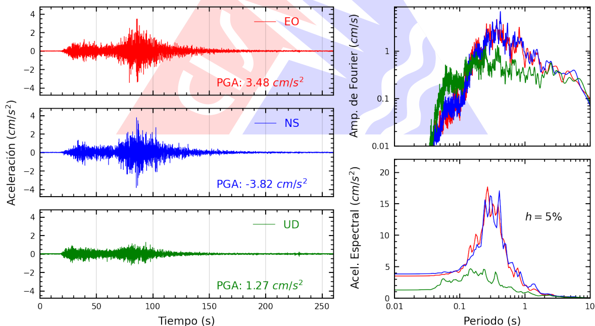
Figura A.20: Registros tiempo-historia, espectros de Fourier y de respuesta en las direcciones EO, NS y vertical de la estación ACAPU. Sismo de Coracora, Parinacochas - Ayacucho del 2026-08-20, 13:00:16 (Hora local)
