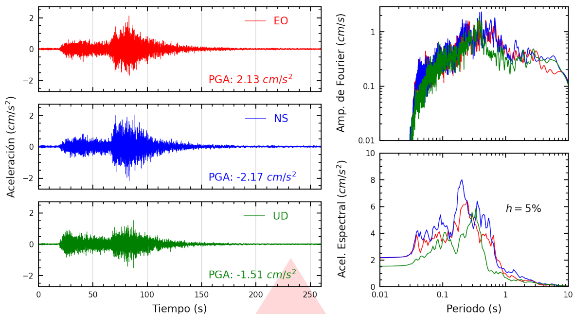
Figura A.39: Registros tiempo-historia, espectros de Fourier y de respuesta en las direcciones EO, NS y vertical de la estación COMAS. Sismo de Coracora, Parinacochas - Ayacucho del 2026-08-20, 13:00:16 (Hora local)
