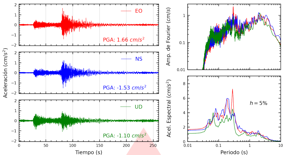
Figura A.45: Registros tiempo-historia, espectros de Fourier y de respuesta en las direcciones EO, NS y vertical de la estación UJBG2. Sismo de Coracora, Parinacochas - Ayacucho del 2026-08-20, 13:00:16 (Hora local)
