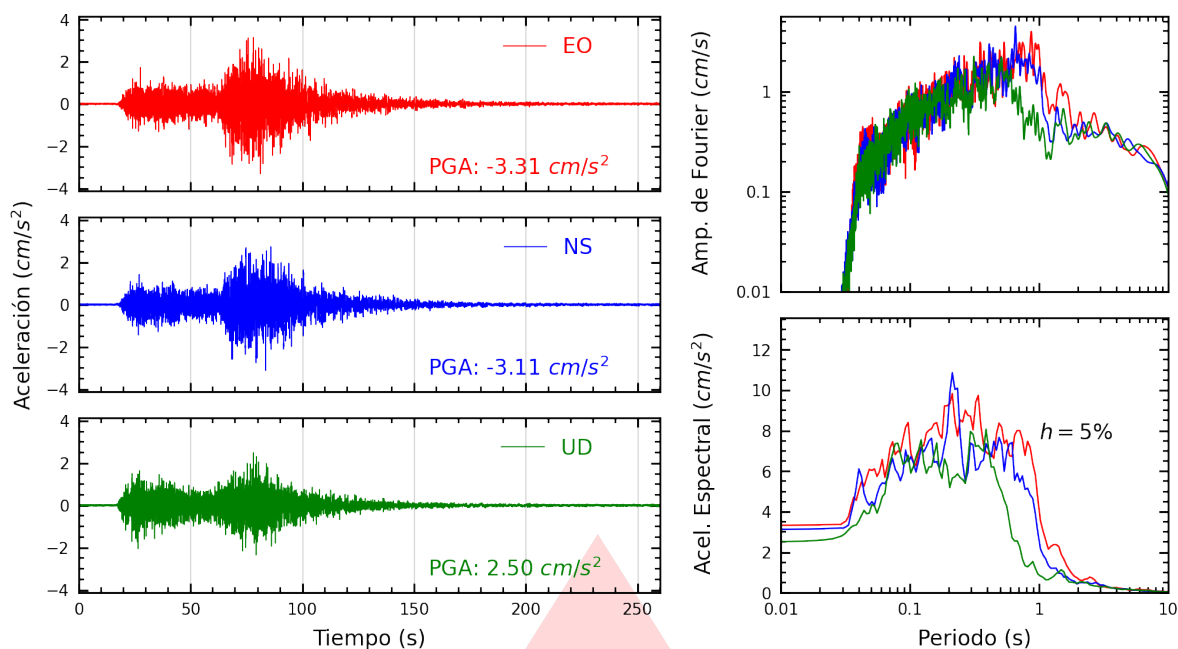
Figura A.25: Registros tiempo-historia, espectros de Fourier y de respuesta en las direcciones EO, NS y vertical de la estación UCVAT. Sismo de Coracora, Parinacochas - Ayacucho del 2026-08-20, 13:00:16 (Hora local)
