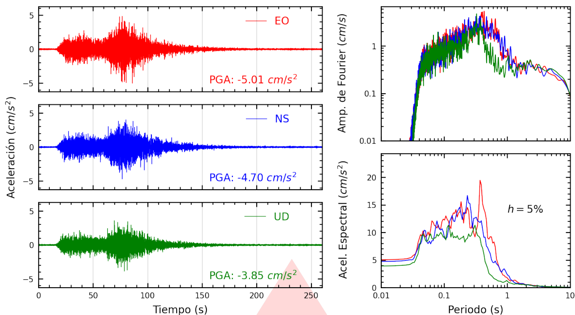
Figura A.11: Registros tiempo-historia, espectros de Fourier y de respuesta en las direcciones EO, NS y vertical de la estación UNTEL. Sismo de Coracora, Parinacochas - Ayacucho del 2026-08-20, 13:00:16 (Hora local)
