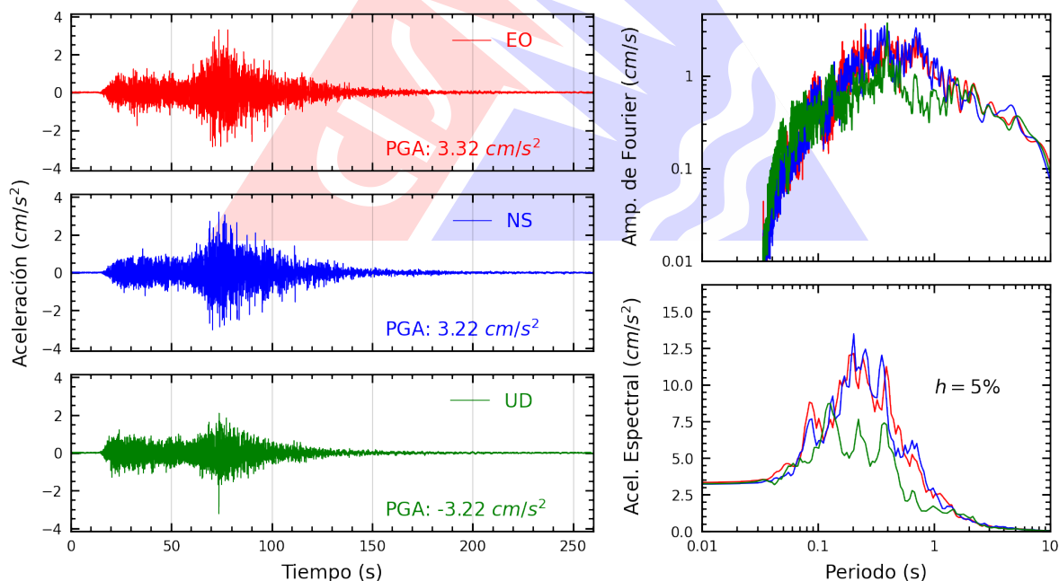
Figura A.24: Registros tiempo-historia, espectros de Fourier y de respuesta en las direcciones EO, NS y vertical de la estación USILP. Sismo de Coracora, Parinacochas - Ayacucho del 2026-08-20, 13:00:16 (Hora local)
