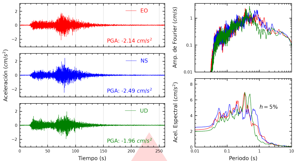
Figura A.35: Registros tiempo-historia, espectros de Fourier y de respuesta en las direcciones EO, NS y vertical de la estación IMCA. Sismo de Coracora, Parinacochas - Ayacucho del 2026-08-20, 13:00:16 (Hora local)
