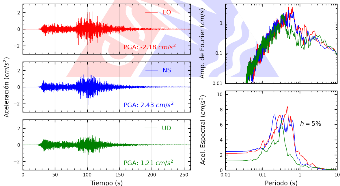
Figura A.36: Registros tiempo-historia, espectros de Fourier y de respuesta en las direcciones EO, NS y vertical de la estación CARAL. Sismo de Coracora, Parinacochas - Ayacucho del 2026-08-20, 13:00:16 (Hora local)
