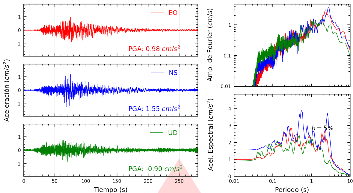
Figura A.47: Registros tiempo-historia, espectros de Fourier y de respuesta en las direcciones EO, NS y vertical de la estación SCHYO. Sismo de Coracora, Parinacochas - Ayacucho del 2026-08-20, 13:00:16 (Hora local)
