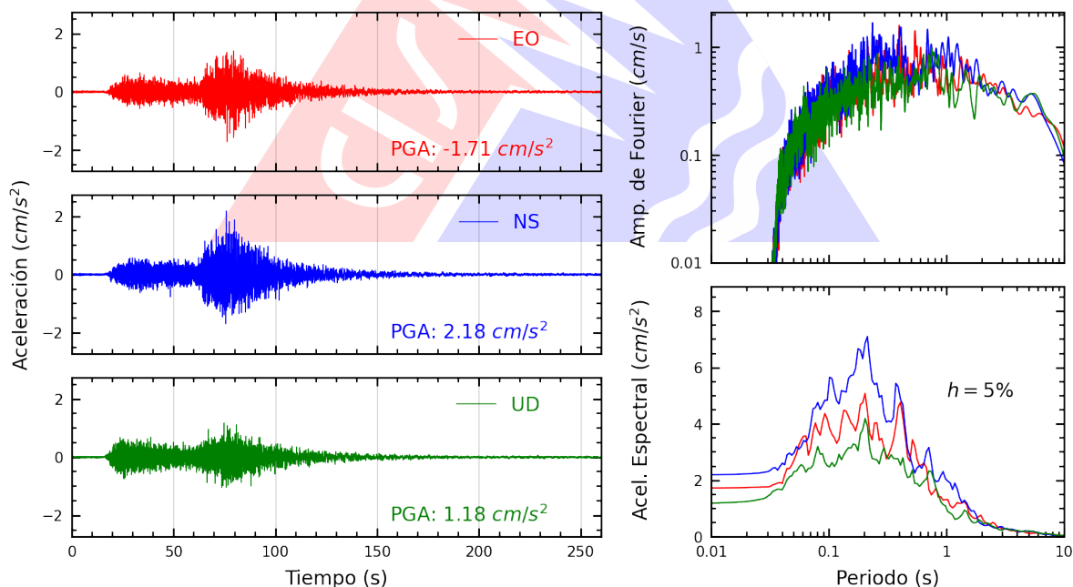
Figura A.38: Registros tiempo-historia, espectros de Fourier y de respuesta en las direcciones EO, NS y vertical de la estación SERVI. Sismo de Coracora, Parinacochas - Ayacucho del 2026-08-20, 13:00:16 (Hora local)
