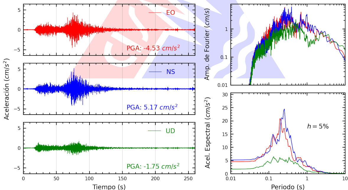
Figura A.10: Registros tiempo-historia, espectros de Fourier y de respuesta en las direcciones EO, NS y vertical de la estación BRISA. Sismo de Coracora, Parinacochas - Ayacucho del 2026-08-20, 13:00:16 (Hora local)
