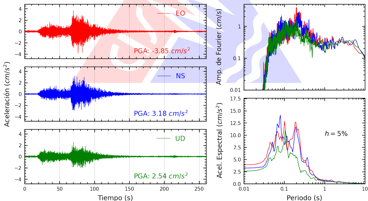
Figura A.18: Registros tiempo-historia, espectros de Fourier y de respuesta en las direcciones EO, NS y vertical de la estación INDEP. Sismo de Coracora, Parinacochas - Ayacucho del 2026-08-20, 13:00:16 (Hora local)
