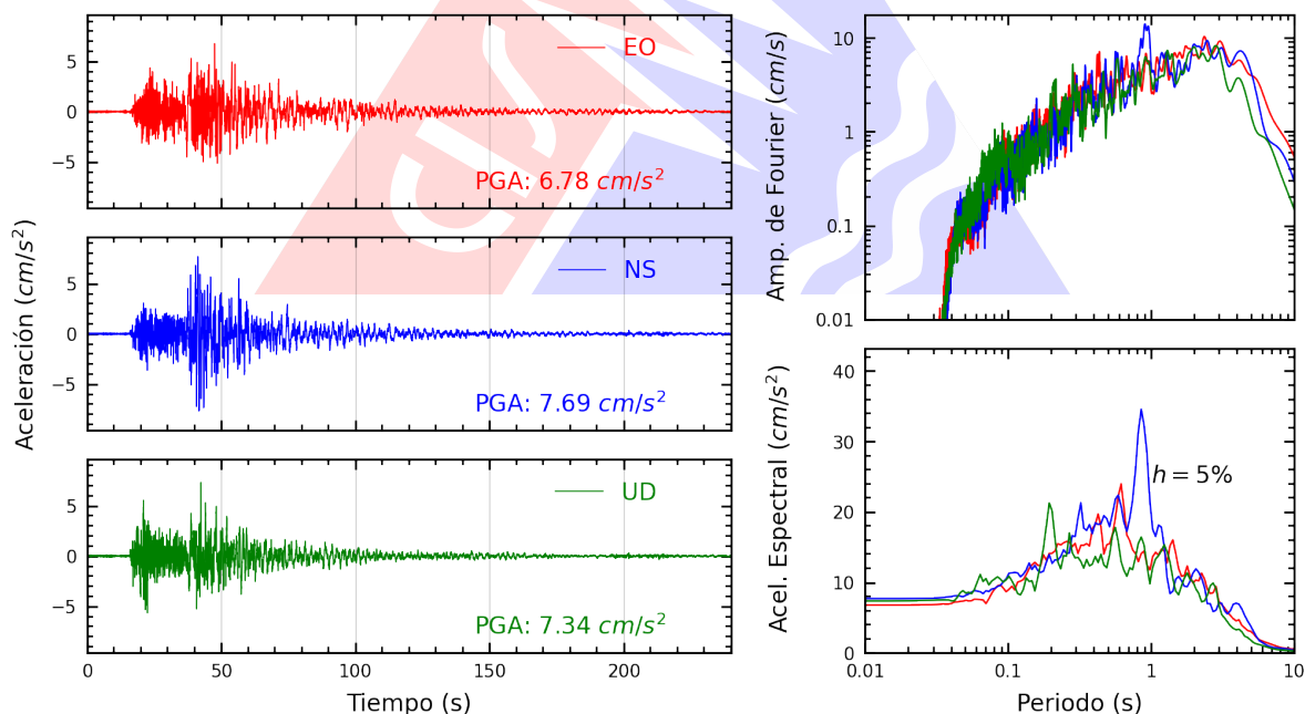
Figura A.4: Registros tiempo-historia, espectros de Fourier y de respuesta en las direcciones EO, NS y vertical de la estación SCAYA. Sismo de Coracora, Parinacochas - Ayacucho del 2026-08-20, 13:00:16 (Hora local)
