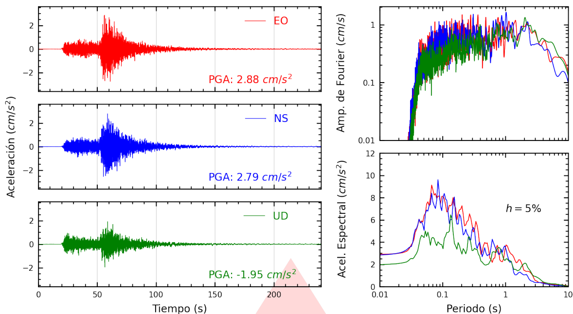
Figura A.31: Registros tiempo-historia, espectros de Fourier y de respuesta en las direcciones EO, NS y vertical de la estación UNSA2. Sismo de Coracora, Parinacochas - Ayacucho del 2026-08-20, 13:00:16 (Hora local)
