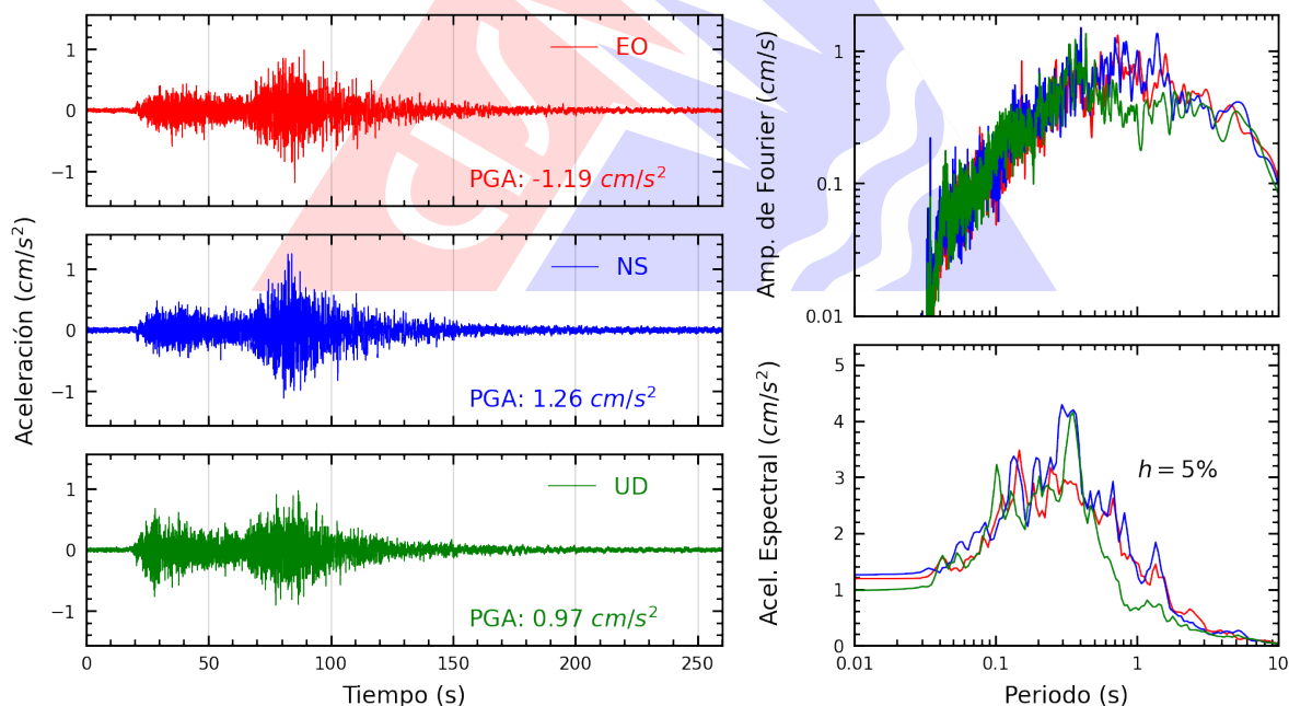
Figura A.54: Registros tiempo-historia, espectros de Fourier y de respuesta en las direcciones EO, NS y vertical de la estación BONDY. Sismo de Coracora, Parinacochas - Ayacucho del 2026-08-20, 13:00:16 (Hora local)
