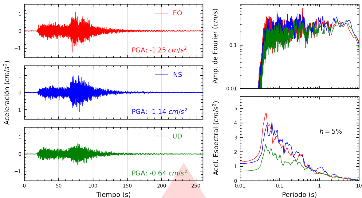
Figura A.55: Registros tiempo-historia, espectros de Fourier y de respuesta en las direcciones EO, NS y vertical de la estación UCSS. Sismo de Coracora, Parinacochas - Ayacucho del 2026-08-20, 13:00:16 (Hora local)
