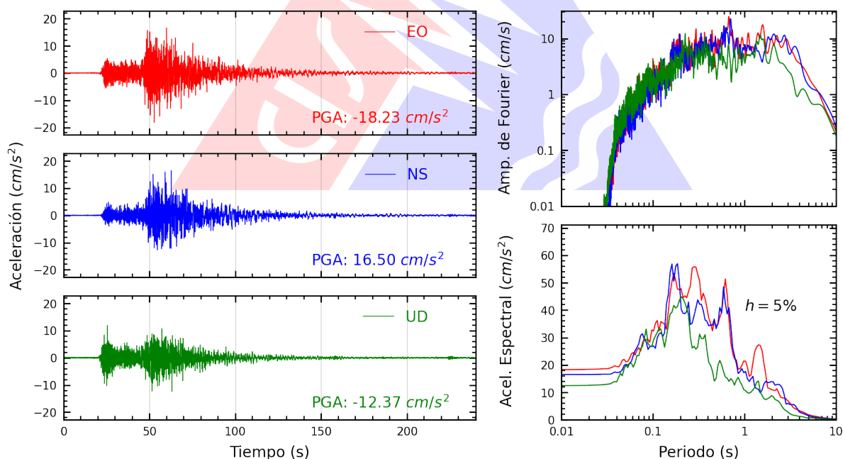
Figura A.2: Registros tiempo-historia, espectros de Fourier y de respuesta en las direcciones EO, NS y vertical de la estación SCICA. Sismo de Coracora, Parinacochas - Ayacucho del 2026-08-20, 13:00:16 (Hora local)
