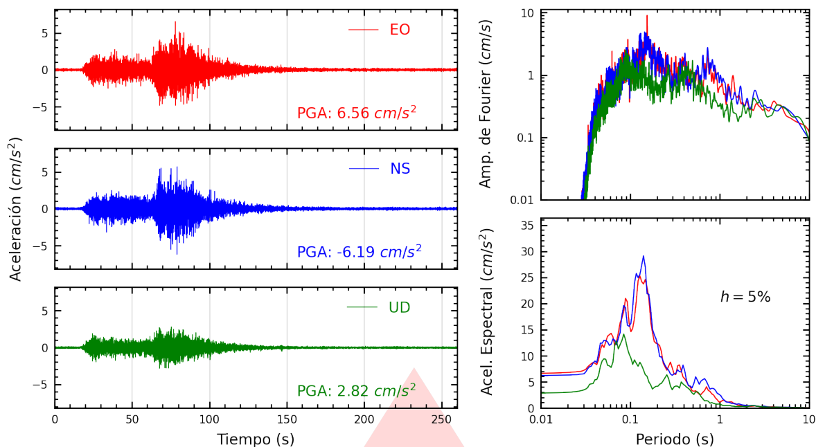
Figura A.7: Registros tiempo-historia, espectros de Fourier y de respuesta en las direcciones EO, NS y vertical de la estación USILM. Sismo de Coracora, Parinacochas - Ayacucho del 2026-08-20, 13:00:16 (Hora local)
