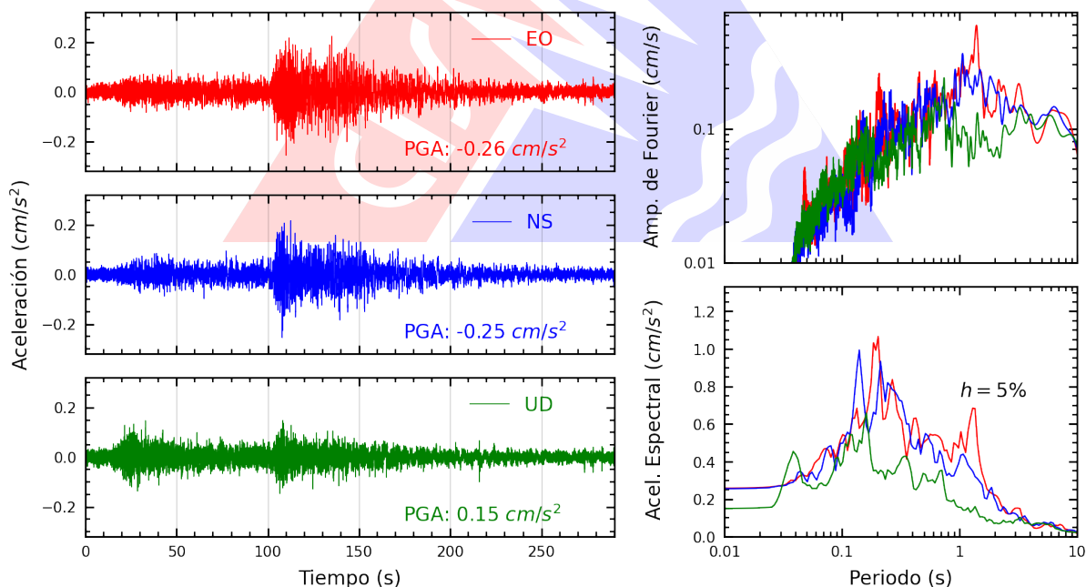
Figura A.60: Registros tiempo-historia, espectros de Fourier y de respuesta en las direcciones EO, NS y vertical de la estación UPAOT. Sismo de Coracora, Parinacochas - Ayacucho del 2026-08-20, 13:00:16 (Hora local)
