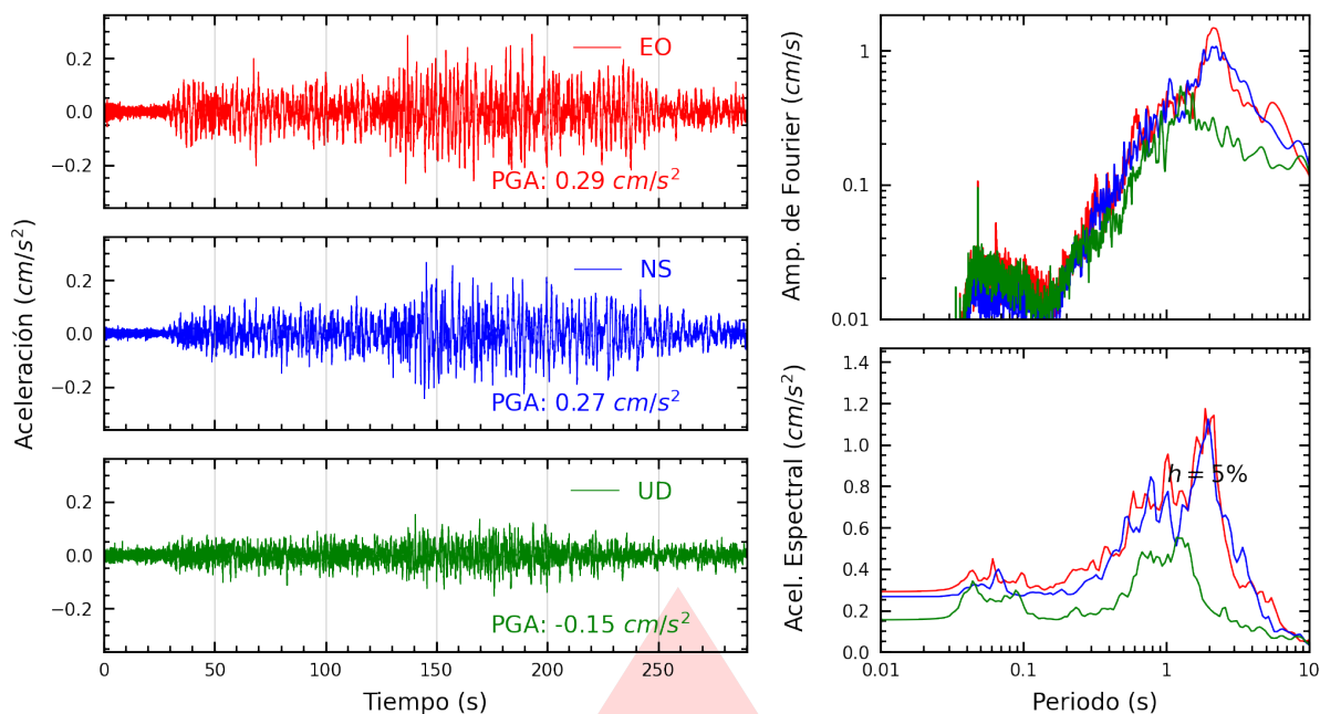
Figura A.59: Registros tiempo-historia, espectros de Fourier y de respuesta en las direcciones EO, NS y vertical de la estación UNC. Sismo de Coracora, Parinacochas - Ayacucho del 2026-08-20, 13:00:16 (Hora local)
