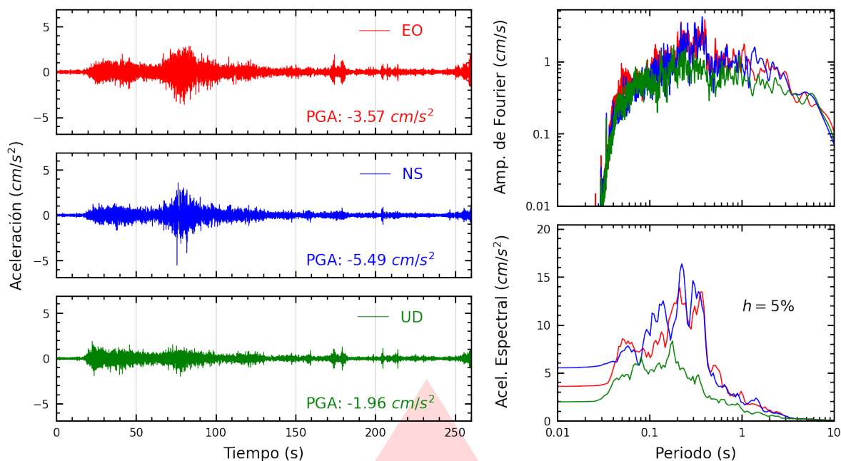
Figura A.9: Registros tiempo-historia, espectros de Fourier y de respuesta en las direcciones EO, NS y vertical de la estación SOBAR. Sismo de Coracora, Parinacochas - Ayacucho del 2026-08-20, 13:00:16 (Hora local)
