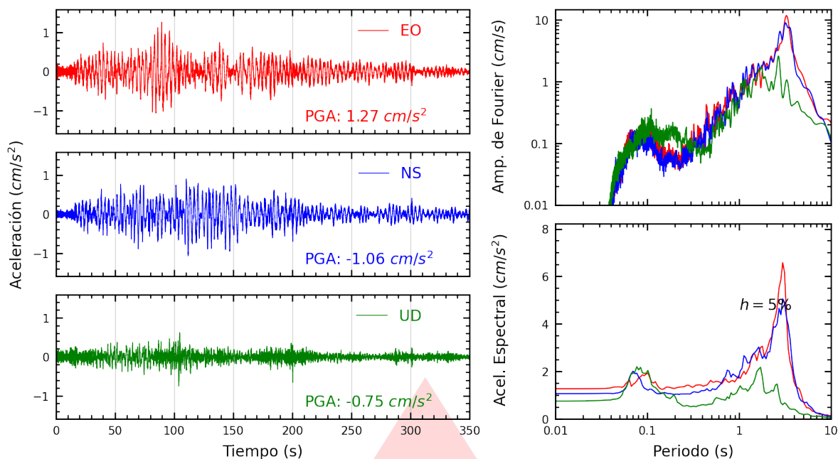
Figura A.53: Registros tiempo-historia, espectros de Fourier y de respuesta en las direcciones EO, NS y vertical de la estación UANCV. Sismo de Coracora, Parinacochas - Ayacucho del 2026-08-20, 13:00:16 (Hora local)
