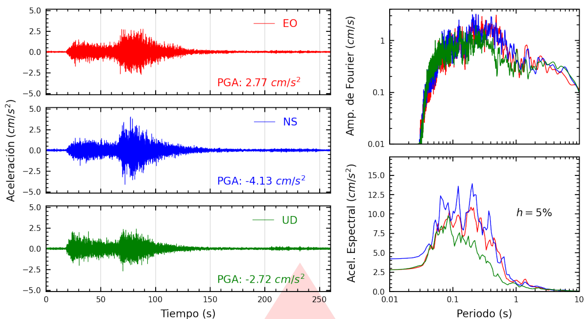
Figura A.17: Registros tiempo-historia, espectros de Fourier y de respuesta en las direcciones EO, NS y vertical de la estación SJLSC. Sismo de Coracora, Parinacochas - Ayacucho del 2026-08-20, 13:00:16 (Hora local)
