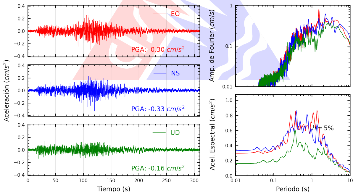
Figura A.58: Registros tiempo-historia, espectros de Fourier y de respuesta en las direcciones EO, NS y vertical de la estación UNASA. Sismo de Coracora, Parinacochas - Ayacucho del 2026-08-20, 13:00:16 (Hora local)
