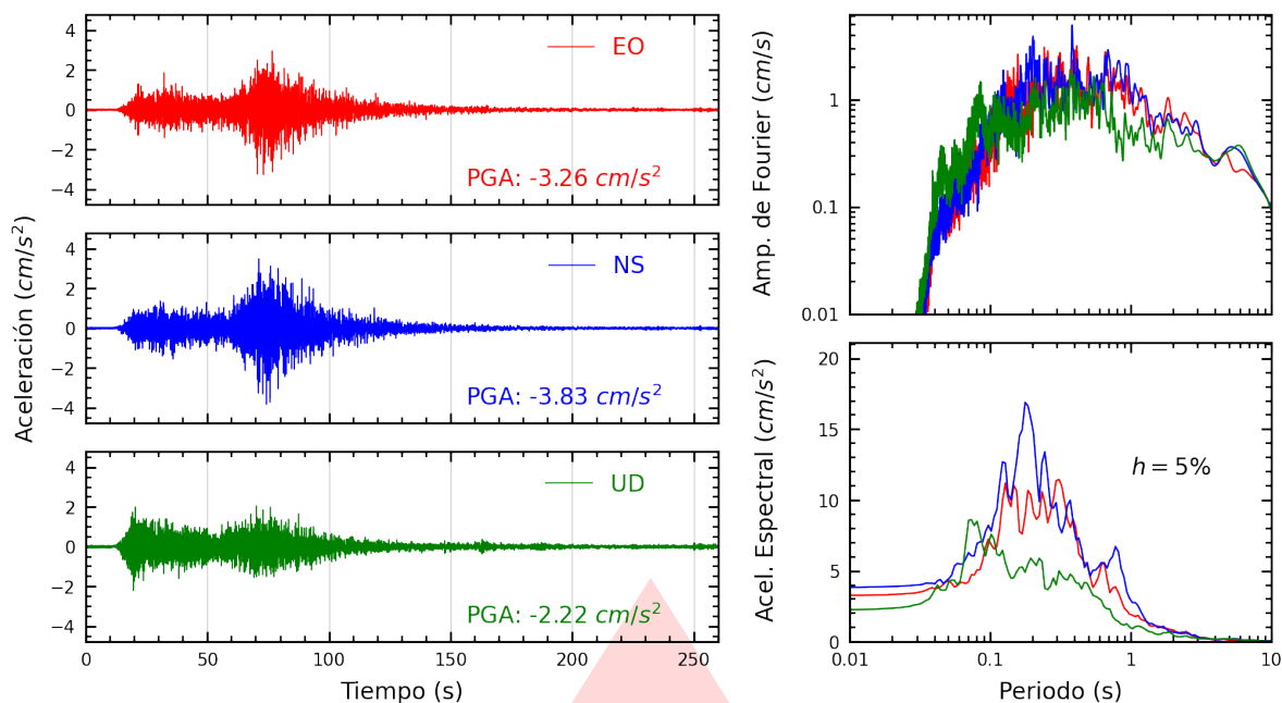
Figura A.19: Registros tiempo-historia, espectros de Fourier y de respuesta en las direcciones EO, NS y vertical de la estación SOCHO. Sismo de Coracora, Parinacochas - Ayacucho del 2026-08-20, 13:00:16 (Hora local)
