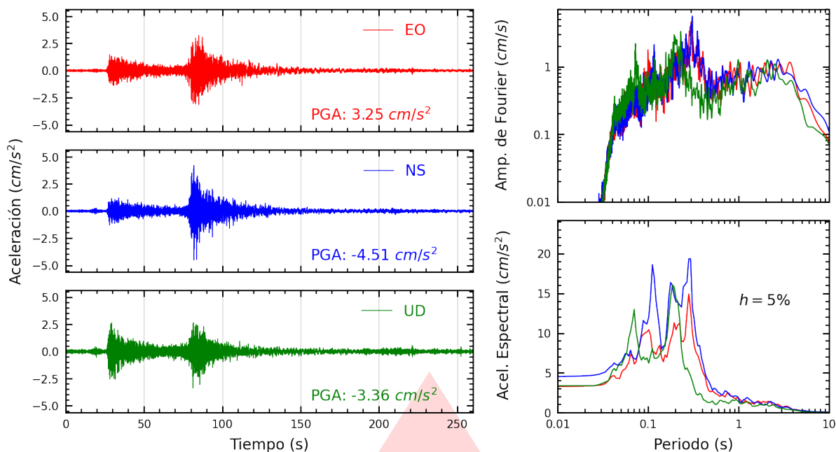
Figura A.13: Registros tiempo-historia, espectros de Fourier y de respuesta en las direcciones EO, NS y vertical de la estación SCTAC. Sismo de Coracora, Parinacochas - Ayacucho del 2026-08-20, 13:00:16 (Hora local)
