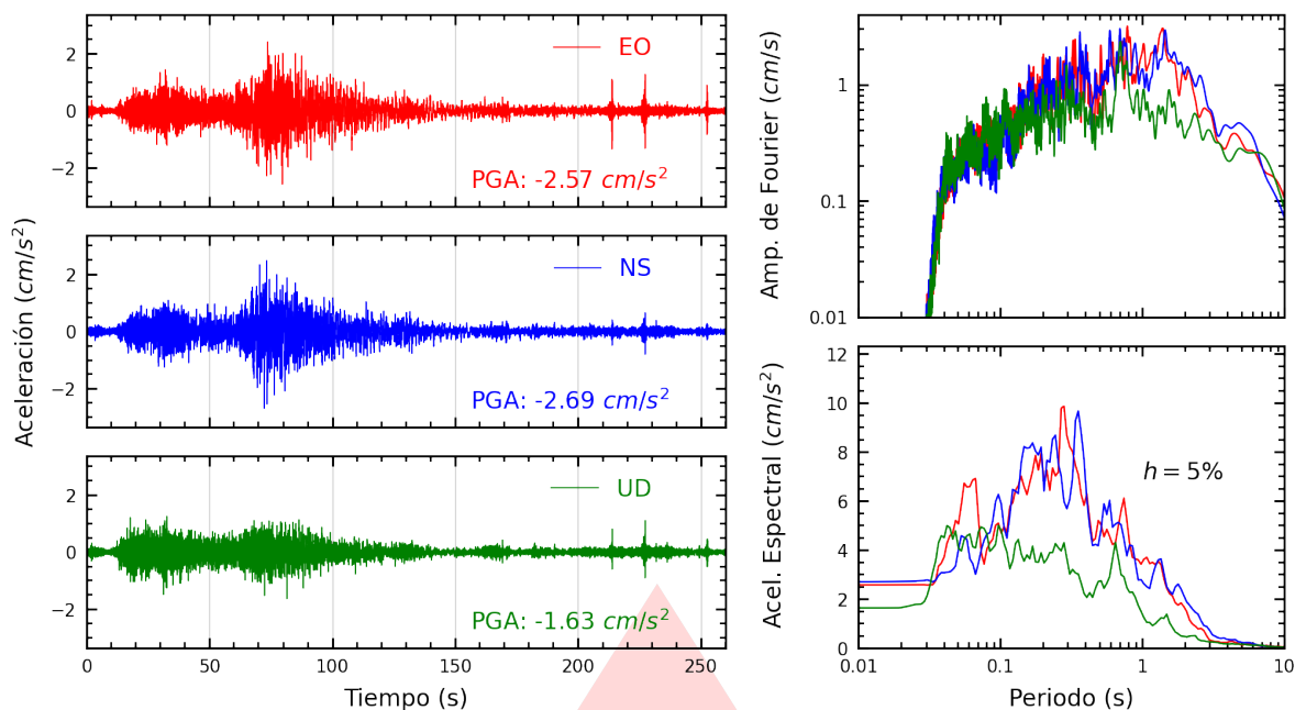
Figura A.33: Registros tiempo-historia, espectros de Fourier y de respuesta en las direcciones EO, NS y vertical de la estación PRADO. Sismo de Coracora, Parinacochas - Ayacucho del 2026-08-20, 13:00:16 (Hora local)
