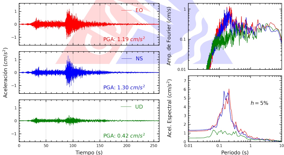
Figura A.52: Registros tiempo-historia, espectros de Fourier y de respuesta en las direcciones EO, NS y vertical de la estación UNAS. Sismo de Coracora, Parinacochas - Ayacucho del 2026-08-20, 13:00:16 (Hora local)
