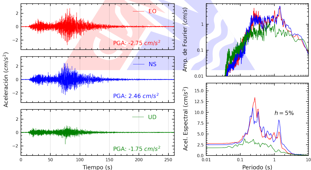
Figura A.32: Registros tiempo-historia, espectros de Fourier y de respuesta en las direcciones EO, NS y vertical de la estación DSML. Sismo de Coracora, Parinacochas - Ayacucho del 2026-08-20, 13:00:16 (Hora local)
