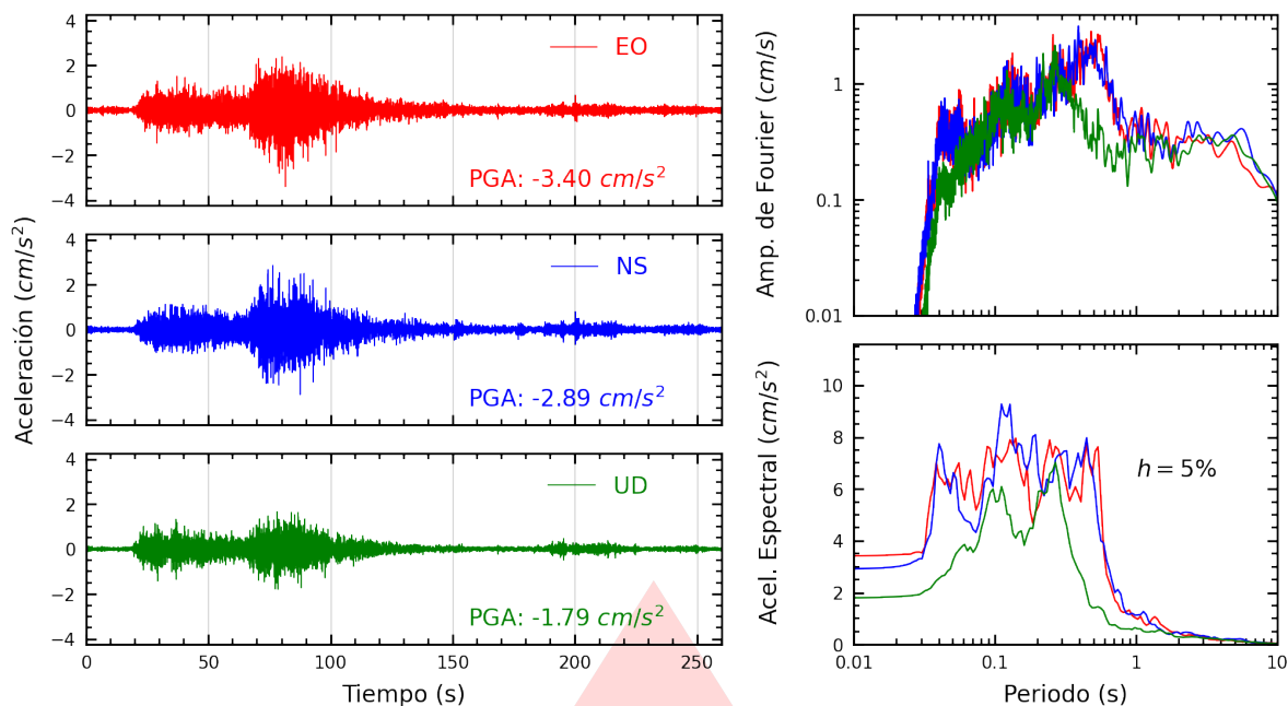
Figura A.23: Registros tiempo-historia, espectros de Fourier y de respuesta en las direcciones EO, NS y vertical de la estación OLIVO. Sismo de Coracora, Parinacochas - Ayacucho del 2026-08-20, 13:00:16 (Hora local)
