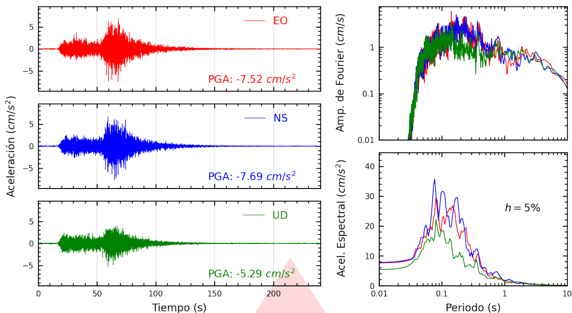
Figura A.5: Registros tiempo-historia, espectros de Fourier y de respuesta en las direcciones EO, NS y vertical de la estación ASIA. Sismo de Coracora, Parinacochas - Ayacucho del 2026-08-20, 13:00:16 (Hora local)
