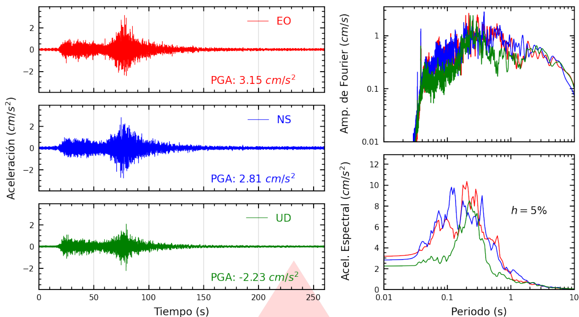
Figura A.27: Registros tiempo-historia, espectros de Fourier y de respuesta en las direcciones EO, NS y vertical de la estación UPCVI. Sismo de Coracora, Parinacochas - Ayacucho del 2026-08-20, 13:00:16 (Hora local)
