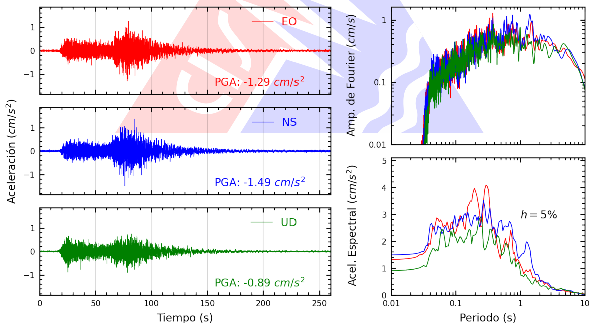
Figura A.48: Registros tiempo-historia, espectros de Fourier y de respuesta en las direcciones EO, NS y vertical de la estación BORJA. Sismo de Coracora, Parinacochas - Ayacucho del 2026-08-20, 13:00:16 (Hora local)
