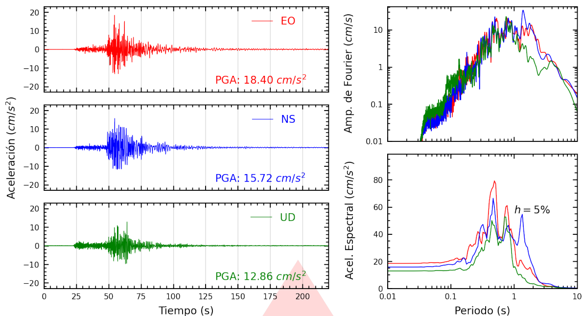
Figura A.1: Registros tiempo-historia, espectros de Fourier y de respuesta en las direcciones EO, NS y vertical de la estación SCCUS. Sismo de Coracora, Parinacochas - Ayacucho del 2026-08-20, 13:00:16 (Hora local)
