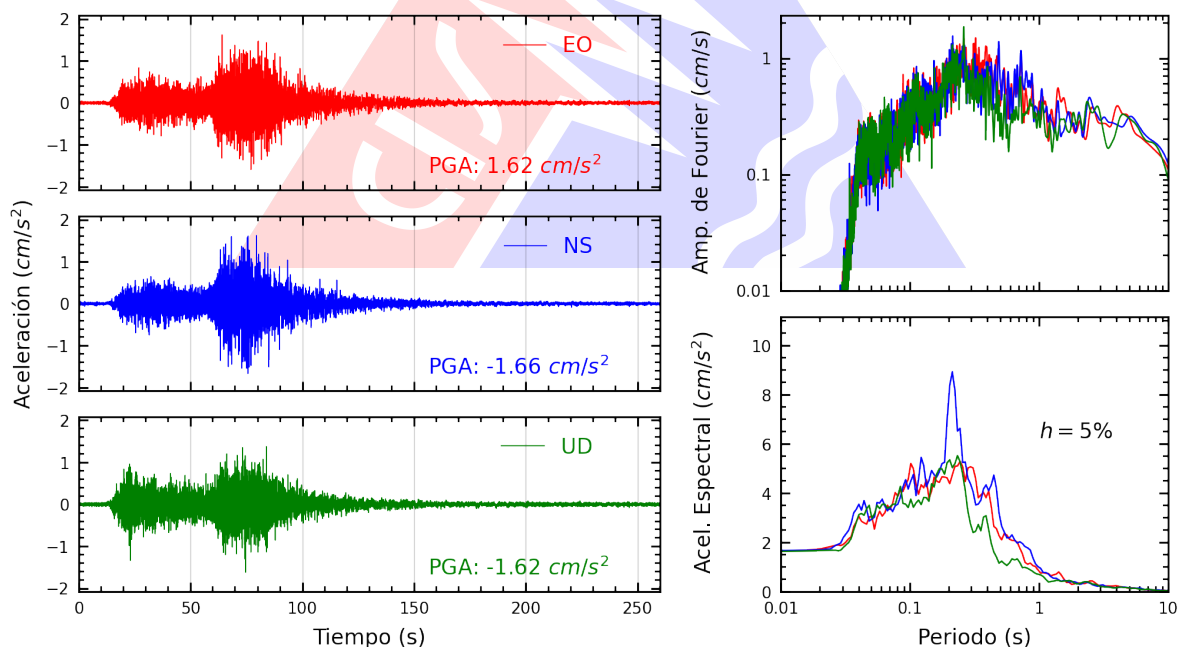
Figura A.44: Registros tiempo-historia, espectros de Fourier y de respuesta en las direcciones EO, NS y vertical de la estación USMP. Sismo de Coracora, Parinacochas - Ayacucho del 2026-08-20, 13:00:16 (Hora local)
