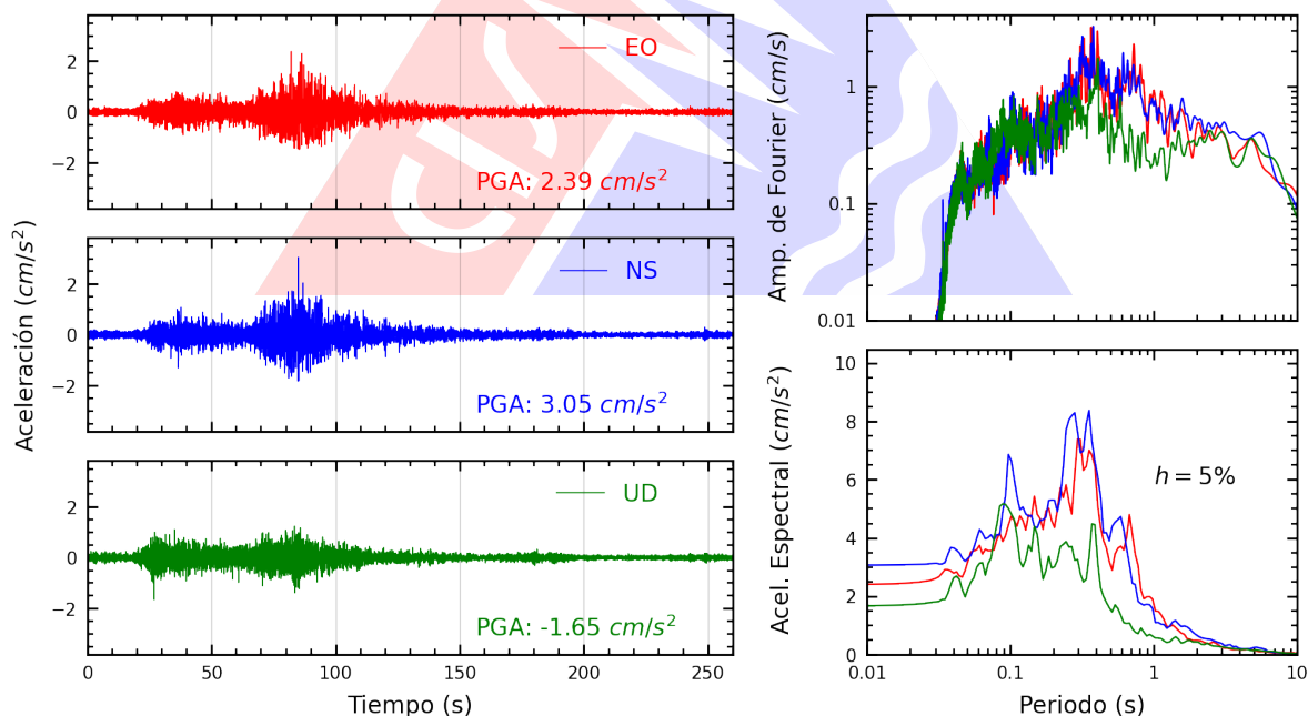
Figura A.28: Registros tiempo-historia, espectros de Fourier y de respuesta en las direcciones EO, NS y vertical de la estación MADRE. Sismo de Coracora, Parinacochas - Ayacucho del 2026-08-20, 13:00:16 (Hora local)
