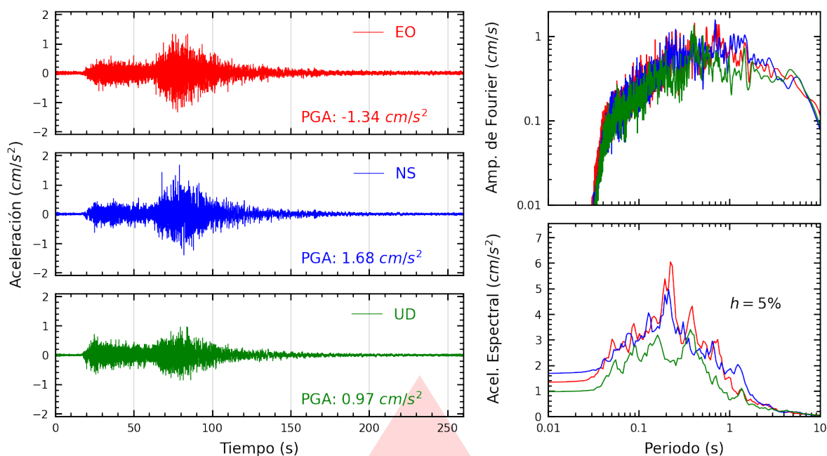
Figura A.43: Registros tiempo-historia, espectros de Fourier y de respuesta en las direcciones EO, NS y vertical de la estación INICT. Sismo de Coracora, Parinacochas - Ayacucho del 2026-08-20, 13:00:16 (Hora local)
