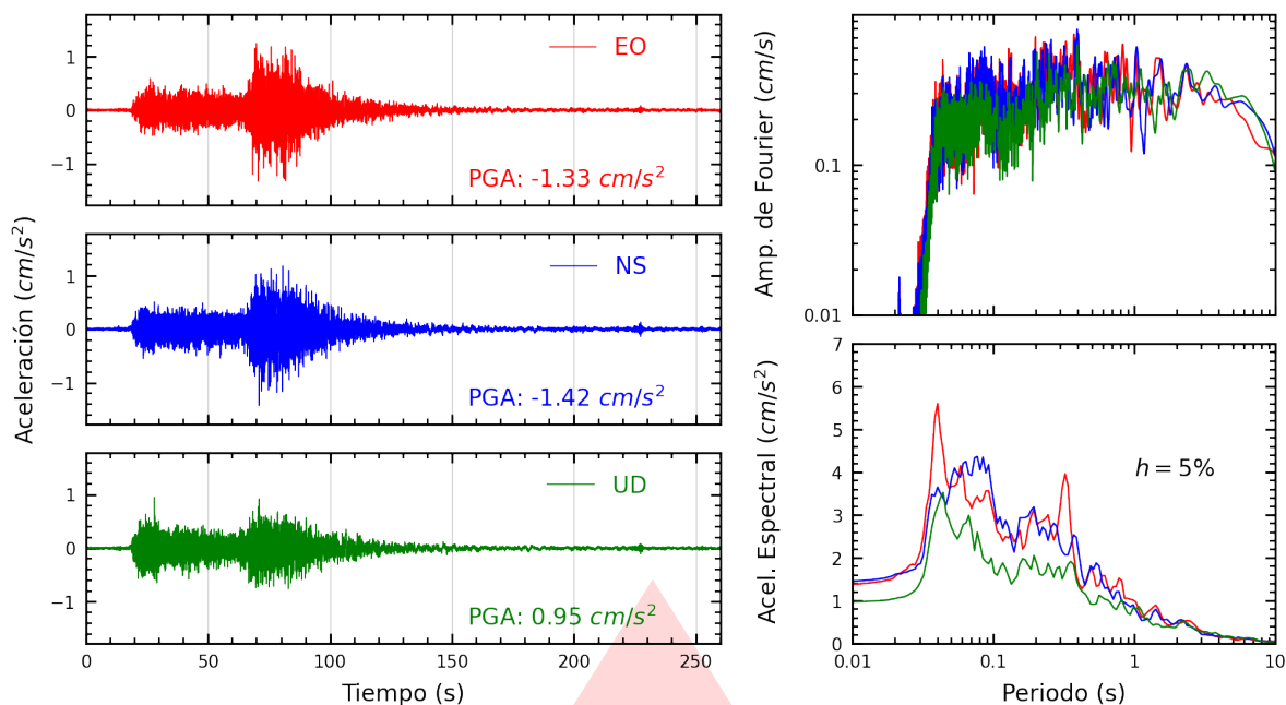
Figura A.51: Registros tiempo-historia, espectros de Fourier y de respuesta en las direcciones EO, NS y vertical de la estación SJLCE. Sismo de Coracora, Parinacochas - Ayacucho del 2026-08-20, 13:00:16 (Hora local)
