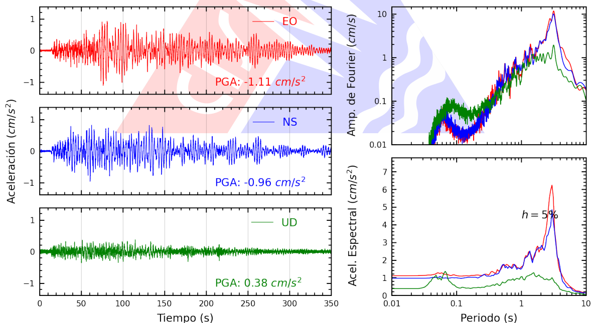
Figura A.56: Registros tiempo-historia, espectros de Fourier y de respuesta en las direcciones EO, NS y vertical de la estación UNAJ. Sismo de Coracora, Parinacochas - Ayacucho del 2026-08-20, 13:00:16 (Hora local)
