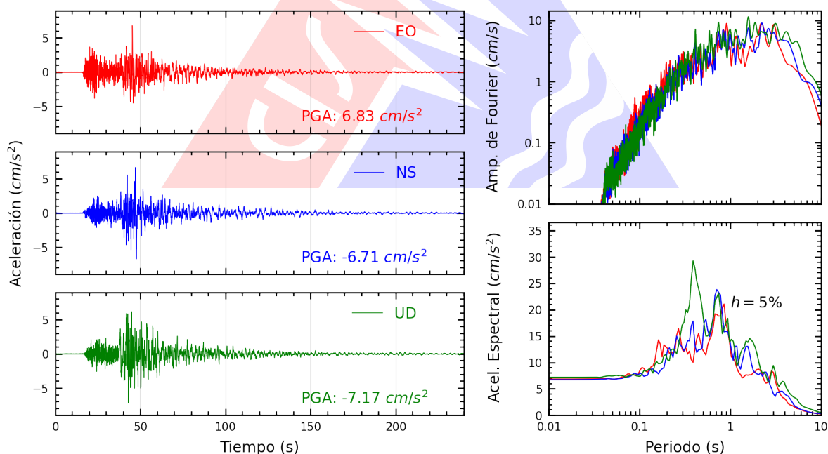
Figura A.6: Registros tiempo-historia, espectros de Fourier y de respuesta en las direcciones EO, NS y vertical de la estación UNSCH. Sismo de Coracora, Parinacochas - Ayacucho del 2026-08-20, 13:00:16 (Hora local)
