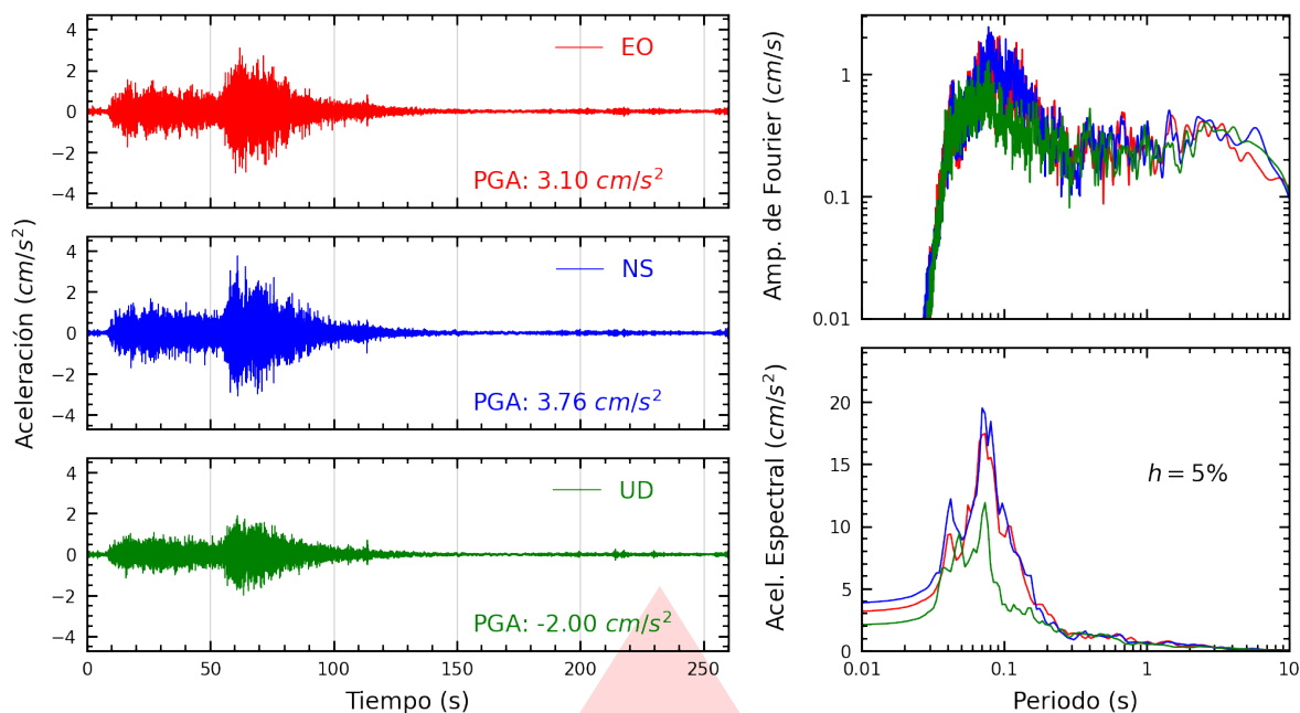
Figura A.21: Registros tiempo-historia, espectros de Fourier y de respuesta en las direcciones EO, NS y vertical de la estación JOSEO. Sismo de Coracora, Parinacochas - Ayacucho del 2026-08-20, 13:00:16 (Hora local)
