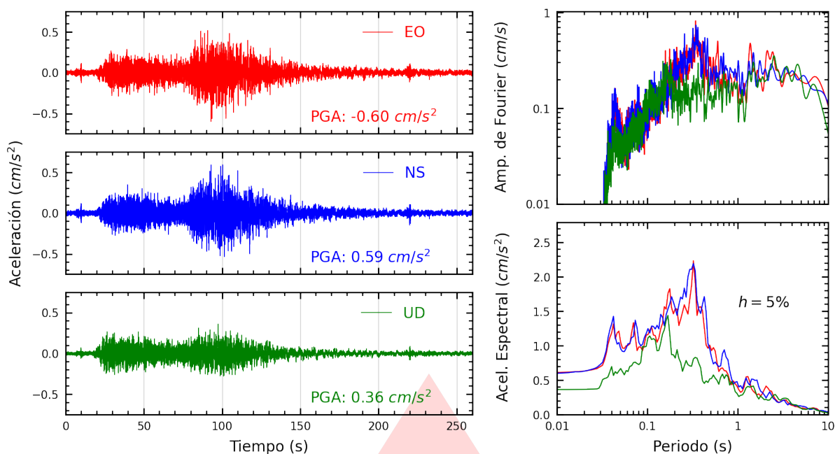
Figura A.57: Registros tiempo-historia, espectros de Fourier y de respuesta en las direcciones EO, NS y vertical de la estación UNAB. Sismo de Coracora, Parinacochas - Ayacucho del 2026-08-20, 13:00:16 (Hora local)
